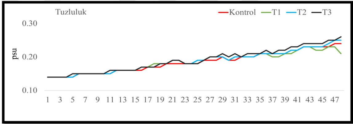
Şekil 4.7 Deney süresince tuzluluk konsantrasyonlarının değişimi
