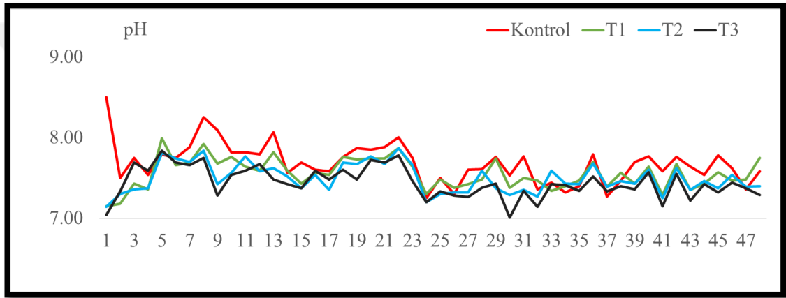
Şekil 4.5 Deney süresince pH değerinin değişimi
