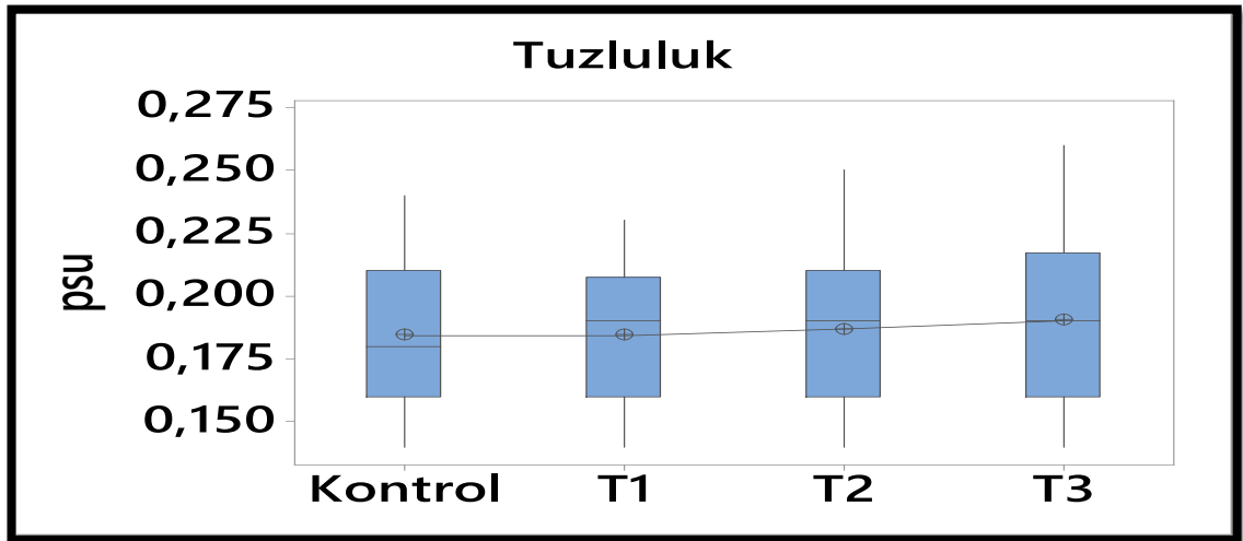
Şekil 4.8 Deney süresince sudaki tuzluluk konsantrasyonlarının değerinin değişiminin kutu grafiği ile gösterimi
