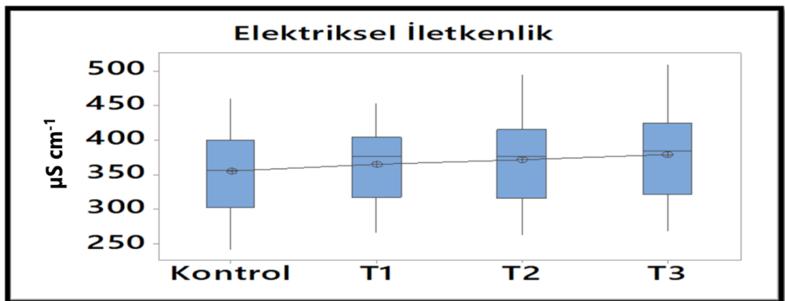
Şekil 4.10 Deneme süresince sudaki elektriksel iletkenlik değeri­nin değışiminin kutu grafiđi ile gösterimi
