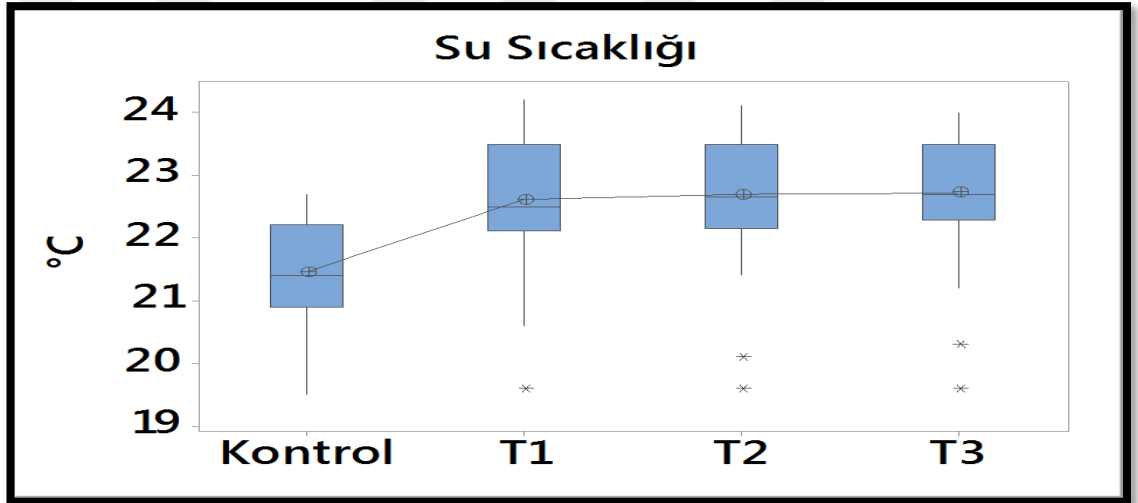
Şekil 4.2 Deney süresince su sıcaklığının değişiminin kutu grafiği ile gösterimi
