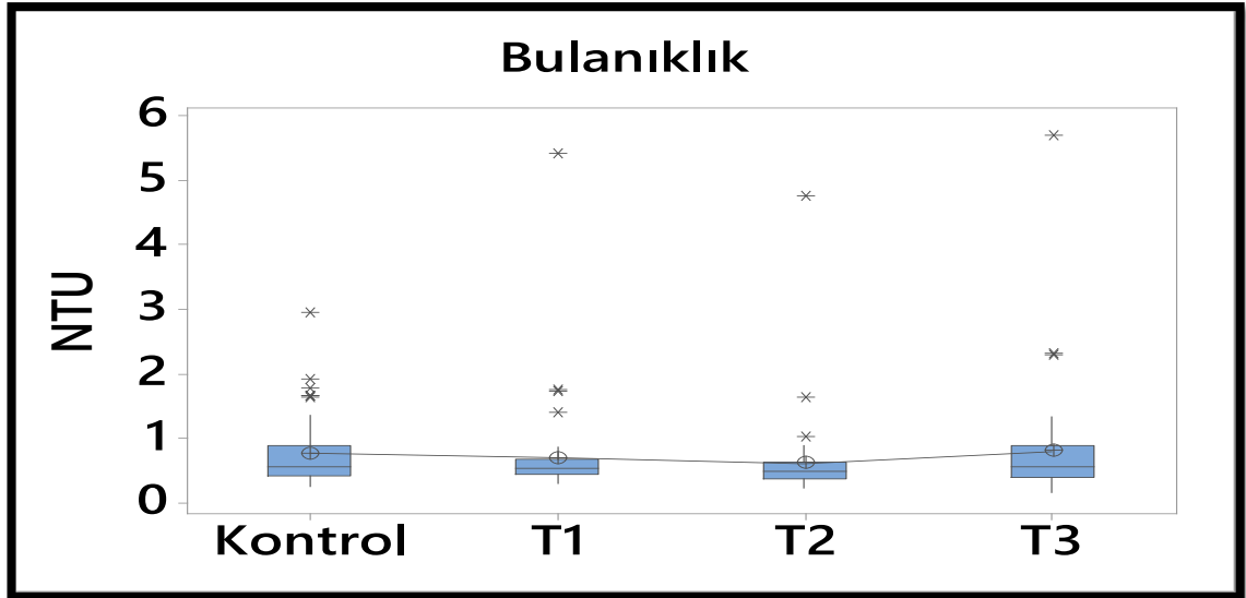
Şekil 4.12 Deney süresince sudaki bulanıklık konsantrasyonlarının değişiminin kutu grafiği ile gösterimi
