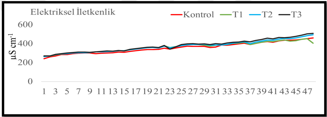
Şekil 4.9 Deney süresince EC değeri­nin değışimi
