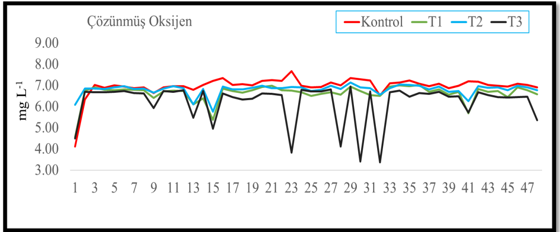
Şekil 4.3 Deney süresince suda çözünmüş oksijen konsantrasyonu değişimi
