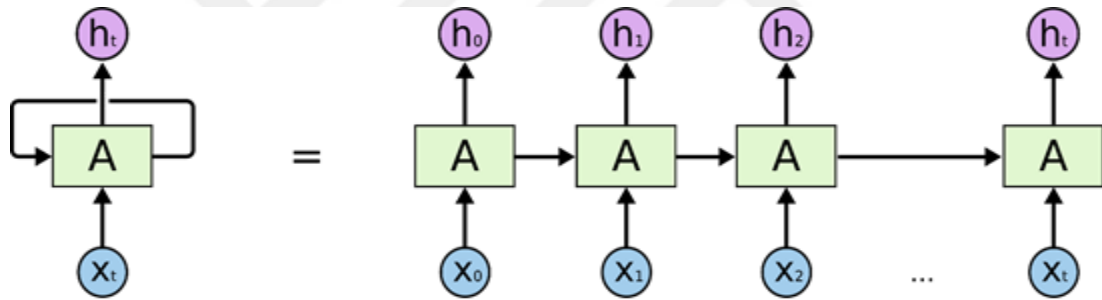
Şekil 6.8 RNN Ağ Modeli[55].
