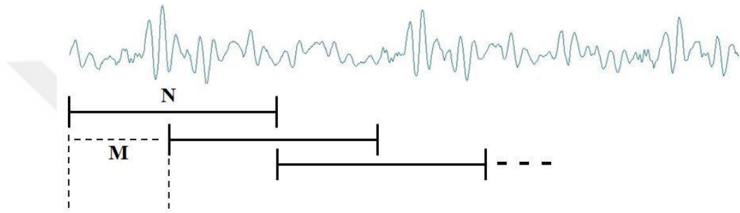
Şekil 7.3 Bir Konuşma İşaretinin Çerçeveleme İşlemi.
