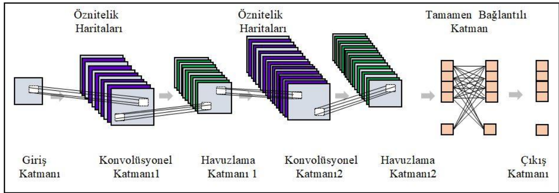
Şekil 6.11 CNN Mimari Yapısı [60].
