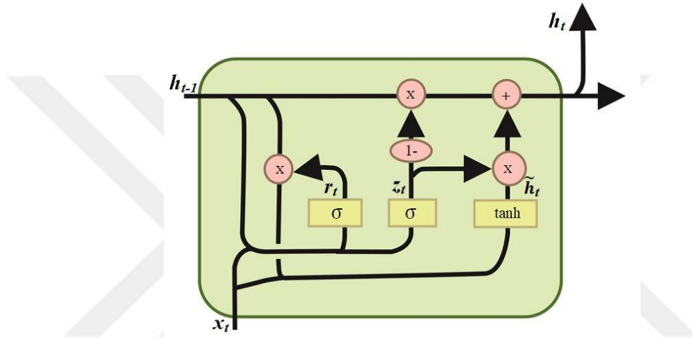
Şekil 7.7 GRU Hücre Mimarisi [73].
