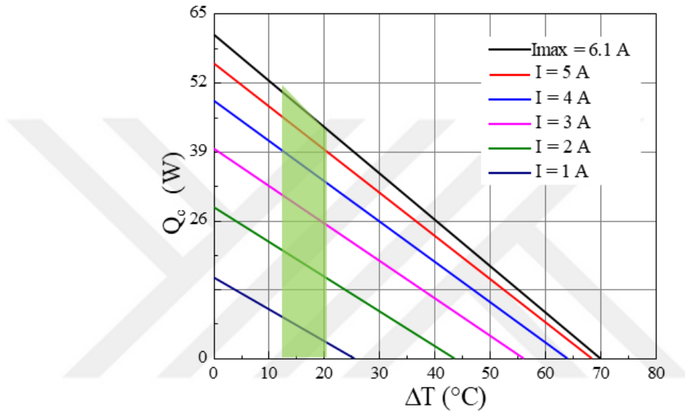
Şekil 3.1 : TEC'in Q_c - \Delta T Performans Eğrileri Grafiği
