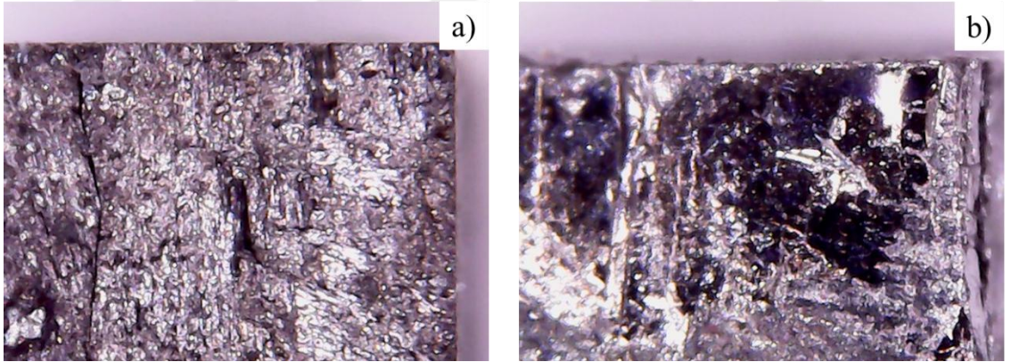
Şekil 4.21 : TEC İçerisinde Bulunan a) p-tipi ve b) n-tipi Yarı İletkenlerin x1000 Büyütmeli Mikroskop Görüntüsü Kaynak: (Bozkurt, 2020)
