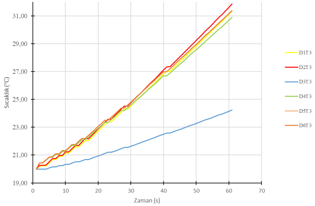
Şekil B.32 : Tüm Deney Düzenekleri T3 0-60 s Aralığı Sıcaklık Zaman Grafiği (Ortam Sıcaklığı 20°C, Bağıl Nem %50)
