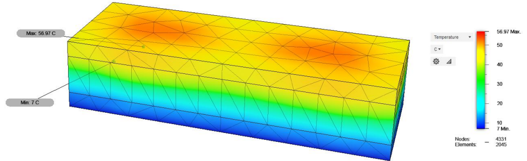
Şekil 4.4 : D4 TEC'in Termal Analizi
