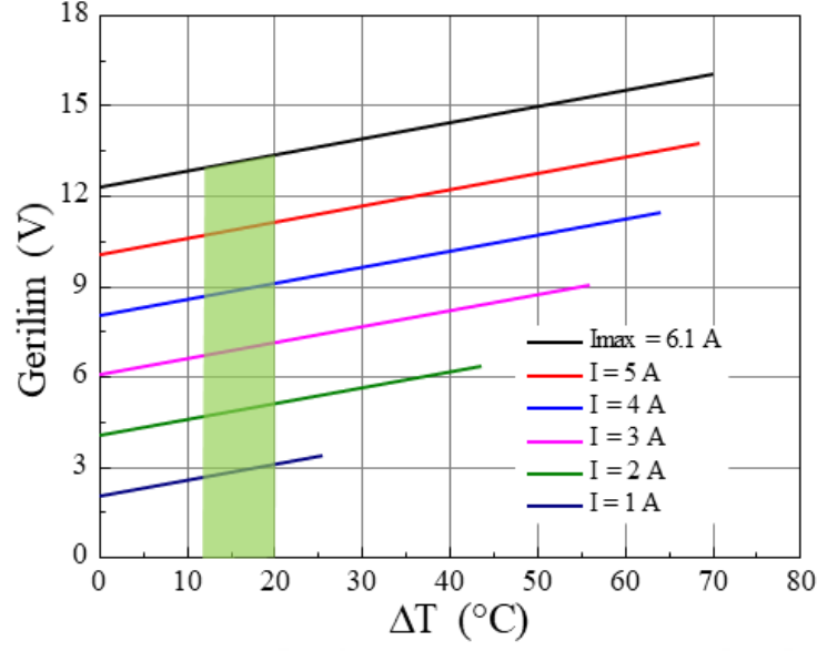
Şekil 3.2 : TEC'in V- \Delta T Performans Eğrileri Grafiği
