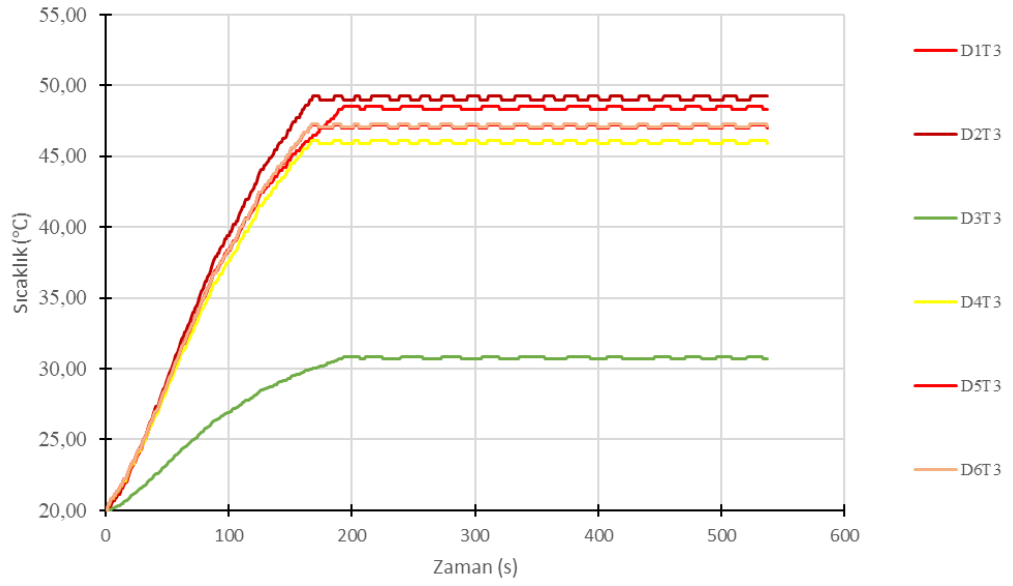
Şekil B.31 : Tüm Deney Düzenekleri T3 0-500 s Aralığı Sıcaklık Zaman Grafiği (Ortam Sıcaklığı 20°C, Bağıl Nem %50)
