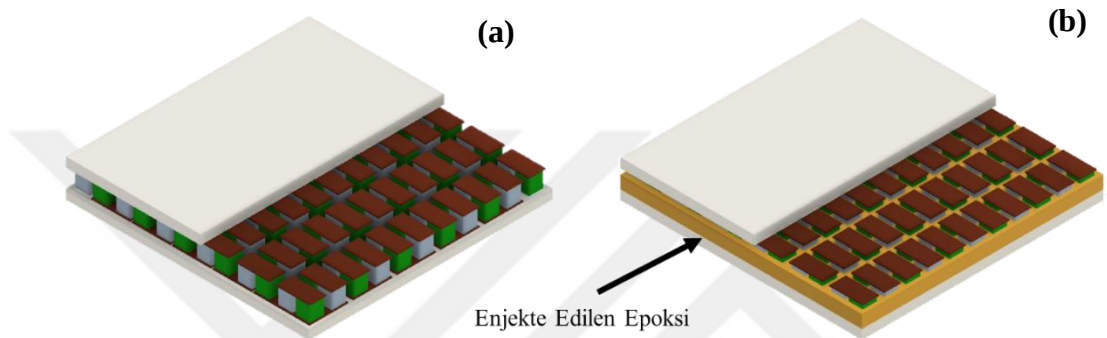
Şekil 3.9 : a) Standart TEC ile b) Epoksi Enjekte Edilen TEC'in 3 Boyutlu Gösterimi Kaynak: (Bozkurt, 2020)
