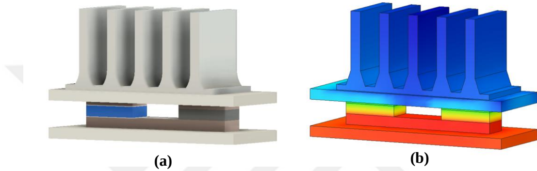
Şekil 3.6 : a) TEM p-n Çifti 3 Boyutlu Çizimi b) p-n Çifti 3 Boyutlu Termal Analizi Kaynak: (Bozkurt, 2020)
