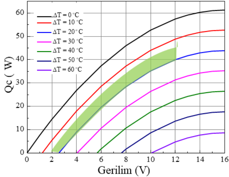
Şekil 3.3 : TEC'in Q_c -V Performans Eğrileri Grafiği
