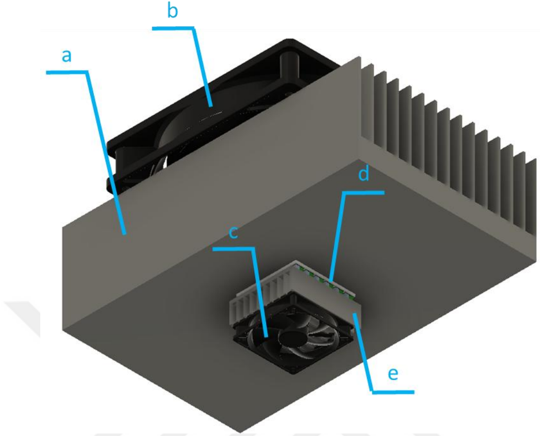
Şekil 3.11 : Soğutucu Ünite Grubu 3 Boyutlu Model Tasarımı
