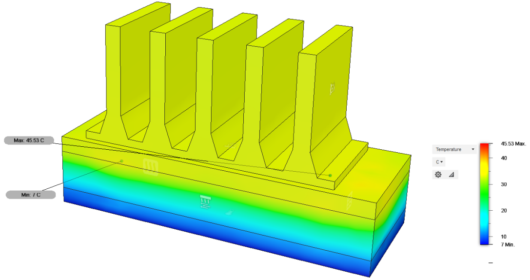
Şekil 4.9 : Alüminyum Blok Eklenmiş D3 TEC'in Termal Analizi
