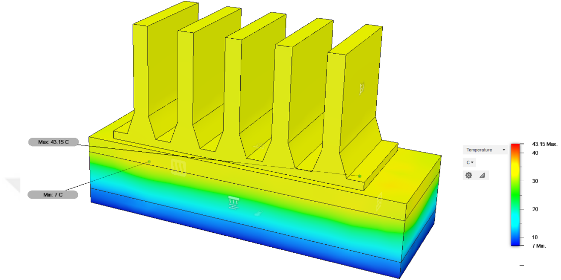
Şekil 4.11 : Alüminyum Blok Eklenmiş D5 TEC'in Termal Analizi
