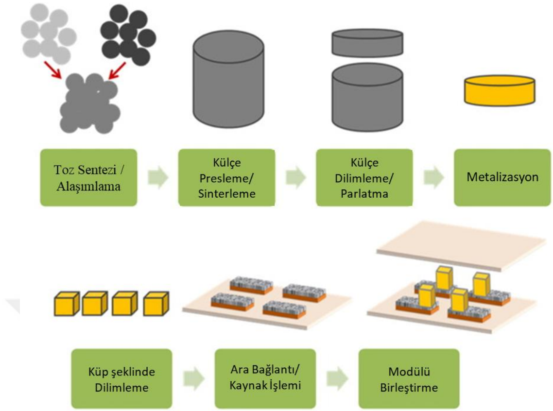
Şekil 2.6 : TEM üretimi süreç şeması
