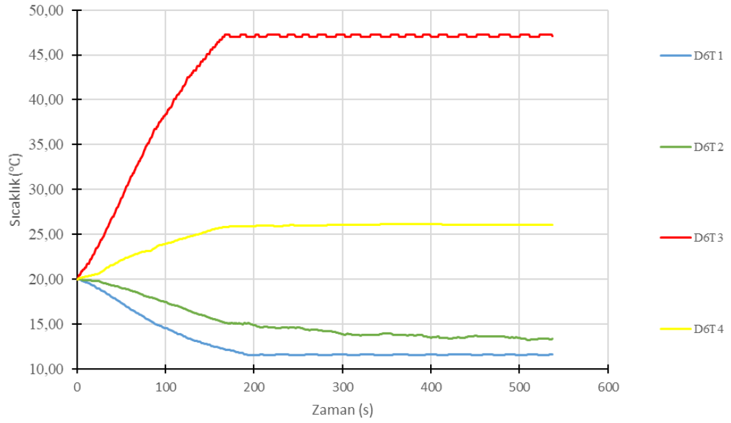
Şekil B.21 : D6 0-500 s Aralığı Sıcaklık Zaman Grafiği (Ortam Sıcaklığı 20°C, Bağlı Nem %50 Havanın Termal İletkenlik Katsayısı 0,05 W/m.K)
