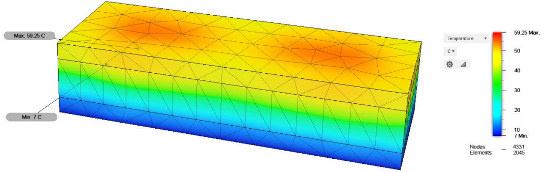
Şekil 4.3 : D3 TEC'in Termal Analizi
