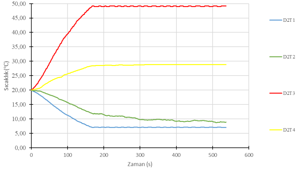
Şekil B.5 : D2 0-500 s Aralığı Sıcaklık Zaman Grafiği (Ortam Sıcaklığı 20°C, Bağlı Nem %50 Havanın Termal İletkenlik Katsayısı 0,01 W/m.K)
