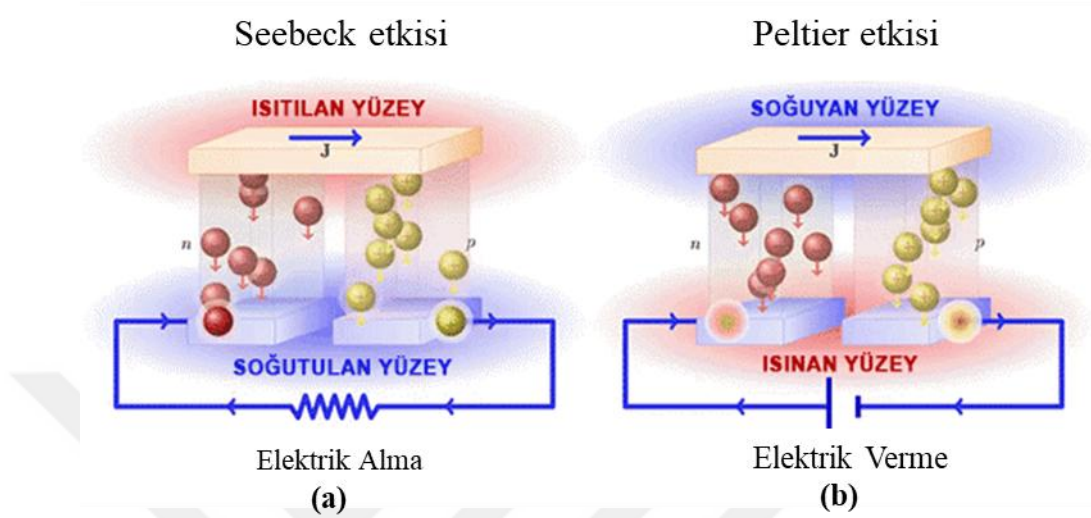
Şekil 2.1 : a) TEG ve b) TEC Gösterimi
