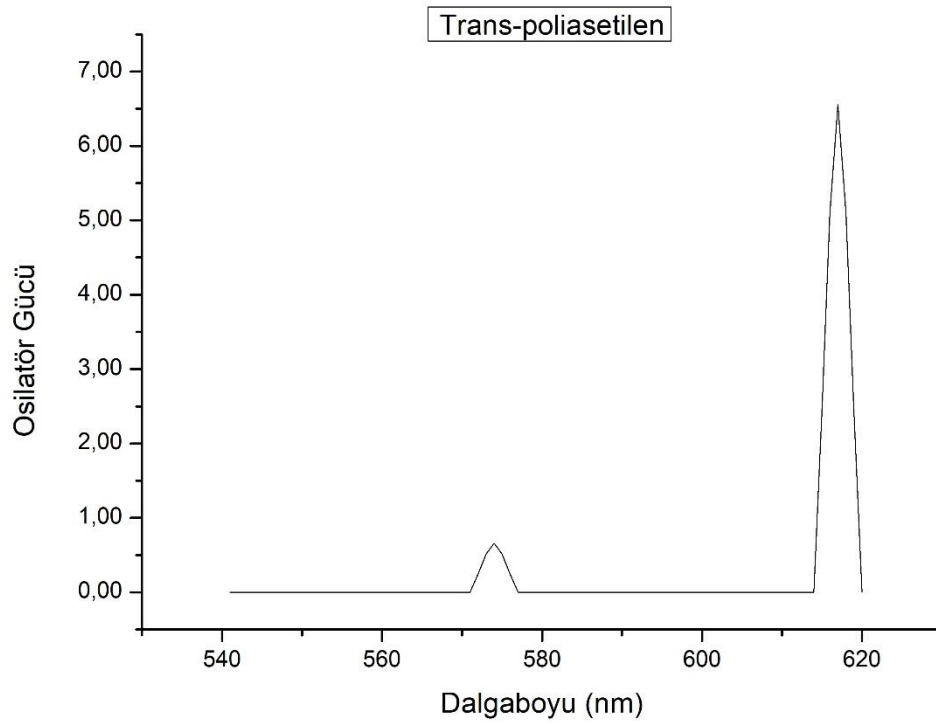
Şekil 4.5. TD-DFT/6-31G*(B3LYP) (n=80) ile Hesaplanmış Osilatör Gücü Grafiği
