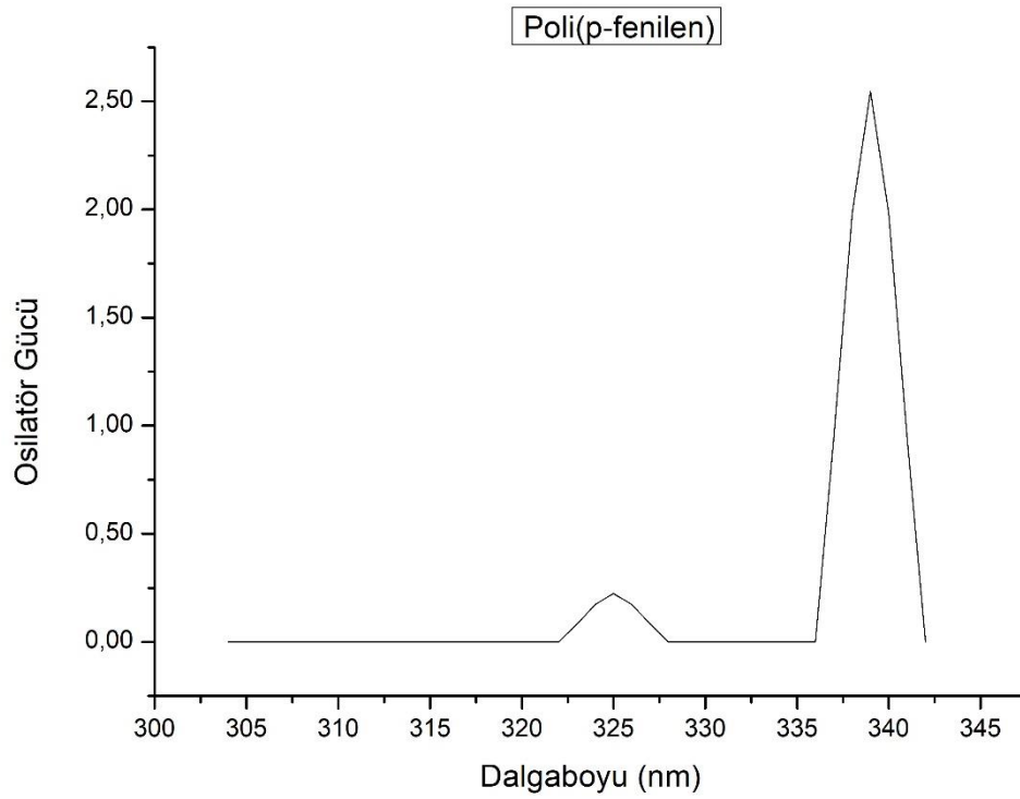
Şekil 4.20. TD-DFT/6-31G*(B3LYP) (n=12) ile Hesaplanmış Osilatör Gücü Grafiği
