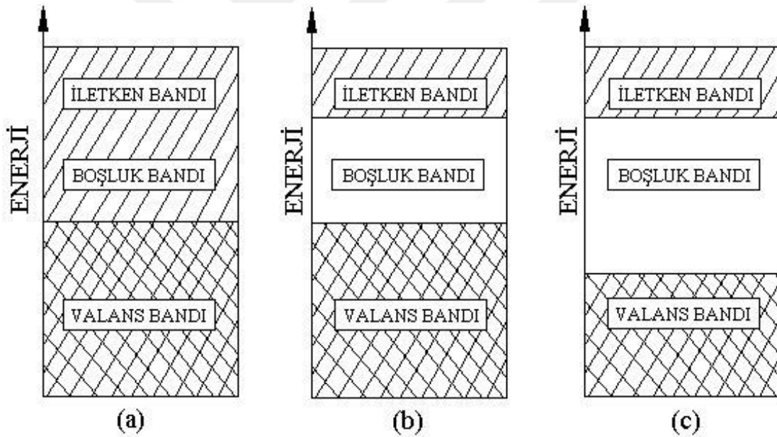
Şekil 1-1. Bant Aralığı Teorisi
