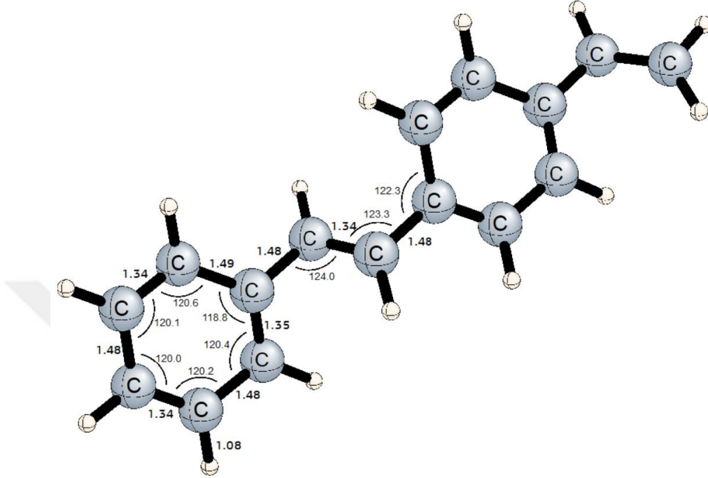
Şekil 4.21. UFF ile Optimize Edilmiş Poli(p-fenilen vinilen) (n=2)
