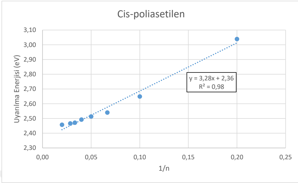
Şekil 4.8. TD-DFT/6-31G*(B3LYP) ile Hesaplanmış Uyarılma Enerjileri
