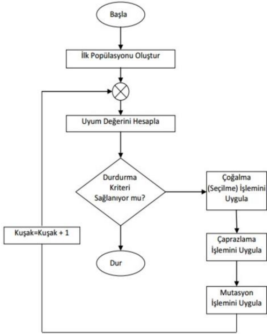
Şekil 3. 12 Genetik algoritmanın işleyişi
