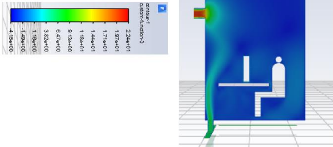
Şekil 3.6. Tabandan soğutma sistemi, cereyan etkisi dağılımı
