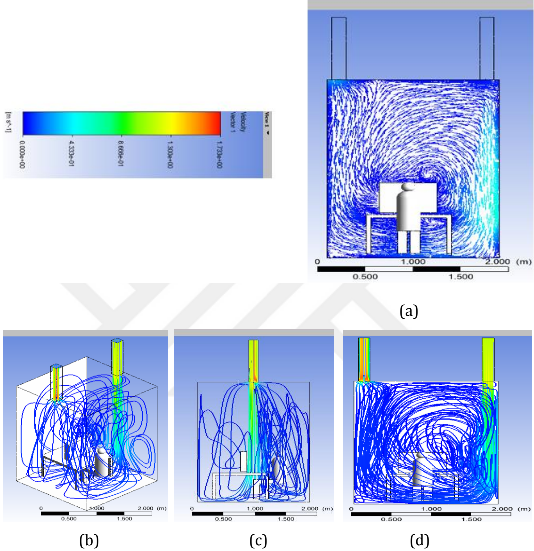
Şekil 3.17. Tavandan soğutulan mahal, mahal, hız dağılımı, vektörel (a) & çizgisel (b), (c), (d) gösterim
