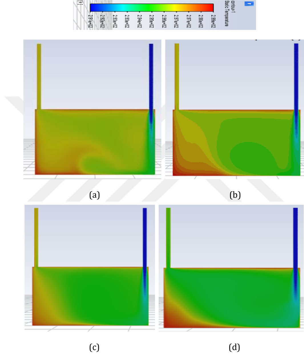
Şekil 2.15. Düşük ağ (a), ortalama yüksek ağ (b), yüksek ağ (c), çok yüksek ağ(d) yapılı modeller, sıcaklık dağılımı
