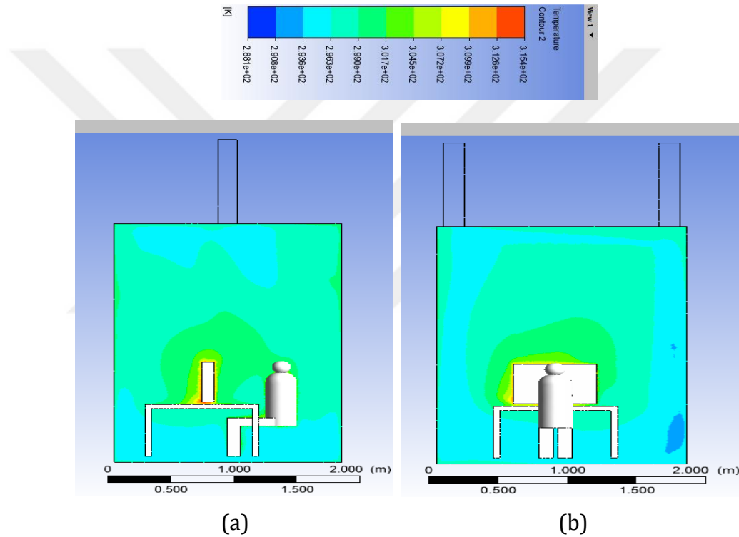
Şekil 3.15. Tavandan soğutulan mahal, sıcaklık dağılımı, kontur gösterimi
