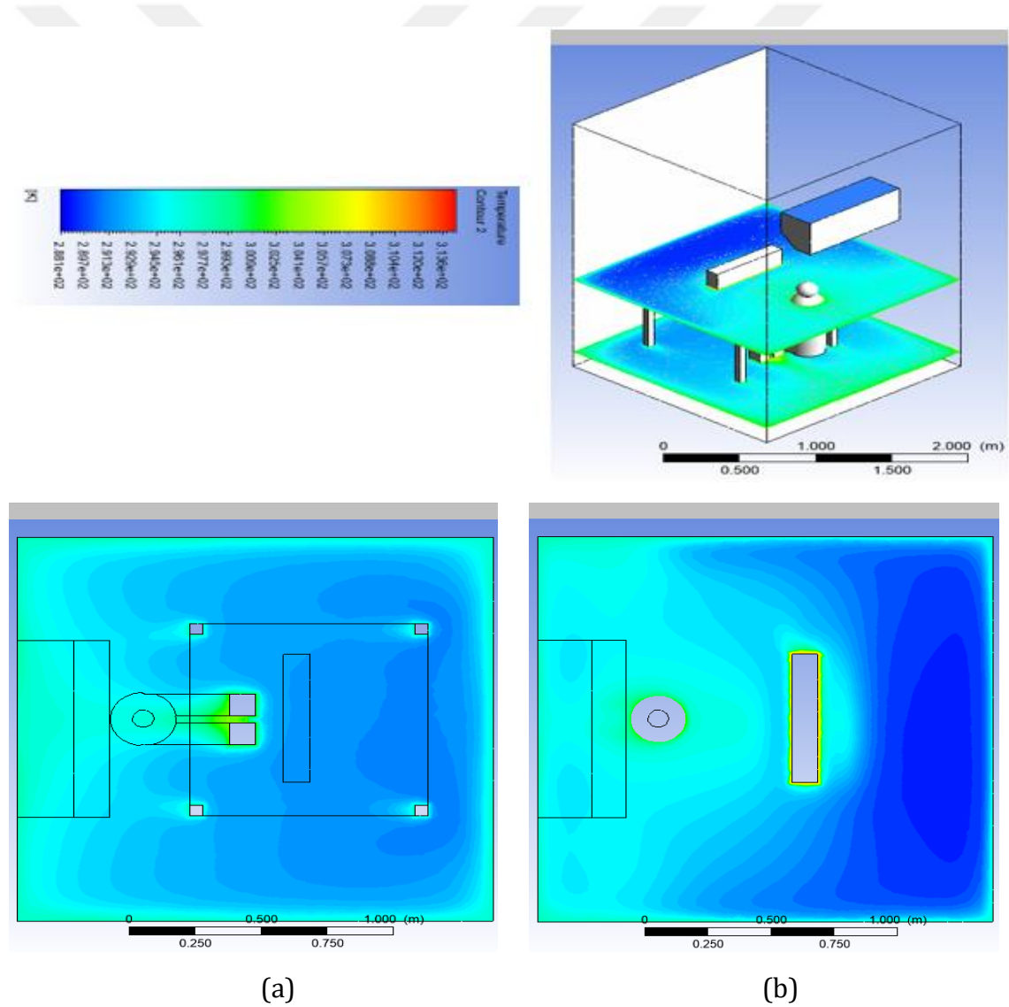
Şekil 3.9. Klima ile soğutulan, 0.1m (a) ve 1.1m (b) kesitlerdeki sıcaklık dağılımı, kontur gösterimi
