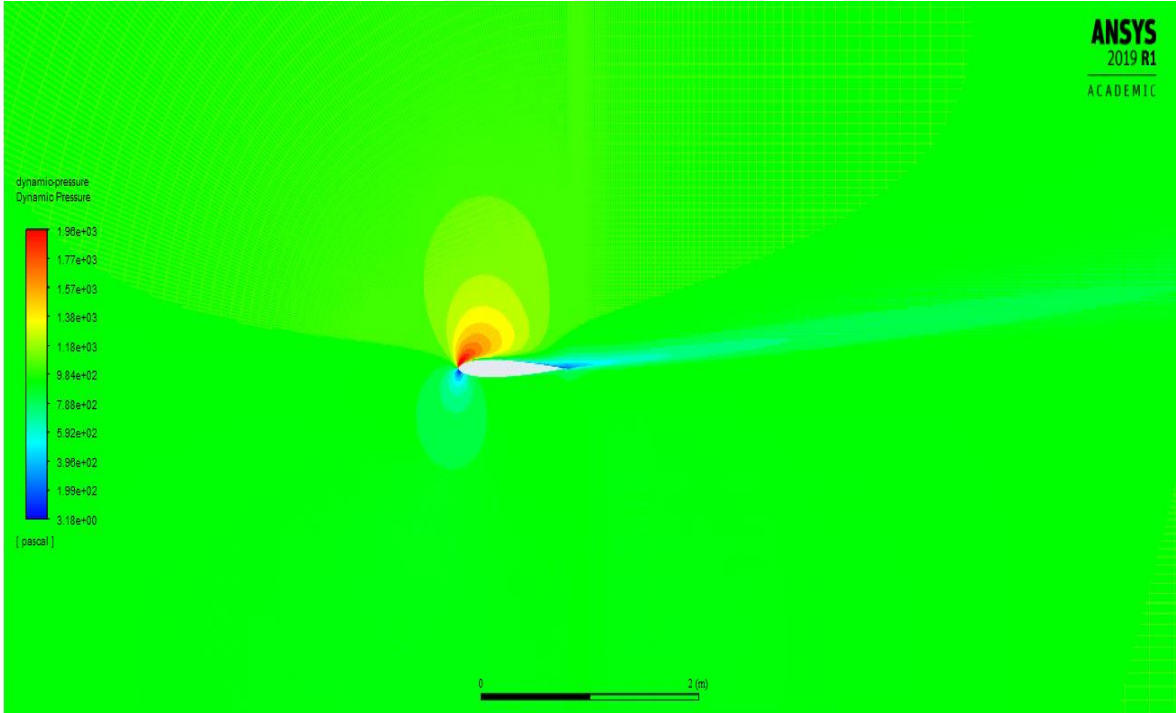
Şekil 4.55. 4° Hücüm açısı ile 40m/s dinamik basınç alanı
