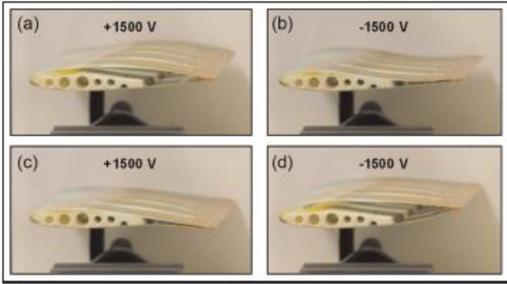
Şekil 3.7. Pizoseramik kompozit aktüatör [9]
