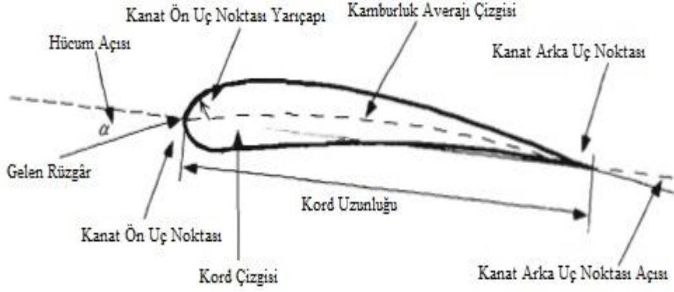
Şekil 2.3. Airfoil terminolojisi
