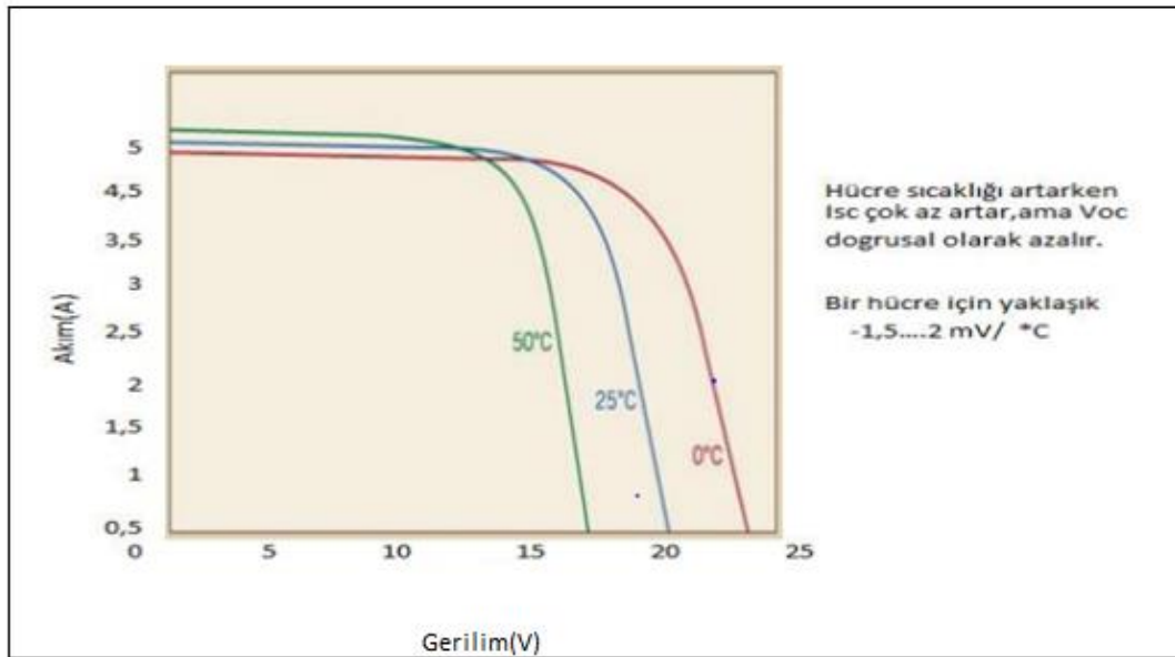
Şekil 2.15. Sıcaklığa bağlı olarak akım ve voltajın değişimi [2].
