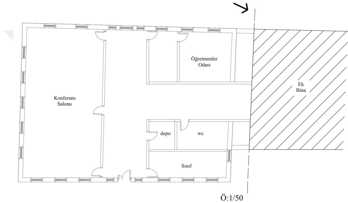
Şekil 3. 108. Oltu Karabekir Okulu rölöve planı (Çizim: Y. E. Durmaz, 2020)
