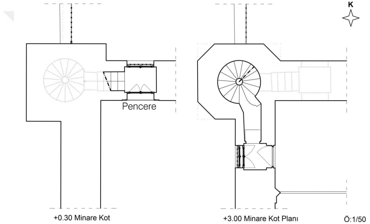
Şekil 3. 71. Minare planı (Çizim: Y. E. Durmaz, 2020)
