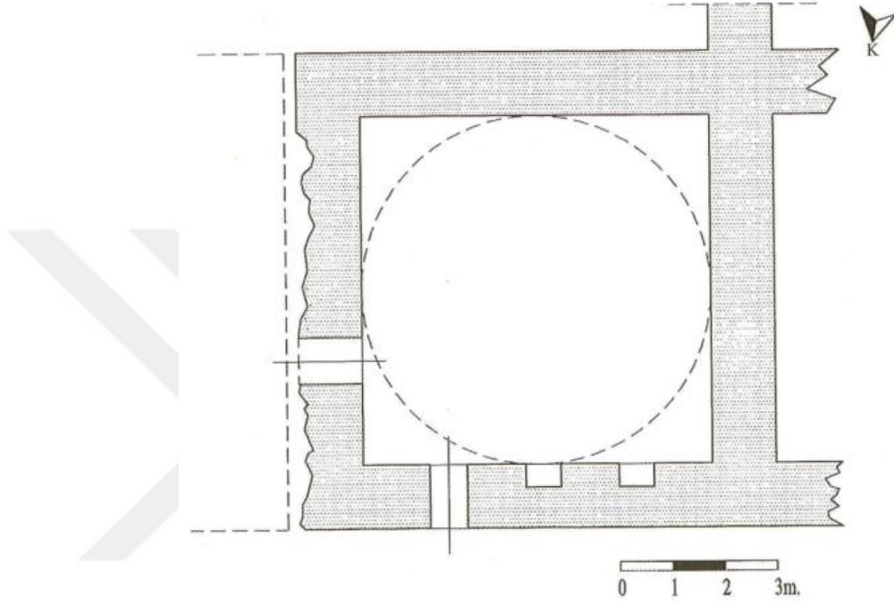
Şekil 3. 90. Arslan Paşa Hamamı planı (Çizim: A. Uluçam, 1983)
