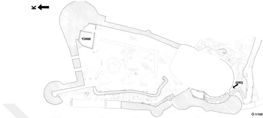
Şekil 3. 6. Oltu Kalesi +30.00 kot planı (EKTVKK Arşivi, 2016) 8
