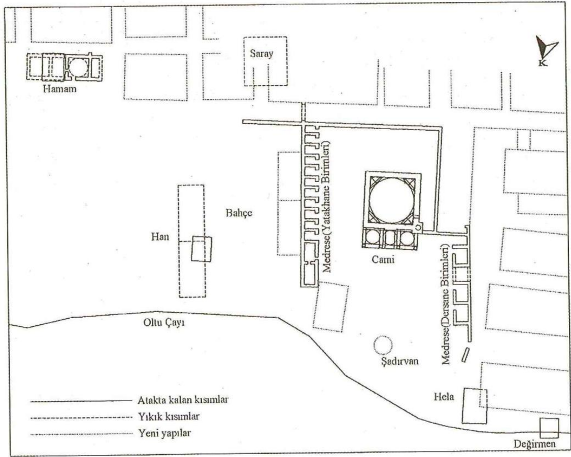
Şekil 3. 39. Arslan Paşa Külliyesi, 1983 Yılı vaziyet planı 26
