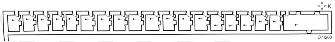
Şekil 3. 83. Doğu Medrese planı (EVBM Arşivi, 2007)
