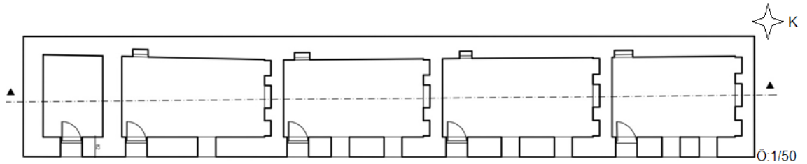
Şekil 3. 75. Batı Medrese planı (EVBM Arşivi, 2007)
