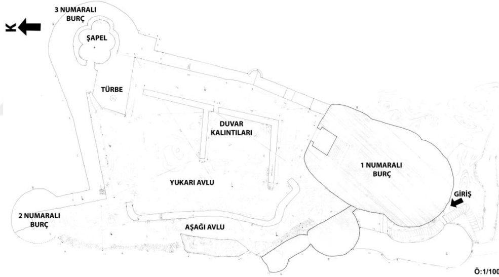
Şekil 3. 7. Oltu Kalesi +37.00 kot planı (EKTVKK Arşivi, 2016) 8
