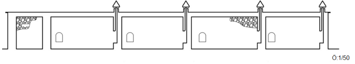
Şekil 3. 76. Batı Medrese kesiti (EVBM Arşivi, 2007)
