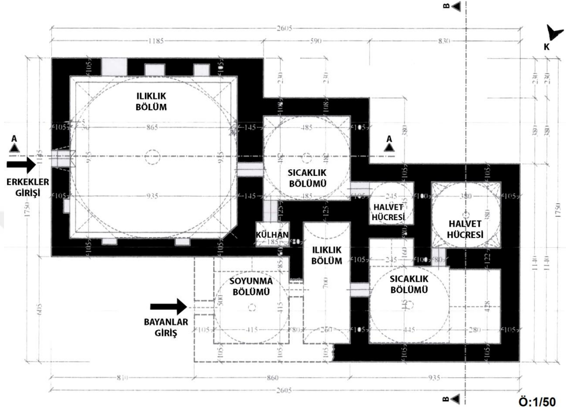
Şekil 3. 31. Selçuklu Hamamı röleve planı (EKTVKK Arşivi, 2003) 21
