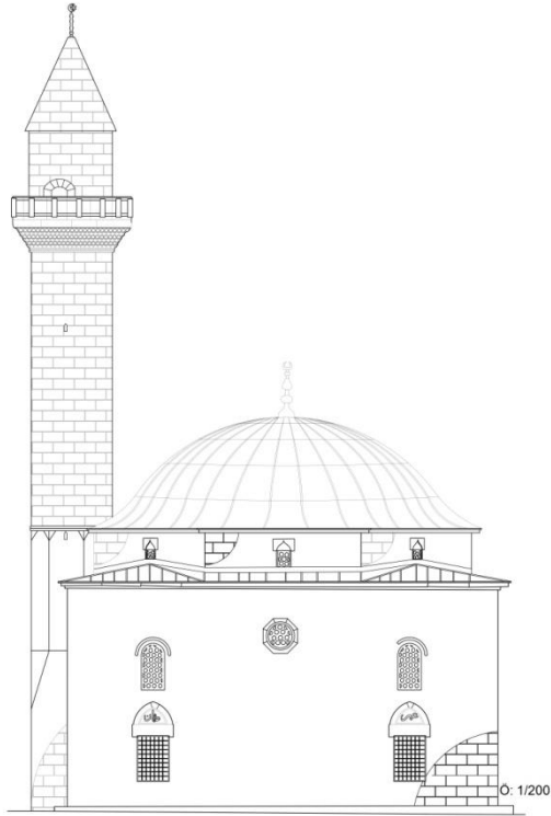
Şekil 3. 68. Arslan Paşa Camii batı görünüşü (EVBM Arşivi, 2007)
