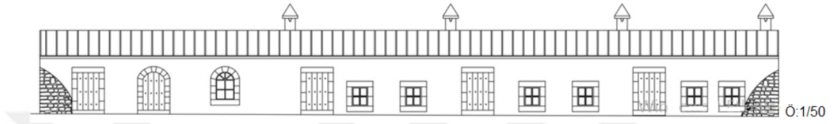
Şekil 3. 77. Batı Medrese görünüşü (EVBM Arşivi, 2007)
