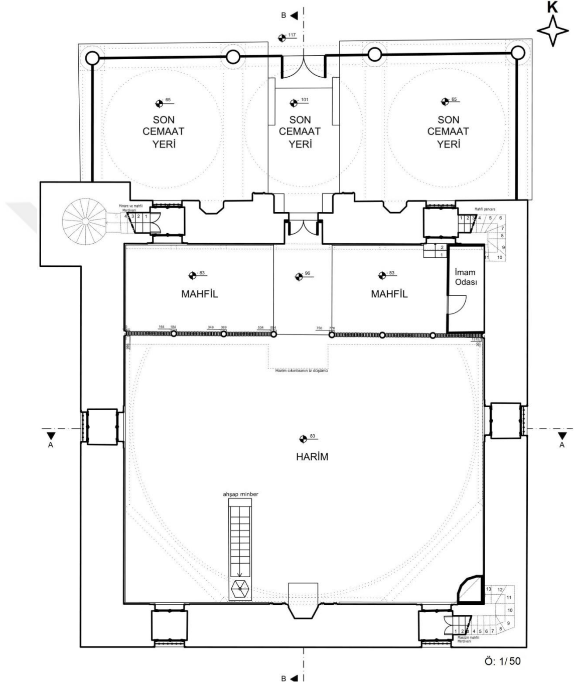
Şekil 3. 54. Arslan Paşa Camii harim planı (EVBM Arşivi, 2007)
