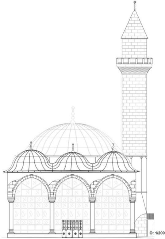
Şekil 3. 66. Arslan Paşa Camii doğu görünüşü (EVBM Arşivi, 2007)
