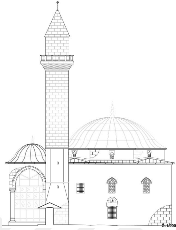
Şekil 3. 68. Arslan Paşa Camii batı görünüşü (EVBM Arşivi, 2007)
