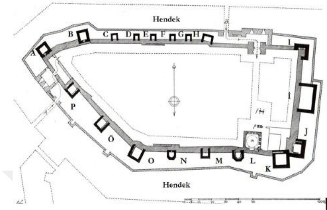
Çizim 13. Kayseri iç kalesinin planı. (Sevgi Parlak, Osmanlı Öncesinde Anadolu Kalelerinde Kapılar , İstanbul Üniversitesi SBE Sanat Tarihi Anabilim Dalı, Yayınlanmamış Doktora Tezi, İstanbul 2010, s. 374.)
