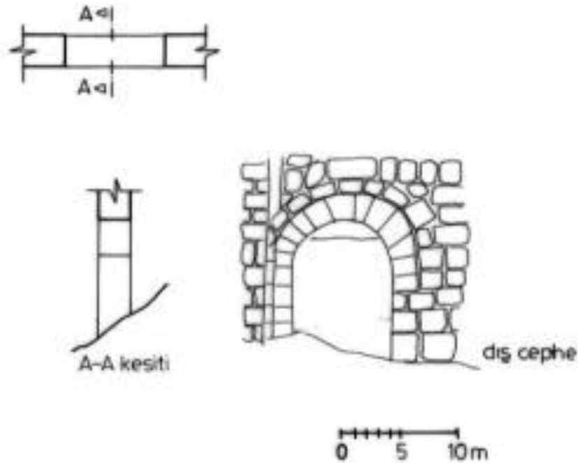
Çizim 16. Kögonya Kalesi, Bizans kapısı. (Ertuğrul Danık, “Şebinkarahisar Kalesi”, Sanat Tarihi Dergisi , XIII/2, Ekim 2004, s. 51-78.)
