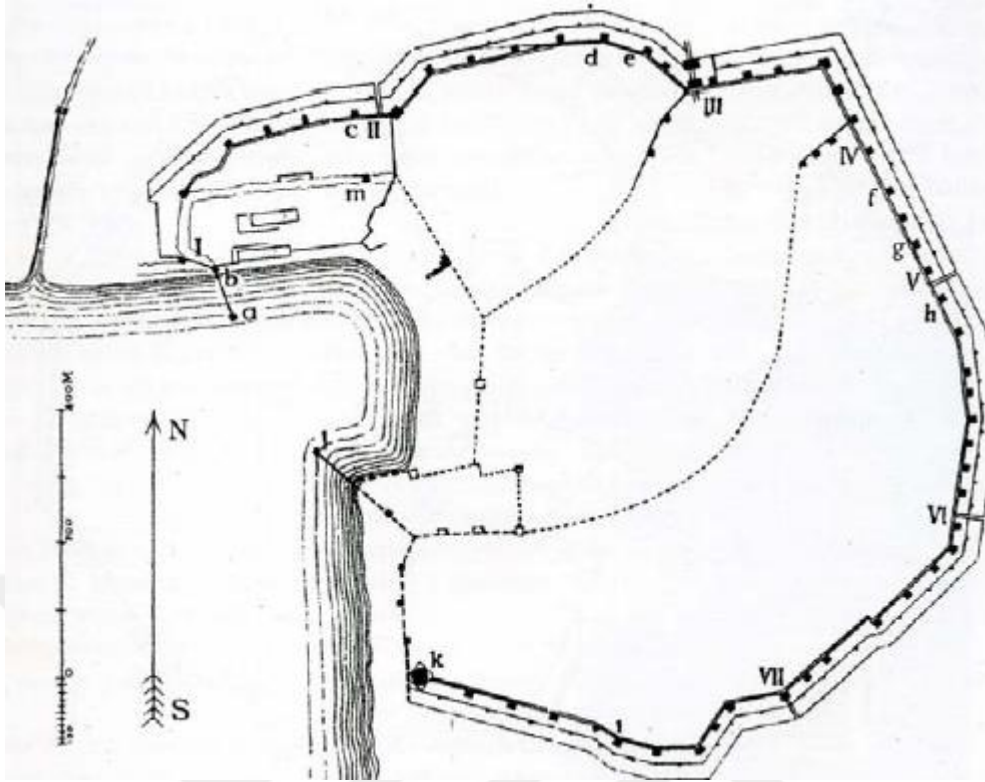
Çizim 3. Antalya surlarının planı. (Sevgi Parlak, Osmanlı Öncesinde Anadolu Kalelerinde Kapılar , İstanbul Üniversitesi SBE Sanat Tarihi Anabilim Dalı, Yayınlanmamış Doktora Tezi, İstanbul 2010, s. 90.)
