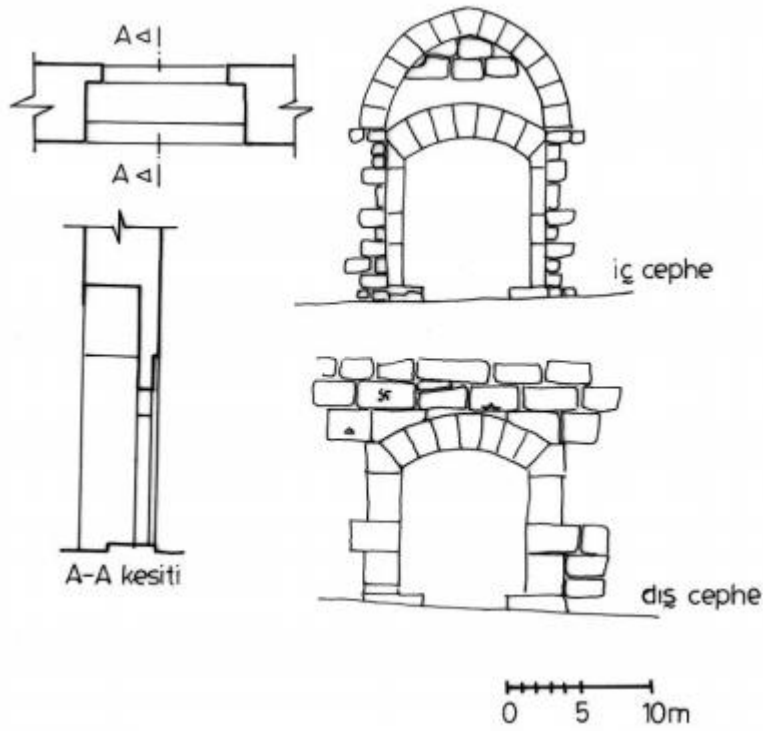
Çizim 17. Kogonya Kalesi, İç kale giriş kapısı. (Ertuğrul Danık, “Şebinkarahisar Kalesi”, Sanat Tarihi Dergisi , XIII/2, Ekim 2004, s. 51-78.)
