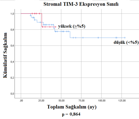
Şekil 9. Kaplan - Meier Yöntemiyle TIM-3 Ekspresyonu ile Sağkalım İlişkisi Grafiği - 2
