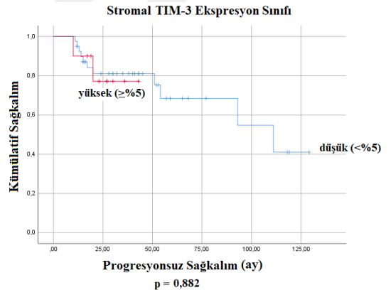
Şekil 9. Kaplan - Meier Yöntemiyle TIM-3 Ekspresyonu ile Sağkalım İlişkisi Grafiği - 2
