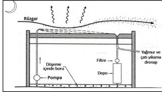
Şekil 3. 38 Islak çatı yöntemi (Lechner, 1991)
