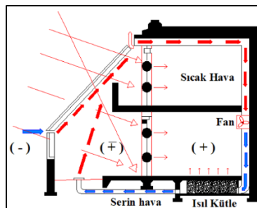
Şekil 3. 26 Kış bahçesinin çalışma ilkesi (Kartal, 2009)
