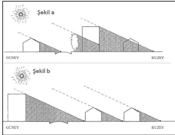
Şekil 3. 7 Bina aralıklarının belirlenmesi (Gazioğlu, 2012)
