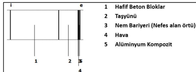
Şekil 5. 70 Mall of Mitrovica cephe detayı (ODA Architects, 2022)
