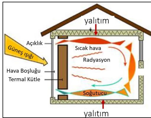
Şekil 3. 15 Hava dolaşımı gündüz açık Trombe duvarı (Chel, Kaushik, 2018)
