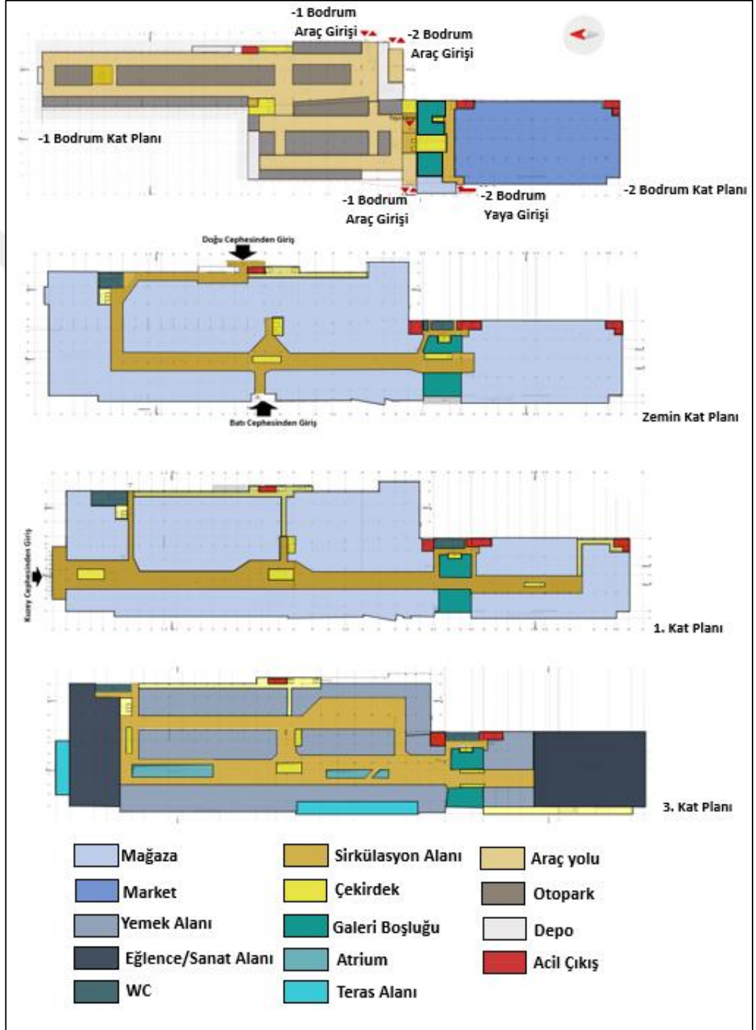
Şekil 5. 7 Albi Mall mimari kat planları (Puka Design, 2022'den geliştirilerek)
