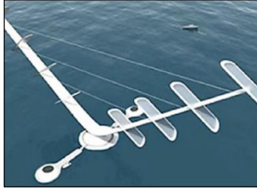
Şekil 3. 49 Eğik Eksenli Rüzgar Türbini (EERT) (Kısa Ovalı & Giousouf, 2022)
