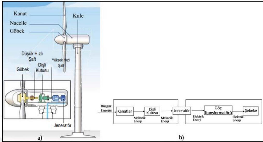
Şekil 3. 47 a. Yatay Eksenli Rüzgar Türbin (YERT) bileşenleri, b. Elektrik enerjisi üretimi (Kaya & Koç, 2015)
