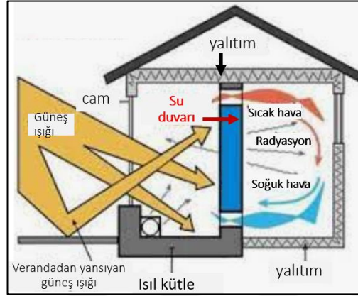
Şekil 3. 18 Su Duvarı şematik gösterimi (Pinterest, 2022)
