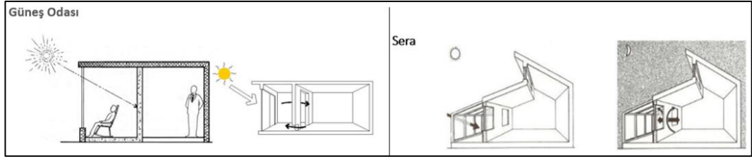
Şekil 3. 29 Isıl özellikleri bakımından kış bahçeleri ( Lechner, 1991; Özdemir, 2005; Khanları, 2013)
