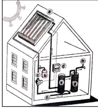
Şekil 3. 40 Konutlar için güneş enerjili aktif sistemler (Öztürk, 2013)
