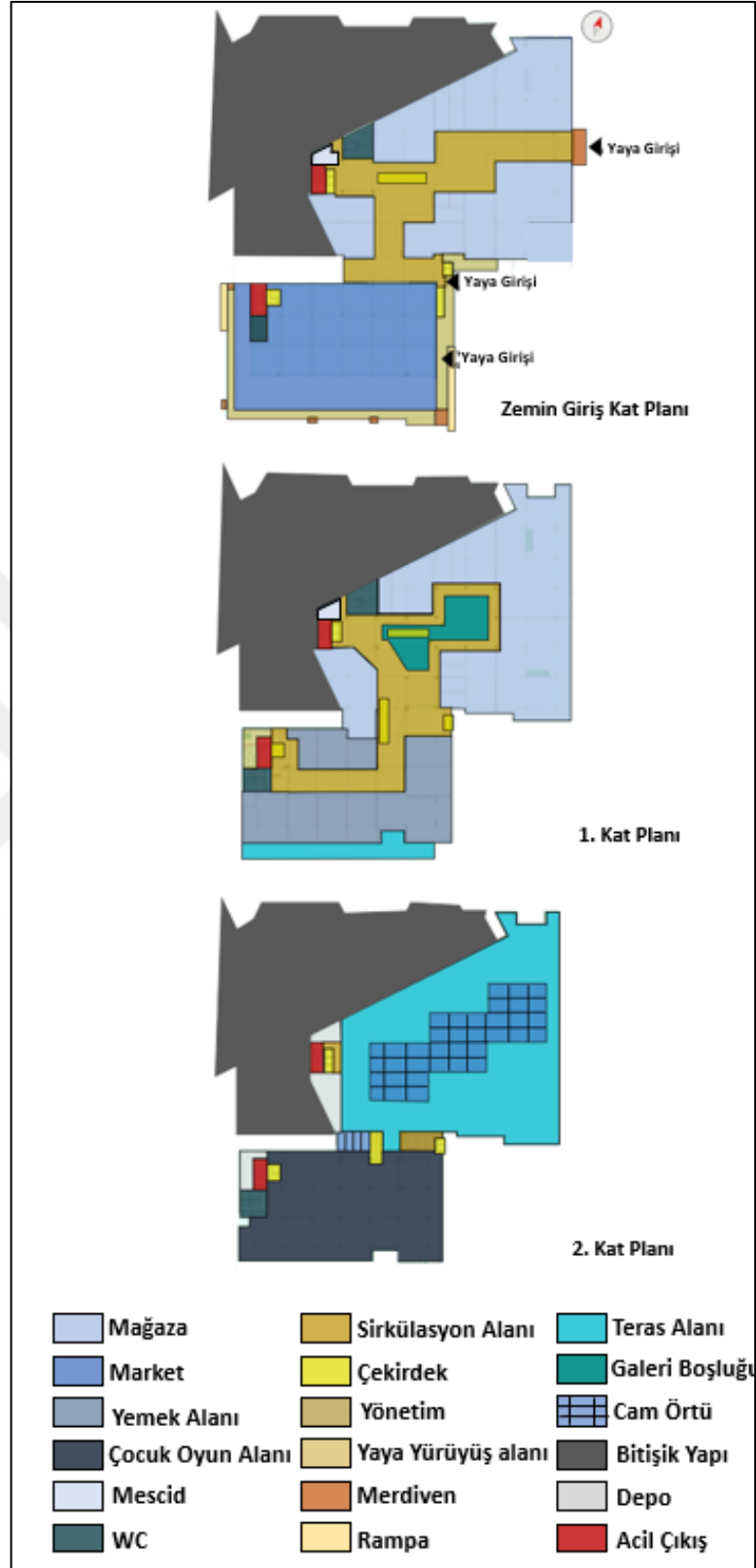
Şekil 5. 61 Mall of Mitrovica mimari kat planları (ODA Architects, 2022'den geliştirerek)
