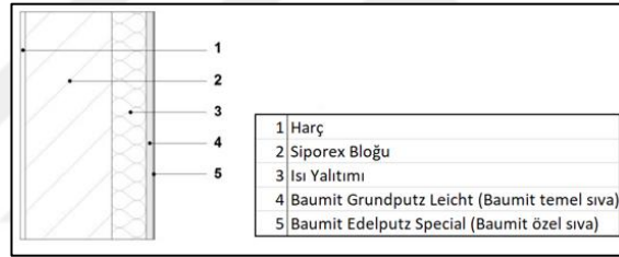
Şekil 5. 16 Albi Mall duvar detayı (Puka Design, 2022)
