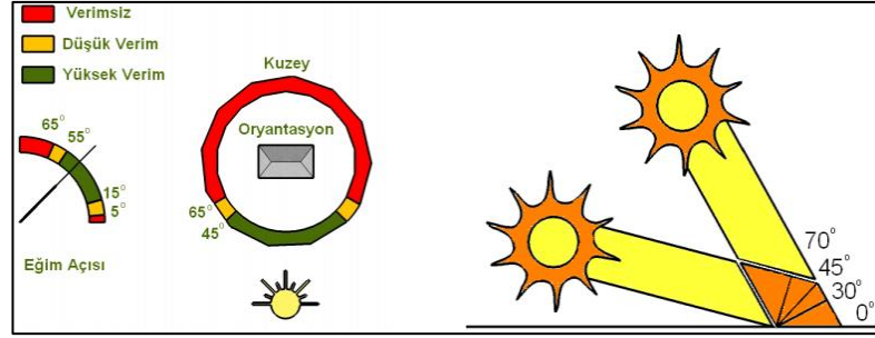
Şekil 3. 45 Yapılarda a) Panel eğimi ve yönlenme, b) Yaz ve kış kullanımı için uygun eğim tespiti (Uzun & Yeğin, 2006)
