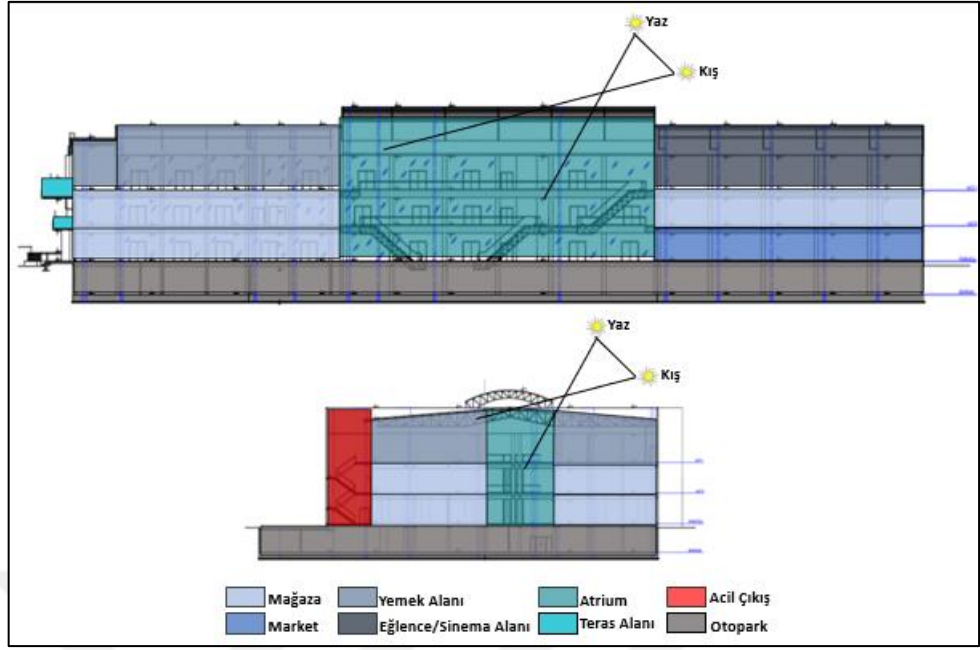
Şekil 5. 37 Ring Mall kesitleri (Ring Mall, 2022'den geliştirerek)
