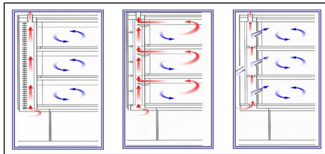
Şekil 3. 25 Çok katlı binalarda cidarlar arasındaki kesintili ve sürekli bulunan tampon bölge (Oğuz, 2007)
