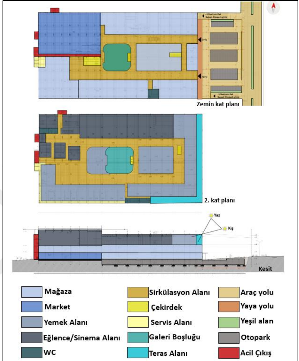
Şekil 5. 18 Galeria Mall mimari kat planları ve kesiti (G+A Architects, 2022'den geliştirilerek)
