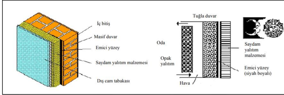
Şekil 3. 20 Saydam yalıtım malzemenin a) Dış duvara uygulanması, b) Trombe duvarında kullanılması (Yeşildal, 2002)
