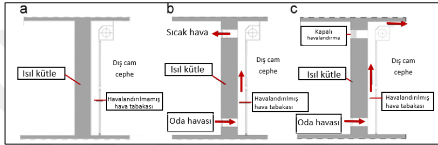
Şekil 3. 16 Trombe Duvarı'nın çeşitli konfigürasyonları: a) Havalandırmasız, b) Sıcak hava döngülü kış modu, c) Çapraz havalandırma ile yaz modu (Saadatian ve diğerleri, 2012)
