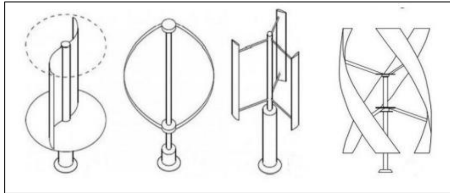
Şekil 3. 48 Dikey Eksenli Rüzgar Türbini (DERT) (Canoğlu, 2022)
