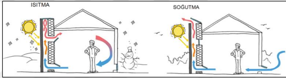
Şekil 3. 35 Güneş bacasının çalışma prensibi (Kalkan, 2017)
