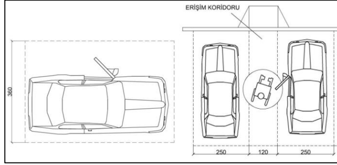
Şekil 4.6 a. Engelli park yeri genişliği, b. Erişim koridoru ile tasarlanmış park yeri (Terece, 2019)
