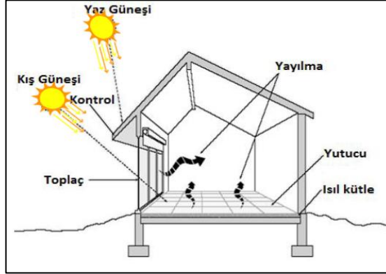
Şekil 3. 11 Doğrudan kazançlı pasif gneş tasarımı (NREL, 2001)
