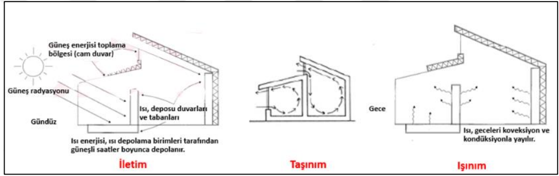
Şekil 3. 10 Isı iletimi (kondüksiyon), taşınım (konveksiyon), ısı ışıınımı (radyasyon) (Damar, 1998; Aksoy, 2019)
