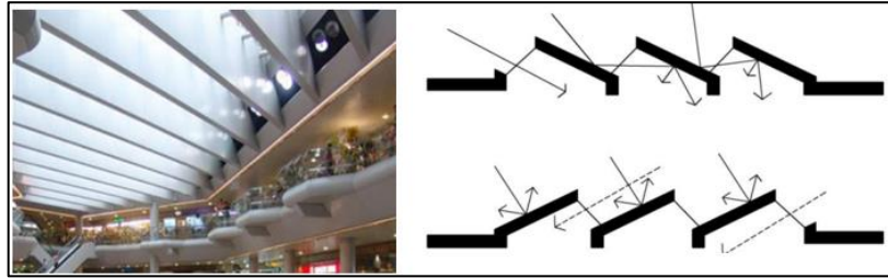
Şekil 4. 5 a. Taşıyıcı sistemin doğal aydınlatmaya etkisi, b. Üst örtünün kaplı olduğu camlama sisteminden güneş ışınımının alınması (Göçer, 2006)
