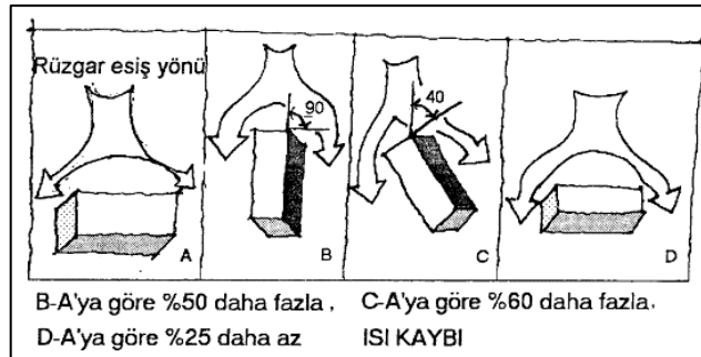
Şekil 3. 4 Hakim rüzgar yönüne göre binaların konumlanması (Uzun, 1997)
