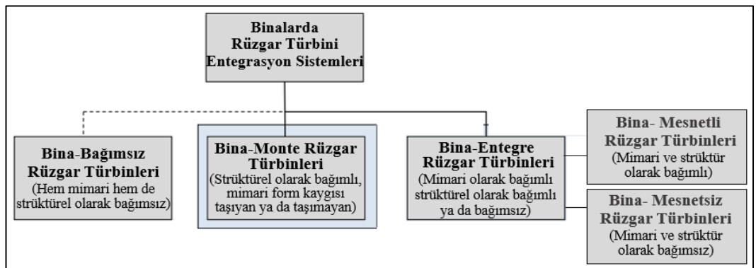
Şekil 3. 50 Binalarda rüzgâr türbini uygulama çeşitleri (Günel & Ilgın, 2008; Kısa Ovalı & Giousouf, 2022; Begeç, 2022’den geliştirerek)
