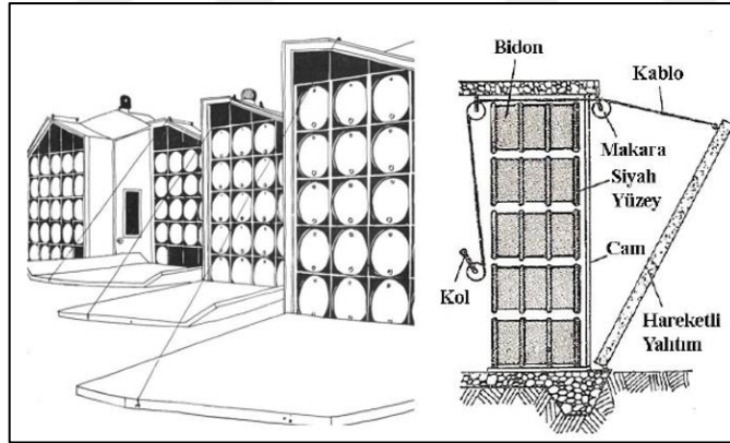
Şekil 3. 19 Su duvarı (Bidon duvar) çalışma prensibi (Efe, 2009; Çakır, 2011)
