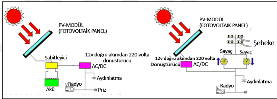
Şekil 3. 44 Şebekeden bağımsız ve şebekeye bağlı PV modül kullanımı (Sayın & Koç, 2011)
