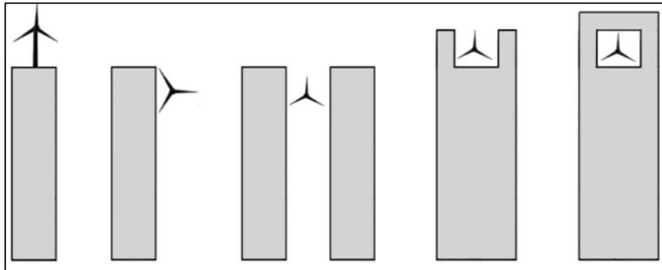
Şekil 3. 51 Bina-monte rüzgar türbinlerinin yapılarda konum çeşitliliği (Ilgın & Günel, 2021)
