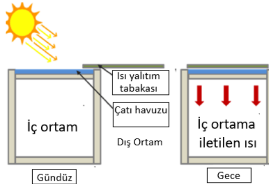
Şekil 3. 21 Çatı havuzu şematik görünümü (Kartal, 2020)
