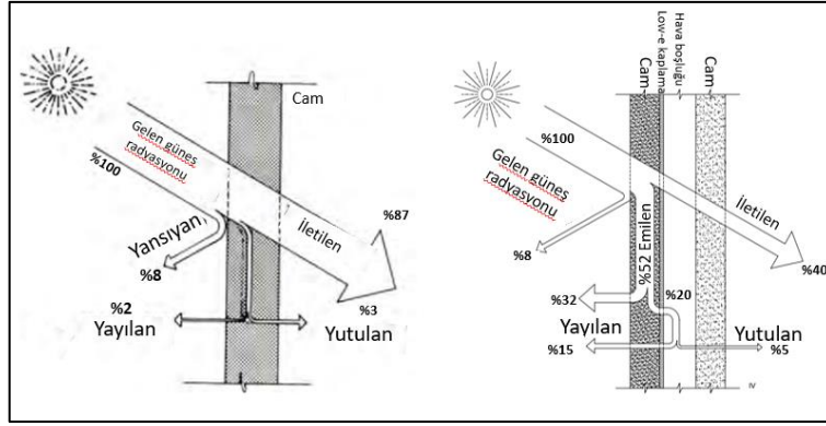
Şekil 3. 8 Tek ve çift camdan güneş ışınlmı geiři (Lechner, 1991)
