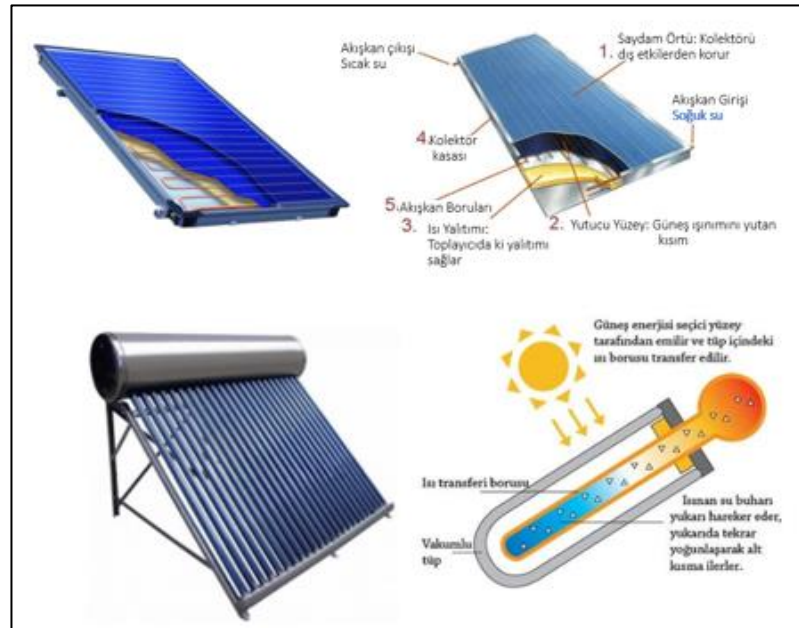
Şekil 3. 41 Düzlemsel ve vakum borulu güneş kolektörü (Altıngöz & Mıhlıyanlar, 2019; Güneysan Güneş Enerjisi, 2022)
