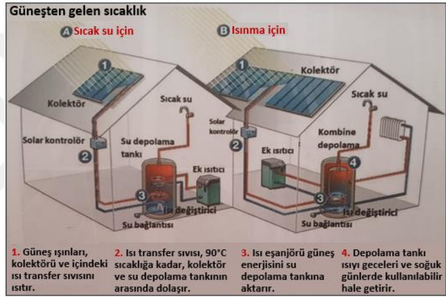
Şekil 3. 42 Konutlar için güneş enerjili aktif sistemler (Ceylan & Gürel, 2018)
