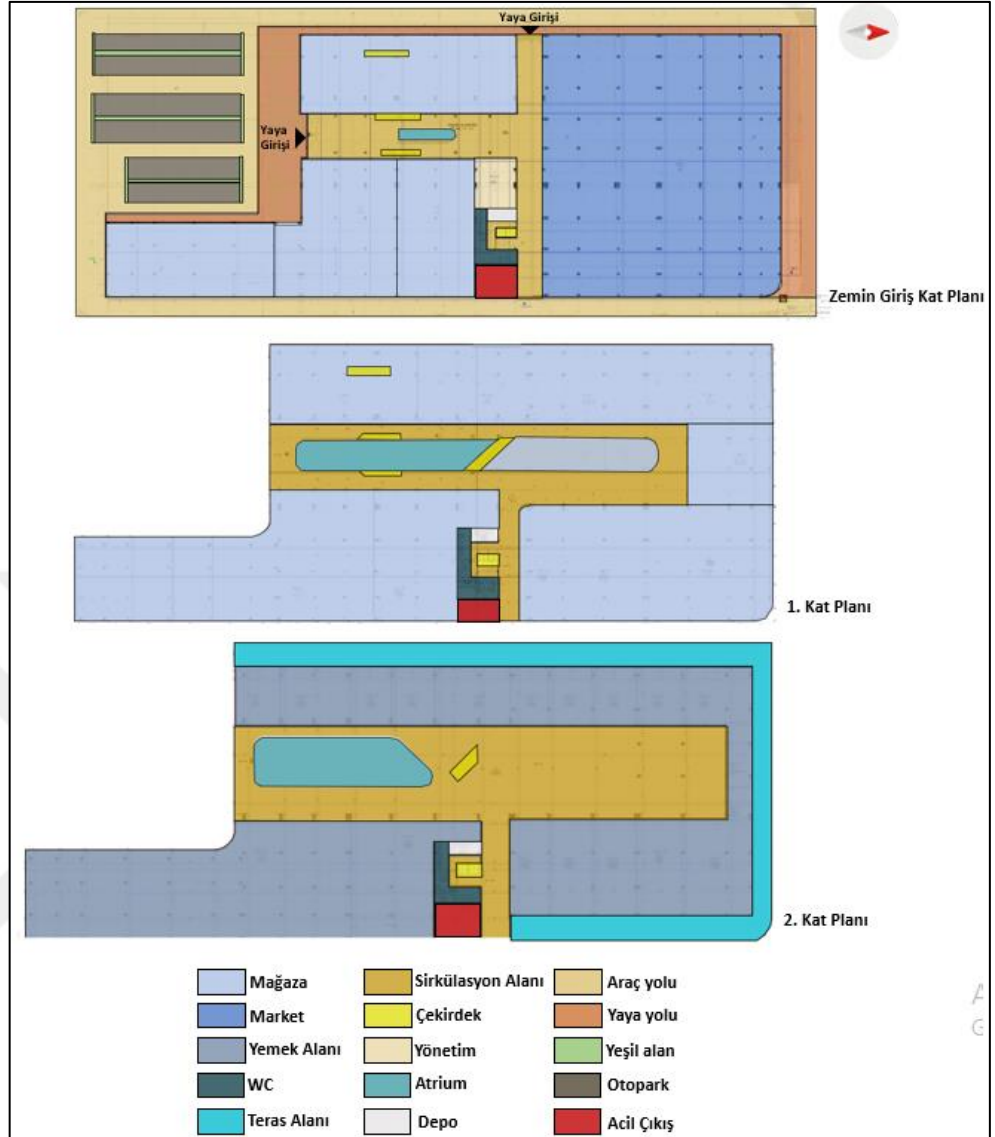
Şekil 5. 53 Yeni Grande Calabria Mall mimari kat planları (Kapak Studio, 2022'den geliştirerek)
