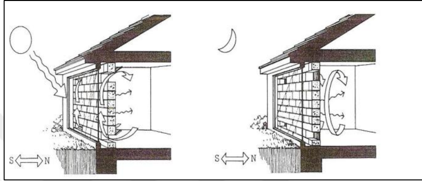
Şekil 3. 14 Trombe Duvarı (Berber, 2012)
