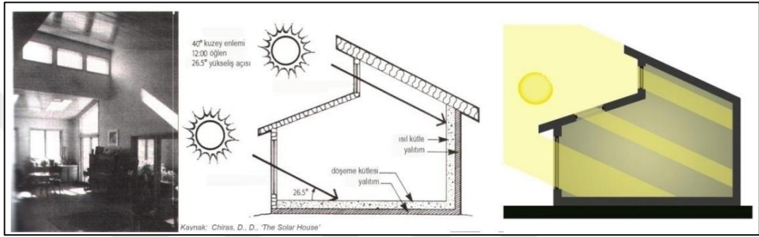
Şekil 3.13 Çatı pencerelerinin konumu (Efe, 2009)
