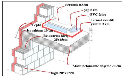
Şekil 5. 59 Grande Calabria Mall detay kesiti (Kapak studio, 2022)
