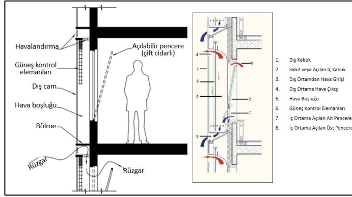
Şekil 3. 23 Çift Cidarlı Cephe Sistemlerinin Çalışma İlkesi (Lechner, 1991; Çakır, 2012)
