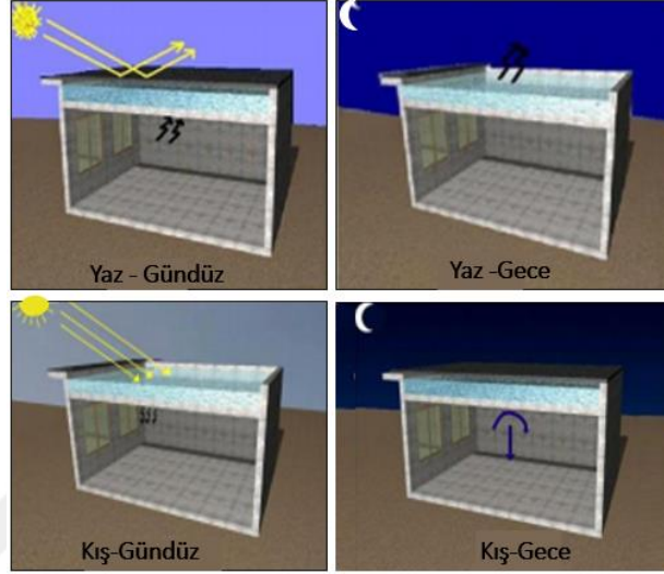
Şekil 3. 22 Çatı havuzunun yaz-kış çalışma ilkesi (Çakır, 2011)
