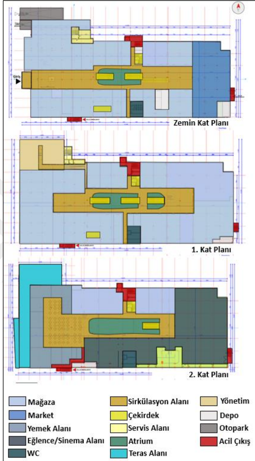
Şekil 5. 36 Ring Mall mimari kat planları (Ring Mall, 2022'den geliştirerek)
