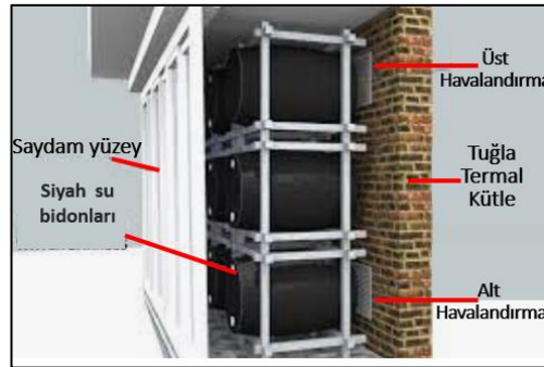
Şekil 3. 17 Su duvarı (Bidon duvar) (Pinterest, 2022)
