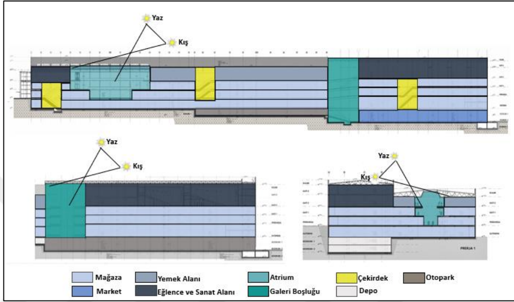
Şekil 5. 8 Albi Mall kesitleri (Puka Design, 2022'den geliştirilerek)
