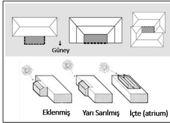
Şekil 3. 28 Binadaki konumlarına göre kış bahçeleri (Modirrousta ve Boostani, 2016)
