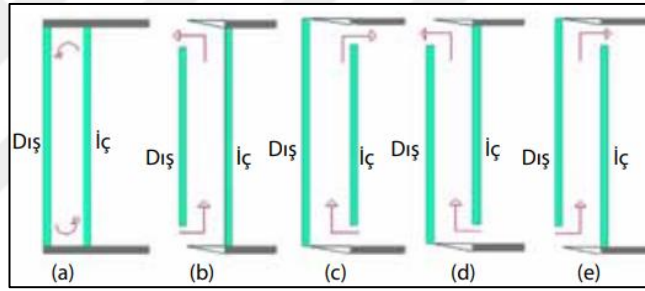
Şekil 3. 24 Çift cidarlı cephelerde hava akış metodları (İnan & Başaran, 2014)
