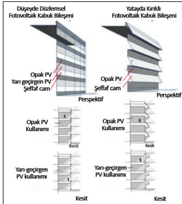
Şekil 3. 46 Güneş pillerinin giydirmce cephe olarak çeşitleri (Sayın & Koç, 2011)
