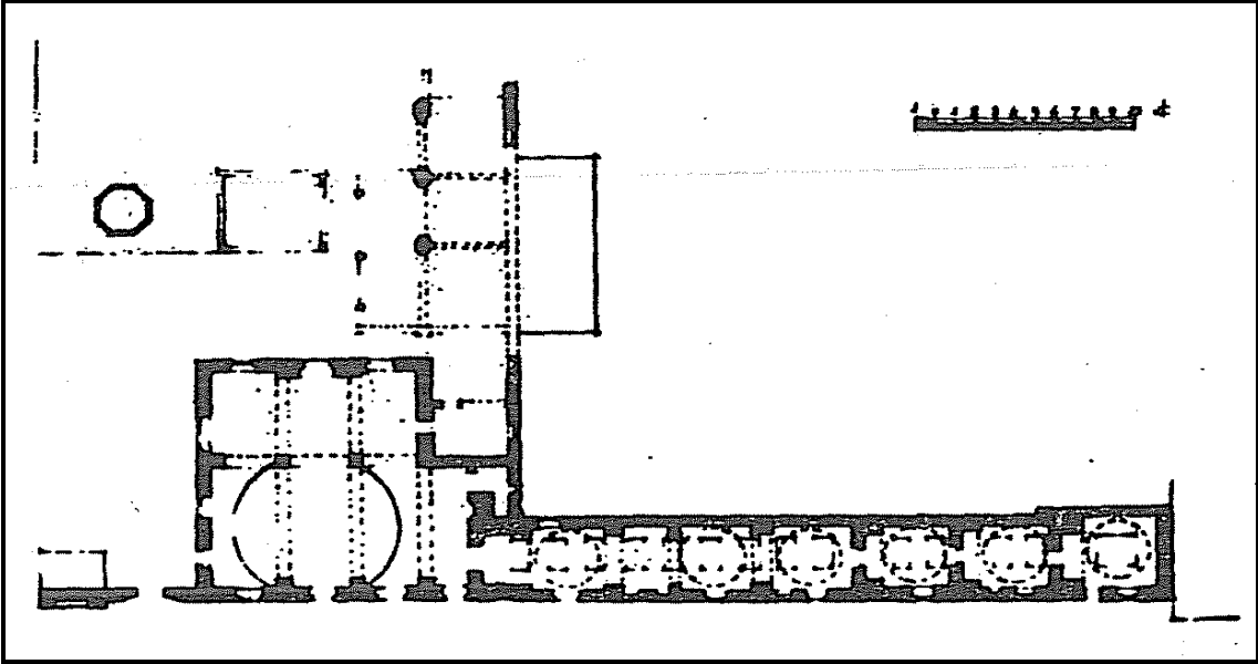
Lefkoşa Mevlevîhâne Planı
