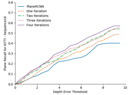
(d) Plane Recall for Sequence 16
