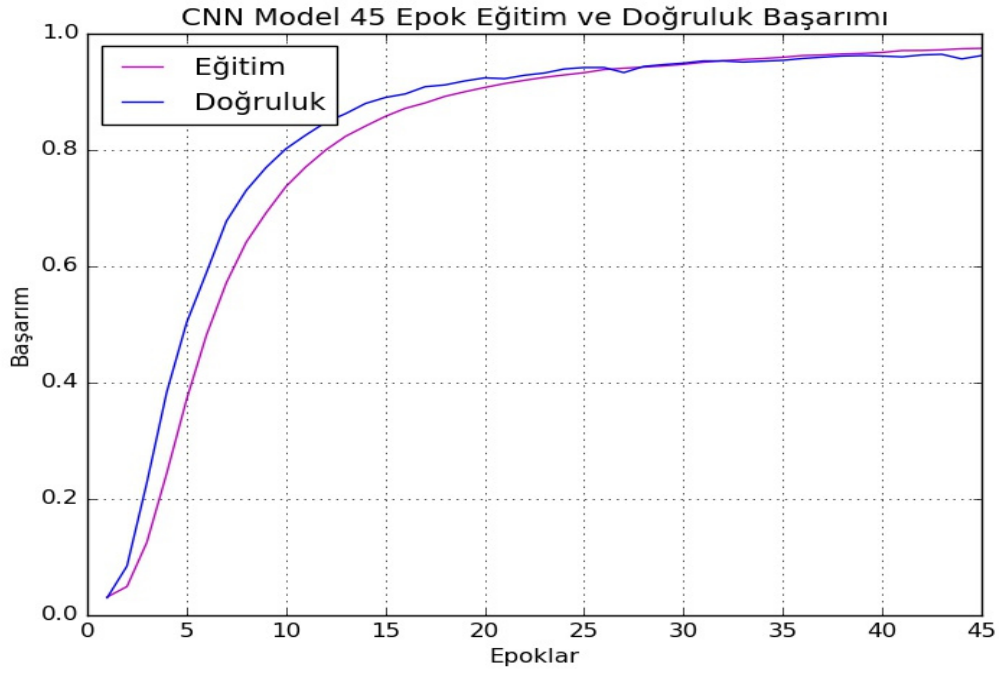
Şekil 6.1. 10 katmanlı ESA'nın başarımlar grafiği
