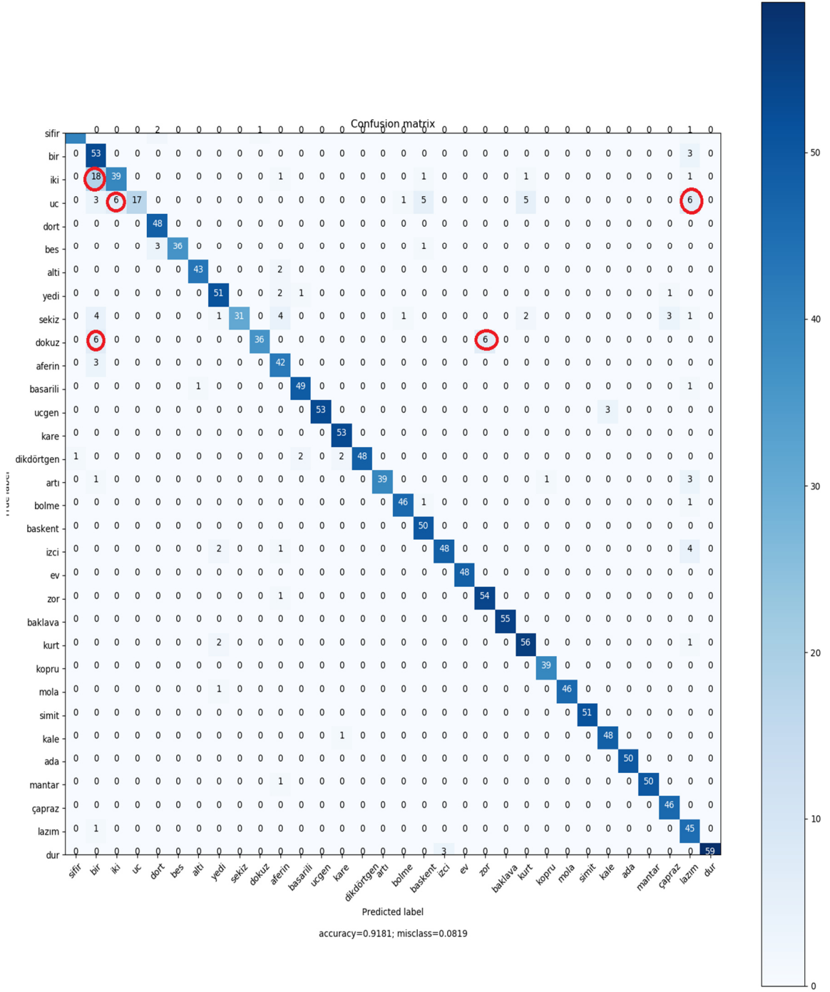
Şekil 6.10. ResNet50 karışıklık matrisi
