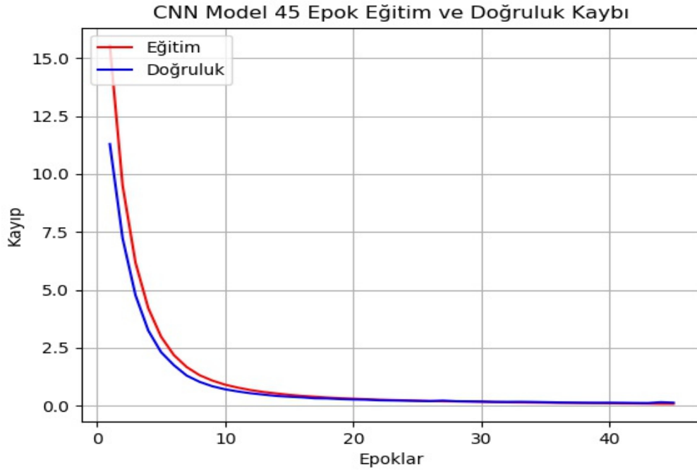
Şekil 6.2. 10 katmanlı ESA'nın kayıplar grafiği
