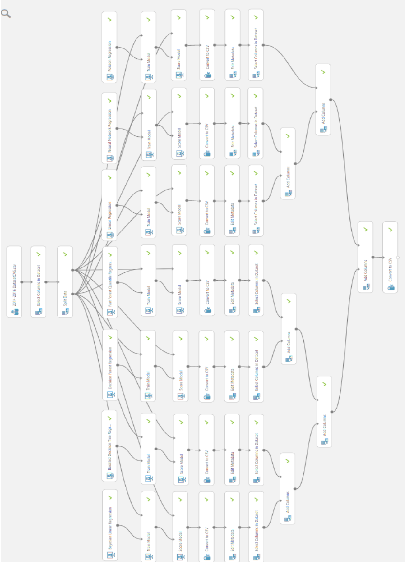
Şekil 7: Kod Şeması
