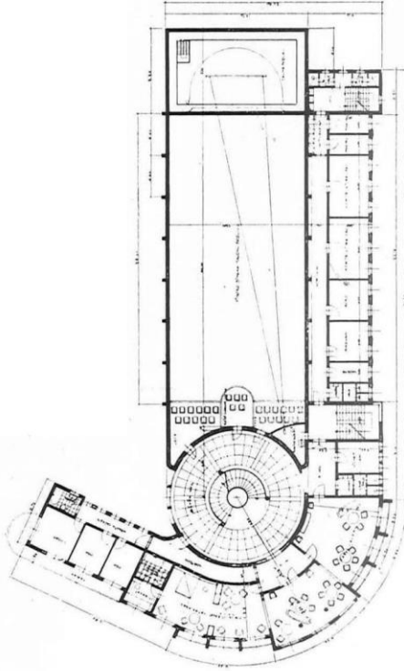
Şekil 2.21. Sivas Halkevi projesi kat planları (Anonim 1939)
