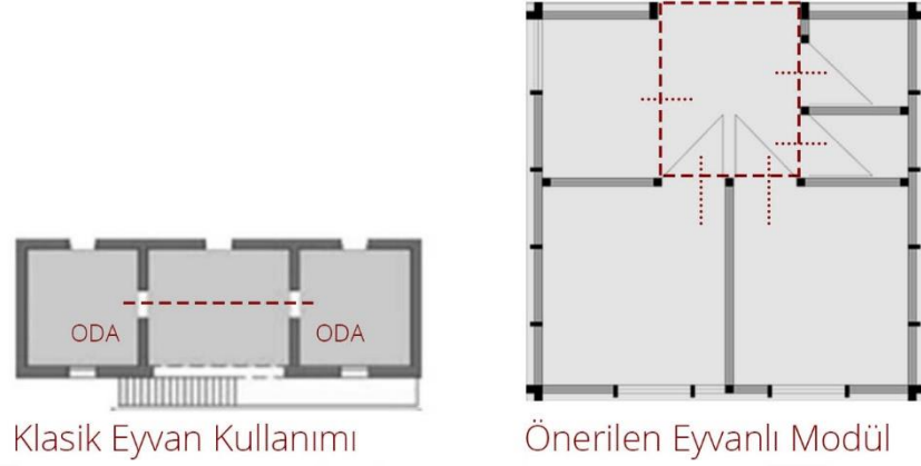
Şekil 4.9. Klasik eyvan kullanımını ve önerilen eyvanlı modül gösterimi
