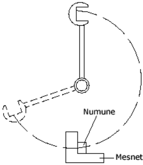
Şekil 4.2. Çentik-darbe deney seti
