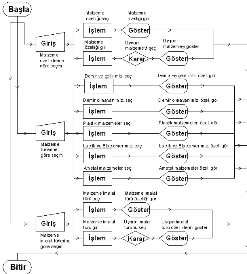
Şekil 5.1. Program akış şeması
