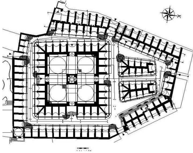
Plan.2.19. Vezirköprü Bedesten ve Arasta Dükkanları (V.G.M.A.)
