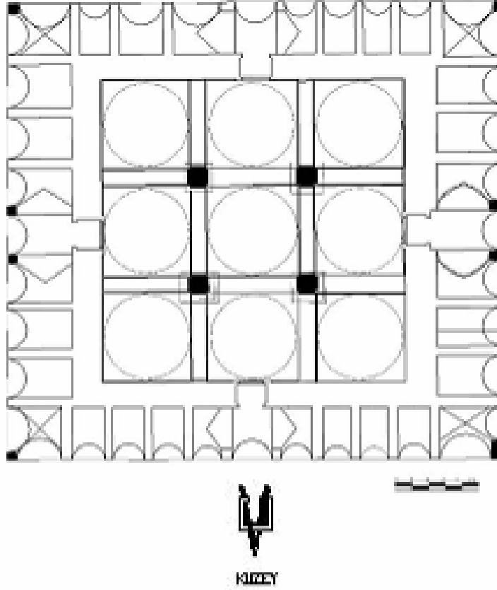
Plan 2.31. Merzifon Bedesteni (V.G.M.A.)
