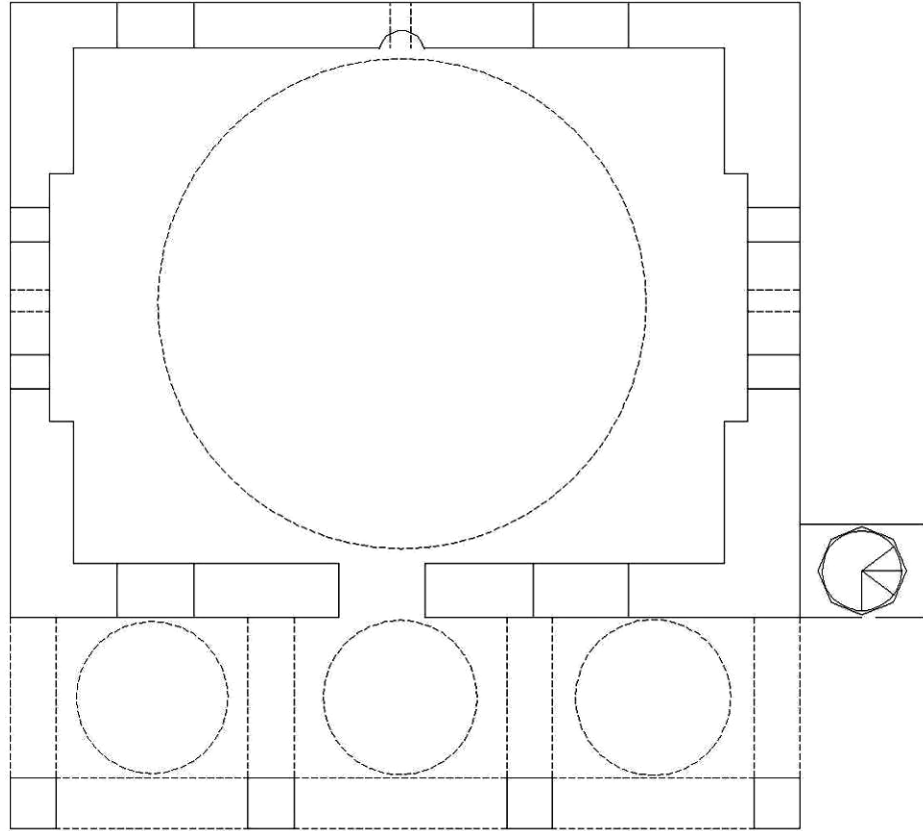
Kroki 2.1. Cısr-i Şuğur Köprülü Mehmet Paşa Camisi (S. Murat Topçu)
