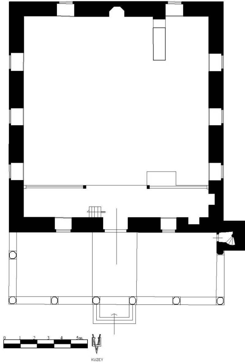
Plan.2.10. Vezirhan Köprülü Mehmet Paşa Camisi (V.G.M.A.)
