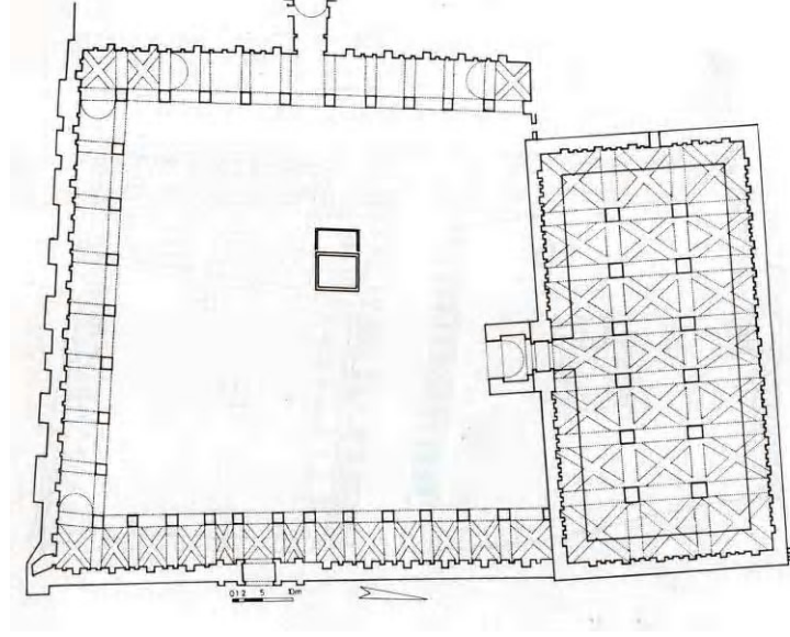
Plan. 2.41. İncesu Kara Mustafa Paşa Kervansaray (M. Denктаş'tan)
