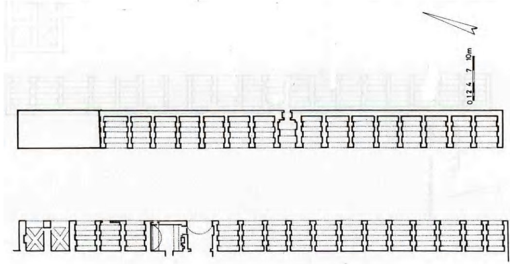
Plan.2.40. İncesu Kara Mustafa Paşa Arastası (M. Denктаş'tan)
