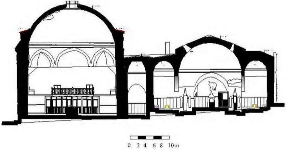
Plan 2.33. Merzifon Paşa Hamamı A-A Kesiti (V.G.M.A.)
