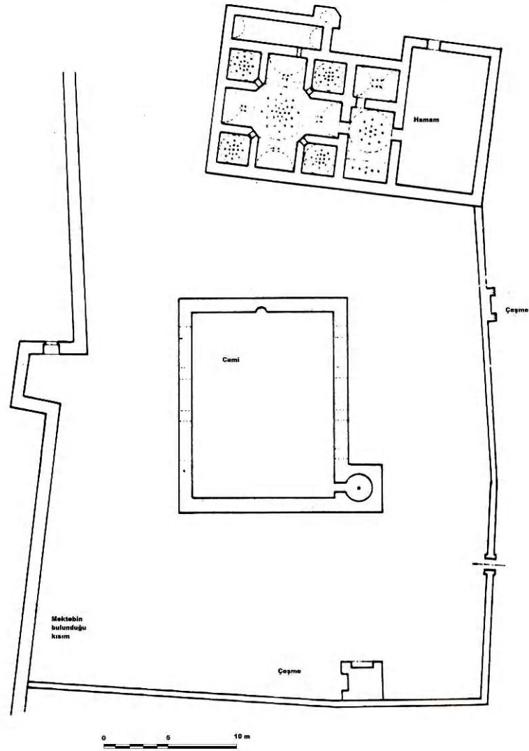
Plan.2.46. İnebahtı Amcazade Hüseyin Paşa Külliyesi Vaziyet Planı (Machiel Kiel'den)
