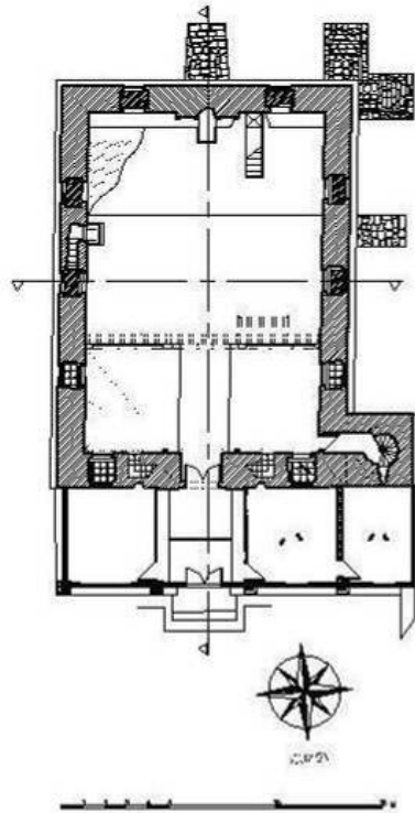
Plan. 2.34. Narince (Kara Mustafa Paşa Köyü) Abide Hanım Camisi (V.G.M.A.)
