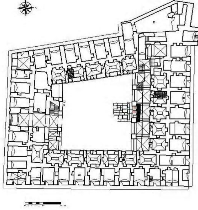
Plan.2.29. Taşhan Zemin kat Planı (V.G.M.A.)
