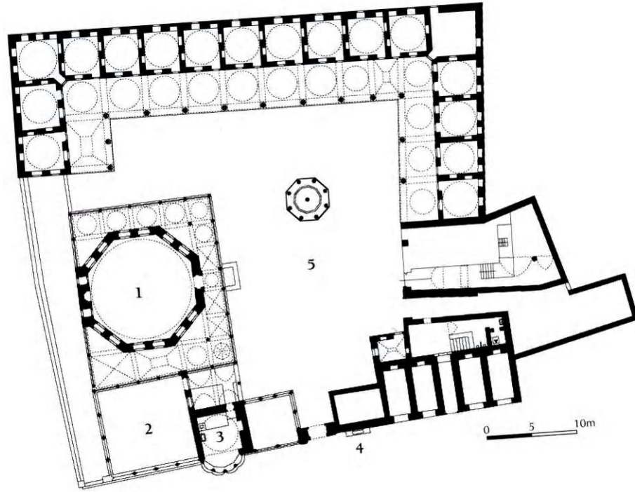
Plan.2.48. Amcazade Hüseyin Paşa Külliyesi Vaziyet Planı (Doğan Kuban'dan)
