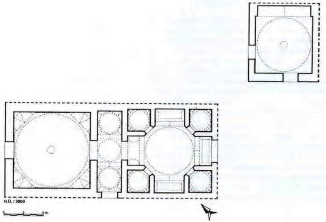
Plan.2.44. Yeşildirek Hamamı (Harun Ürer'den)
