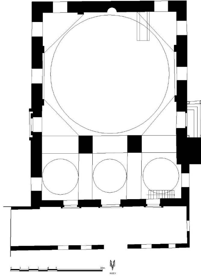
Plan. 2.6. Gümüşhacıköy Köprülü Mehmet Paşa Camisi (Fahriye Bayram'dan)
