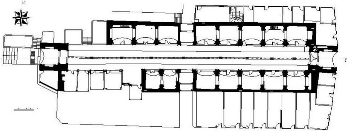
Plan.2.51. Gümüşhacıköy Köprülü Mehmet Paşa Arastası (V.G.M.A.)
