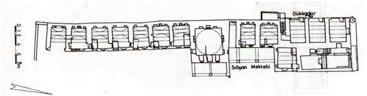
Plan 2.38. İncesu Kara Mustafa Paşa Medresesi (M. Denктаş'tan)
