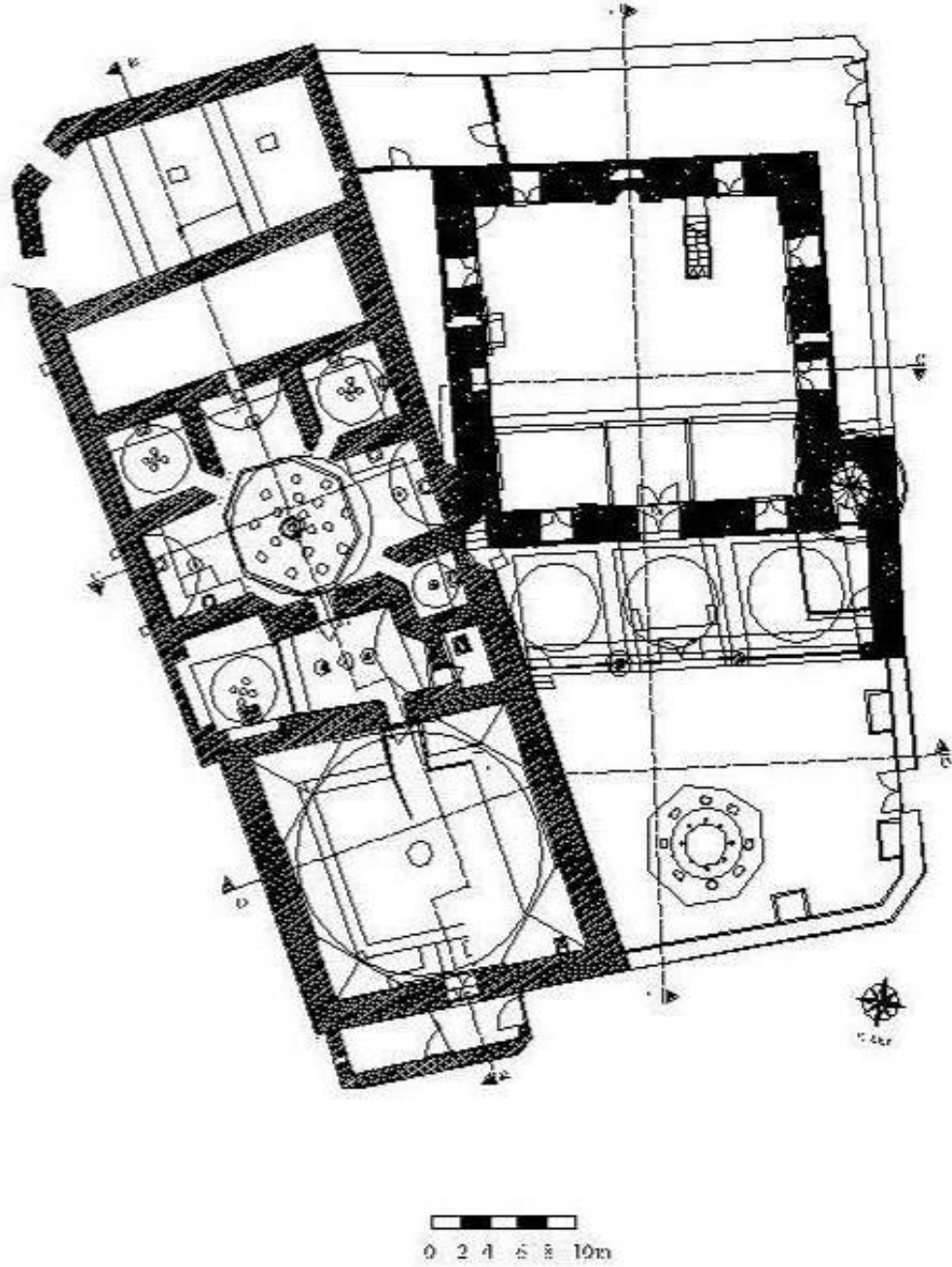
Plan.2.17. Vezirköprü Kale Hamamı (V.G.M.A.)
