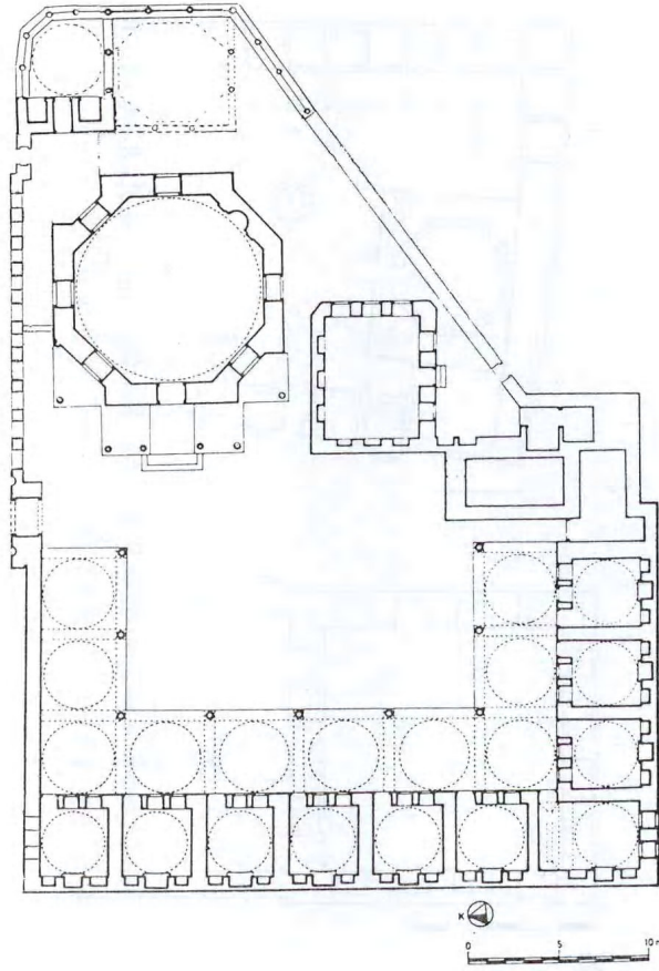
Plan.2.45. İstanbul Merzifonlu Kara Mustafa Paşa Külliyesi Vaziyet Planı (A.Vefa Çobanoğlu'ndan)
