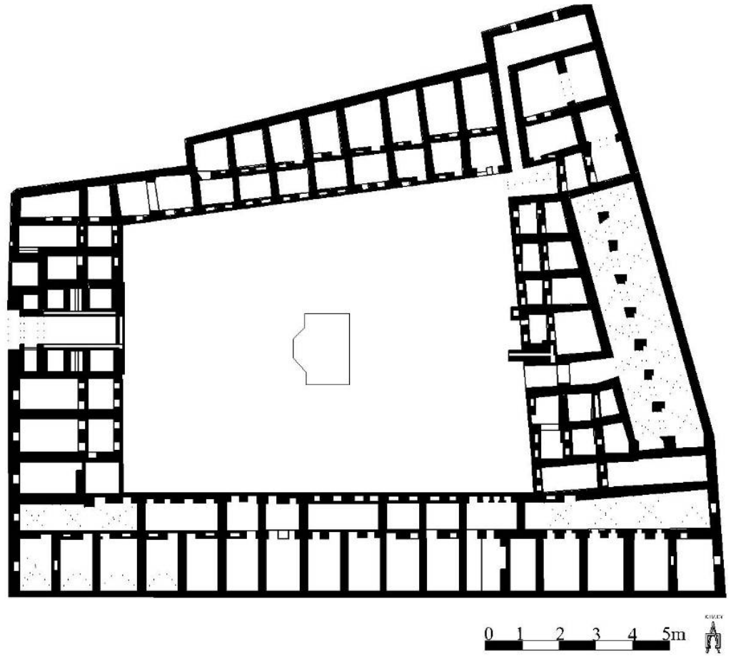
Plan.2.43. Halep Vezir Hanı ( Watenpaugh'dan )
