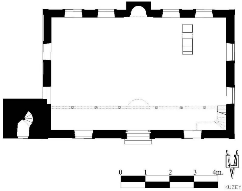
Plan.2.13. Bozcaada Köprülü Mehmet Paşa Camisi (V.G.M.A.)
