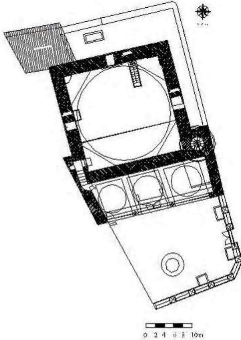
Plan.2.20. Vezirköprü Kale Camisi
