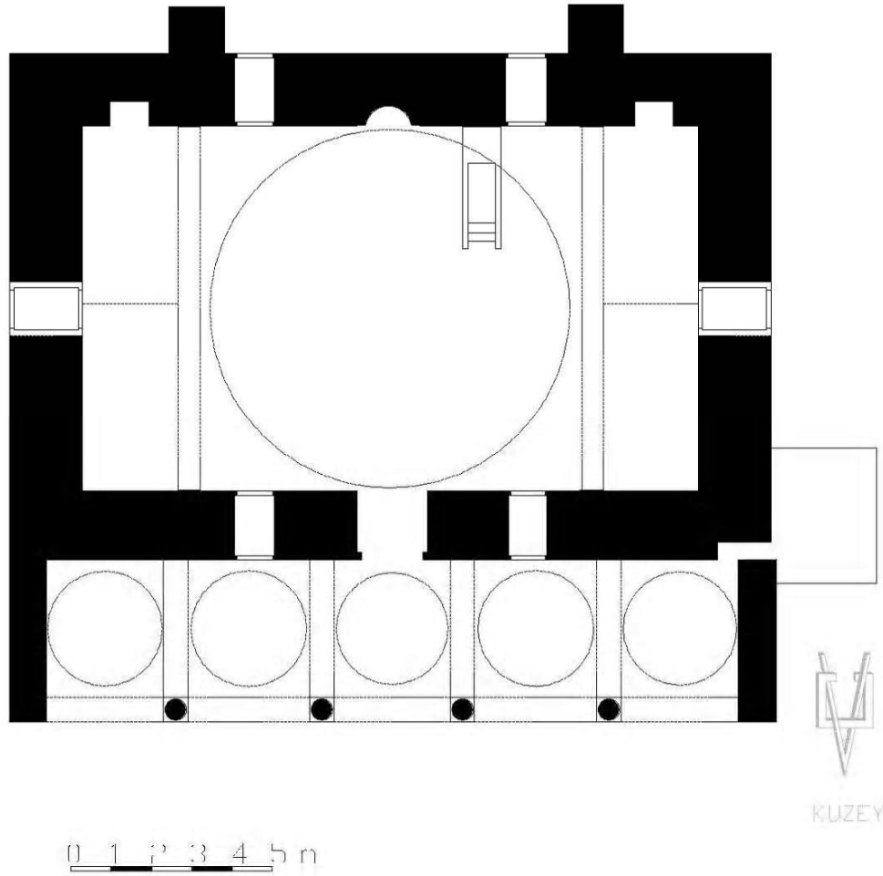
Plan.2.5. Malatya-Herkimhan Köprülü Mehmet Paşa Camisi (S.Murat Topçu)
