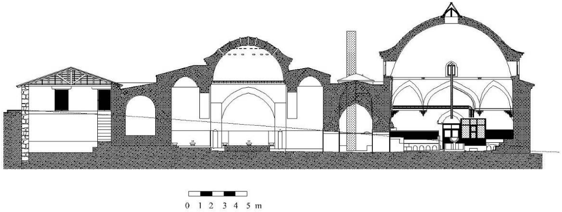
Plan.2.23. Vezirköprü Çifte Hamam A-A Kesiti (V.G.M.A.)
