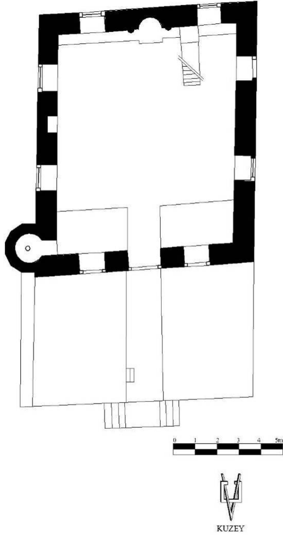
Plan.2.50. Makedonya Köprülü (Velez) Köprülüzade Elhac Ahmet Paşa Camisi (M. Zeki İbrahimgil Arşivinden)
