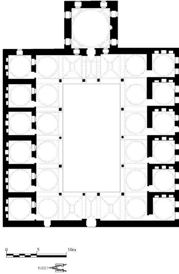
Plan 2.27. Vezirköprü Fazıl Ahmet Paşa Medresesi (Oktay Aslanapa'dan)
