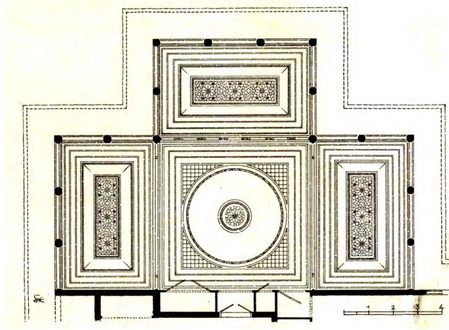
Plan.2.47. İstanbul-Amcazade Hüseyin Paşa Yalısı Divanhanesi
