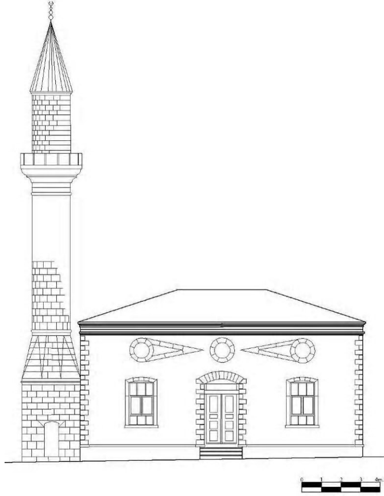
Çizim 2.2. Bozcaada Köprülü Mehmet Paşa Camisi Kuzey Cephesi (V.G.M.A.)
