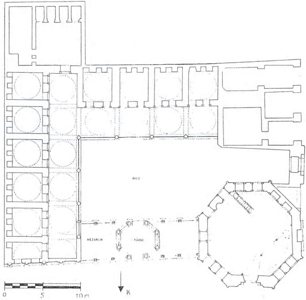
Plan.2.14. Köprülü Külliyesi Vaziyet Planı (A. Vefa Çobanoğlu'ndan)
