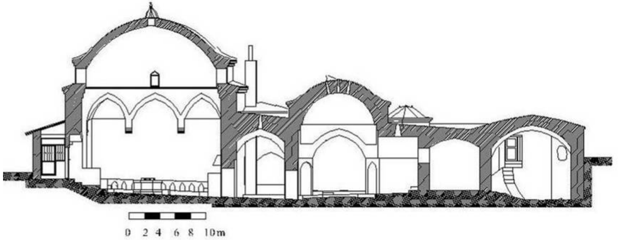
Plan.2.18. Vezirköprü Kale Hamamı B-B Kesiti (V.G.M.A.)
