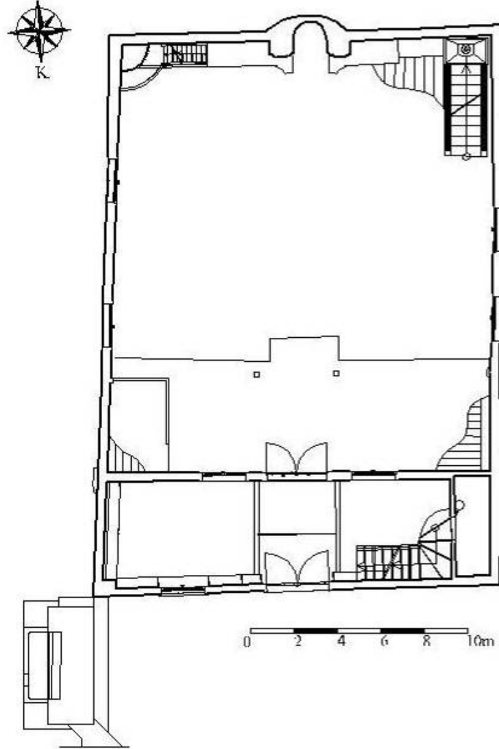
Plan.2.3. Vezirköprü Namazgah Camisi (V.G.M.A.)
