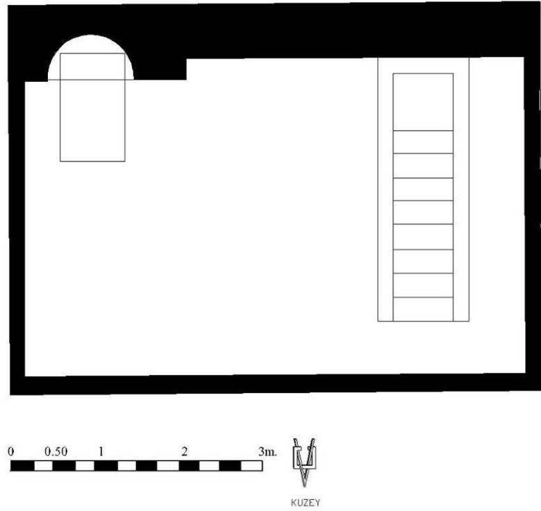
Plan 2.2. Vezirköprü Namazgah Camisi (M.Sami Bayraktar'dan)
