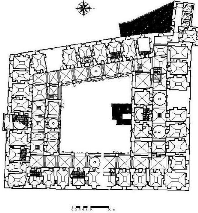
Plan. 2.30. Taşhan Üst Kat Planı (V.G.M.A.)
