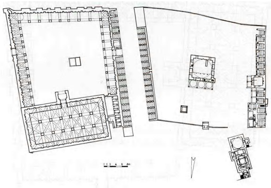
Plan.2.36. İncesu Merzifonlu Kara Mustafa Paşa Menzil Külliyesi Vaziyet Planı (Mustafa Denктаş'tan)
