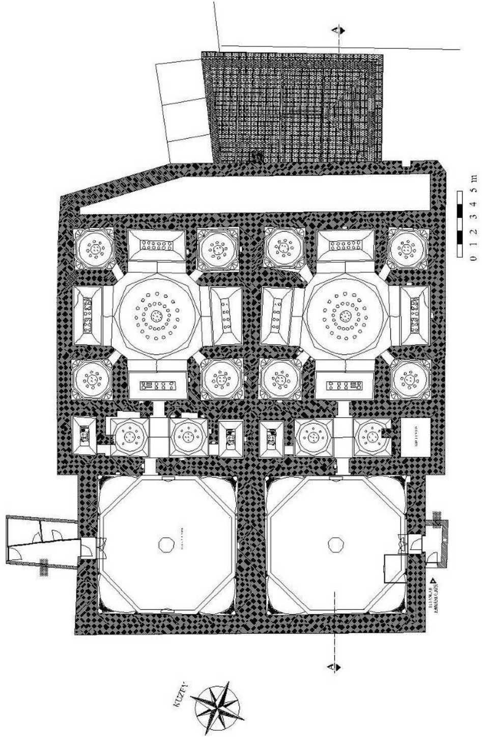
Plan.2.22. Vezirköprü Çifte Hamam (V.G.M.A.)
