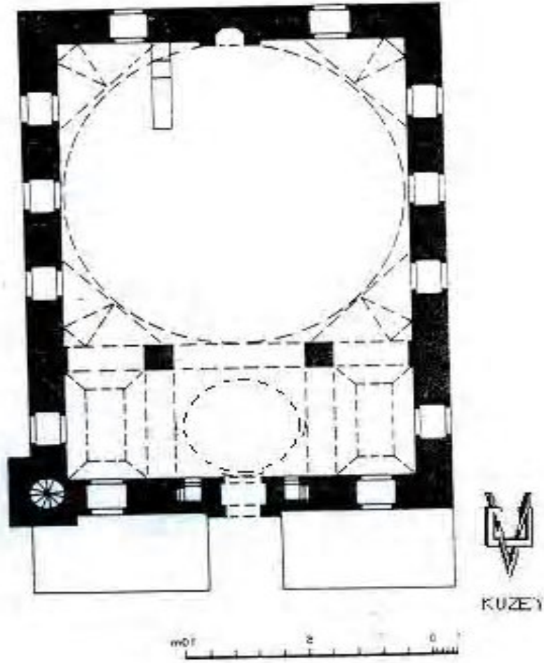
Plan.2.28. Merzifon Paşa Camisi (Goodwin'den)
