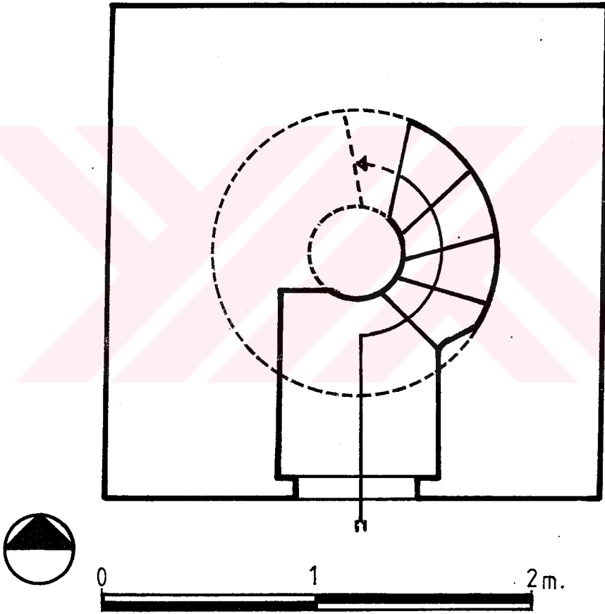
Lev.24 AKSARAY, Yıkık ( Sırçalı ) Minare, Rölöve Planı ( 1991, M. Meinecke' den Tamamlanarak )
