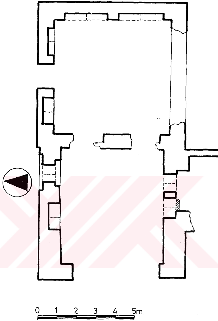
Lev.30 AKSARAY, II. Kılıç Arslan Köşkü?, Rölöve Planı
