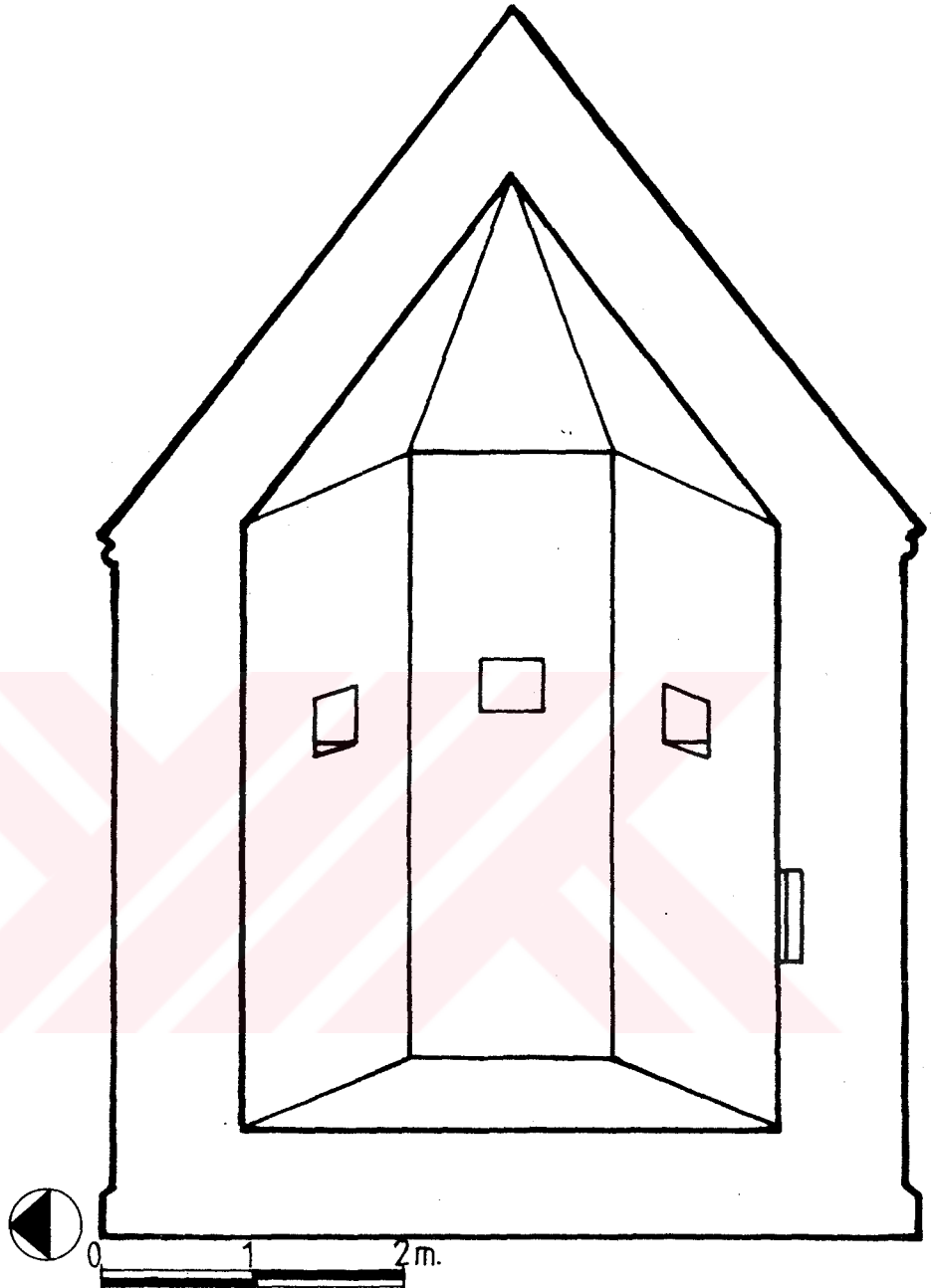
Lev.42 AKSARAY, Kılıç Arslan? Türbesi, Rölöve Kesidi (1974, İ.H. KONYALI)
