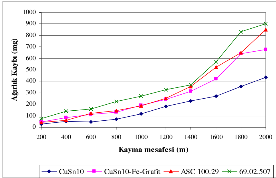
EK-B2. 0,44 m/sn ve 40N yük altında kayma mesafesi ağırlık kaybı değişimi
