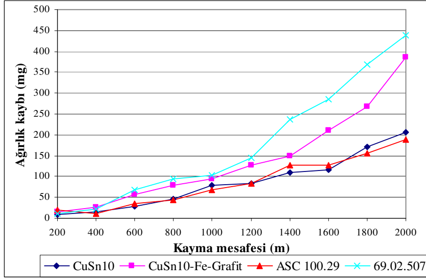
Şekil 10.19. 0,94 m/sn ve 10N yük altında kayma mesafesi ağırlık kaybı değişimi
