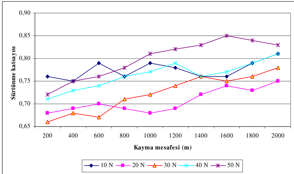
EK-J4. 69.02.507 yataklarına ait 0,94 m/sn'de yüke bağlı kayma mesafesi sürtünme katsayısı değişimi
