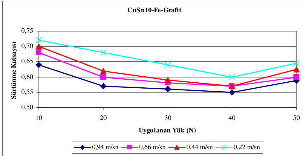
Şekil 10.10. CuSn10-Fe-Grafit yataklarına uygulanan yük ve sürtünme katsayısının hıza göre değişim grafiği
