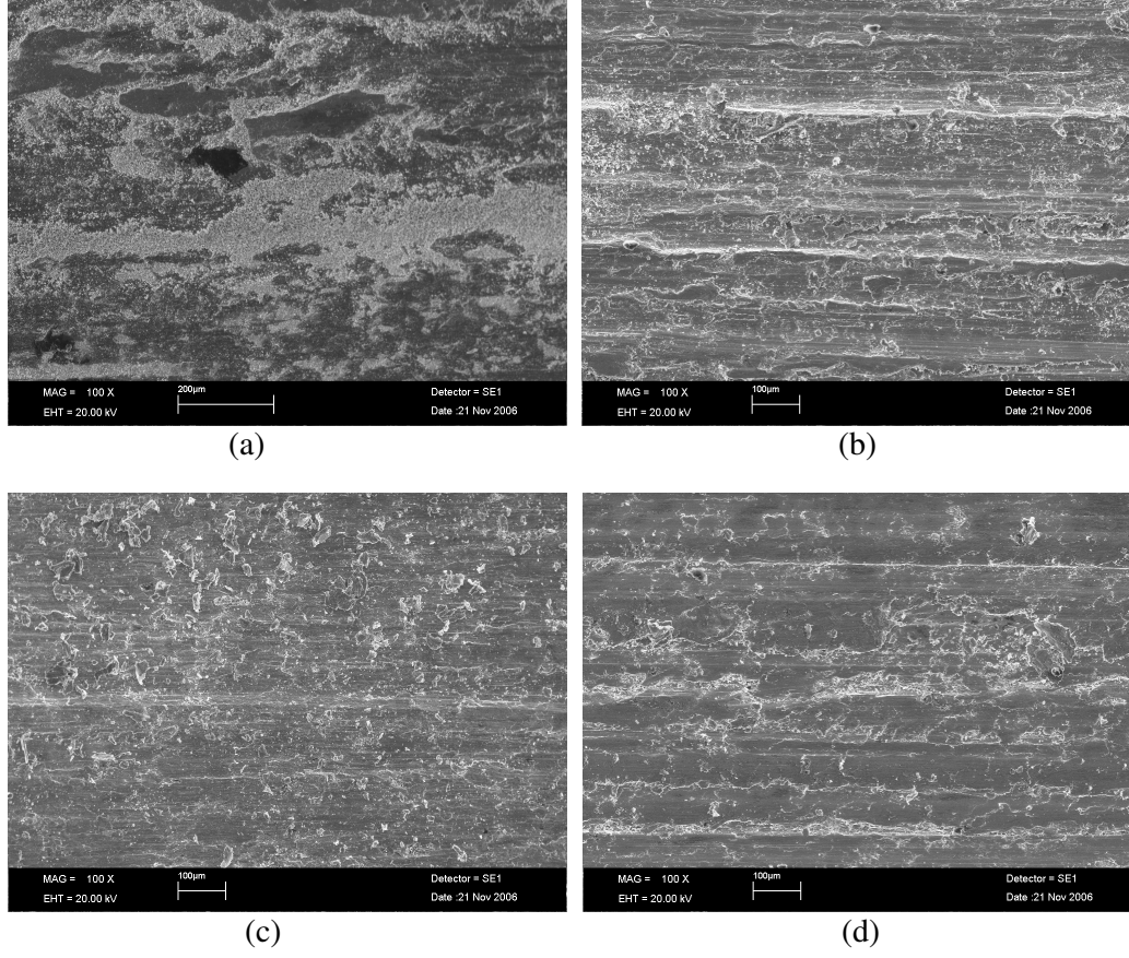
Şekil 10.35. 1100 d/dk ve 30 N yük altında çalışan numunelerin aşınma izleri
