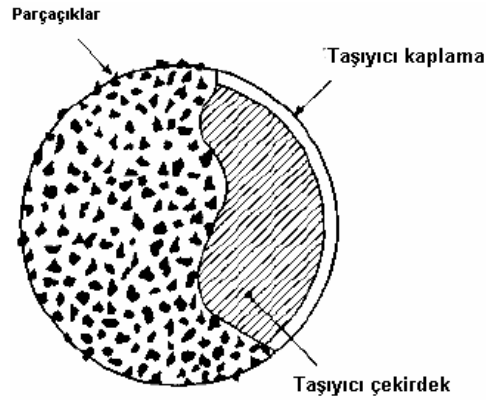
Şekil 7.7. Fotokopi tonerinin şekli (Saritaş 1992)
