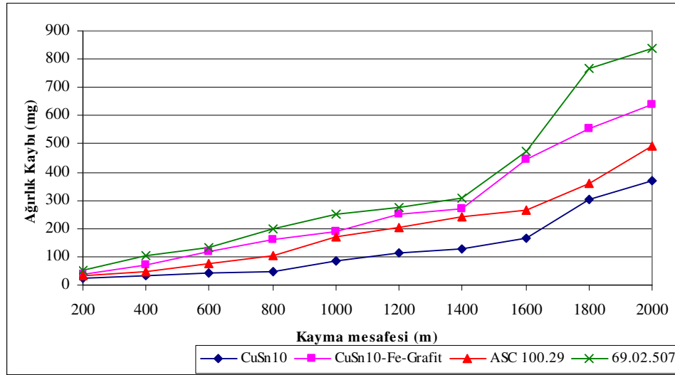
Şekil 10.16. 0,44 m/sn ve 30N yük altında kayma mesafesi ağırlık kaybı değişimi
