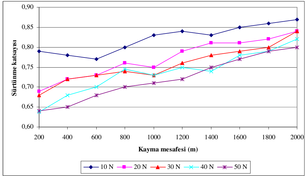
EK-H3.ASC 100.29 yataklarına ait 0,22 m/sn'de yüke bağlı kayma mesafesi Sürtünme katsayısı değişimi
