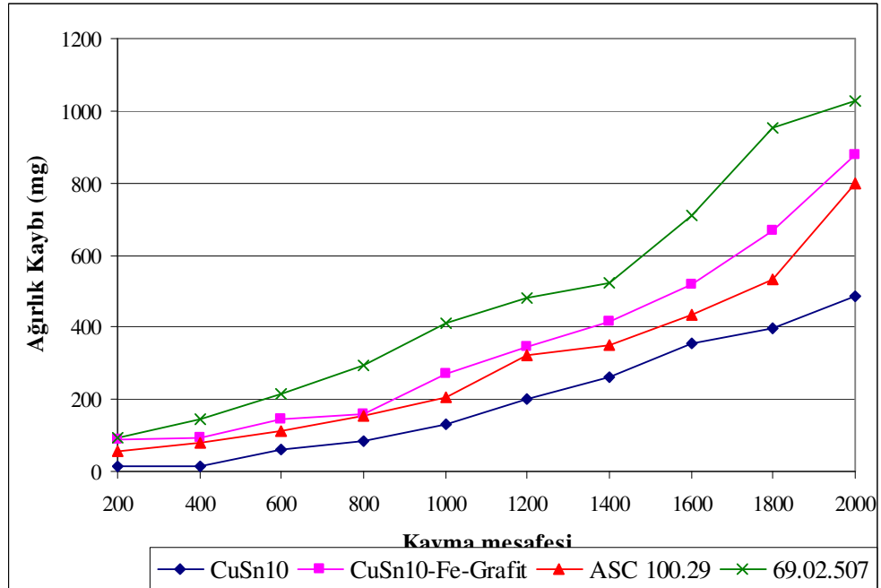
EK-C2 0,66 m/sn ve 40N yük altında kayma mesafesi ağırlık kaybı değişimi
