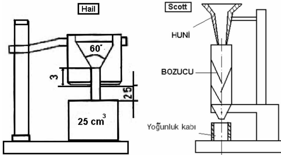
Şekil 4.3. Hail ve Scott akış hunileri (German, 1984)
