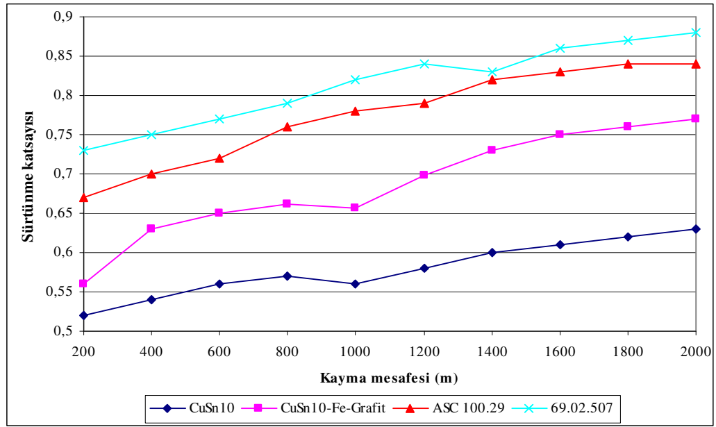
EK-G3. 0,66 m/sn ve 50 N yük altında kayma mesafesi sürtünme katsayısı değişimi
