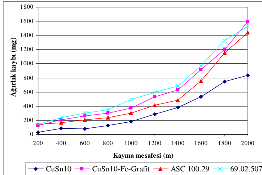
EK-D3. 0,94 m/sn ve 50N yük altında kayma mesafesi ağırlık kaybı değişimi
