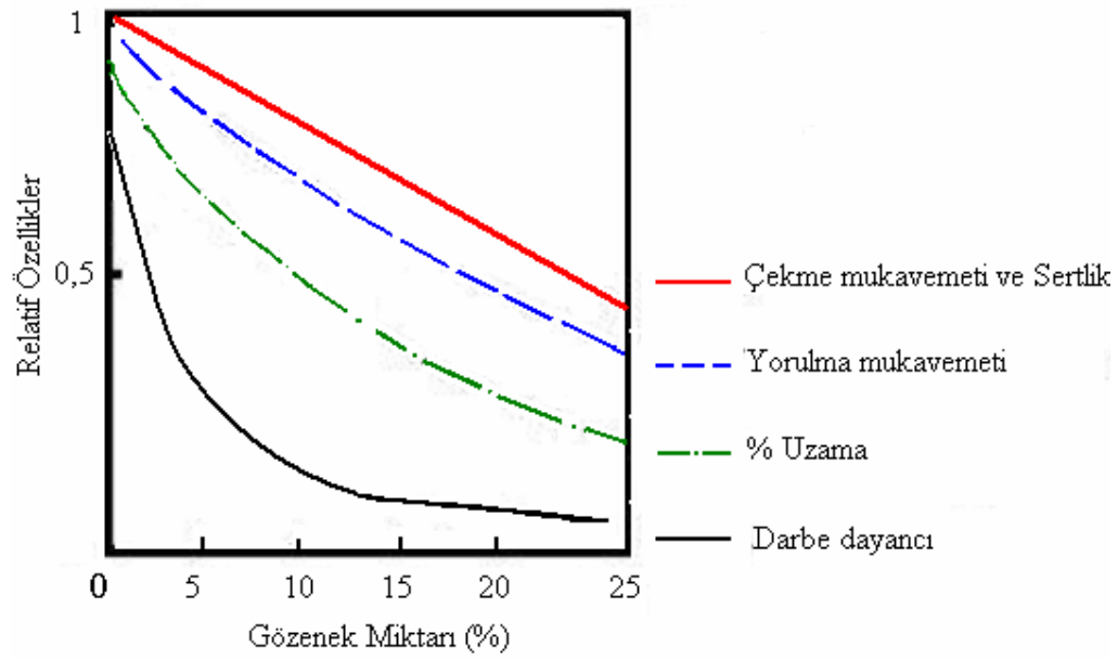
Şekil 6.15. Kalıcı gözeneğin mekanik özelliklere etkisi (TTMD)
