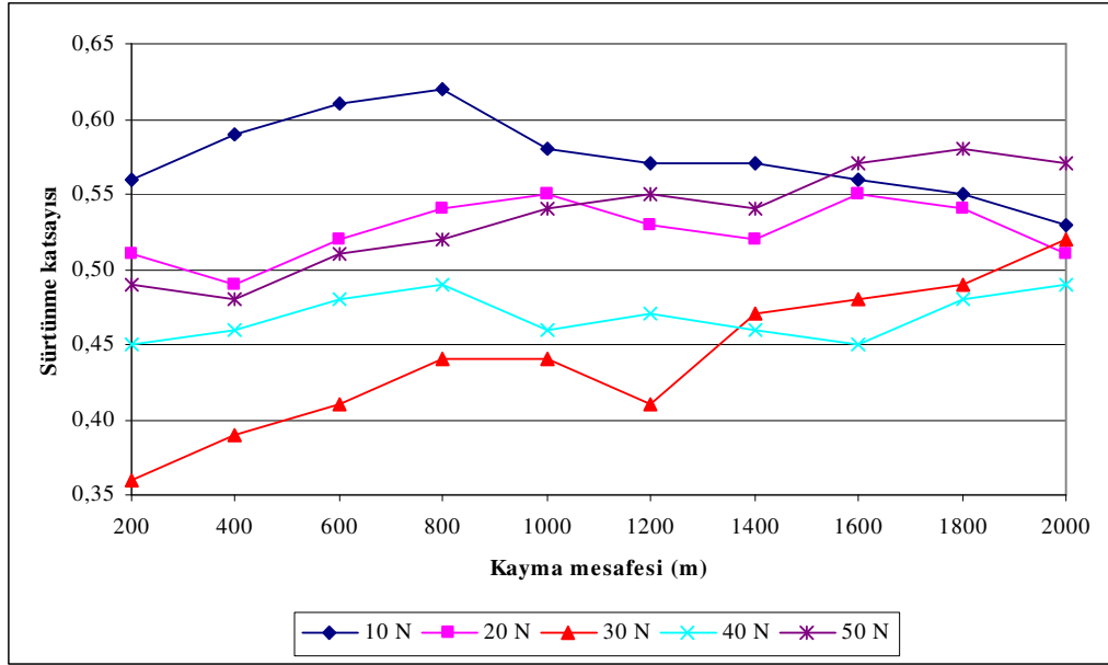
EK-J1. CuSn10 yataklarına ait 0,94 m/sn'de yüke bağlı kayma mesafesi sürtünme katsayısı değişimi
