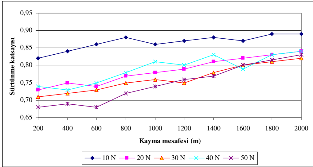
EK-I4. 69.02.507 yataklarına ait 0,44 m/sn’de yüke bağlı kayma mesafesi sürtünme katsayısı değişimi
