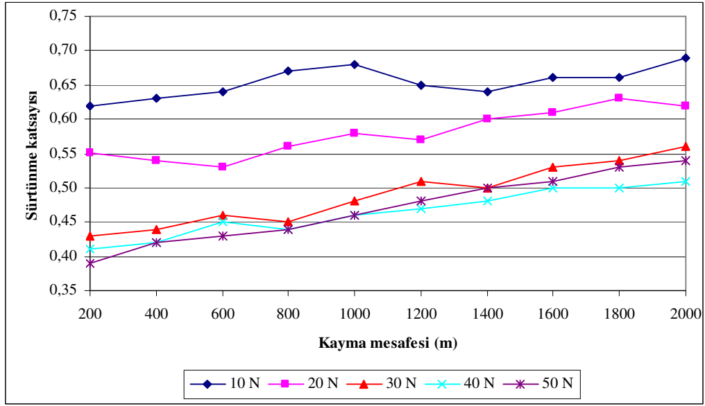
EK-I1. CuSn10 yataklarına ait 0,44 m/sn’de yüke bağlı kayma mesafesi sürtünme katsayısı değişimi
