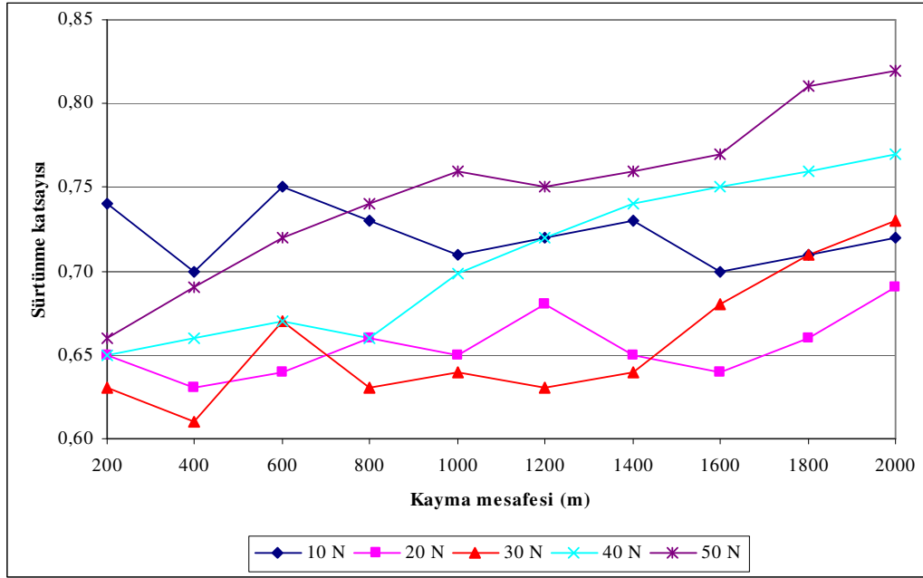
EK-J3.ASC 100.29 yatağına ait 0,94 m/sn'de yüke bağlı kayma mesafesi sürtünme katsayısı değişimi
