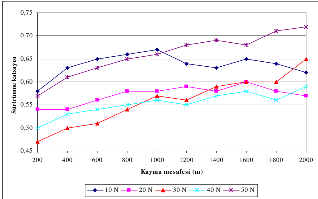
EK-J1. CuSn10 yataklarına ait 0,94 m/sn'de yüke bağlı kayma mesafesi sürtünme katsayısı değişimi
