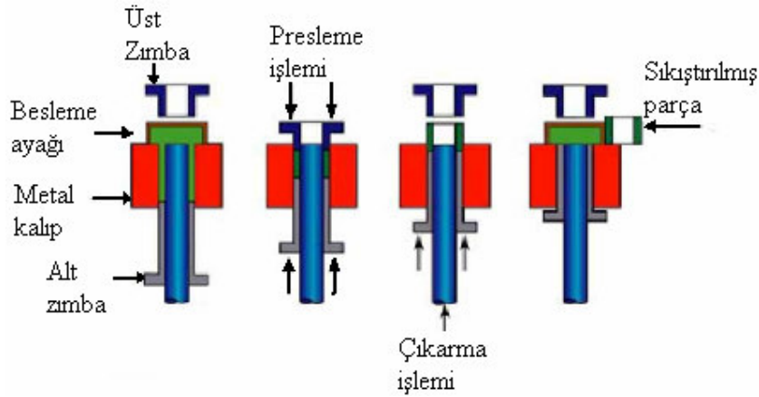
Şekil 7.9. Toz metalurjisi yöntemiyle yatak üretiminde sıkıştırma aşamaları
