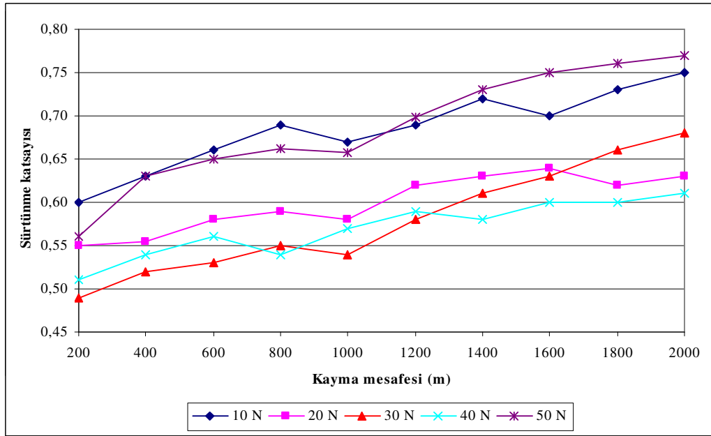
EK-İ2. CuSn10-Fe-Grafit yataklarına ait 0,66 m/sn’de yüke bağlı kayma mesafesi sürtünme katsayısı değişimi
