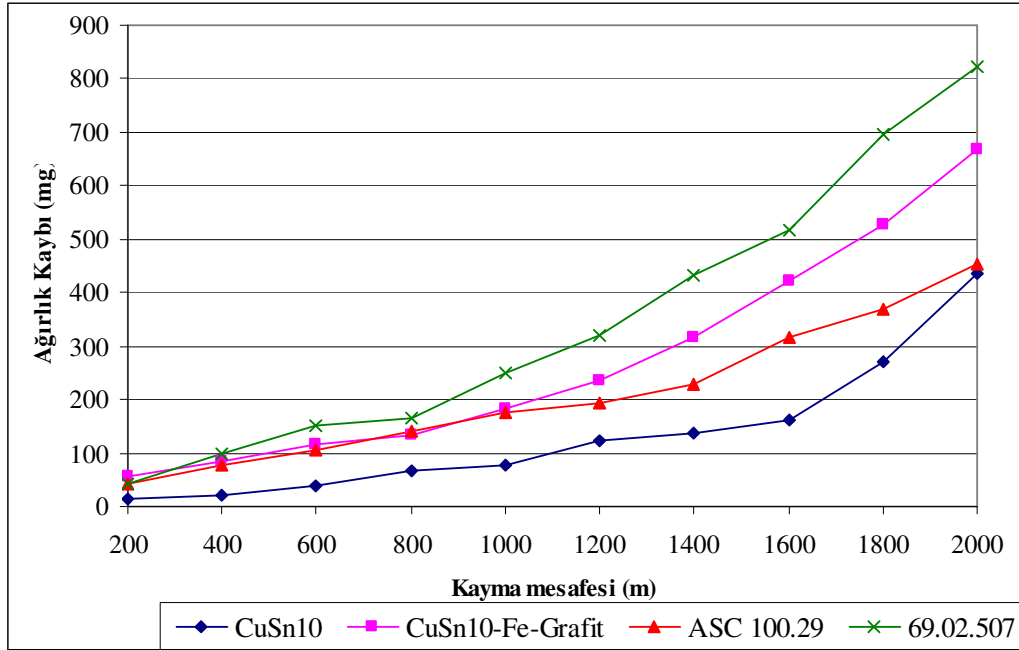
Şekil 10.14. 0,22 m/sn ve 30N yük altında kayma mesafesi ağırlık kaybı değişimi
