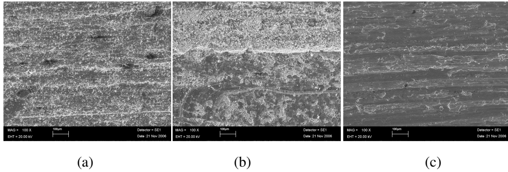
Şekil 10.39. 710 d/dk ve 30 N yük altında çalışan numunelerin aşınma izleri
