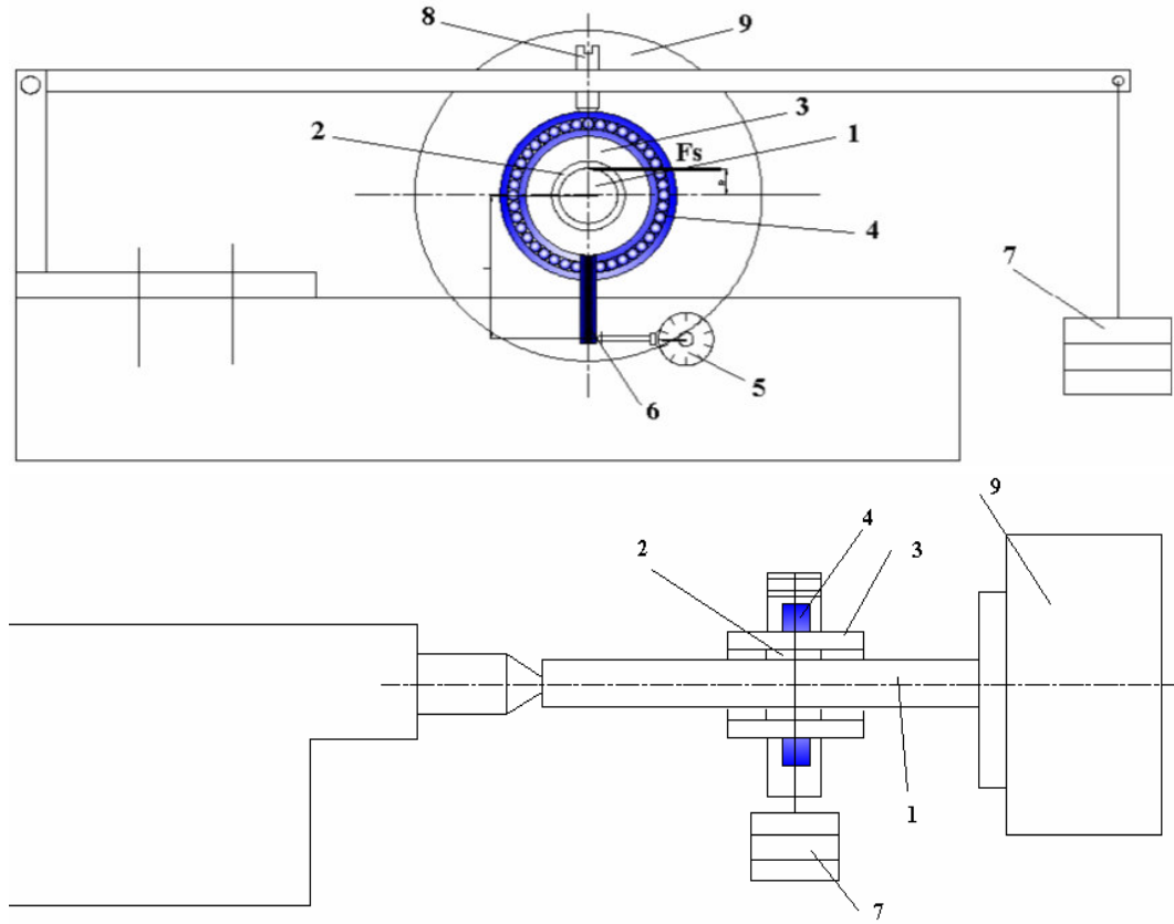
1.Aşındırıcı mil, 2.Kaymalı yatak numunesi, 3.Kaymalı yatak tutucusu, 4.Yük Temas Noktası (Rulman), 5. Komparetör, 6.Plaka, 7.Ağırlık, 8.Yük pimi, 9.Torna Aynası
