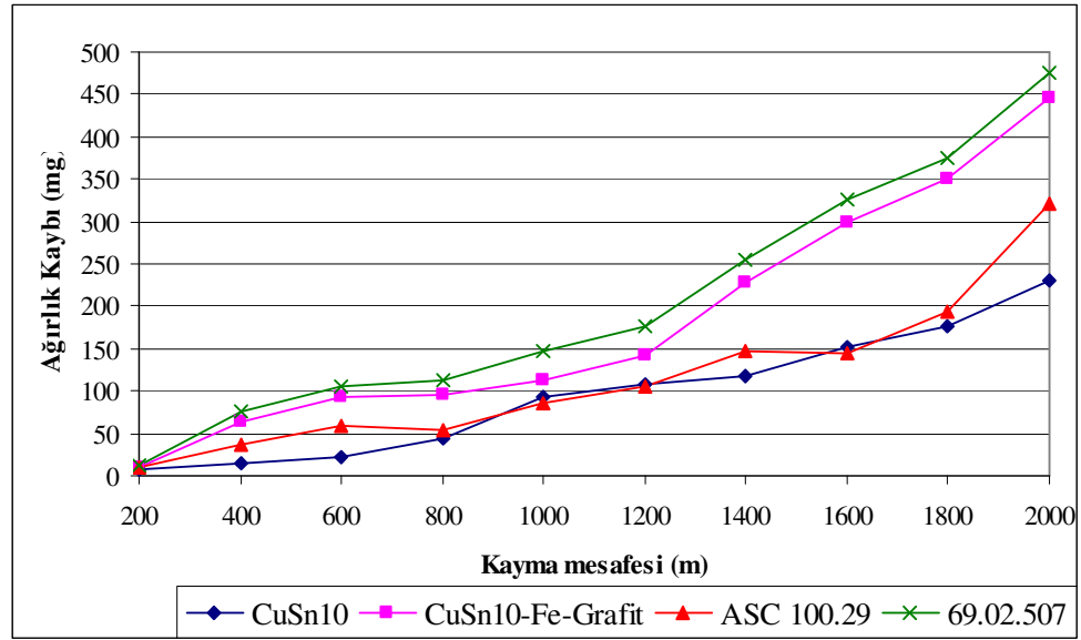
EK-C1. 0,66 m/sn ve 20N yük altında kayma mesafesi ağırlık kaybı değişimi
