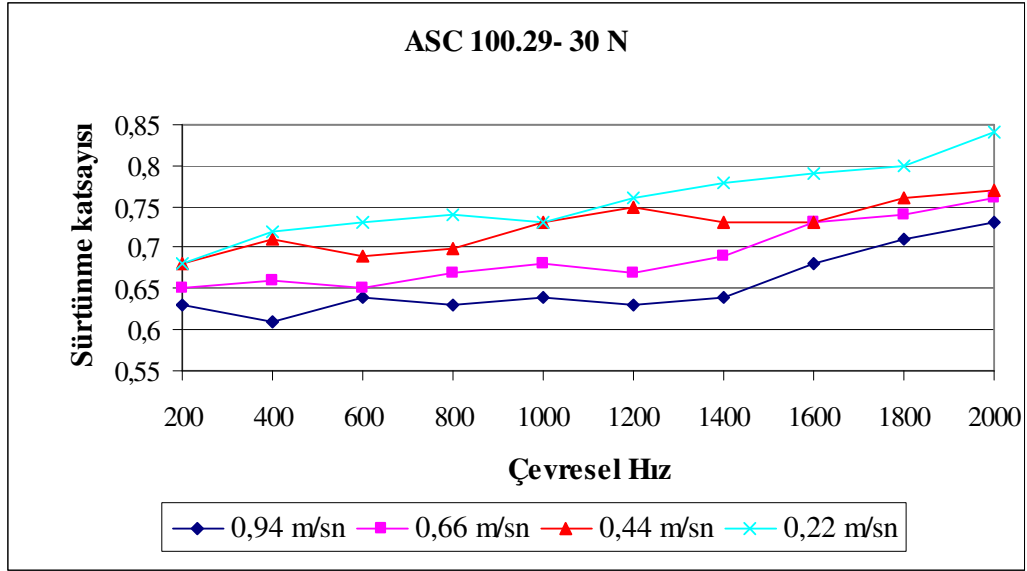
EK-K3. ASC 100.29 yataklarına ait çevresel hıza bağlı devir sayısı sürtünme katsayısı değişimi
