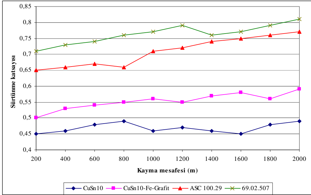
EK-Ğ2. 0,94 m/sn ve 40 N yük altında kayma mesafesi sürtünme katsayısı değişimi
