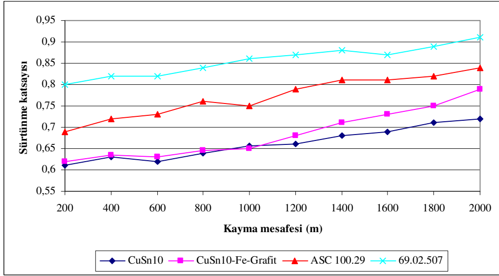
EK-E1. 0,22 m/sn ve 20 N yük altında kayma mesafesi sürtünme katsayısı değişimi.
