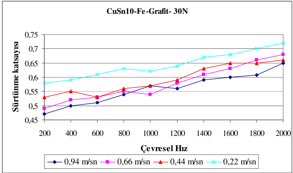
EK-K2. CuSn10-Fe-Grafit yataklarına ait çevresel hıza bağlı devir sayısı sürtünme katsayısı değişimi
