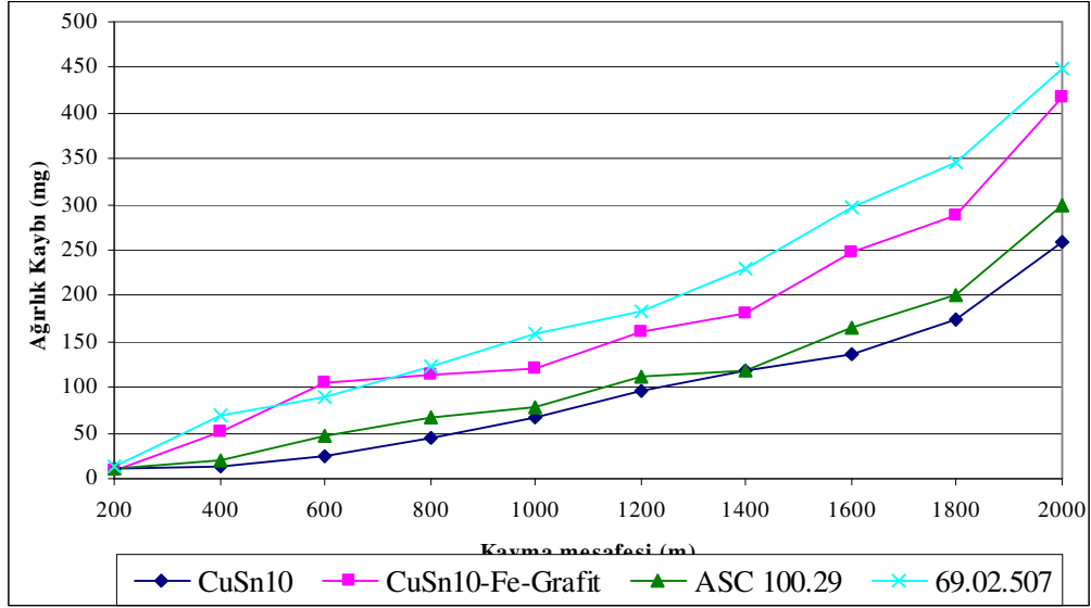
EK-A1. 0,22 m/sn ve 20N yük altında kayma mesafesi ağırlık kaybı değişimi
