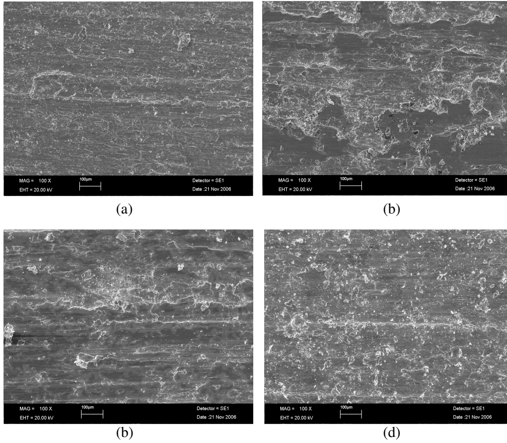
Şekil 10.38. 355 d/dk ve 50 N yük altında çalışan numunelerin aşınma izleri
