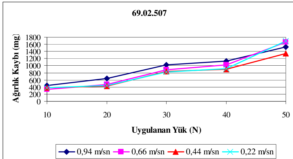
Şekil 10.8 69.02.507 yataklarına uygulanan yük ve ağırlık kaybının hızla göre değişimi
