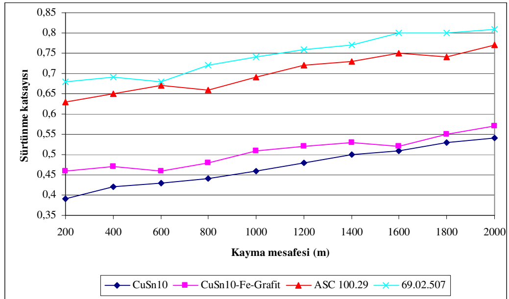
EK-F3. 0,44 m/sn ve 50 N yük altında kayma mesafesi sürtünme katsayısı değişimi
