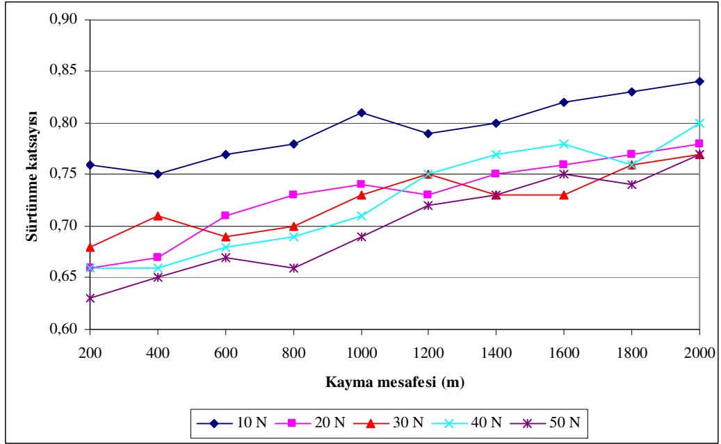
EK-I3.ASC 100.29 yataklarına ait 0,44 m/sn’de yüke bağlı kayma mesafesi sürtünme katsayısı değişimi
