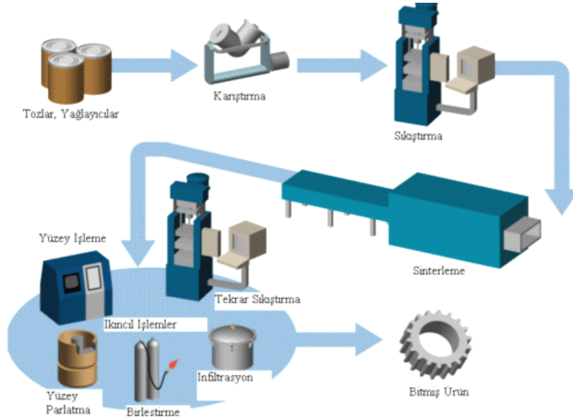
Şekil 1.1. Toz metal parça üretim aşamaları
