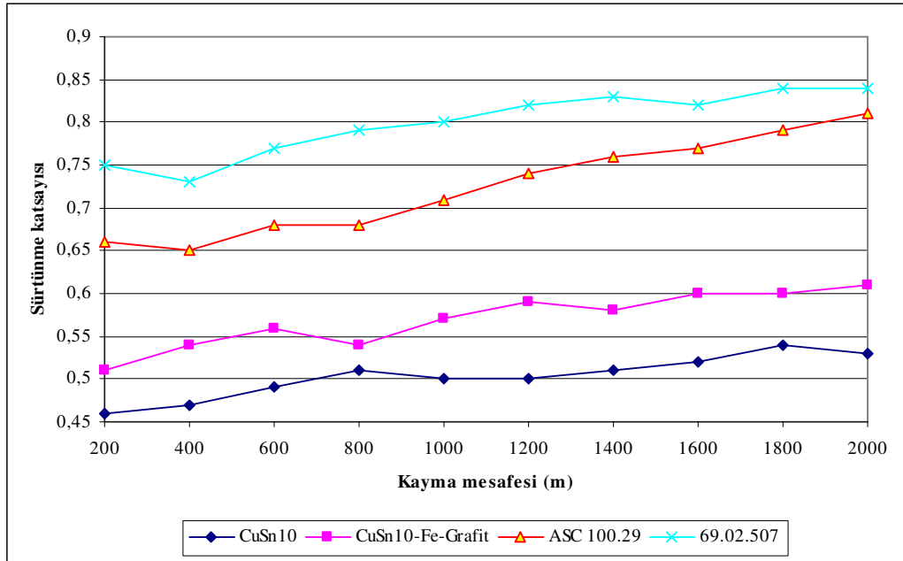
EK-G1. 0,66 m/sn ve 20 N yük altında kayma mesafesi sürtünme katsayısı değişimi
