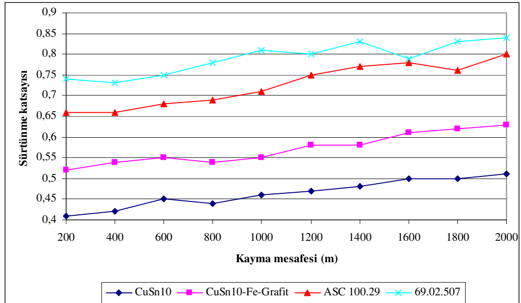
EK-F2. 0,44 m/sn ve 40 N yük altında kayma mesafesi sürtünme katsayısı değişimi
