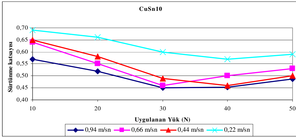
Şekil 10.9. CuSn10 yataklarına uygulanan yük ve sürtünme katsayısının hıza göre değişim grafiği
