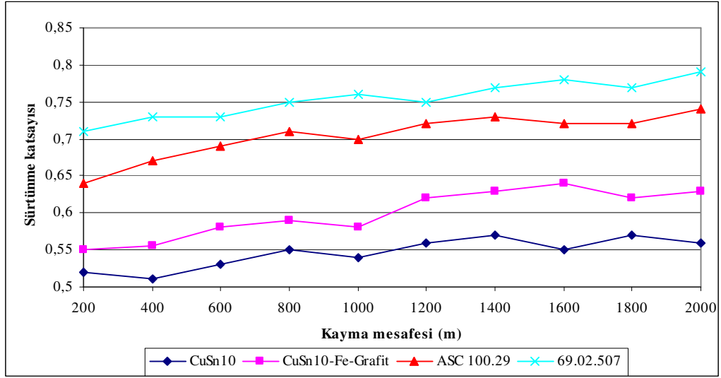
EK-G1. 0,66 m/sn ve 20 N yük altında kayma mesafesi sürtünme katsayısı değişimi
