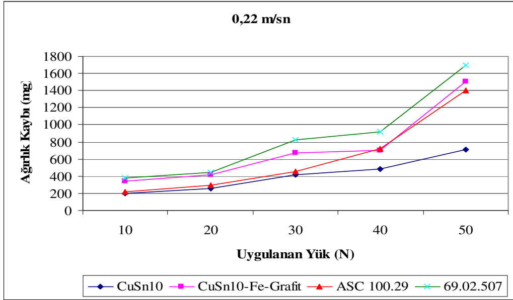
Şekil 10.4. 0,22 m/sn çevresel hızda T/M yatakların yük ağırlık kaybı ilişkisi
