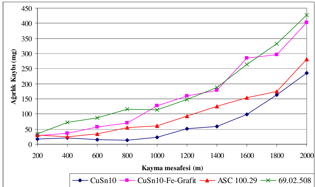
EK-B1. 0,44 m/sn ve 20N yük altında kayma mesafesi ağırlık kaybı değişimi
