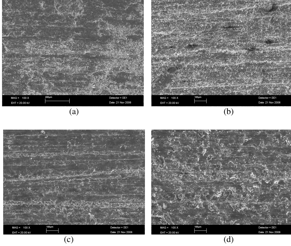
Şekil 10.40. 710 d/dk ve 20 N yük altında çalışan numunelerin aşınma izleri
