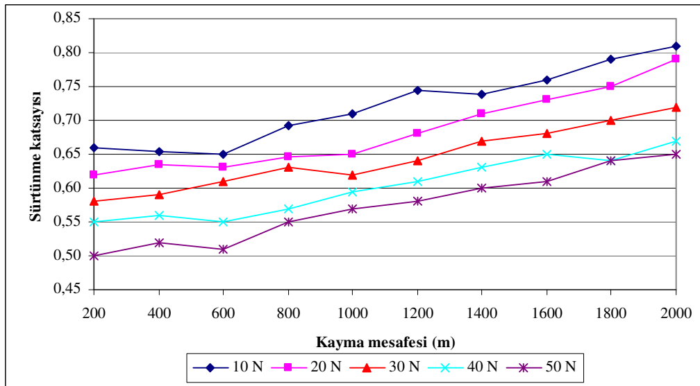
EK-H2. CuSn10-Fe-Grafit yataklarına ait 0,22 m/sn’de yüke bağlı kayma mesafesi sürtünme katsayısı değişimi
