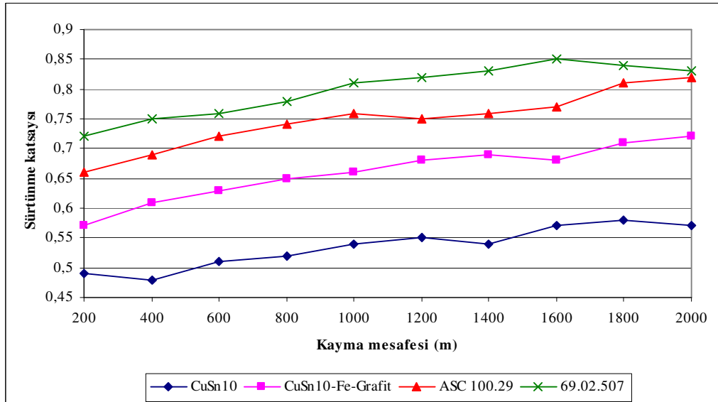
EK-Ğ3. 0,94 m/sn ve 50 N yük altında kayma mesafesi sürtünme katsayısı değişimi
