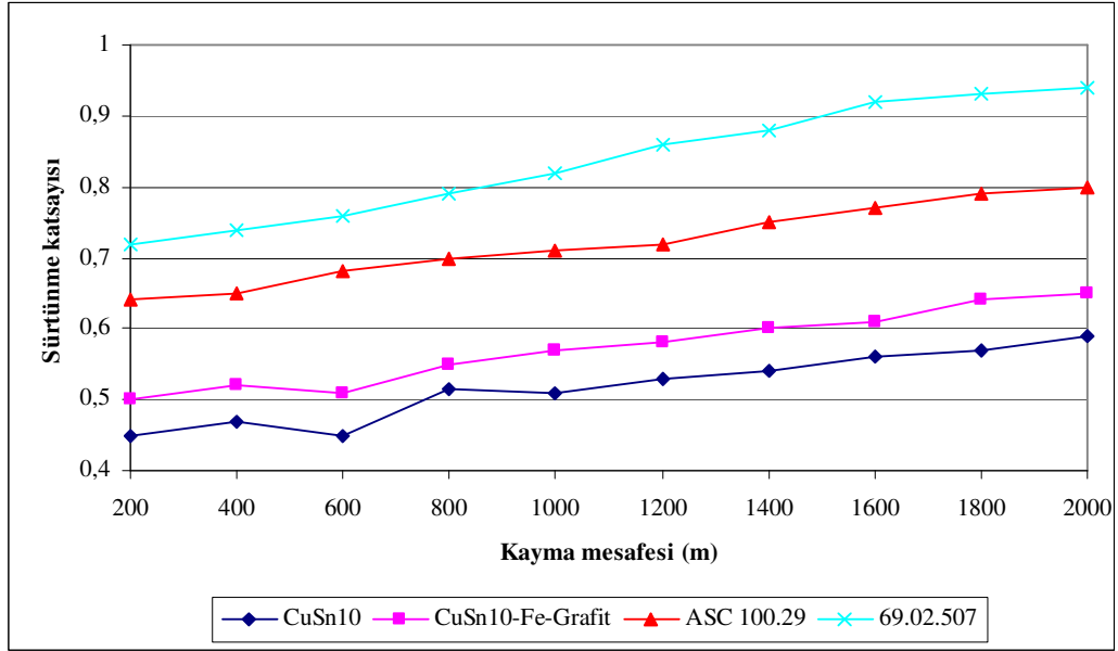
EK-E3. 0,22 m/sn ve 50 N yük altında kayma mesafesi sürtünme katsayısı değişimi.
