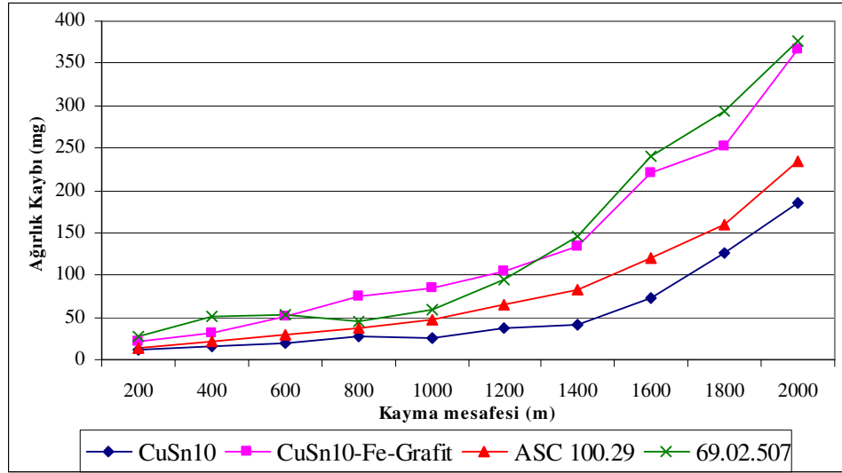
Şekil 10.15. 0,44 m/sn ve 10N yük altında kayma mesafesi ağırlık kaybı değişimi
