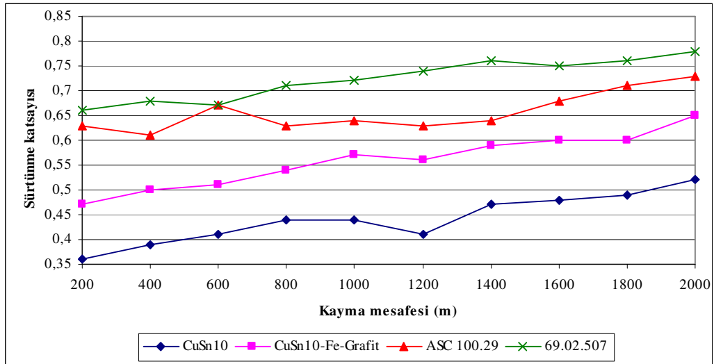
Şekil 10.28. 0,94 m/sn ve 30 N yük altında kayma mesafesi sürtünme katsayısı değişimi
