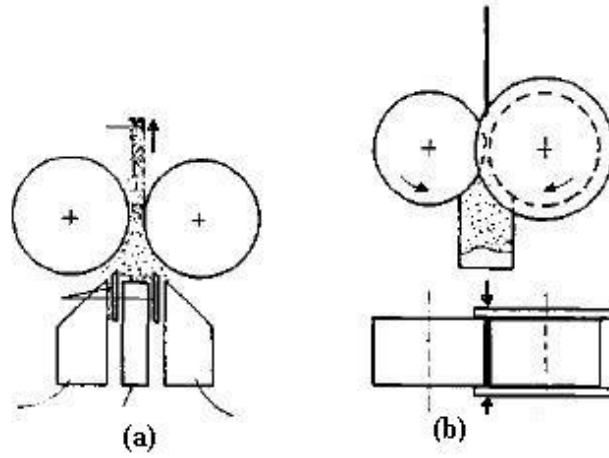
Şekil 6.7. Toz haddeleme: (a) Tek metal, (b) İki metal
