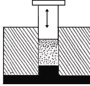
Şekil 6.3. Tek etkili presleme
