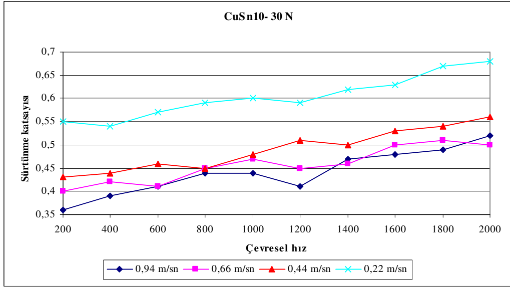
EK-K1. CuSn10 yataklarına ait çevresel hıza bağlı devir sayısı sürtünme katsayısı değişimi
