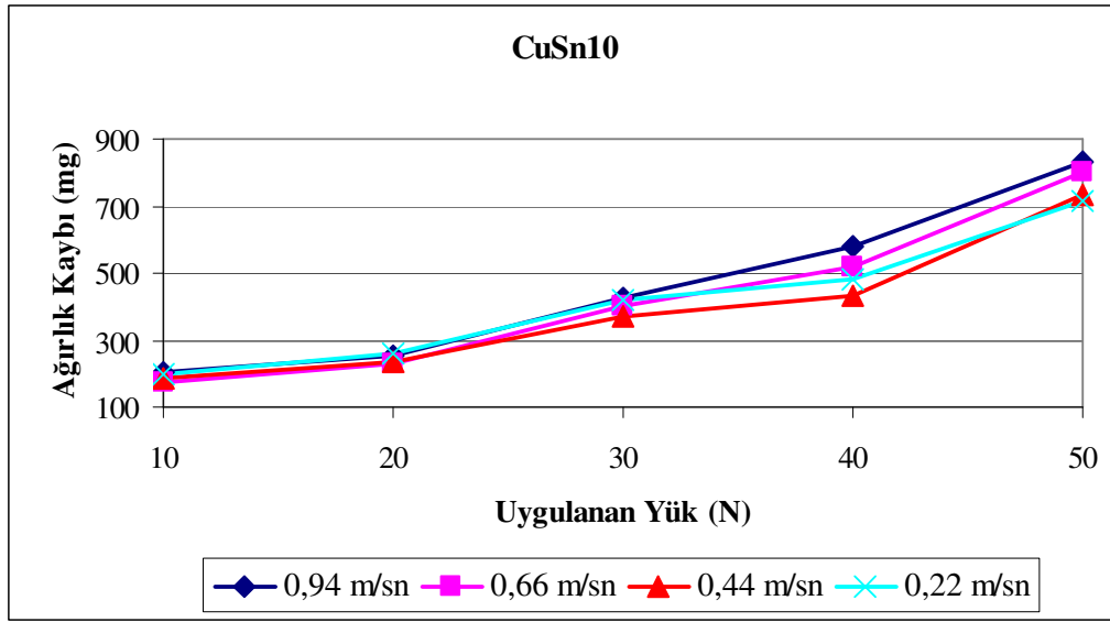
Şekil 10.5. CuSn10 yataklarına uygulanan yük ve ağırlık kaybının hıza göre değişimi
