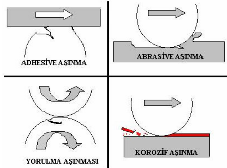
Şekil 8.1. Dört aşınma tipinin şematik gösterimi (Yıldız, 2006)
