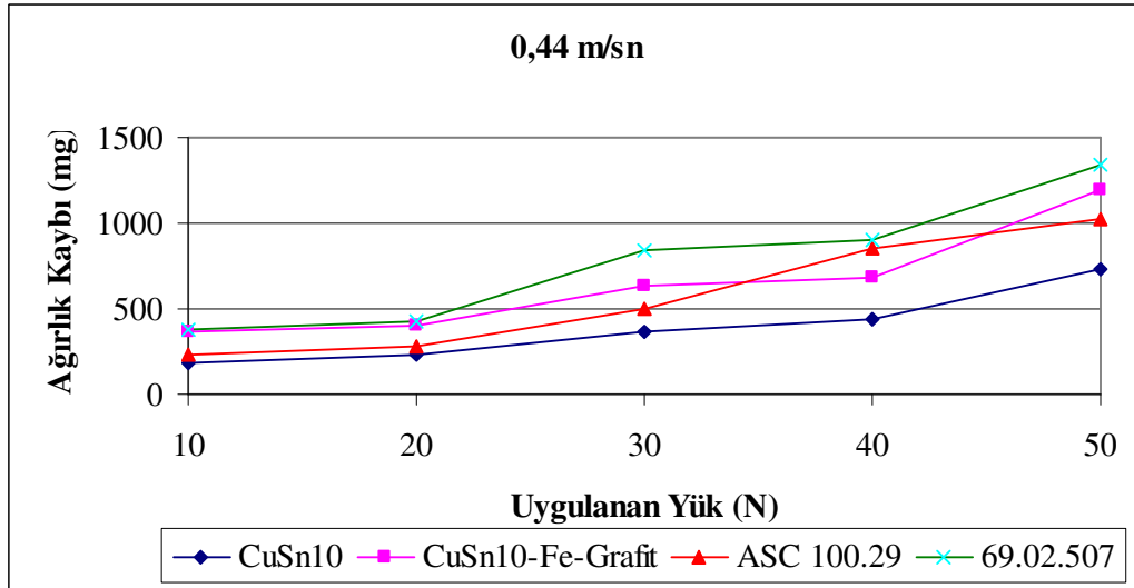
Şekil 10.3. 0,44 m/sn çevresel hızda T/M yatakların yük ağırlık kaybı ilişkisi
