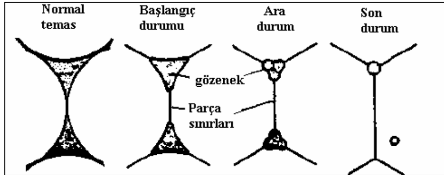
Şekil 6.8. Sinterlemenin mikroyapıya etkisi (German, 1990)
