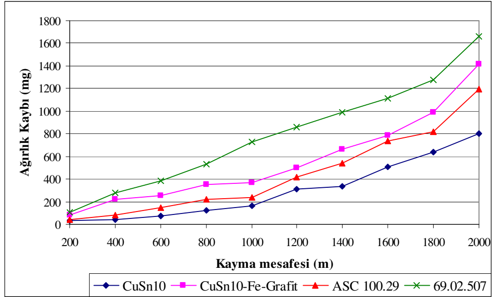
EK-C3. 0,66 m/sn ve 50N yük altında kayma mesafesi ağırlık kaybı değişimi
