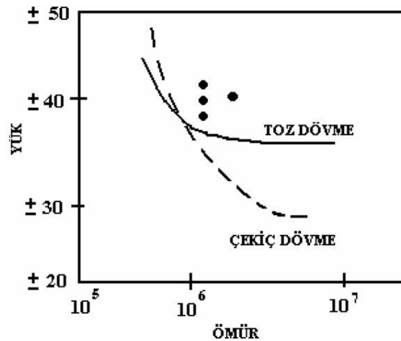
Şekil 6.14. Dövme ve T/M biyel kollarının yorulma özelliklerinin karşılaştırılması (Saritaş,1985)
