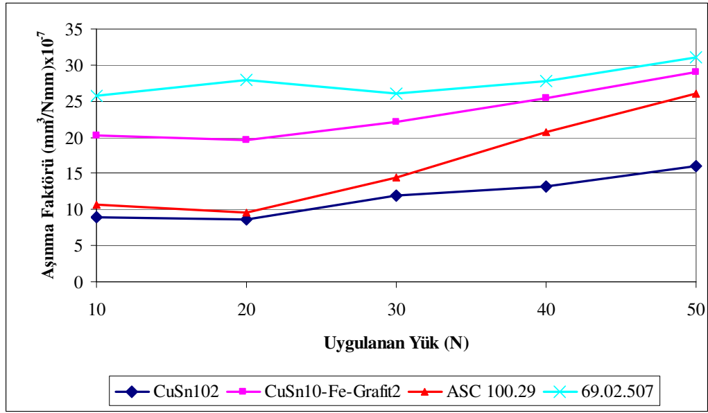
Şekil 10.31. 2000 m'lik kayma mesafesi V:0.44 m/sn'de aşınma faktörü yük değişimi
