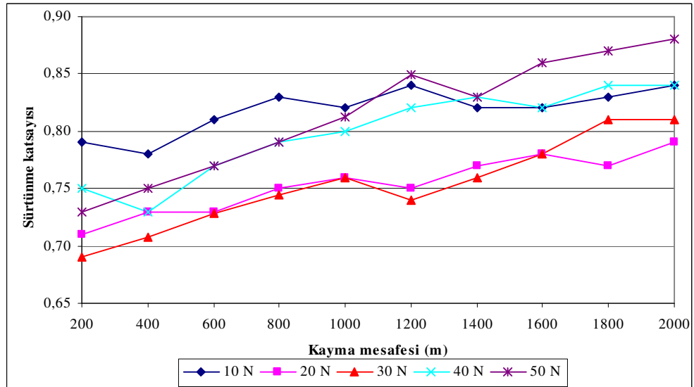
EK-İ4. 69.02.507 yataklarına ait 0,66 m/sn'de yüke bağlı kayma mesafesi sürtünme katsayısı değişimi
