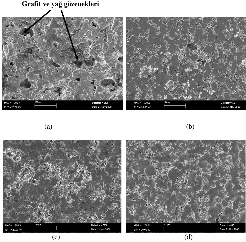
Şekil 10.34. Deney yapılmamış numunelerin mikro yapıları
