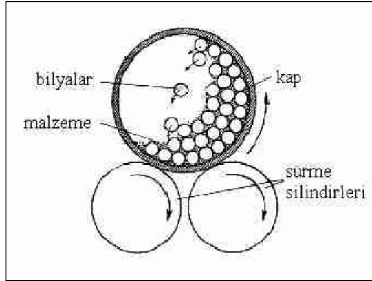
Şekil 5.4. Mekanik öğütme metodu
