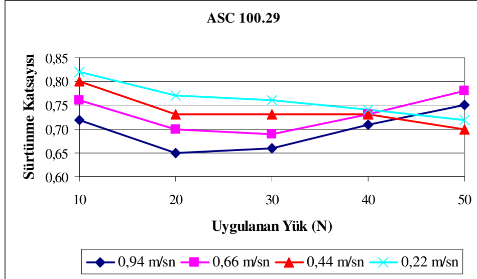
Şekil 10.11. ASC 100.29 yataklarına uygulanan yük ve sürtünme katsayısının hızla göre değişim grafiği
