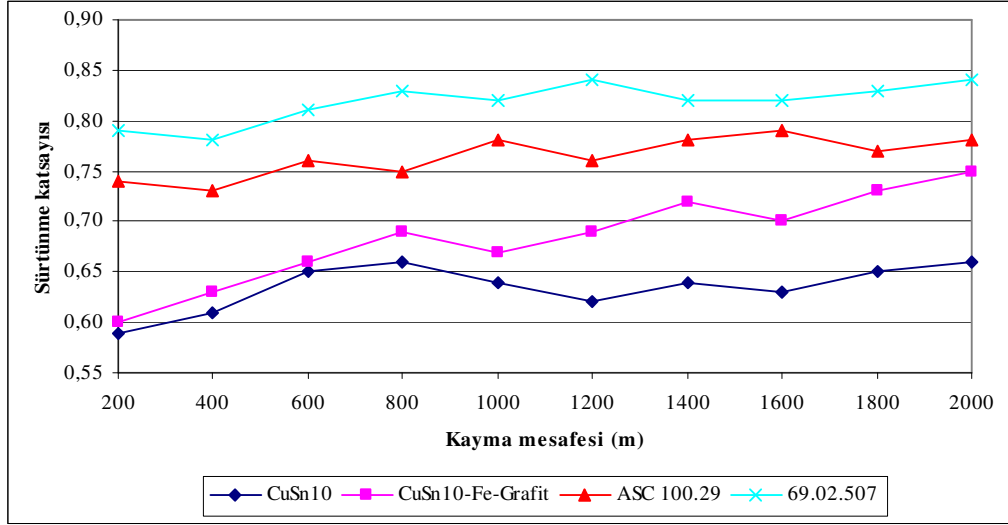
Şekil 10.25. 0,66 m/sn ve 10 N yük altında kayma mesafesi sürtünme katsayısı değişimi
