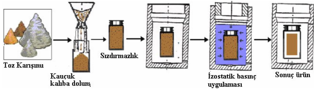
Şekil 6.5. Soğuk İzostatik presleme işlem adımları
