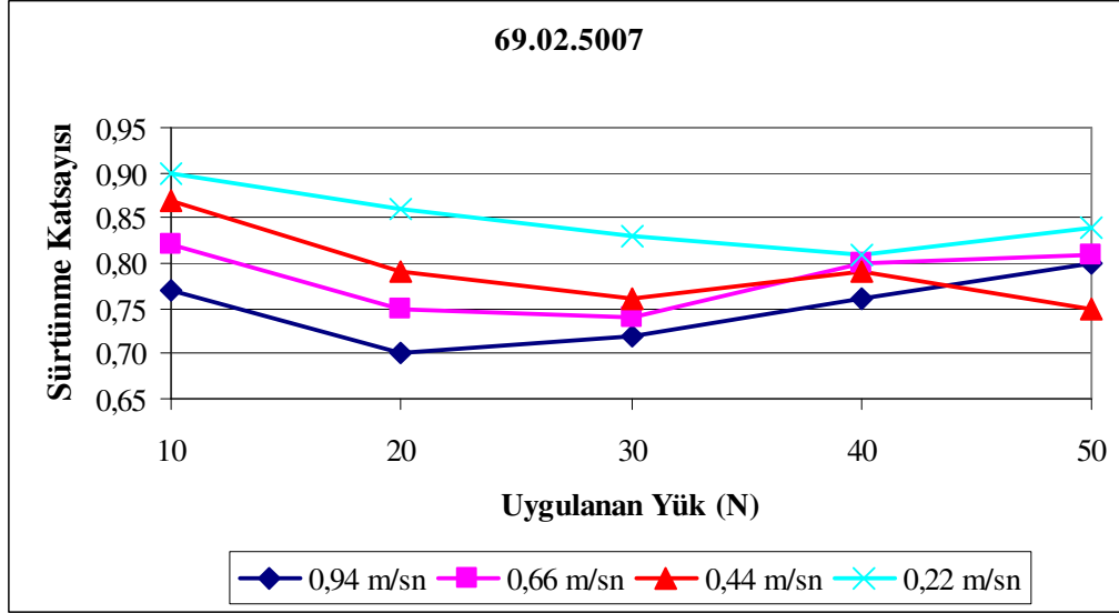
Şekil 10.12. 69.02.507 yataklarına uygulanan yük ve sürtünme katsayısının hıza göre değişim grafiği
