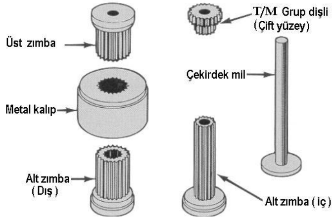
Şekil 6.4. Çift yönlü çalışan bir pres tertibatı parçaları
