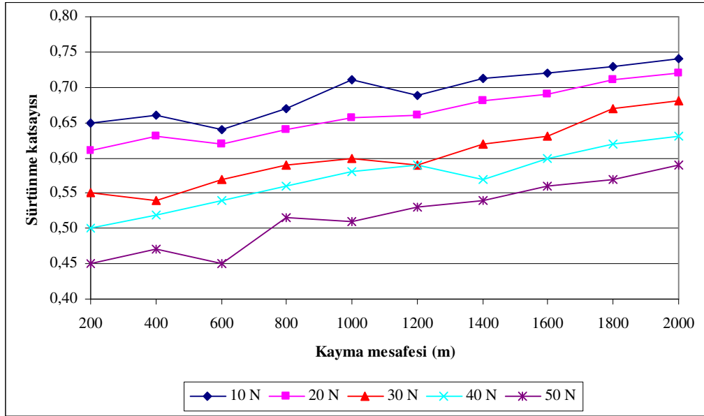
EK-H1. CuSn10 yataklarına ait 0,22 m/sn’de yüke bağlı kayma mesafesi sürtünme katsayısı değişimi
