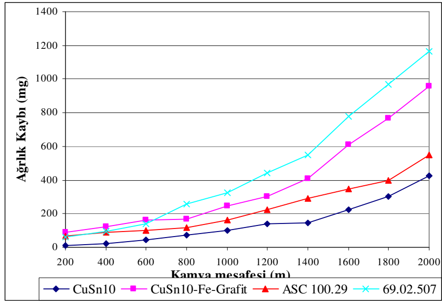
EK-D2. 0,94 m/sn ve 40N yük altında kayma mesafesi ağırlık kaybı değişimi
