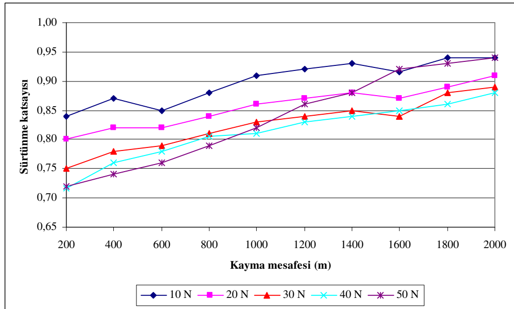
EK-H4. 69.02.507 yataklarına ait 0,22 m/sn'de yüke bağlı kayma mesafesi sürtünme katsayısı değişimi
