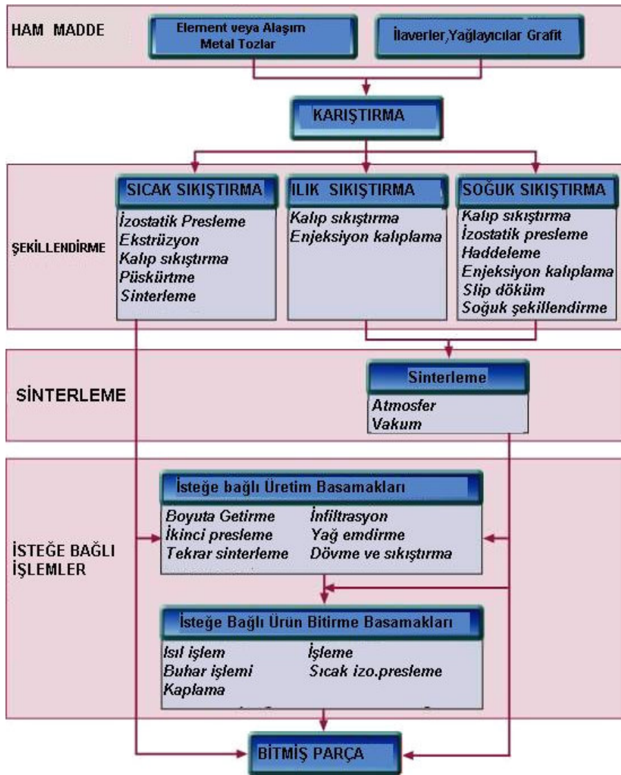
Şekil 6.13. Toz metal prosesinde işlem adımları
