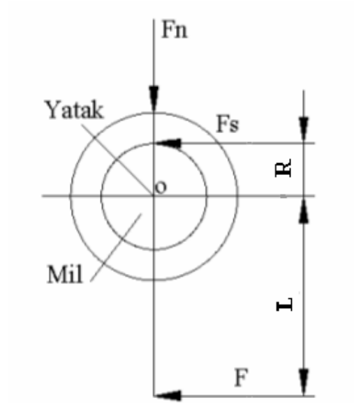
Şekil 9.4. Kaymalı yatakta sürtünme kuvvetinin oluşumu
