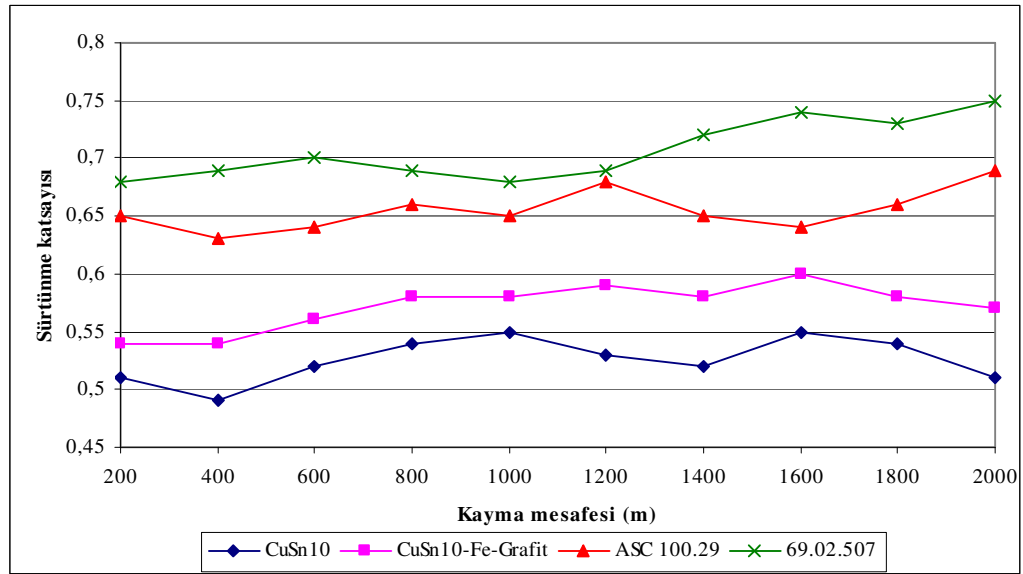
EK-Ğ1. 0,94 m/sn ve 20 N yük altında kayma mesafesi sürtünme katsayısı değişimi
