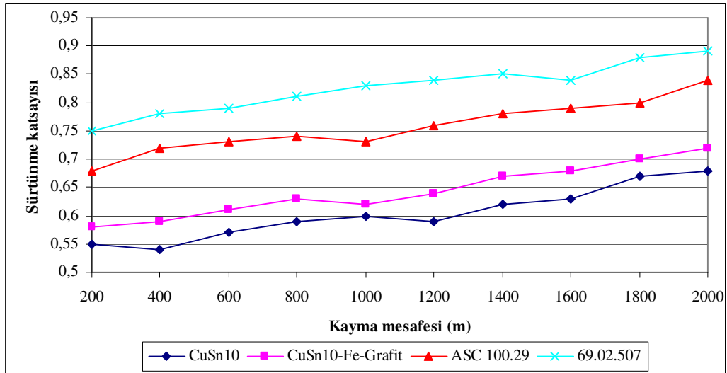
Şekil 10.22. 0,22 m/sn ve 30 N yük altında kayma mesafesi sürtünme katsayısı değişimi
