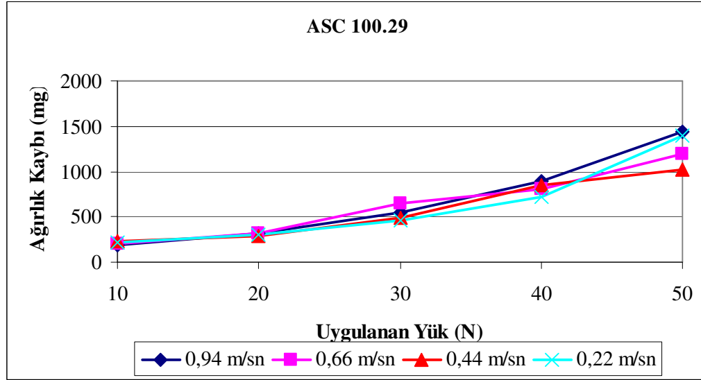
Şekil 10.7 ASC 100.29 yataklarına uygulanan yük ve ağırlık kaybının hızla göre değişimi
