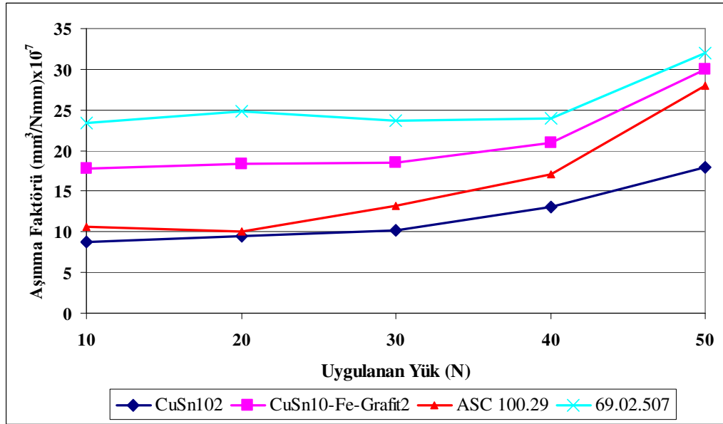
Şekil 10.32. 2000 m'lik kayma mesafesi V:0.22 m/sn'de aşınma faktörü ile yük değişimi
