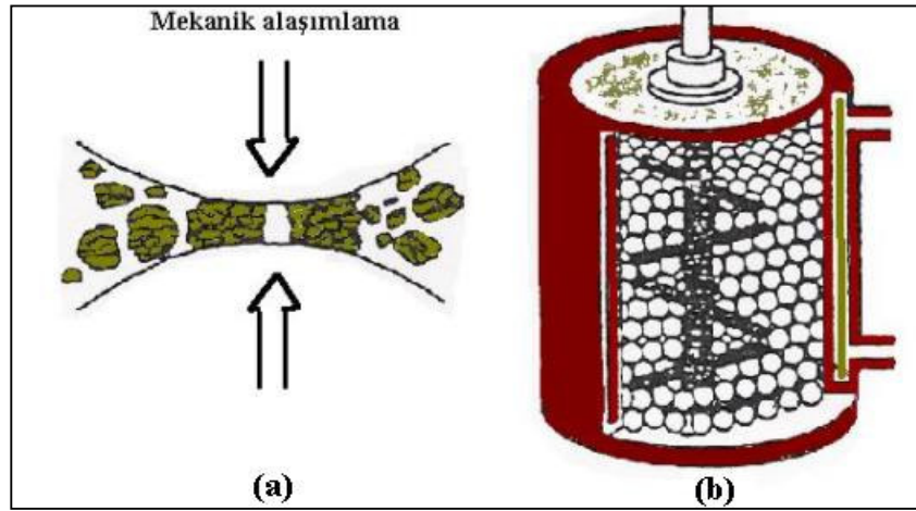
Şekil 5.5. a) Mekanik alaşımlamada toz/toz etkisi b) Atrinörün şematik görünümü
