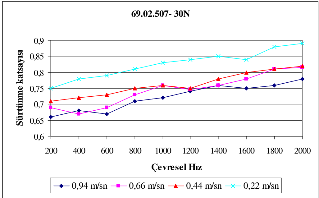
EK-K4. 69.02.507 yataklarına ait çevresel hıza bağlı devir sayısı sürtünme katsayısı değişimi
