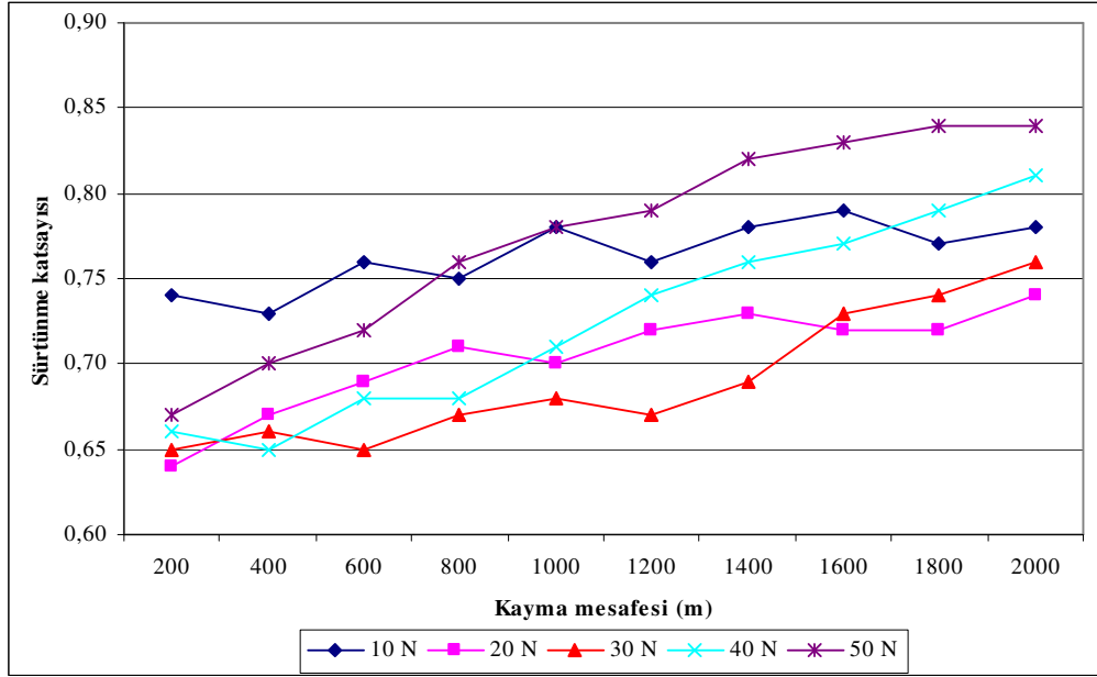
EK-İ3.ASC 100.29 yatağına ait 0,66 m/sn'de yüke bağlı kayma mesafesi sürtünme katsayısı değişimi
