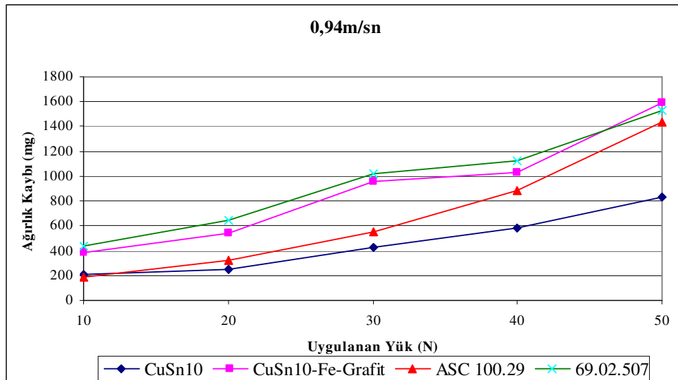
Şekil 10.1. 0,94 m/sn çevresel hızda T/M yatakların yük ağırlık kaybı ilişkisi
