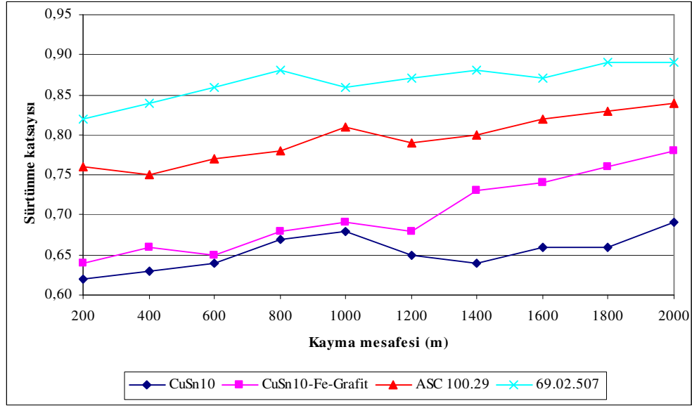
Şekil 10.23. 0,44 m/sn ve 10 N yük altında kayma mesafesi sürtünme katsayısı değişimi
