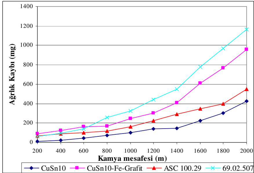
Şekil 10.20. 0,94 m/sn ve 30N yük altında kayma mesafesi ağırlık kaybı değişimi
