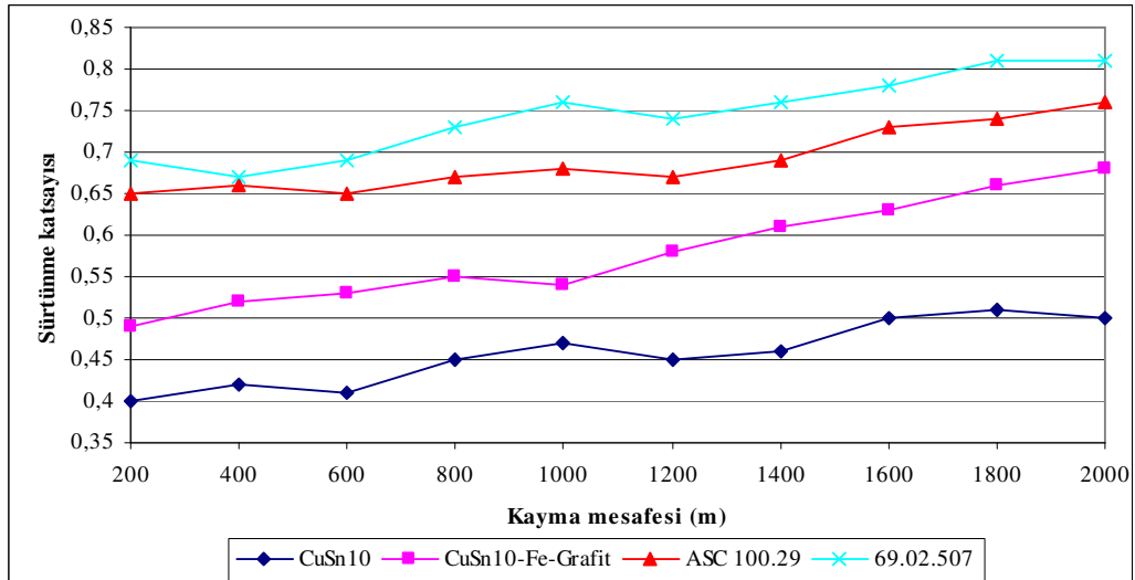
Şekil 10.26. 0,66 m/sn ve 30 N yük altında kayma mesafesi sürtünme katsayısı değişimi
