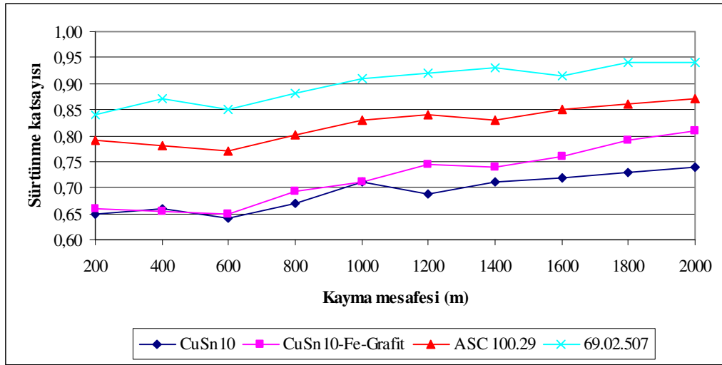
Şekil 10.21. 0,22 m/sn ve 10 N yük altında kayma mesafesi sürtünme katsayısı değişimi
