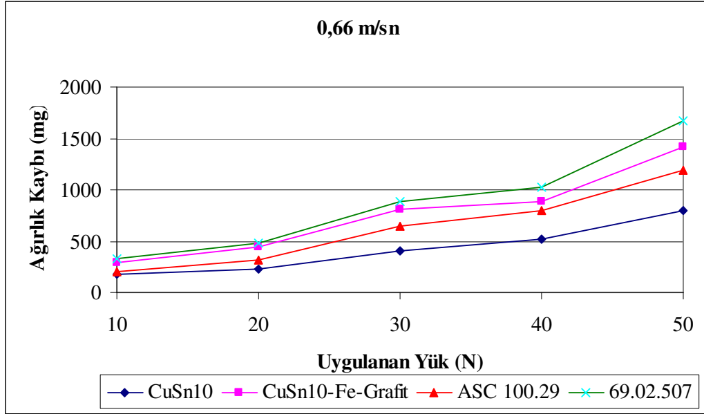
Şekil 10.2. 0,66 m/sn çevresel hızda T/M yatakların yük ağırlık kaybı ilişkisi
