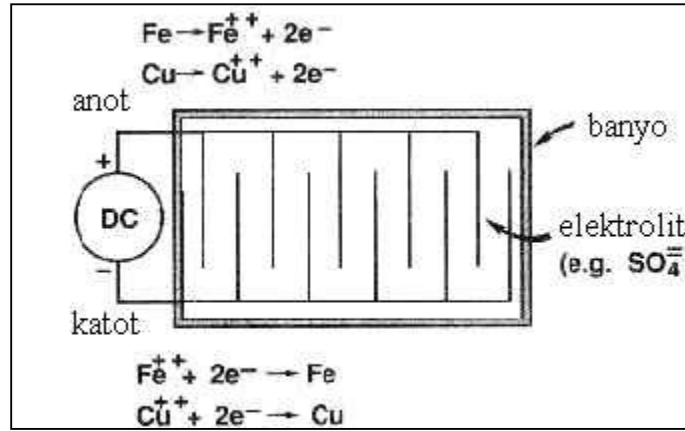
Şekil 5.1. Elektroliz hücresi şeması (German, 1984)
