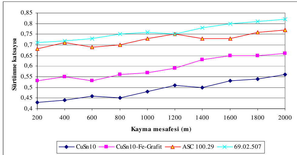
Şekil 10.24. 0,44 m/sn ve 30 N yük altında kayma mesafesi sürtünme katsayısı değişimi
