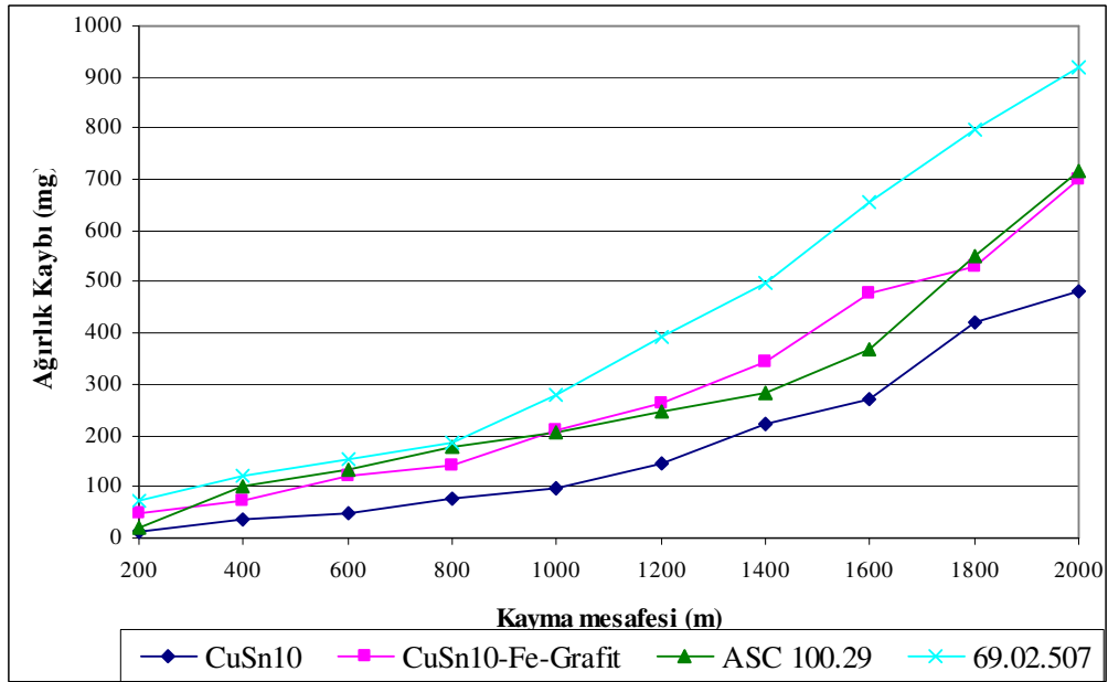
EK-A2. 0,22 m/sn ve 40N yük altında kayma mesafesi ağırlık kaybı değişimi
