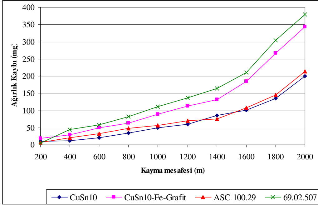
Şekil 10.13. 0,22 m/sn ve 10N yük altında kayma mesafesi ağırlık kaybı değişimi
