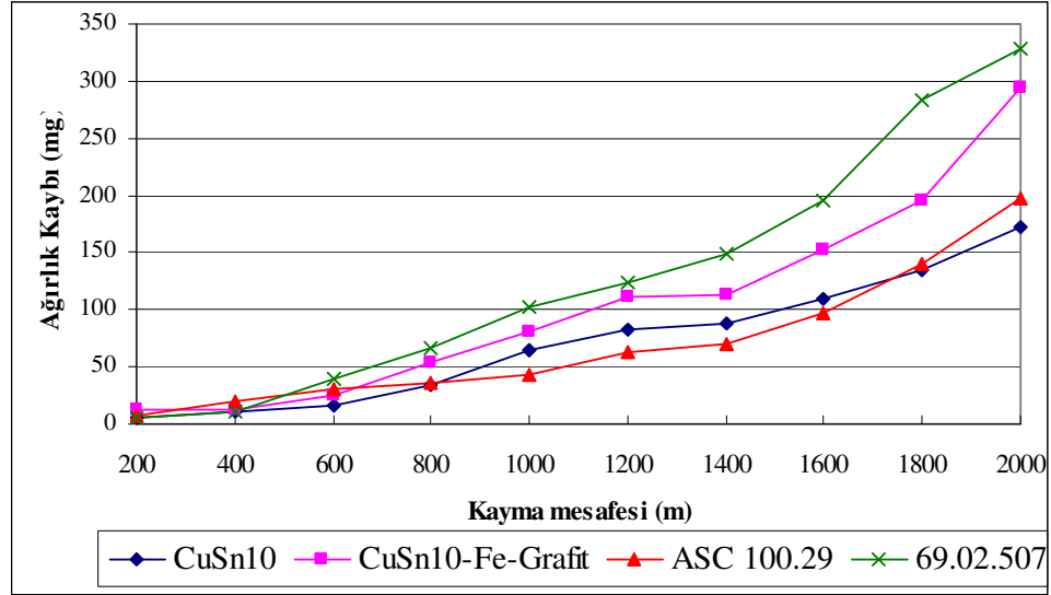
Şekil 10.17. 0,66 m/sn ve 10N yük altında kayma mesafesi ağırlık kaybı değişimi
