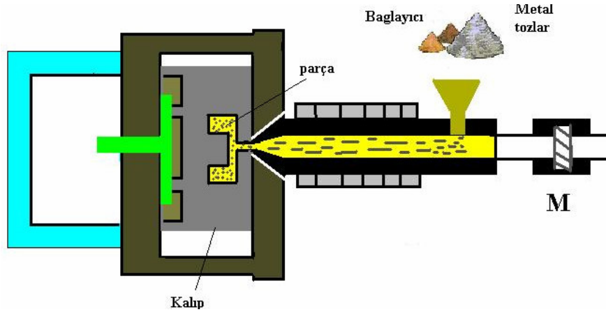
Şekil. 6.6. Enjeksiyonla kalıplama
