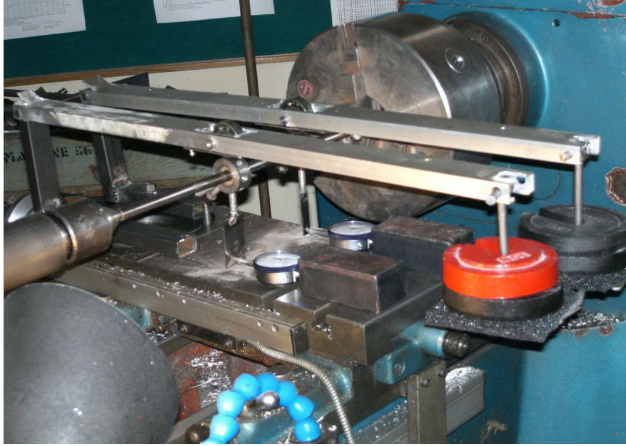
Şekil 9.2. Aşınma deneyinde kullanılan düzenek
