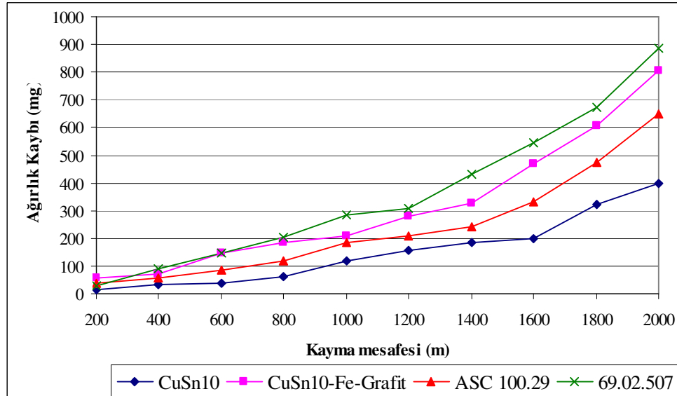
Şekil 10.18. 0,66 m/sn ve 30N yük altında kayma mesafesi ağırlık kaybı değişimi
