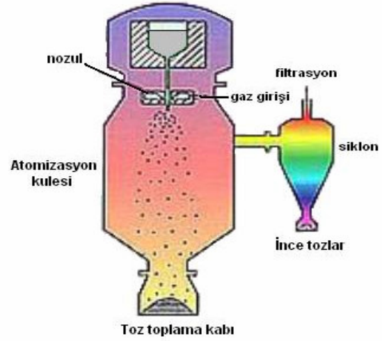
Şekil 5.3. Atomizasyon ünitesi ve kısımları
