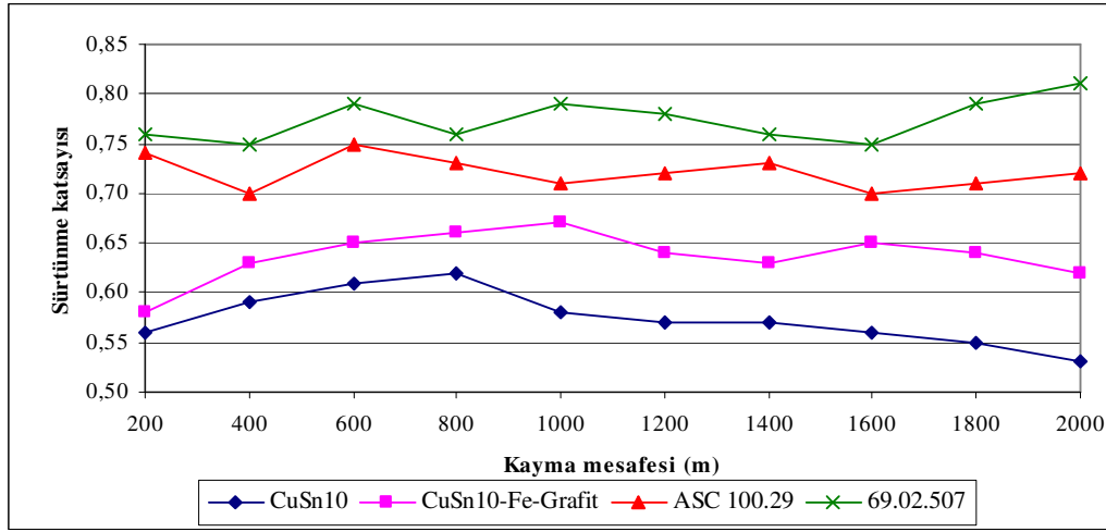
Şekil 10.27. 0,94 m/sn ve 10 N yük altında kayma mesafesi sürtünme katsayısı değişimi
