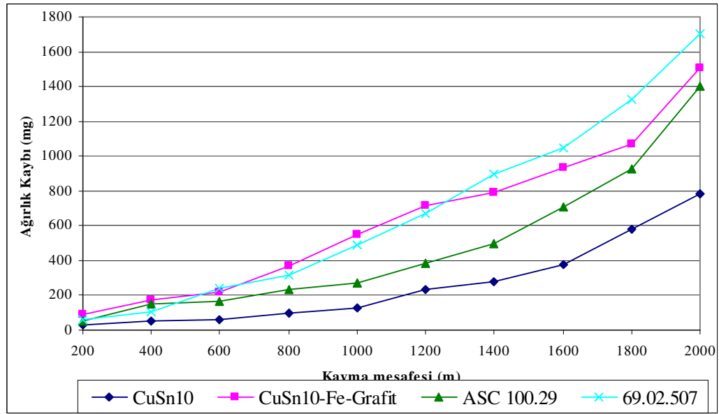
EK-A3. 0,22 m/sn ve 50N yük altında kayma mesafesi ağırlık kaybı değişimi
