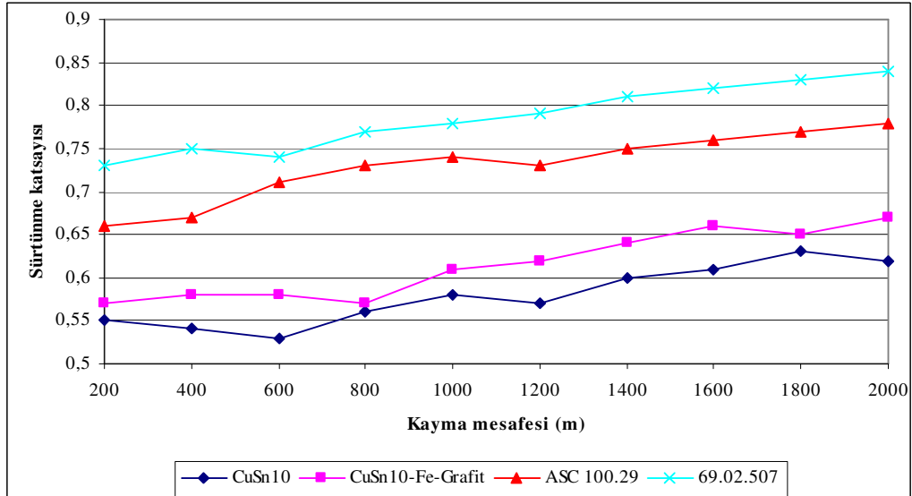
EK-E3. 0,22 m/sn ve 50 N yük altında kayma mesafesi sürtünme katsayısı değişimi.
