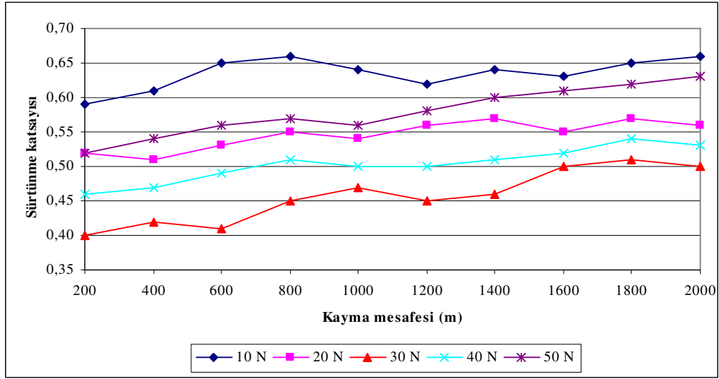
EK-İ1. CuSn10 yataklarına ait 0,66 m/sn’de yüke bağlı kayma mesafesi sürtünme katsayısı değişimi
