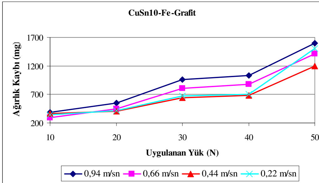
Şekil 10.5. CuSn10 yataklarına uygulanan yük ve ağırlık kaybının hıza göre değişimi
