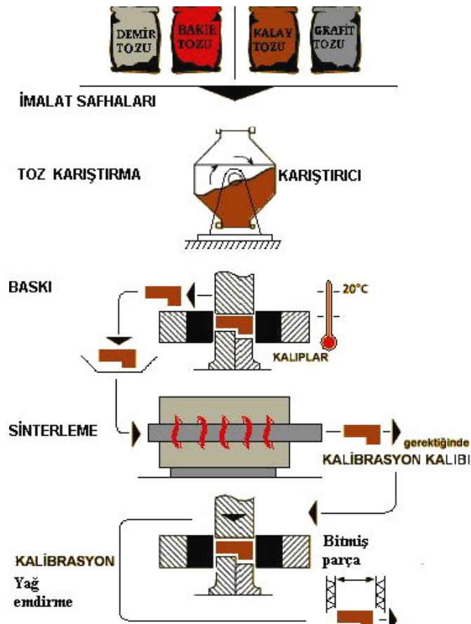
Şekil 6.12. Bakır-Demir alaşımlı T/M parça üretim basamakları (Karataş 1996)
