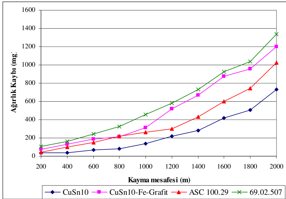
EK-B3. 0,44 m/sn ve 50N yük altında kayma mesafesi ağırlık kaybı değişimi
