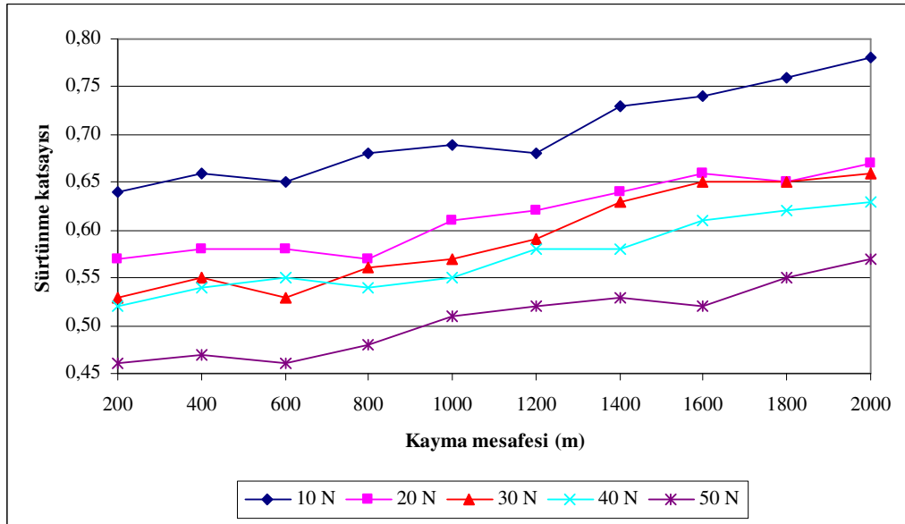
EK-I2. CuSn10-Fe-Grafit yataklarına ait 0,44 m/sn’de yüke bağlı kayma mesafesi sürtünme katsayısı değişimi
