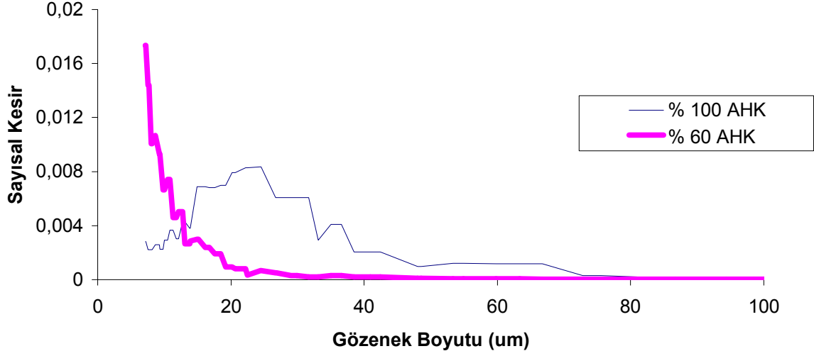
Şekil 6.42. Aynı koşullarda üretilmiş farklı miktarda yer tutucu ilave içeren köpüklerin gözenek boyutu ve dağılımı grafikleri.
