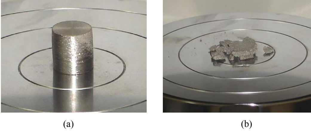
Şekil 6.33. Aynı miktarda (% 60) AHK içeren ve aynı sıcaklıkta (1200 °C) sinterlenen (a) ince, (b) kaba Ti tozundan üretilen köpüklerin basma testi sonundaki görüntüleri.
