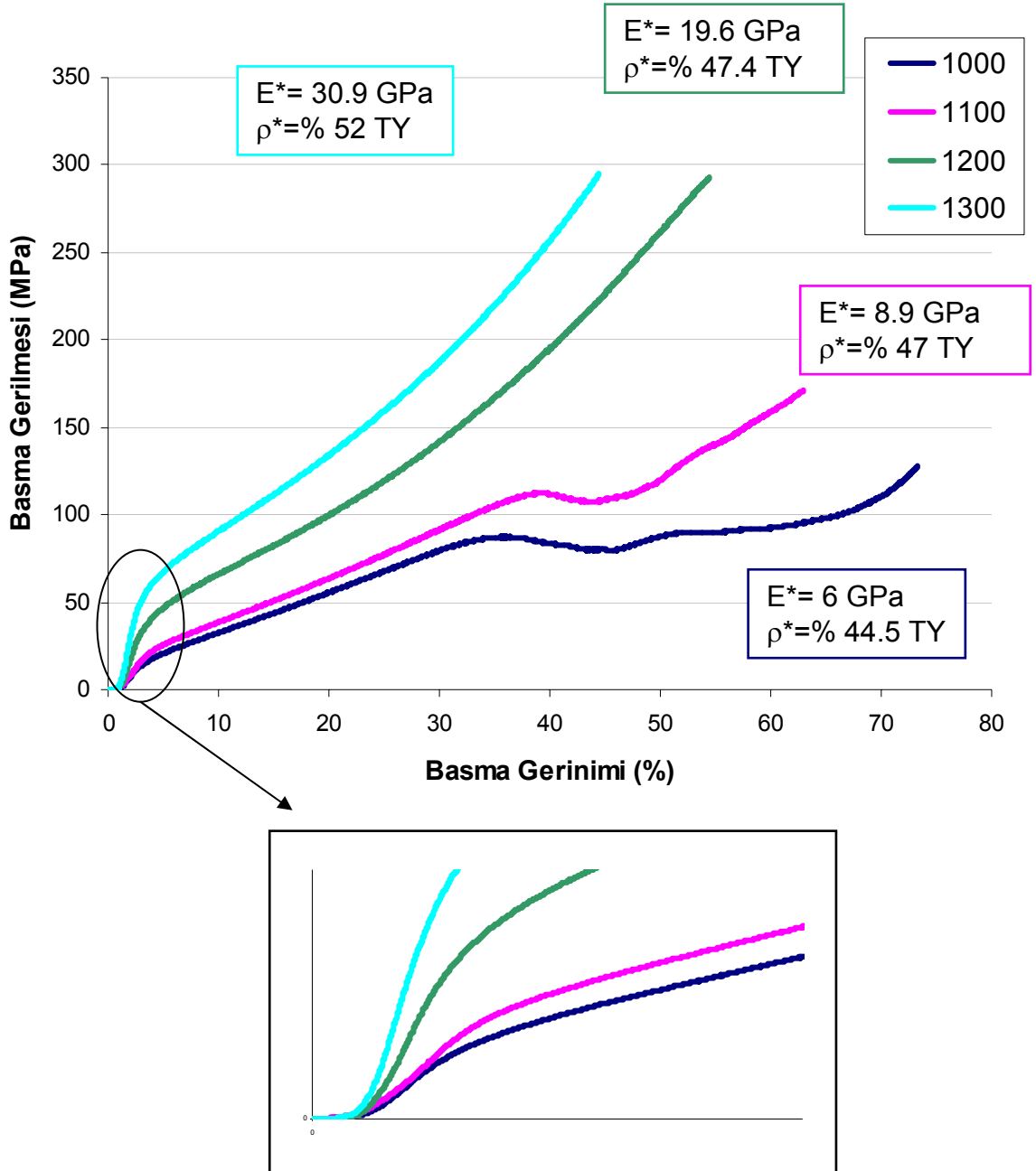
Şekil 6.38. Kaba Ti tozunun ağırlığına oranla % 40 AHK içeren ve farklı sıcaklıklarda sinterlenen köpüklerin gerilme-gerinim grafikleri.
