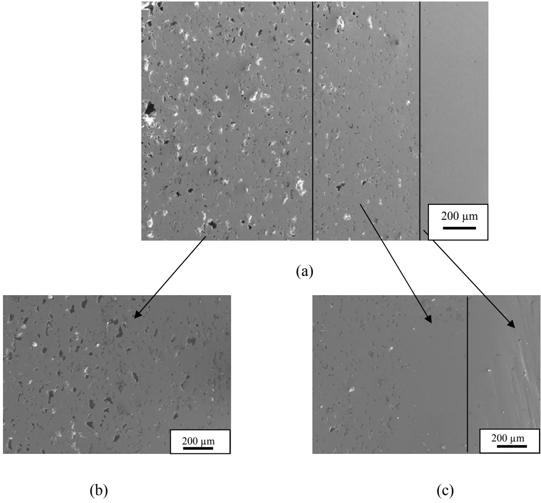
Şekil 6.49. Fonksiyonel aşamalı Ti köpük malzemenin SEM-SEI görüntüleri. (a) Köpük kesitinin 150 büyütme görüntüsü, (b) Ağırlıkça % 60 AHK içeren en gözenekli bölgenin 250 büyütme görüntüsü, (c) Ağırlıkça % 30 AHK içeren ve hiç yer tutucu malzeme içermeyen bölgelerin 250 büyütme görüntüsü.
