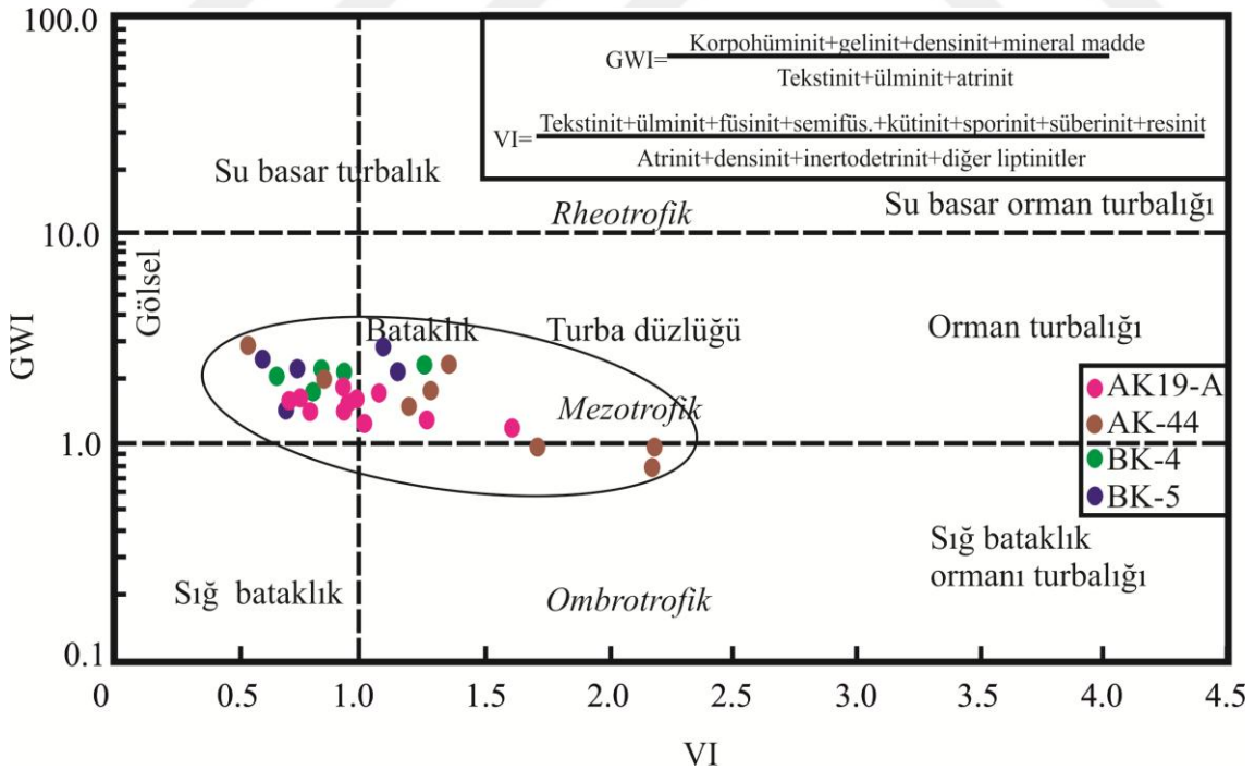
Şekil 5.45. Tez çalışması kapsamında AK19-A, AK-44, BK-4 ve BK-5 no'lu sondajlardan alınan kömür ve killi kömür örneklerinin VI-GWI diyagramları üzerindeki dağılımları (Kalaitzidis ve ark. 2004'den düzenlenerek alınmıştır).
