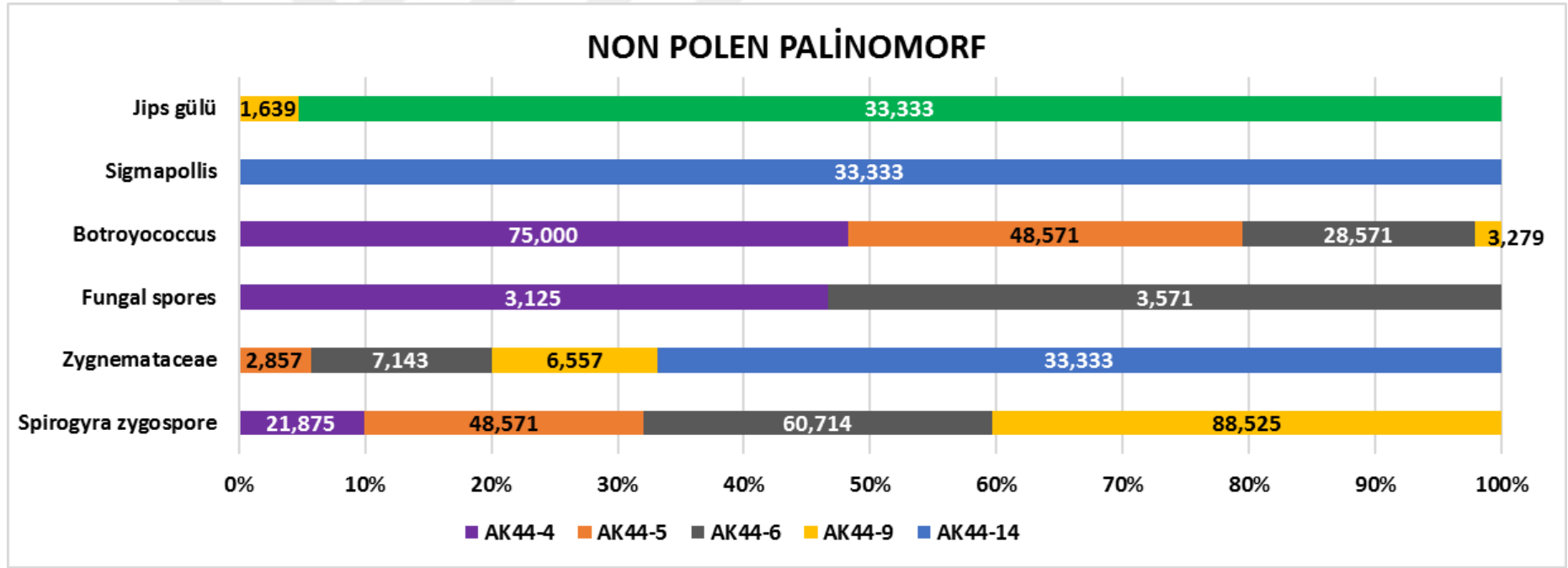
Şekil 5.53. AK 44 sondajından tanımlanmış non polen palinomorfların yüzde bolluklarını gösteren diyagram.
