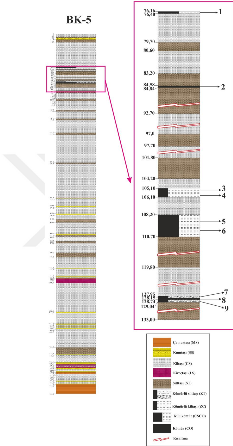
Şekil 4.4. BK-5 no'lu sondajdan alınan örneklerin sondaj logu üzerindeki konumları.
