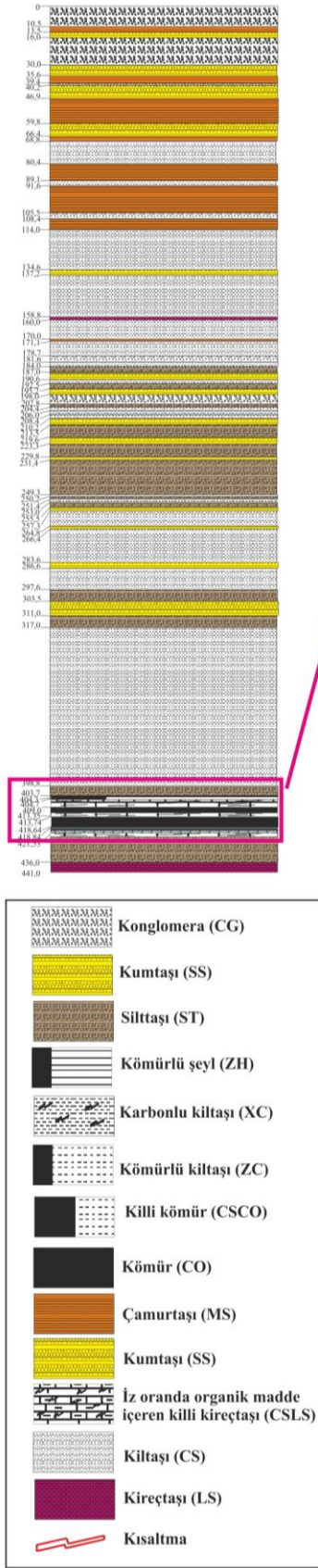
Şekil 4.2. AK-44 no'lu sondajdan alınan örneklerin sondaj logu üzerindeki konumları.
