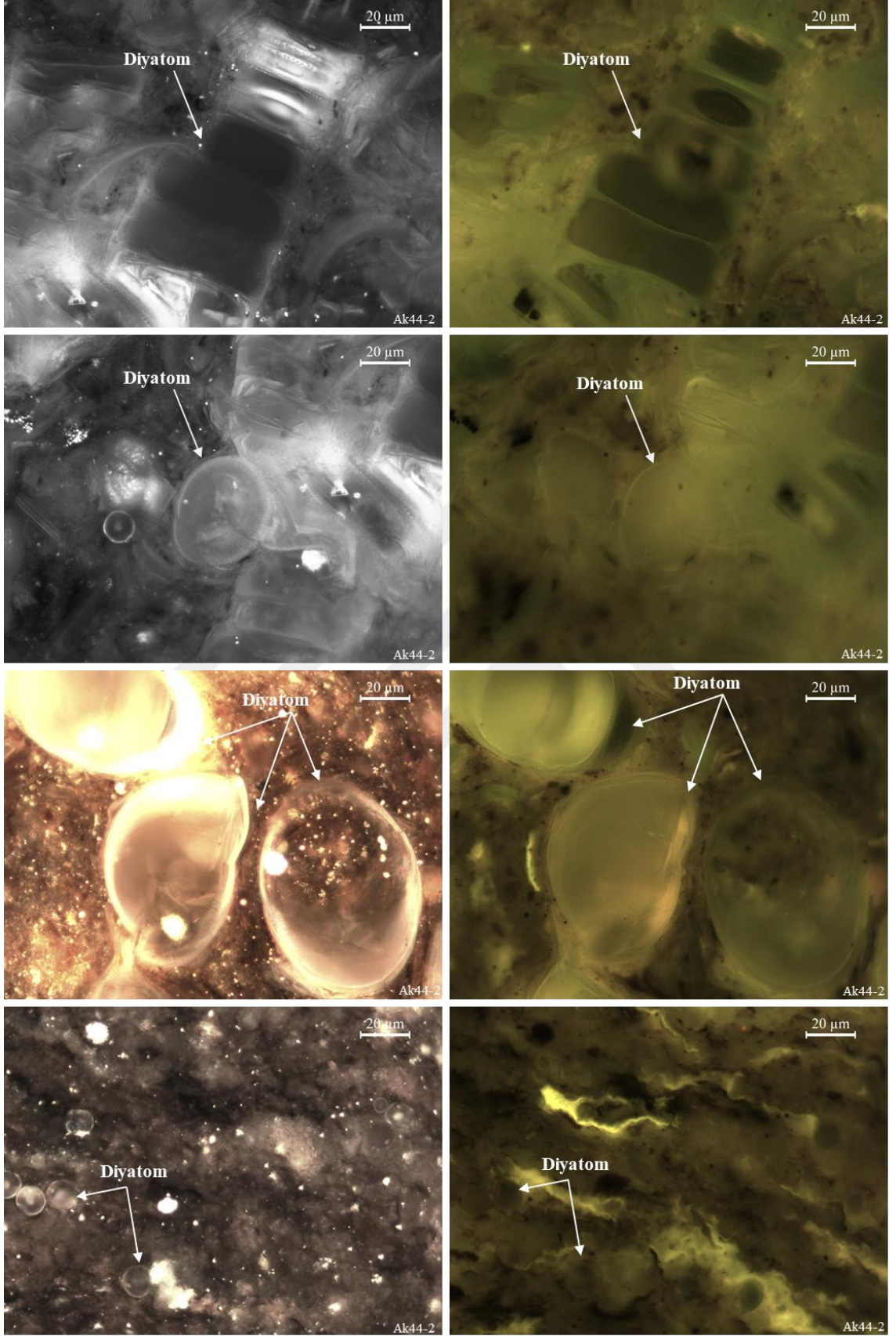
Şekil 5.40. Tez kapsamında incelenen AK44-2 no'lu örnekte üstten aydınlatmalı normal ışıktaki ve mavi ışık, turuncu filtrede diatom kavkı görüntüleri.
