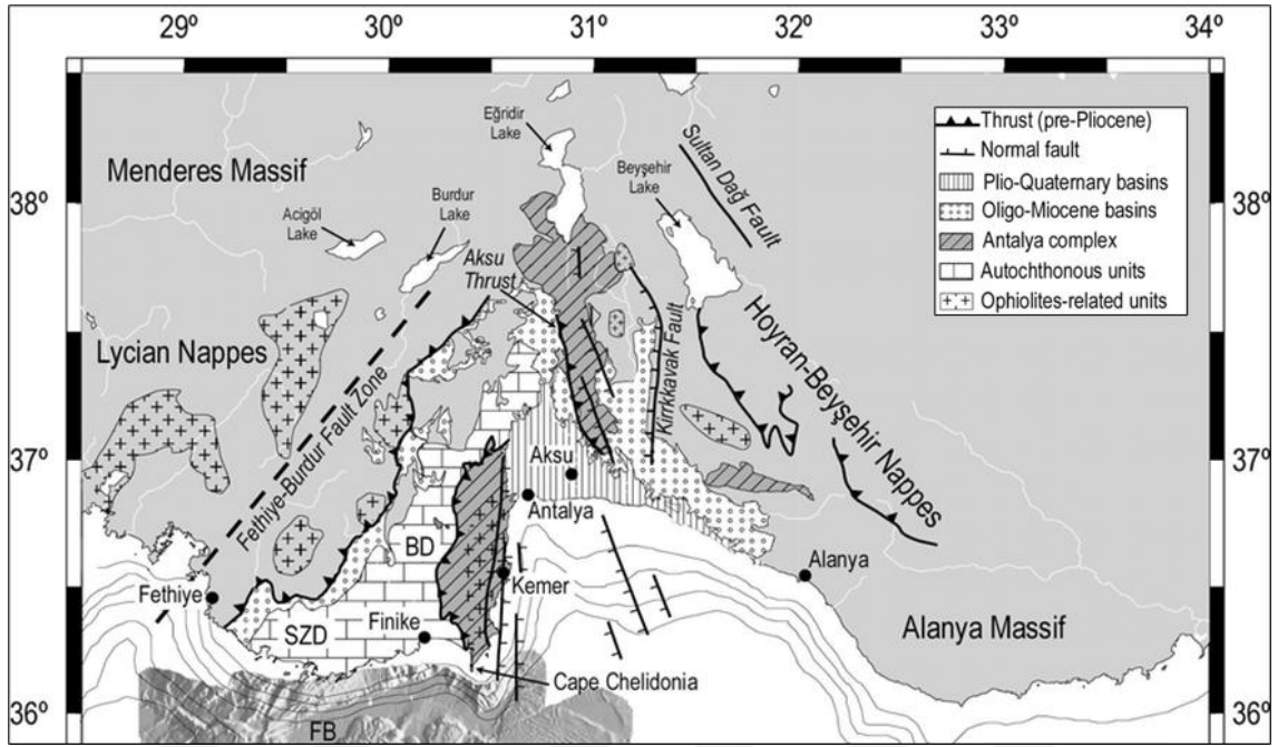
Şekil 1.9. Çalışma alanının Isparta açısı ve Fethiye-Burdur Fay zone içerisindeki konumu (Tiphaine, 2004).
