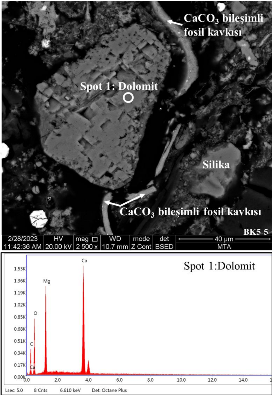
Şekil 5.23. Tez kapsamında BK5-5 nolu örneğin parlak kesiti üzerinde SEM-EDS yardımıyla tanımlanan fosil kavrısı, silika ve dolomit minerali ve SEM-EDS bileşimi.
