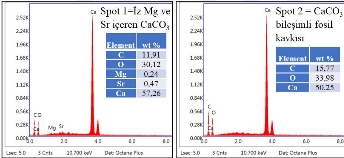
Şekil 5.22. Tez kapsamında BK4-1 nolu örneğin parlak kesiti üzerinde SEM-EDS yardımıyla tanımlanan \text{CaCO}_3 , iz oranda Mg ve Sr içeren \text{CaCO}_3 ve fosil kavkısı ve bunların SEM-EDS bileşimleri.
