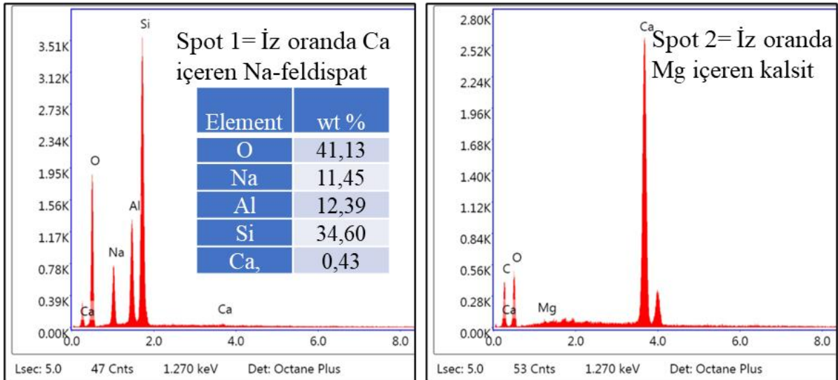
Şekil 5.26. Tez kapsamında BK4-2 nolu örneğin parlak kesiti üzerinde SEM-EDS yardımıyla tanımlanan iz oranda Mg içeren kalsit, iz oranda Ca içeren Na-feldispat, illit/miika mineralleri ve diyatom kavkısı.
