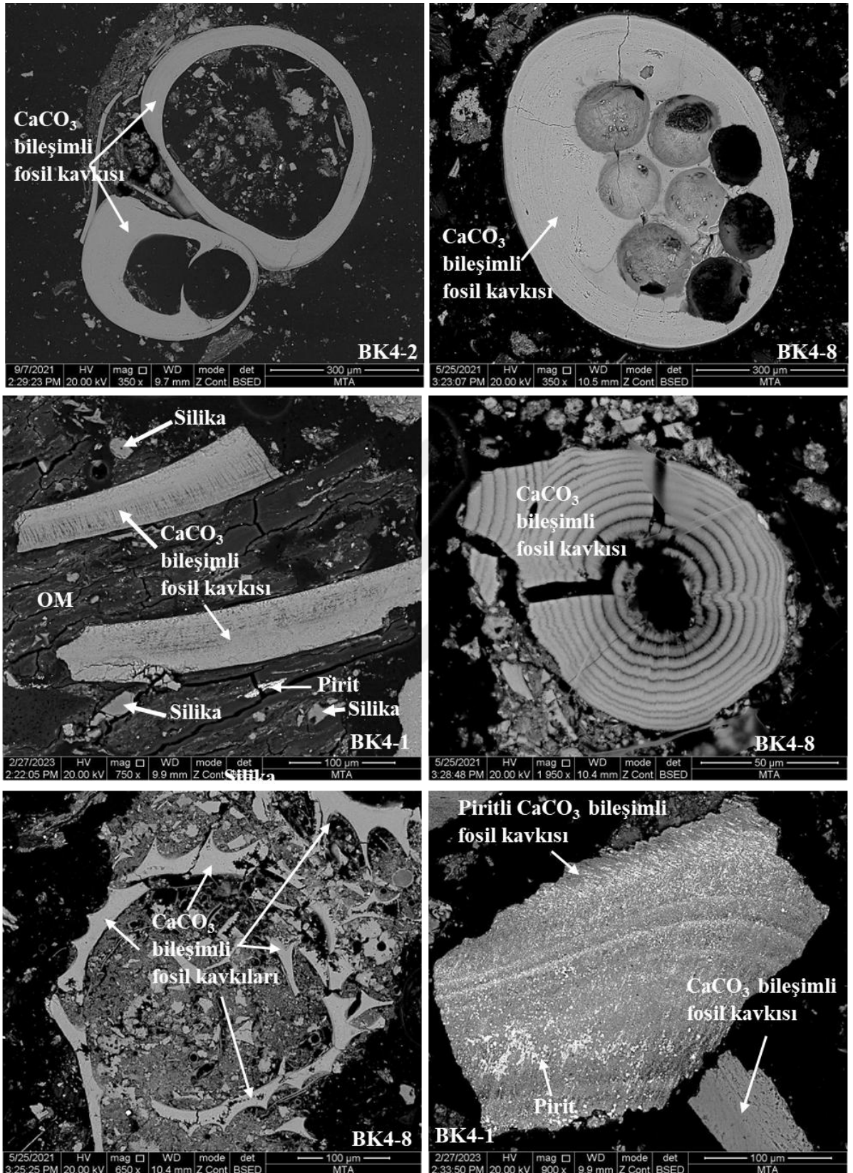
Şekil 5.35. Tez kapsamında incelenen örneklerin parlak kesitleri üzerinde SEM-EDS yardımıyla tanımlanan fosil kavkuları, pirit ve silika mineralleri.
