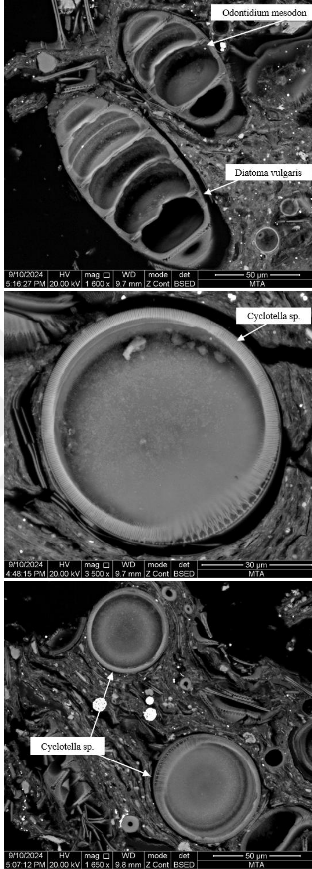
Şekil 5.61. AK44-2 no'lu kömürlü şeyl örneğinde tanımlanan diatomların ( Diatoma vulgaris ve Cyclotella sp. ) SEM görüntüleri.
