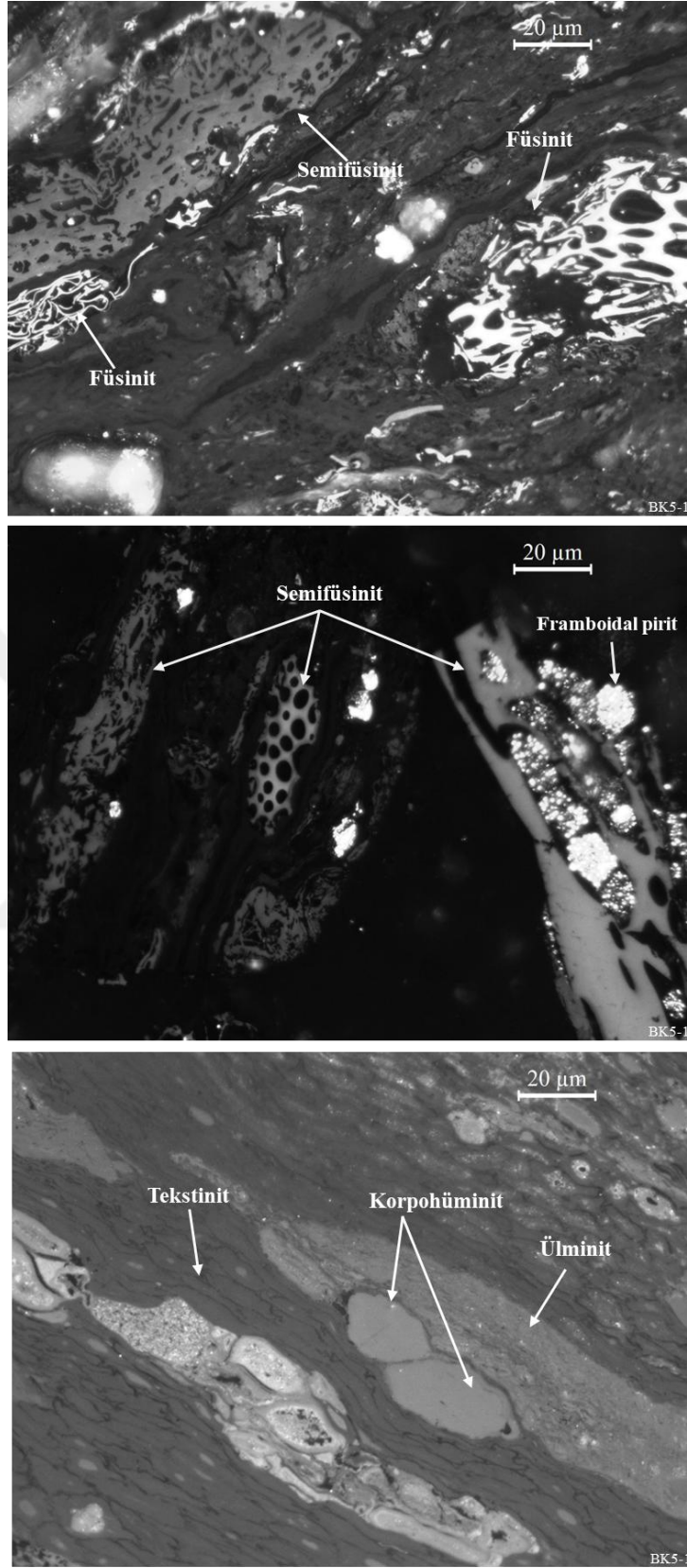
Şekil 5.39.Tez kapsamında incelenen BK5-1 no'lu örnekte tanımlanan füsinit, semifüsinit, korpohüminif, ülminif, tekstinit maseralleri ve framboidal pirit oluşumları.
