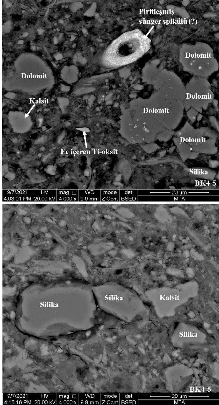
Şekil 5.27. Tez kapsamında BK4-5 nolu örneğin parlak kesiti üzerinde SEM-EDS yardımıyla tanımlanan dolomit, kalsit, silika, Fe-içeren Ti-oksit ve Piritleşmiş sünger spikülü (?) oluşumları.
