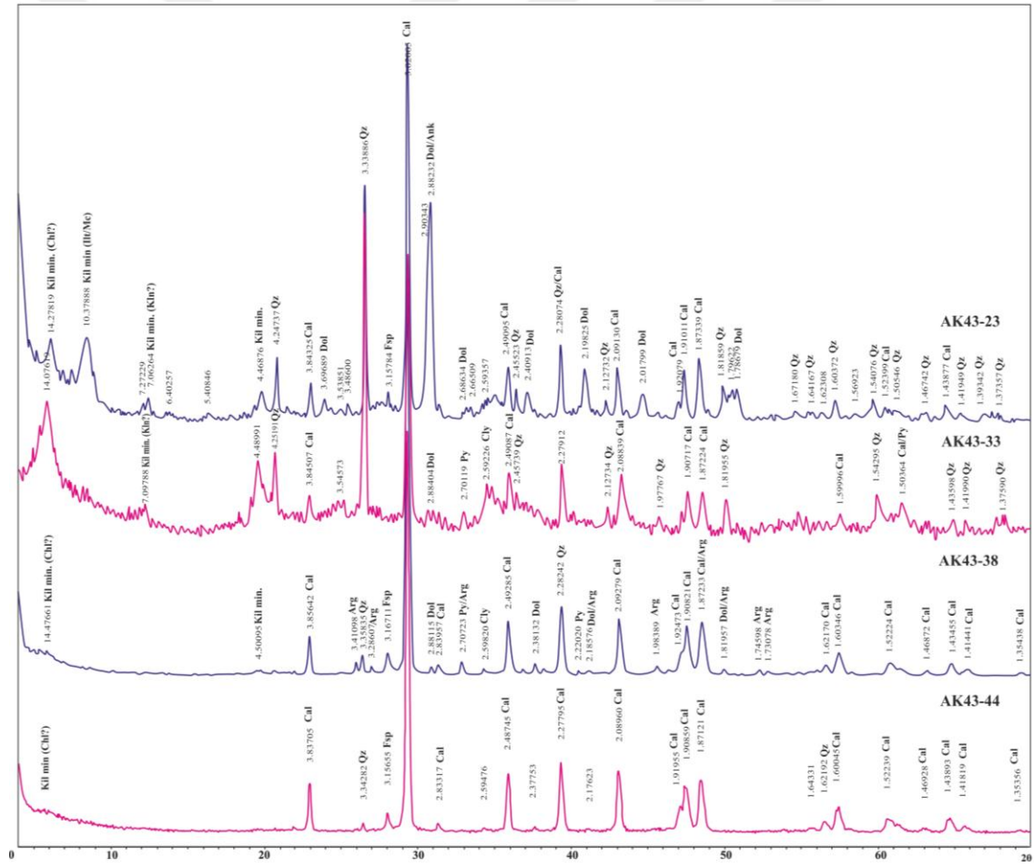
Şekil 5.8. Tez kapsamında AK-43 no'lu sondajdan seçilen temsili kayaç örneklerin XRD-TK diyagramlarında tanımlanan mineraller (Arg: aragonit, Ank: ankerit, Cly: kil minerali, Chl: klorit, Cal: kalsit, Dol: dolomit, Fsp: feldispat, Gp: jips, Illt/mc: illit/mika, Py: pirit, Qz: kuvars).
