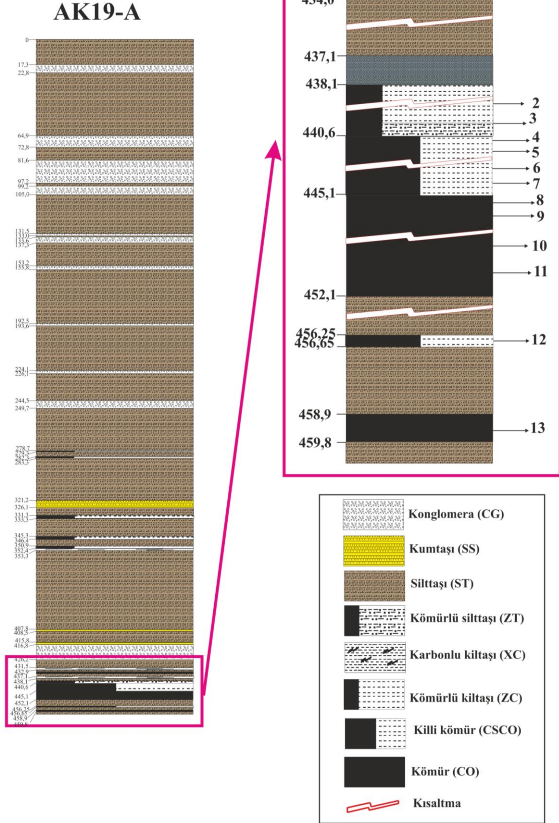
Şekil 4.1. AK-19A no'lu sondajdan alınan örneklerin sondaj logu üzerindeki konumları.
