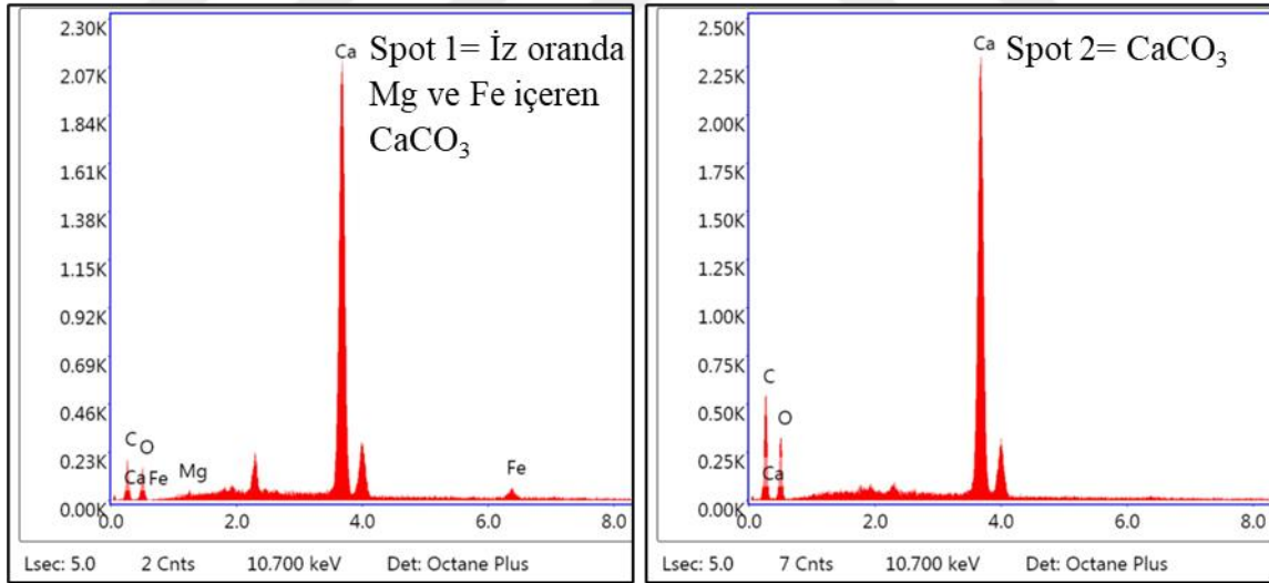
Şekil 5.15. Tez kapsamında BK4-1 nolu örneğin parlak kesiti üzerinde SEM-EDS yardımıyla tanımlanan pirit, \text{CaCO}_3 ve iz oranda Mg ve Fe içeren \text{CaCO}_3 ve SEM-EDS bileşimleri.
