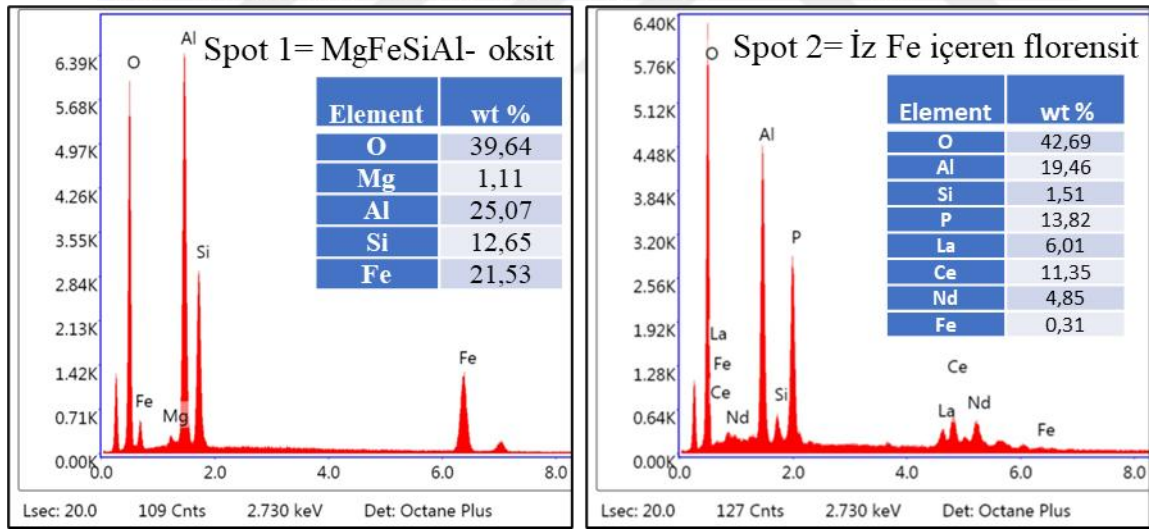
Şekil 5.24. Tez kapsamında BK4-2 nolu örneğin parlak kesiti üzerinde SEM-EDS yardımıyla tanımlanan mineraller ve SEM-EDS bileşimleri.
