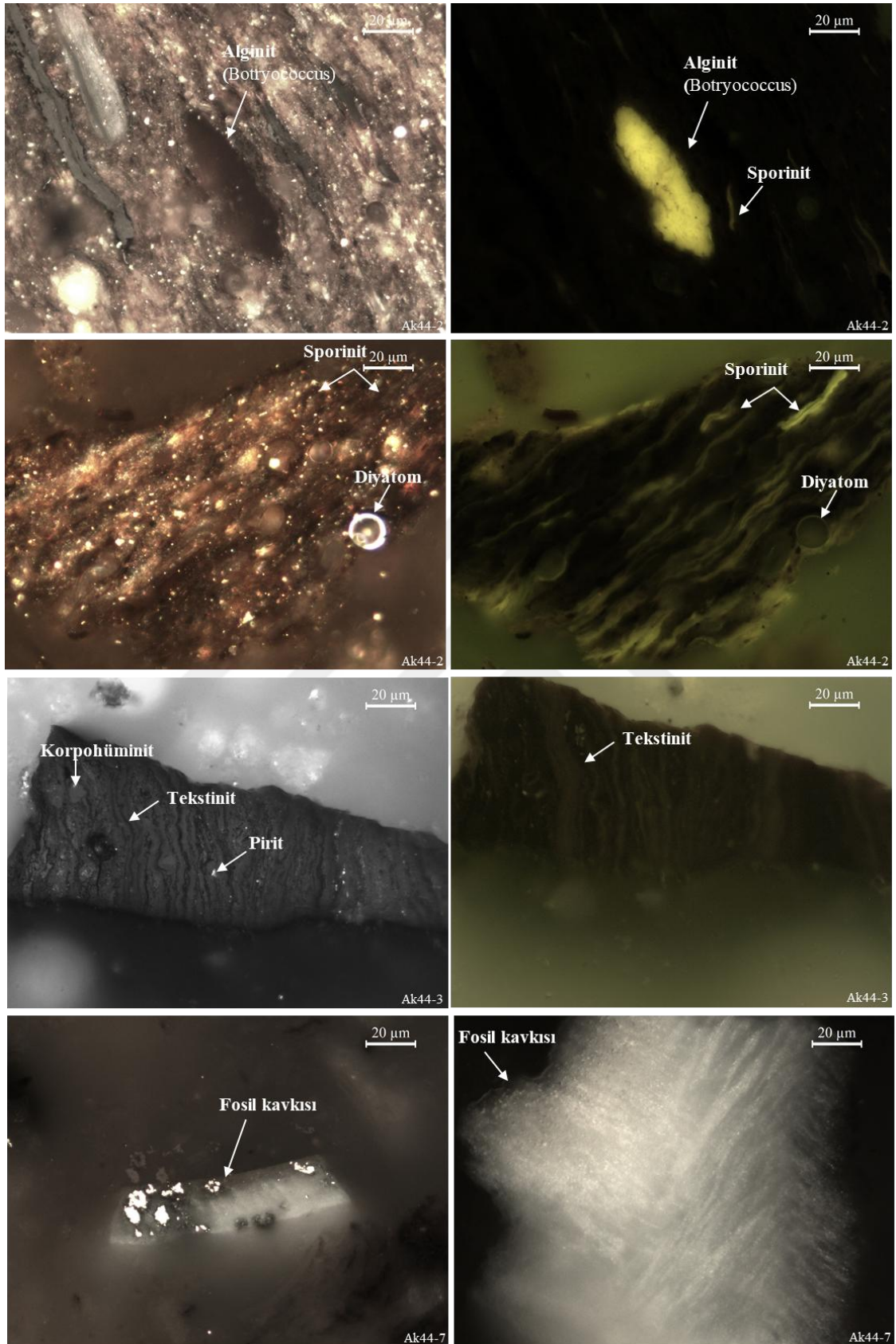
Şekil 5.38. Tez kapsamında incelenen örneklerde tanımlanan maserallerin üstten aydınlatmalı normal ışıktaki ve mavi ışık, turuncu filtrede görünüşleri.
