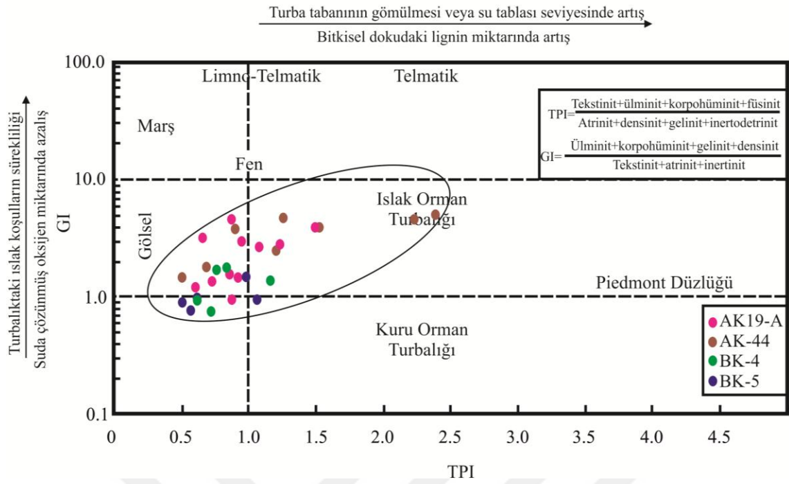
Şekil 5.44. Tez çalışması kapsamında AK19-A, AK-44, BK-4 ve BK-5 no'lu sondajlardan alınan kömür ve killi kömür örneklerinin TPI-GI diyagramları üzerindeki dağılımları (Kalaitzidis ve ark. 2004'den düzenlenerek alınmıştır).
