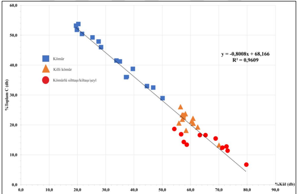
Şekil 5.5. Tez kapsamında incelenen örneklerin kuru bazda (db) %kül içeriği ile %toplam karbon değerlerinin karşılaştırılması.
