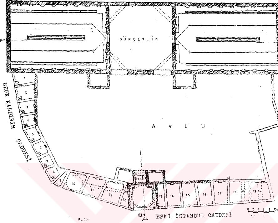
ÇİZİM.V.IV.3.1-GENEL PLAN ŞEMASI.
