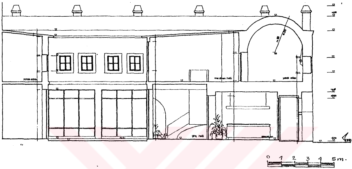
ÇİZİM.V.VI.4.3- A-A KESİTİ , (T.Ü.RÖLÖVE ARŞİVİ.).
