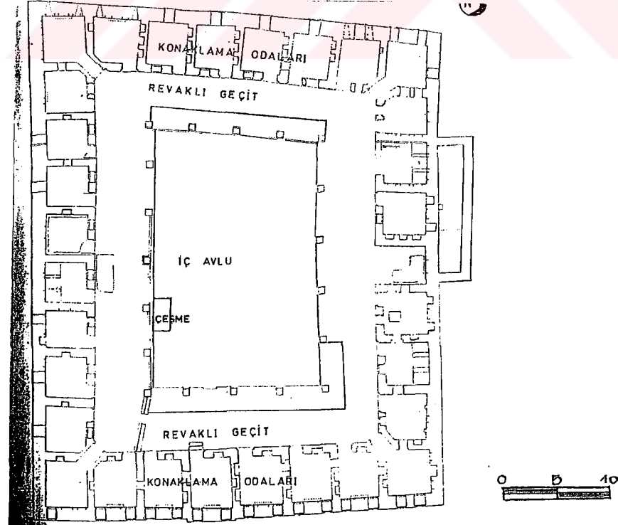
ÇİZİM.V.II.BİRİNCİ KAT PLANI (KILIÇÖTE,C, DEVECİ HAN RESTORASYON SÜRECİ, O.D.T.Ü. TEZ, 1990.).
