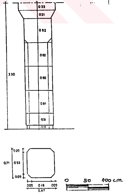
ÇİZİM.V.II.6.11-REVAKLI GALERİYE AİT ,GÖRÜNÜŞ VE KESİT.
