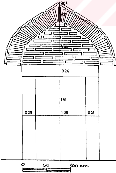
ÇİZİM.V.II.7.16-DOĞU CEPHESİ, GİRİŞ KAPISI.
