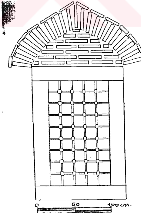
ÇİZİM.V.II.7.15-KONAKLAMA ODASI,BASIK SİVRİ KEMERLİ PENCERE.
