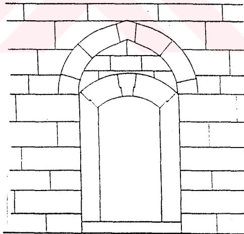
EXMEKÇIOĞLU AHMET PAŞA KERVANSARAYI GİRİŞ MEKANI AVLU YÖNÜNDEKİ HÜCRELERE AİT KAPI DETAYI SEKİL NO: 16
