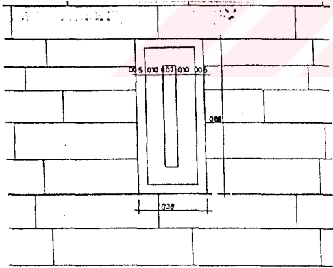
ÇİZİM.V.IV.7.12-ŞEBEKELİ PENCERE.
