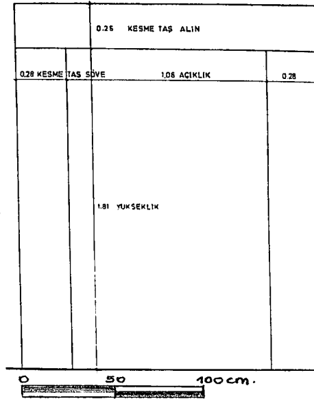
ÇİZİM.V.II.7.19-KONAKLAMA ODASI, KAPISI.
