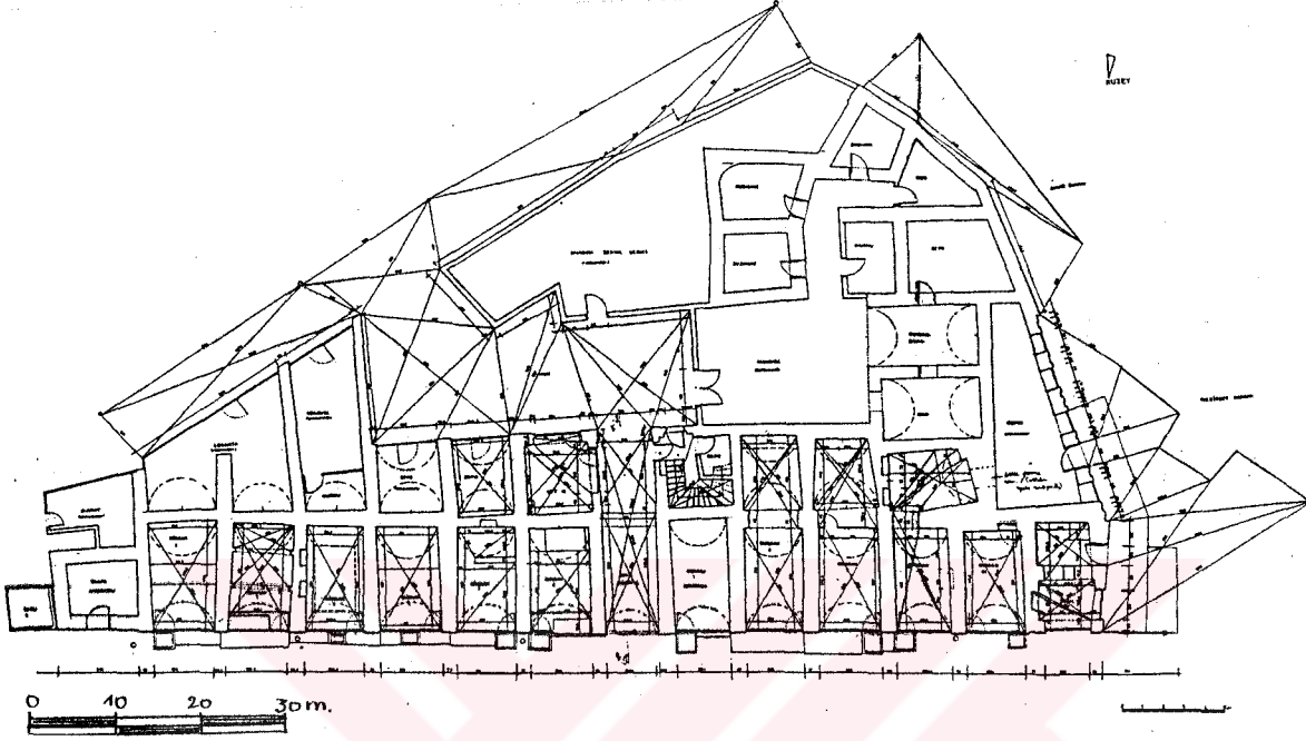
ÇİZİM.V.V.3.1- ZEMİN KAT PLANI, (T.Ü.RÖLÖVE ARŞİVİ.).
