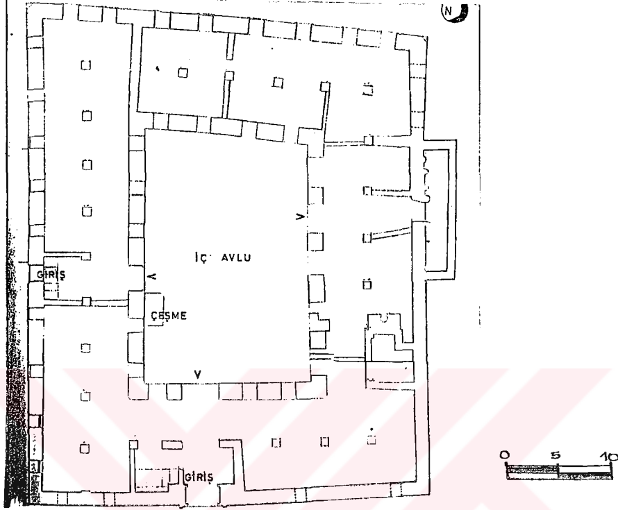
ÇİZİM.V.II.3.1-ZEMİN KAT PLANI (KILIÇÖTE,C, DEVECİ HAN RESTORASYON SÜRECİ, O.D.T.Ü. TEZ, 1990.).
