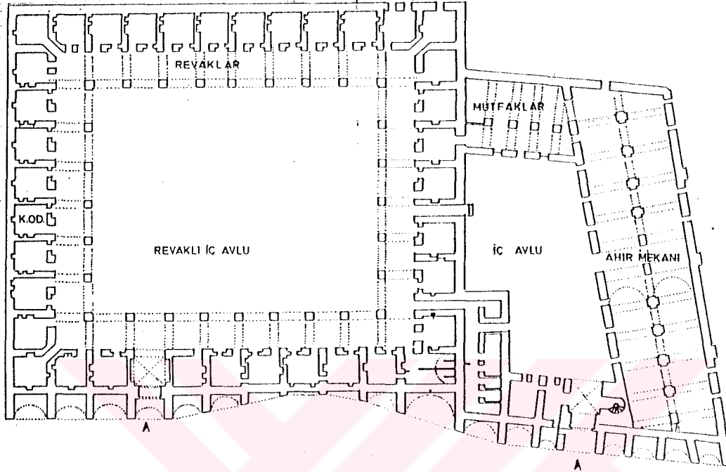
ÇİZİM.V.III.3.1-ZEMİN KAT PLANI , ( T.Ü. RÖLÖVE ARŞİVİ ).
