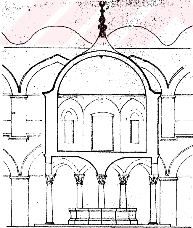
ÇİZİM.V.III.21-ŞADIRVANLI KÖŞK MESCİD, RESTİTÜSYON KESİTİ, (E.T.K.V.K.K. DOSYASINDAN.).
