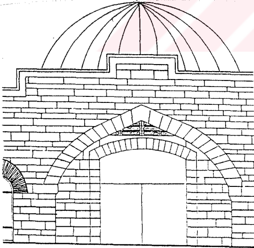
ÇİZİM.V.IV.7.16-KONAKLAMA MEKANI GİRİŞ KAPISI.
