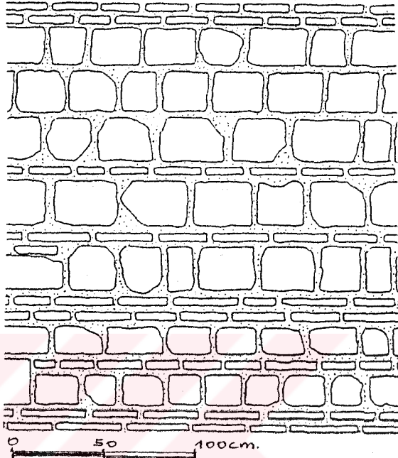
ÇİZİM.V.V.6.10-GİRİŞ GEÇİTİNE AIT ,DUVAR DETAYI.
