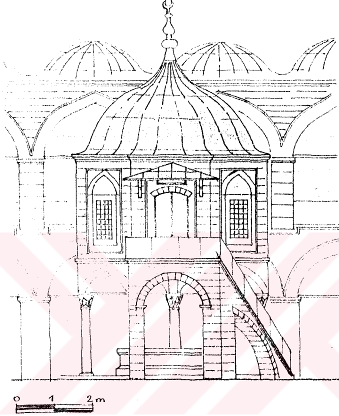
ÇİZİM.V.III.11.22-ŞADIRVANLI KÖŞK MESCİDİN RESTİTÜSYON, GÖRÜNÜŞÜ (E.T.K.V.K.K. DOSYASINDAN.).
