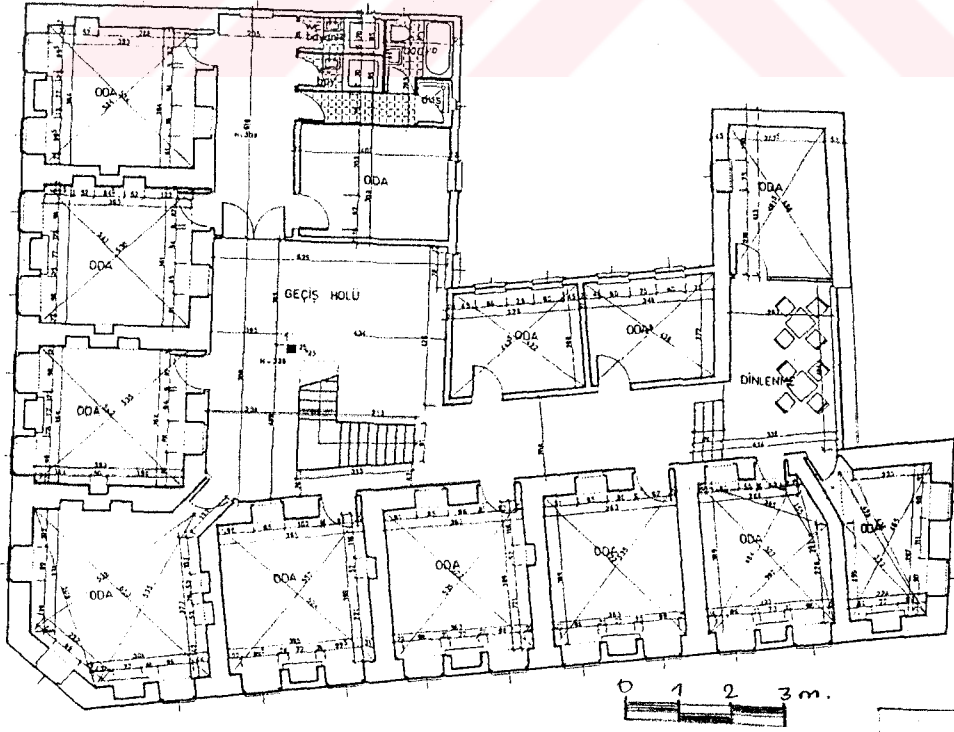
ÇİZİM.V.VI.3.2-BİRİNCİ KAT PLANI , (T.Ü.RÖLÖVE ARŞİVİ.).
