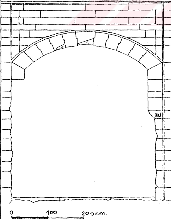
V.V.7.11-GİRİŞ KAPISI RÖLEVESİ.
