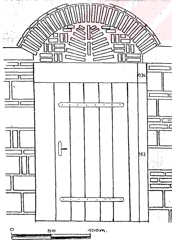
ÇİZİM.V.III.7.14-KONAKLAMA ODASI KAPISI.
