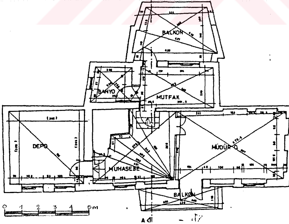
ÇİZİM.V.V.3.2-I.KAT PLANI, (T.Ü.RÖLÖVE ARŞİVİ.).
