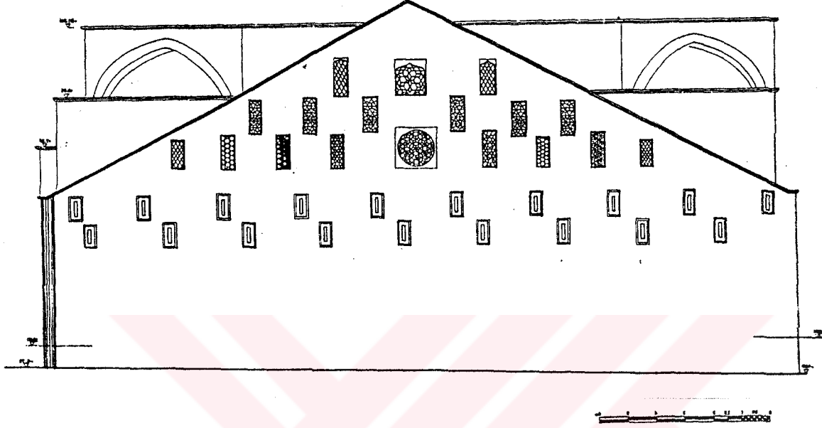
ÇİZİM.V.IV.6.7-BATI (YAN) CEPHESİ , (T.Ü.RÖLÖVE ARŞİVİ.).
