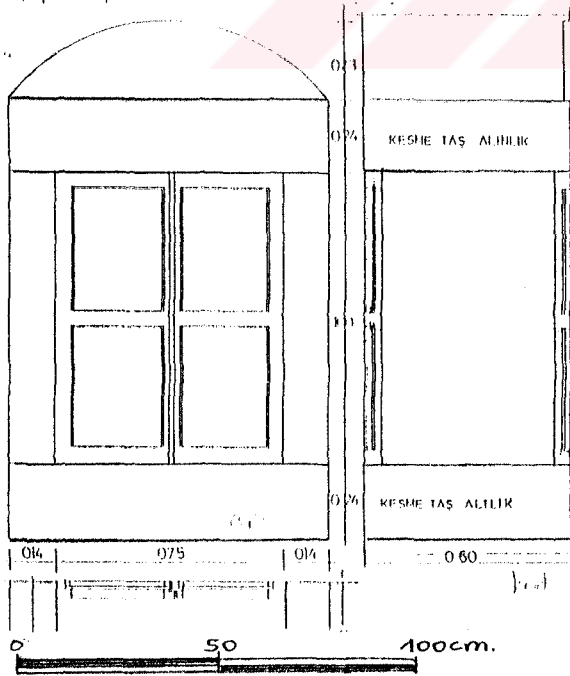
ÇİZİM.V.VI.7.9-KONAKLAMA ODASI, KORİDORA BAKAN PENCERE,GÖRÜNÜŞ VE KESİTİ.
