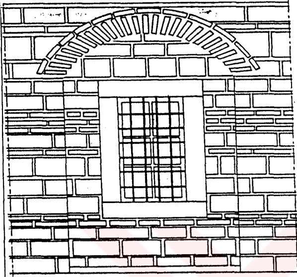
ÇİZİM.V.III.7.8-REVAKLI GEÇİT,ÇÖKERTME DUVAR GÖRÜNÜŞÜ
