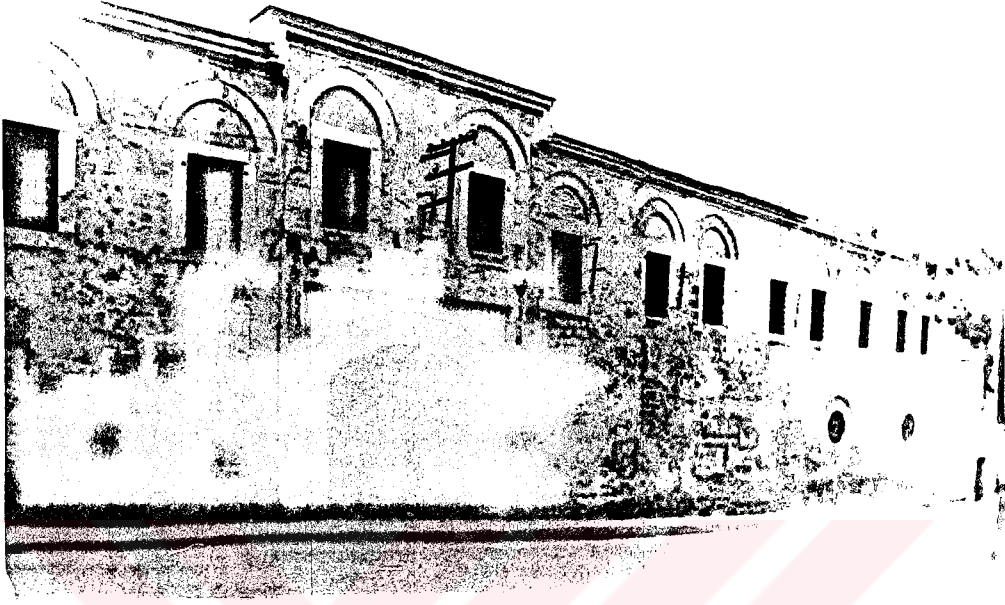
RESİM.V.II.9.23-CEPHEDE, DERZ BOŞALMALARI, TAŞ DÜŞMELERİ (E.T.K.V.K.K.)
