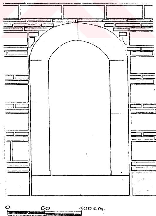
ÇİZİM.V.III.7.15-W.C. KAPISI.
