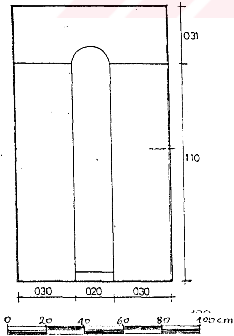
ÇİZİM.V.III.7.10-MAZGAL PENCERE.
