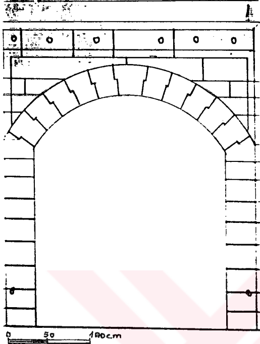
ÇİZİM.V.II.7.16-DOĞU CEPHESİ, GİRİŞ KAPISI.
