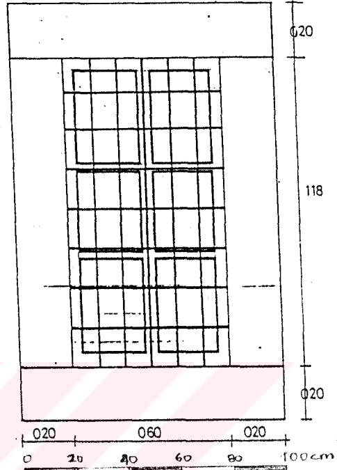
ÇİZİM.V.III.7.9-KONAKLAMA ODASI PENCERESİ.
