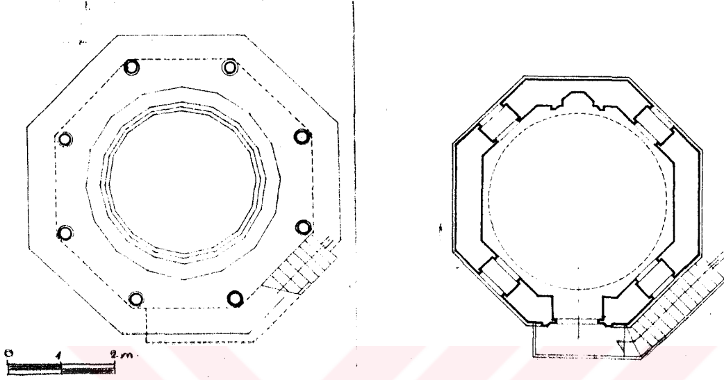
ÇİZİM.V.III.11.20-ŞADIRVANLI KÖŞK MESCİDİN RESTİTÜSYON,ZEMİN VE BİRİNCİ KAT PLANI (E.T.K.V.K.K. DOSYASINDAN.).
