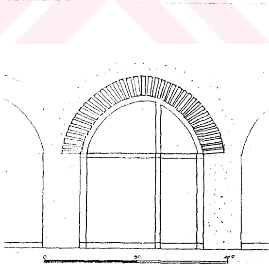
ÇİZİM.V.V.6.10-GİRİŞ GEÇİTİNE AIT ,DUVAR DETAYI.
