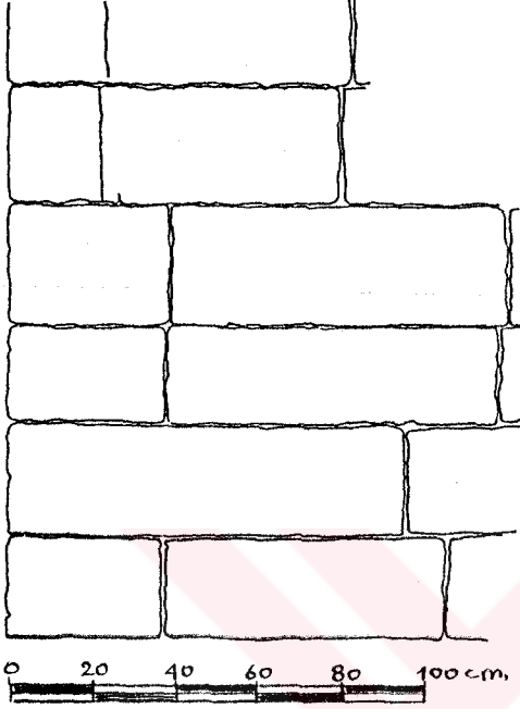
ÇİZİM.V.V.6.9-GİRİŞ GEÇİTİNE AIT DUVAR ÖRGÜ DETAYI.
