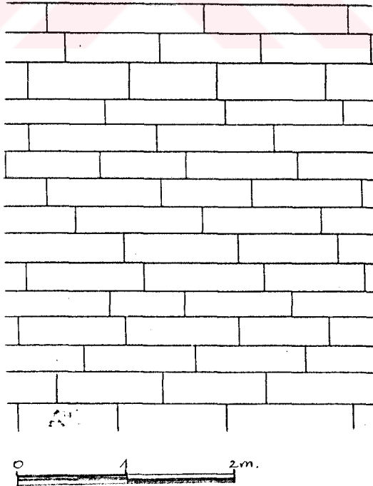
ÇİZİM.V.IV.6.11-DOĞU CEPHESİ,DUVAR ÖRGÜSÜ..
