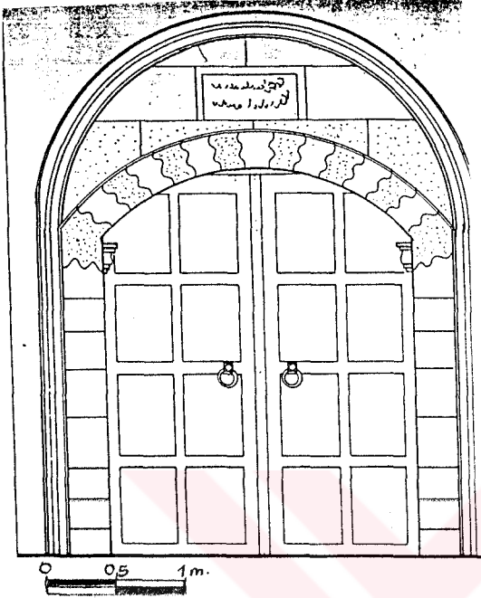
ÇİZİM.V.III.7.12-BÜYÜK AVLU GİRİŞ KAPISI.
