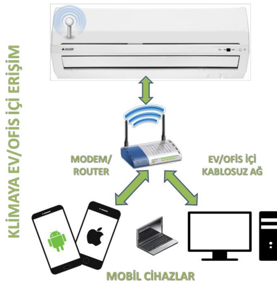
Şekil 3.1 Klimaya ev/ofis içerisinde bulunan kablosuz yerel ağ üzerinden erişim
