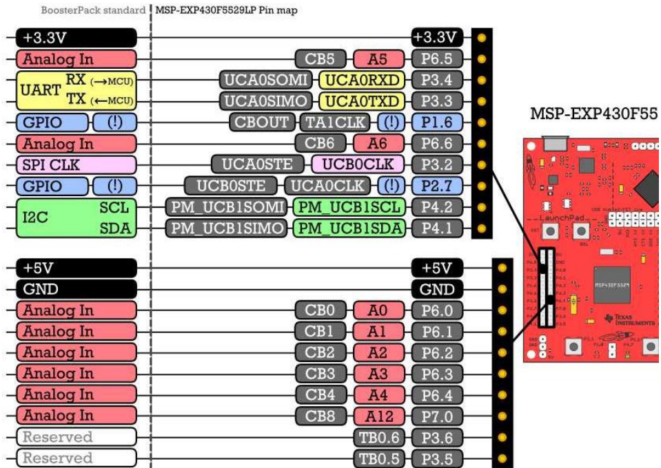
Şekil 2.4 MSP430F5529 LP pin şematığı 1 [35]
