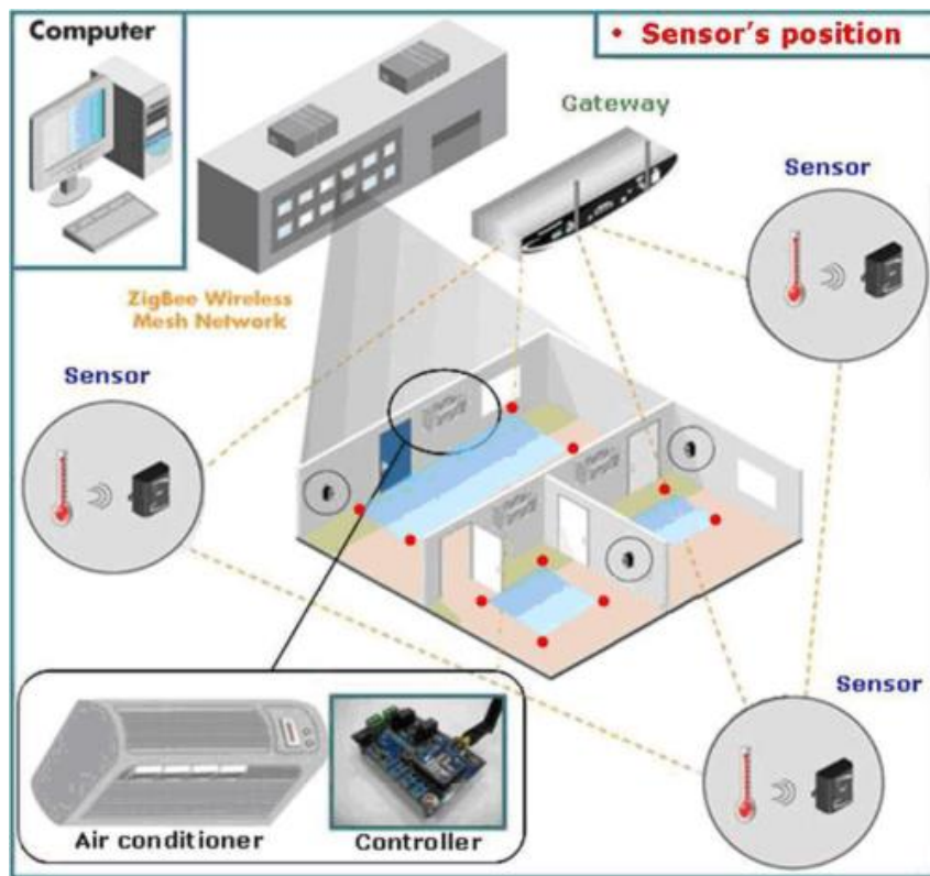
Şekil 1.11 Kablosuz sensör ağı sistemi [12]
