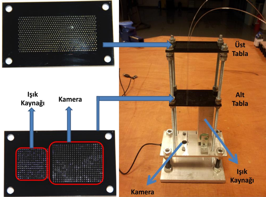
Şekil 7.4 Algılayıcı elek yapısı, kamera ve ışık kaynağı
