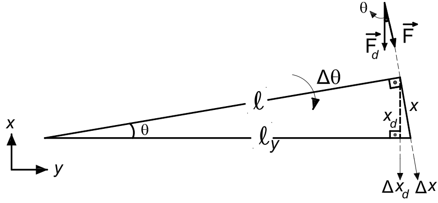
Şekil 9.7 Sabit kuvvet uygulanabilen ve yer değiştirmenin ölçüldüğü deney düzeneğinin serbest cisim diyagramı
