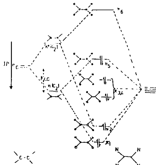
Şekil 1.1. E.z.o.larda \pi -Moleküler orbital enerji diyagramı
