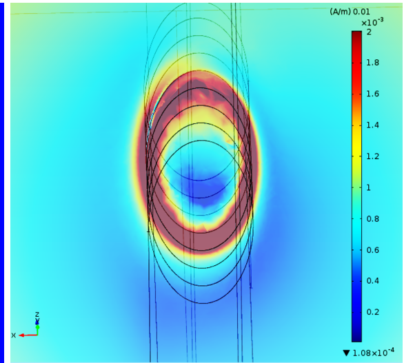
(d) Tilted coil on tilting plane
