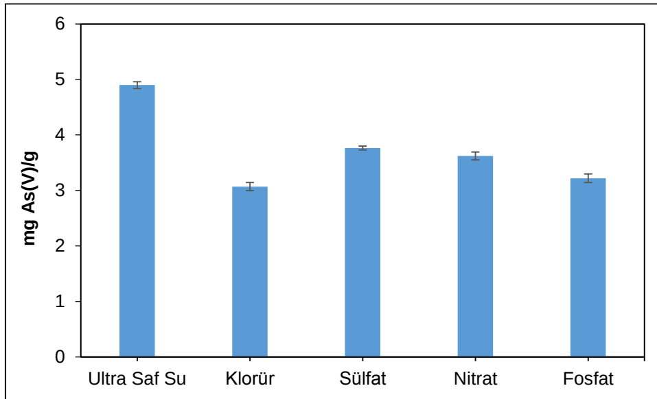
Şekil 4.14. 4-AMP-PS partiküllerinin As(V) adsorpsiyonuna anyon etkisi. (Deneysel koşullar: 10 mg 4-AMP-PS, Çözelti hacmi: 20 mL, As(V) iyonları derişimi: 10 ppm ve \text{Cl}^- , \text{PO}_4^{3-} , \text{NO}_3^- , \text{SO}_4^{2-} iyonları derişimi: 100 ppm, pH:6.00)
