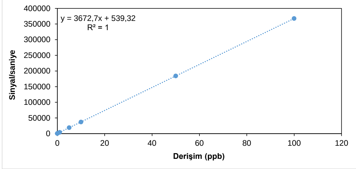
Şekil 3.1. As analizlerinde kullanılan kalibrasyon grafiği.
