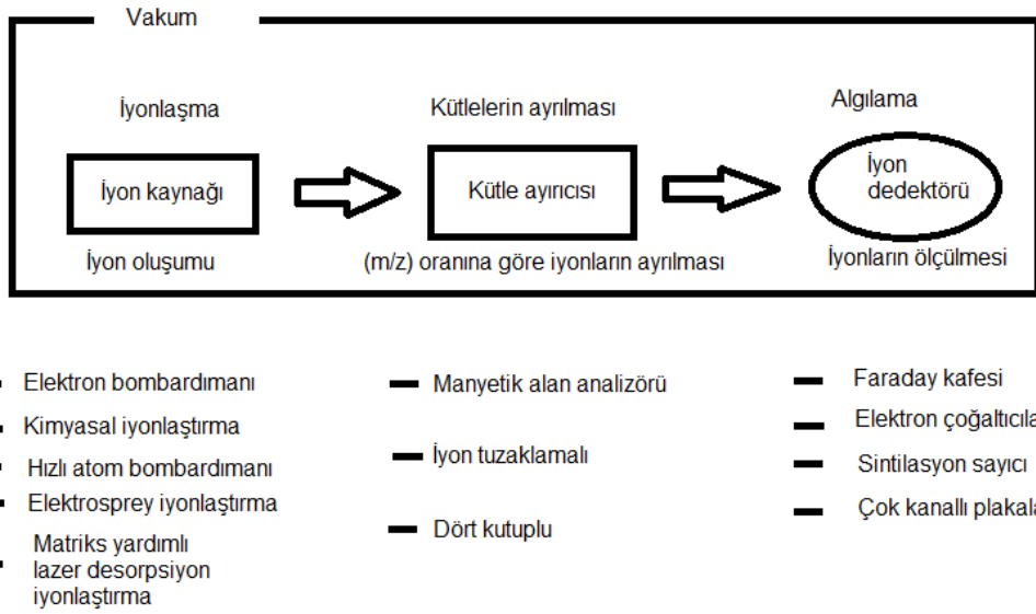
Şekil 2.10. Kütle spektrometresinin şematik gösterimi.
