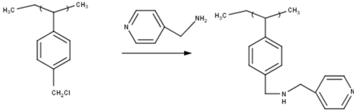
Şekil 3.2. 4-AMP-PS partiküllerin hazırlanmasının şematik gösterimi.
