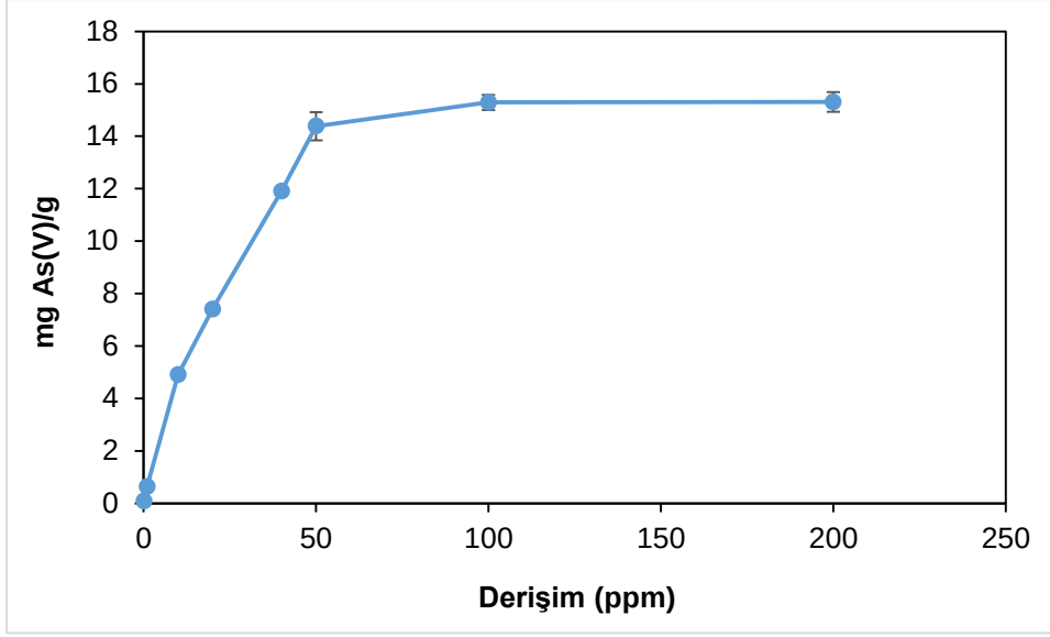
Şekil 4.12. 4-AMP-PS partiküllerinin As(V) adsorpsiyona başlangıç derişiminin etkisi. (Deneyisel Koşullar: 10 mg 4-AMP-PS, çözelti hacmi: 20 mL, pH: 6.00, karıştırma hızı:100 rpm, adsorpsiyon süresi: 16 saat)
