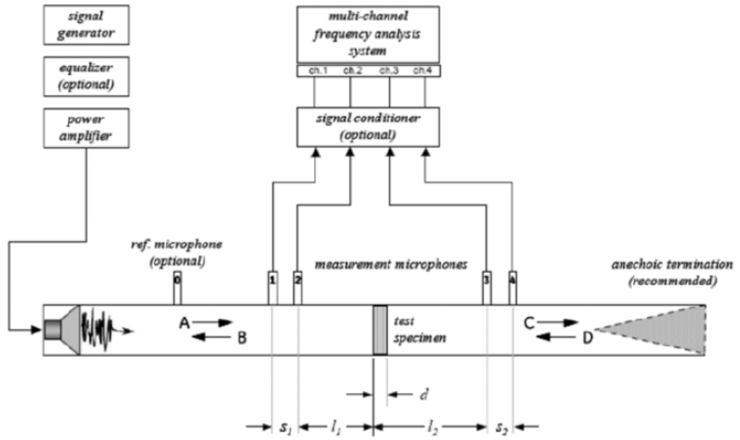
Şekil 4.1 : Ses ölçüm düzeneği şeması.
