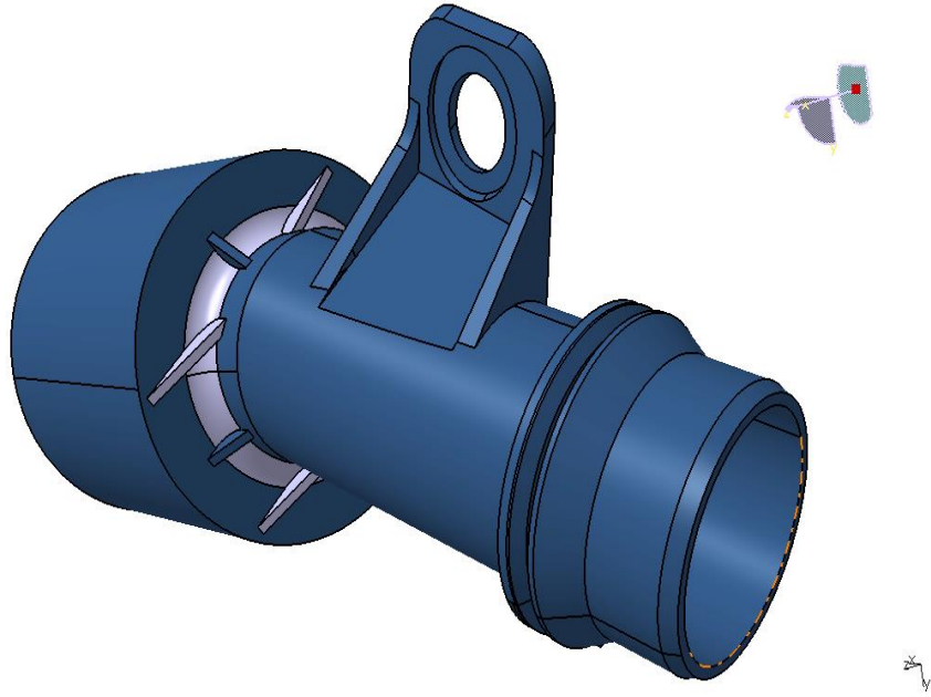
Şekil 1.6 : Feder sayısı ve Radius genişliği artırılmış üçüncü tasarım.
