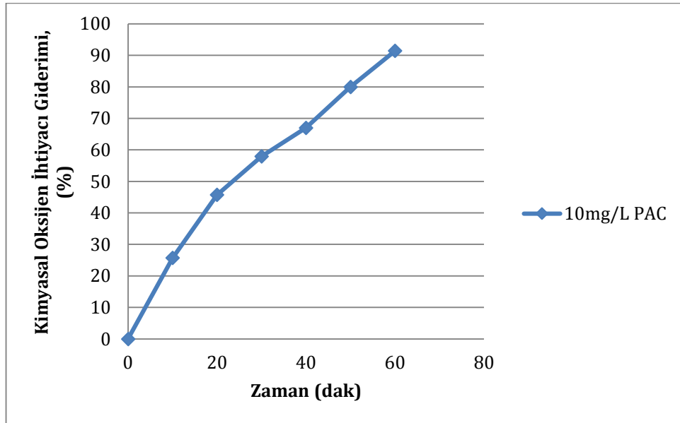
Şekil 7.32 Elektrokimyasal çöktürme (RASHIG halkası şeklindeki demir elektrot) yöntemiyle gerçekleştirilen arıtım çalışması, 10 mg/L PAC ilavesi ile zamana bağlı KOİ giderimlerinin değişimi
