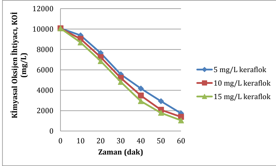
Şekil 7.13. Elektrokimyasal çöktürme (paralel plaka demir elektrot) yöntemiyle gerçekleştirilen arıtım çalışmasında farklı derişimlerde keraflok ilavelerinde zamana bağı KOİ değerlerinin değışimi
