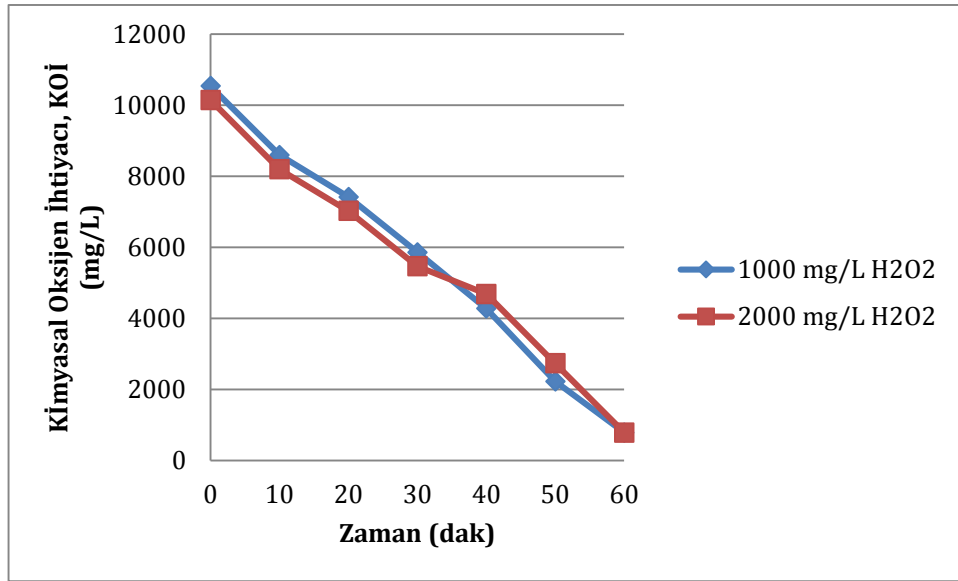
Şekil 7.39. Elektro-Fenton yöntemiyle gerçekleştirilen arıtım çalışmasında farklı H 2 O 2 derişimlerine bağı olarak zamanla KOİ yüklerinin değışimi.
