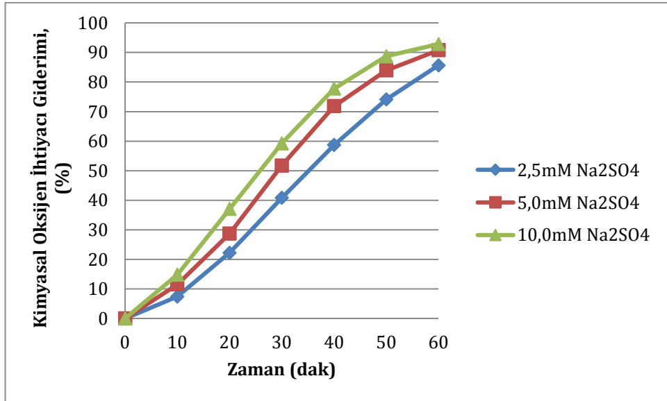
Şekil 7.8. Elektrokimyasal çöktürme (paralel plaka demir elektrot) yöntemiyle gerçekleştirilen arıtım çalışmasında farklı derişimlerde \text{Na}_2\text{SO}_4 ilavesinde KOİ giderimlerinin değişimi
