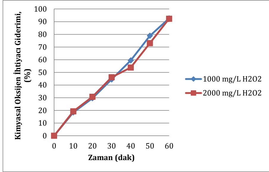
Şekil 7.40. Elektro-Fenton yöntemiyle gerçekleştirilen arıtım çalışmasında farklı H 2 O 2 derişimlerine bağı olarak zamana KOİ giderimlerinin değışimi
