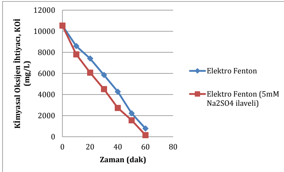
Şekil 7.42. Elektro-Fenton yöntemiyle gerçekleştirilen arıtım çalışması destek elektrolit ilavesine bağılı olarak zamanla KOİ yüklerinin değışimi.
