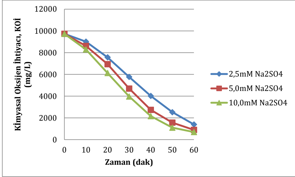
Şekil 7.7. Elektrokimyasal çöktürme (paralel plaka demir elektrot) yöntemiyle gerçekleştirilen arıtım çalışmasında farklı derişimlerde \text{Na}_2\text{SO}_4 ilavesinde KOİ yüklerinin değişimi
