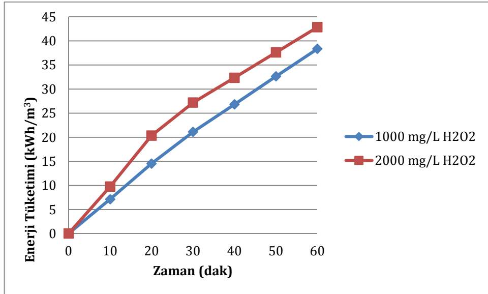
Şekil 7.41. Elektro-Fenton yöntemiyle gerçekleştirilen arıtım çalışmasında farklı H 2 O 2 derişimlerine bağı olarak enerji tüketimlerinin değışimi
