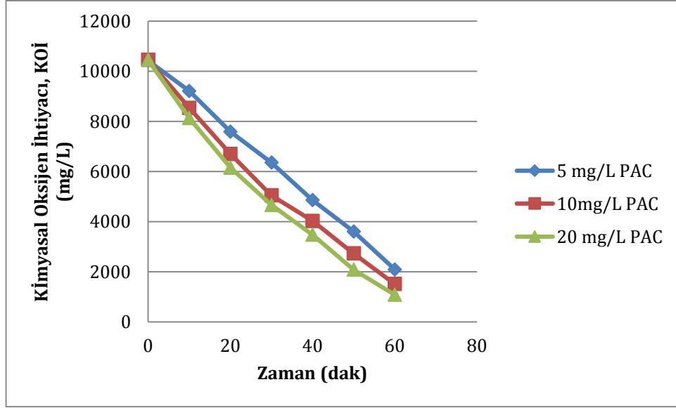
Şekil 7.10. Elektrokimyasal çöktürme (paralel plaka demir elektrot) yöntemiyle gerçekleştirilen arıtım çalışmasında farklı derişimlerde PAC ilavesinde zamanla KOİ değerlerinin değışimi.
