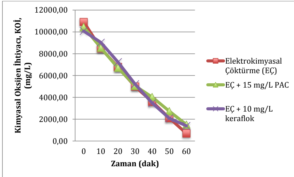
Şekil 7.16. Elektrokimyasal çöktürme (paralel plaka demir elektrot) yöntemiyle gerçekleştirilen artırım çalışmasında farklı koagülasyon yardımcıların ilavelerinde zamana bağlı KOİ değerlerinin değişimi
