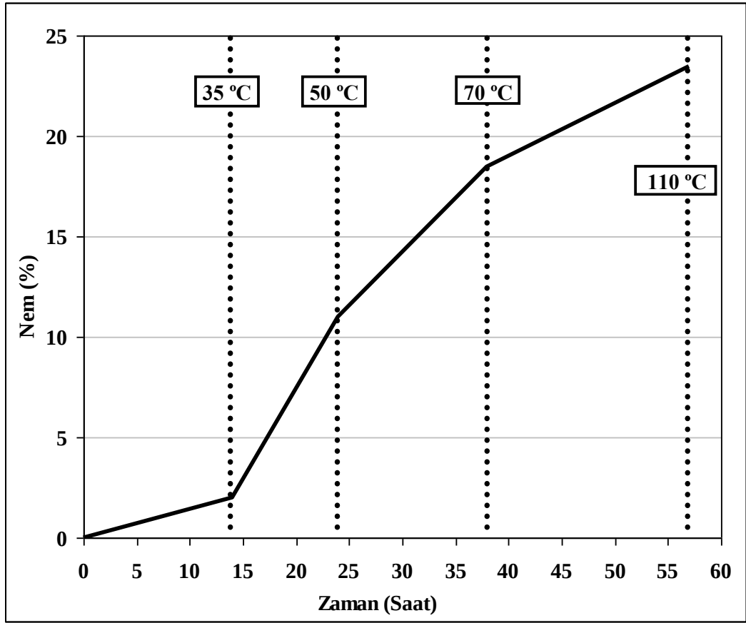
Şekil 3.17. Sıcaklık arttırımı ve ortalama kurutma davranışı
