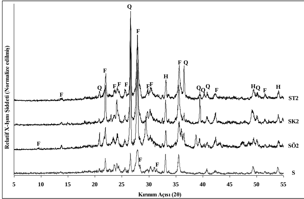
Şekil 4.23. Katkılı ve katkısız ürünlerin temsili XRD analizleri, Kuvars (Q), Müllit (M), Feldispat (F) ve Hematit (H)
