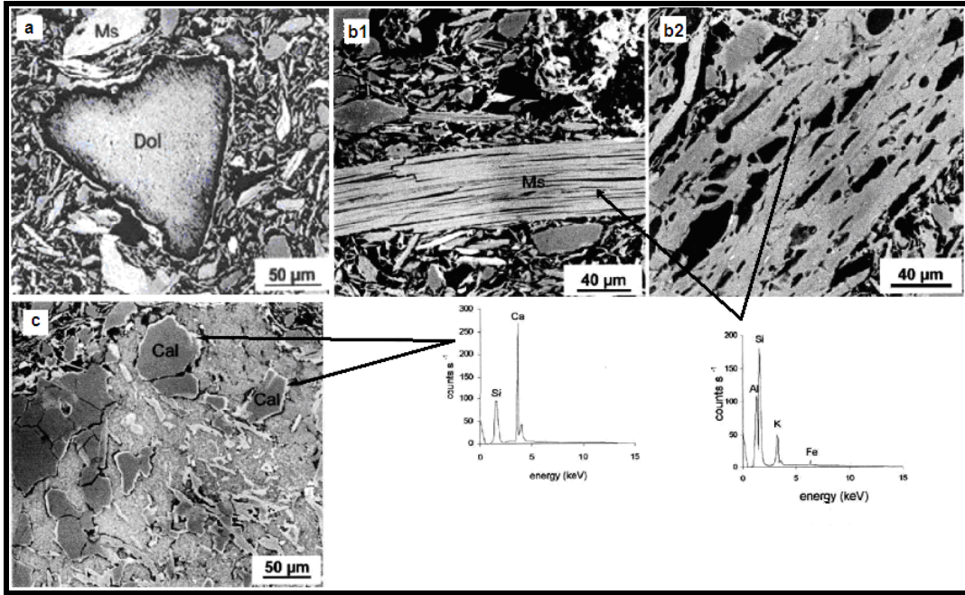
Şekil 2.9. Geri saçınımlı elektron mikroskobu (BE-SEM) görüntüleri (a) dolomit (Dol), (b1 ve b2) muskovit (Ms) ve (c) kalsiyum-silikat (Cal) (Cultrone, 2001)
