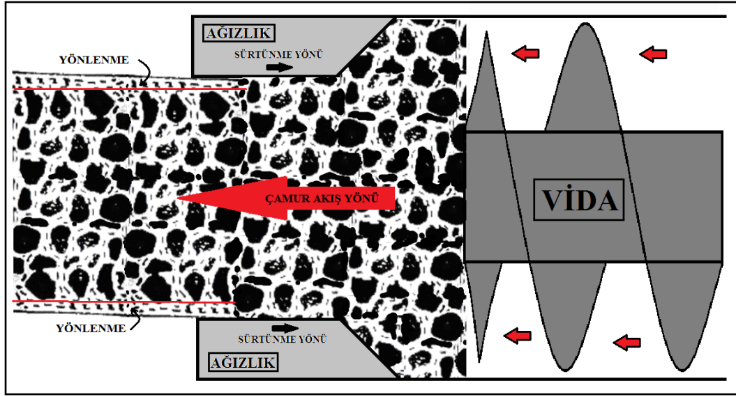
Şekil 4.4. Yaş şekillendirme ve pürüzsüz yüzey oluşumu
