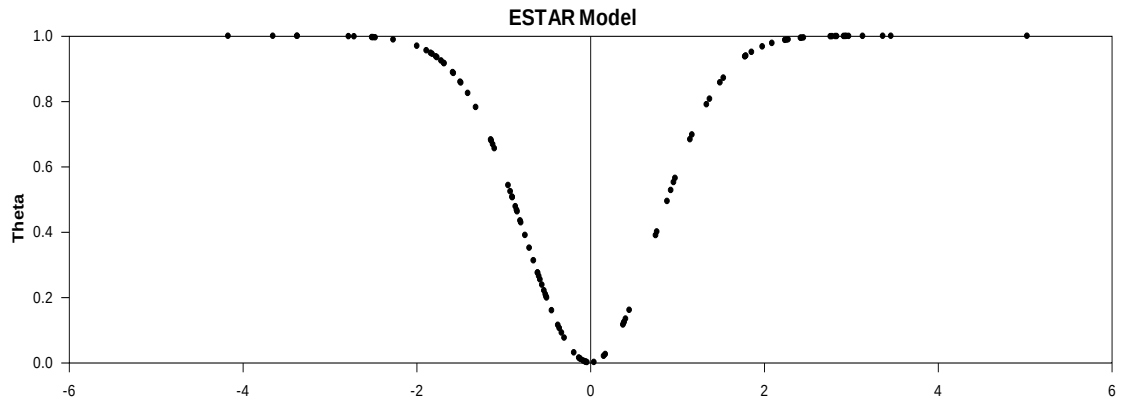
Şekil 16. Hindistan için ESTAR fonksiyonunun geçiş değişkeni etrafındaki dağılım fonksiyonu:
