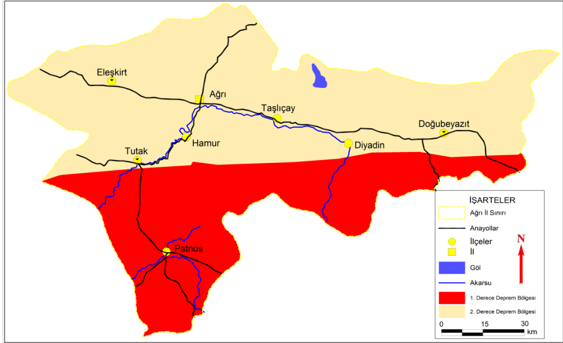
Şekil 4: Ağrı İlinin Deprem Haritası (Kaynak: Bayındırlık ve İskân Bakanlığı'nın Haritasından Düzenlenmiştir.)
