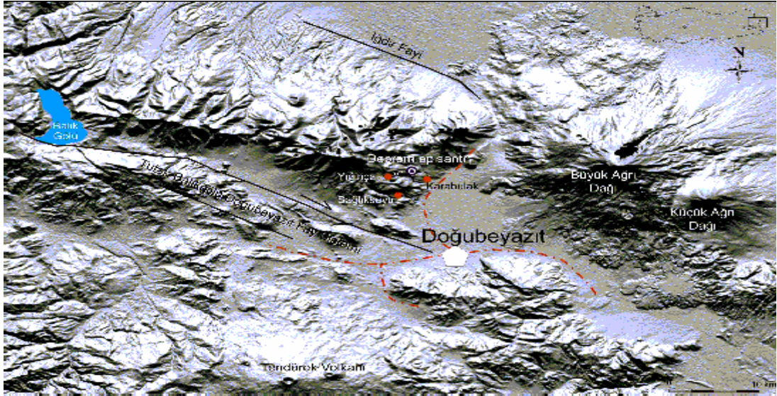
Şekil 5: Doğubeyazıt'ın Çevresinde Bulunan Bazı Fay Zonları (Kaynak: TAPAN-ÖZVAN-ŞENGÜL, 2005, age., s.1076.)
