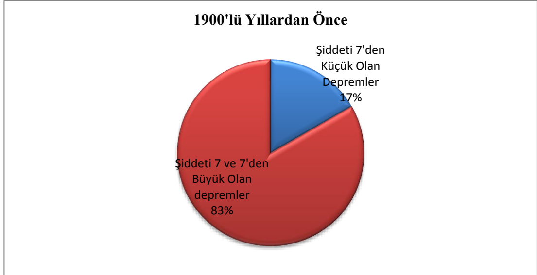
Şekil 6: Ağrı Dağı Çevresinde Meydana Gelen Depremlerin Büyüklüğü (Kaynak: YÜKSEL, 2009, age. , s.373-376)
