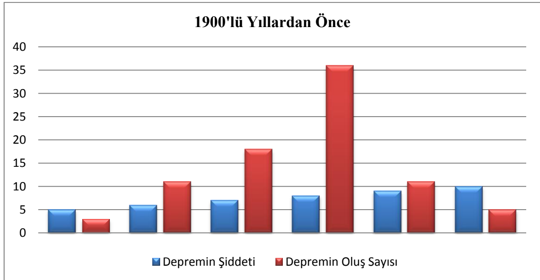
Şekil 7: Ağrı Dağı Çevresinde Meydana Gelen Depremlerin Büyüklükleri ve Meydana Geliş Sayıları (Kaynak: YÜKSEL, 2009, age. , s.372.)
