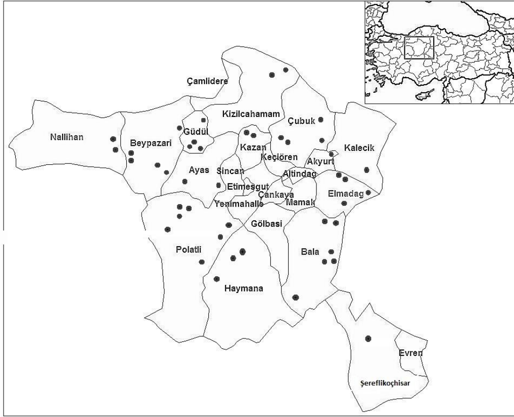
Şekil 2.1. Örnekleme yapılan Ankara ilçeleri ve istasyonlar
