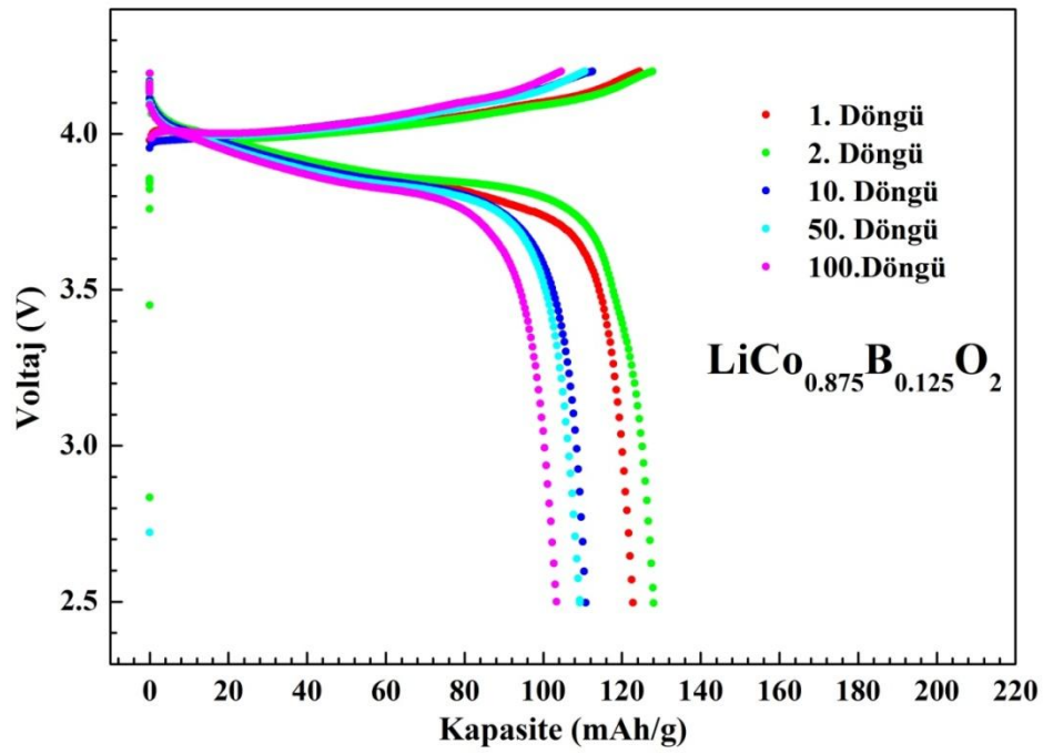
Şekil 3.38. Üretilen \text{LiCo}_{0.875}\text{B}_{0.125}\text{O}_2 malzemesinin katot olarak kullanıldığı pilin kapasitesinin 2.5-4.2 V aralığındaki değişimi.
