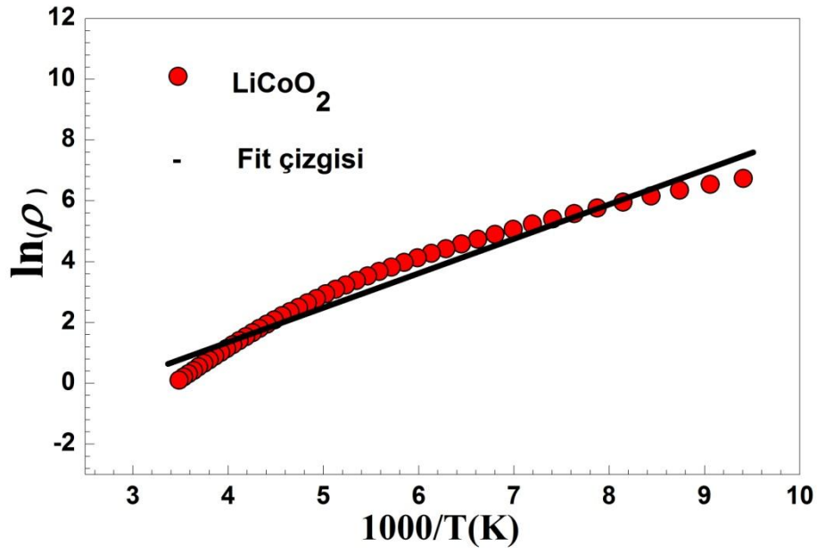
Şekil 3.6. Katkılama yapılmamış örneğin lineer fit edilmiş Arrhenius grafiği.
