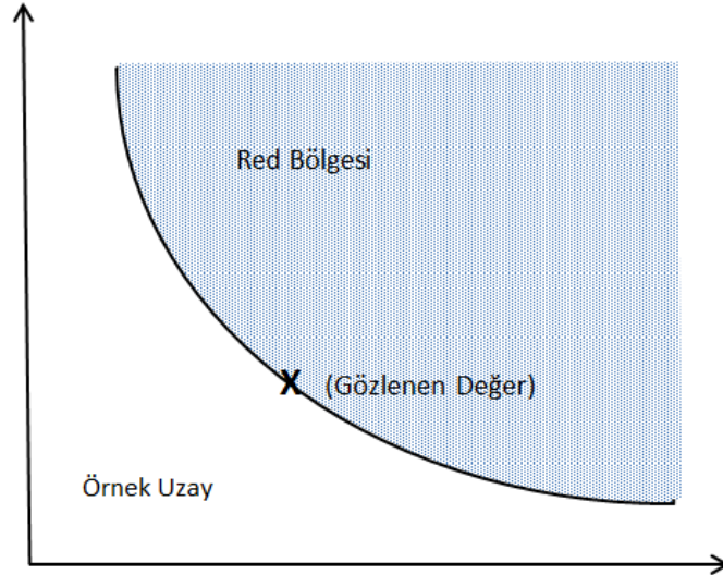
Şekil 1.1. Hipotez testleri için genelleştirilmiş red bölgesi.
