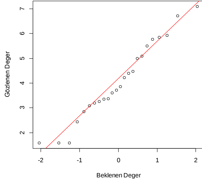
Şekil 5.17. Logaritması alınmış 1. grup için normallik grafiği.
