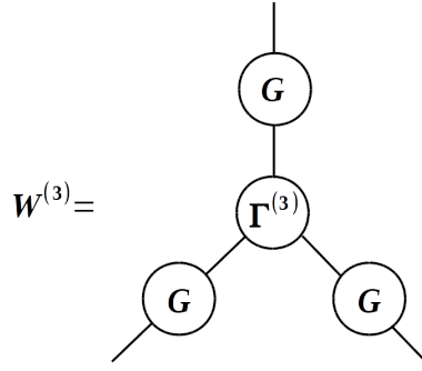
Şekil 4.1: Üçüncü mertebede W[J] ve \Gamma[\phi] arasındaki ilişkinin grafik temsili.
