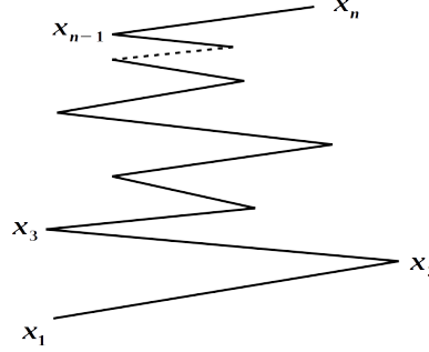
Şekil C.1: Yol integralini hesaplanabilmesi için, yol öncelikle çok sayıdaki ara noktalar üzerinden kesikli hale getirilir.
