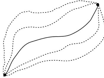
Şekil C.2: Yol integrali, konfigürasyon uzayında iki noktayı birleştiren tüm olası yollar üzerinden toplam içerir.
