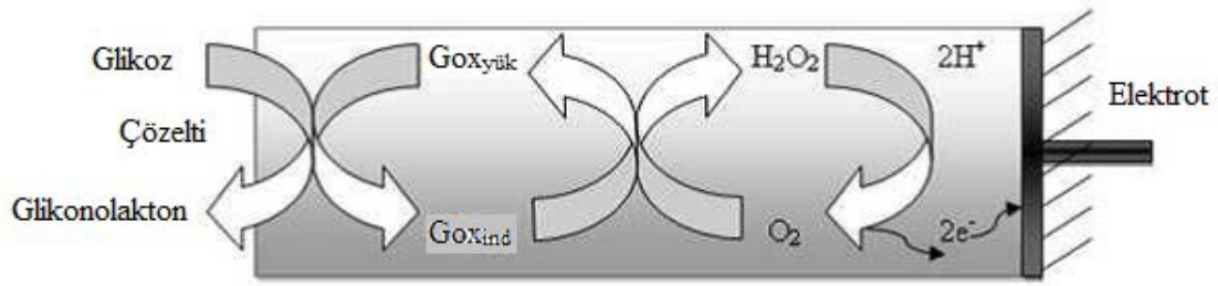
Şekil 4.3. Glikoz tayini için hazırlanan enzim elektrodun çalışma prensibi (Erdem, 2012)
