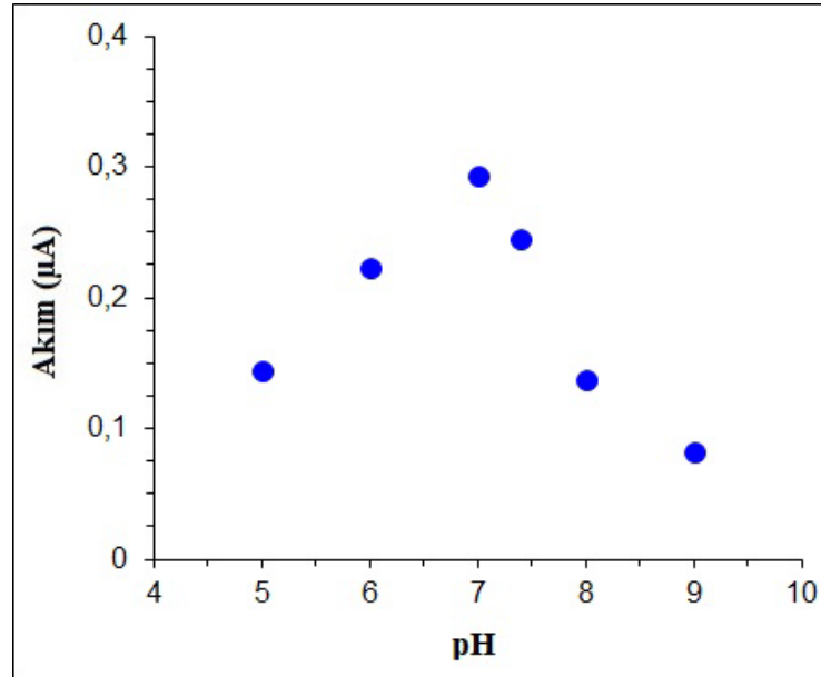
Şekil 8.8. Gox-PoPD/PtNPs/PVF + ClO 4 - /Pt biyosensörü için akım cevabı üzerine pH'ın etkisi (2,02×10 -7 mol PVF cm -2 2,0 mM H 2 PtCl 6 2,00×10 -2 C Pt film kalınlığı, 5 \mu M oPD, 1,0 mg Gox mL -1 , pH'ı 5,0-9,0 aralığında 0,1 M fosfat tamponu, 30°C)
