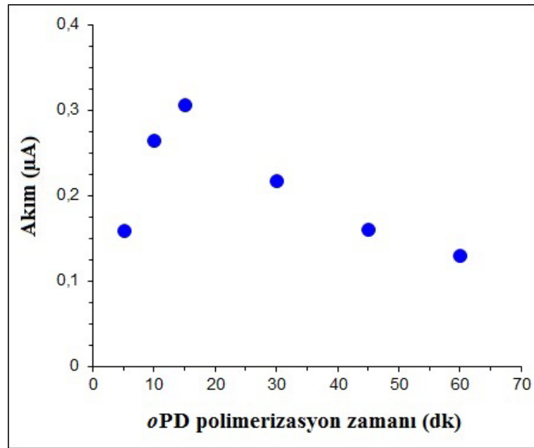
Şekil 8.5. Gox-PoPD/PtNPs/PVF + ClO 4 /Pt biyosensörüne oPD filminin elektropolimerizasyon süresinin akım cevabı üzerine etkisi ( 2,02 \times 10^{-7} mol PVF cm -2 , 2,0 mM H 2 PtCl 6 , 2,00 \times 10^{-2} C Pt film kalınlığı, 5µM oPD, 1,0 mg Gox mL -1 , 0,10 M pH 7,4 fosfat tamponu, 30°C)
