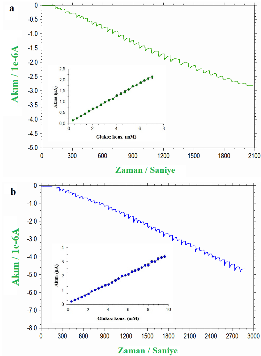
Şekil 9.2.(a) Gox-PoPD/PtNPs/PVF + ClO 4 - /Pt ve (b) Gox-PoPD /PVF + ClO 4 - /Pt biyosensörlerinin akım cevaplarının ölçüm ortamına eklenen glikoz konsantrasyonu ile değişimi ( 2,02 \times 10^{-7} mol PVF cm -2 2,0 mM H 2 PtCl 6 2,00 \times 10^{-2} C Pt film kalınlığı, 5 \mu M oPD, 0,10 M pH 7 fosfat tamponu, 30°C)
