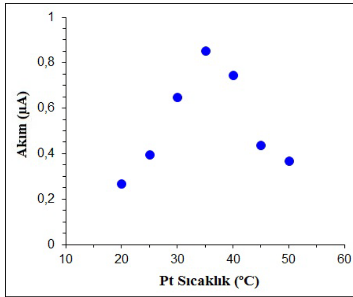
Şekil 8.9. Gox-PoPD/PtNPs/PVF + ClO 4 - /Pt biyosensörü için akım cevabı üzerine sıcaklığın etkisi (2,02×10 -7 mol PVF cm -2 2,0 mM H 2 PtCl 6 2,00×10 -2 C Pt film kalınlığı, 5µM oPD, 1,0 mg Gox mL -1 , 0,10 M pH 7 fosfat tamponu)
