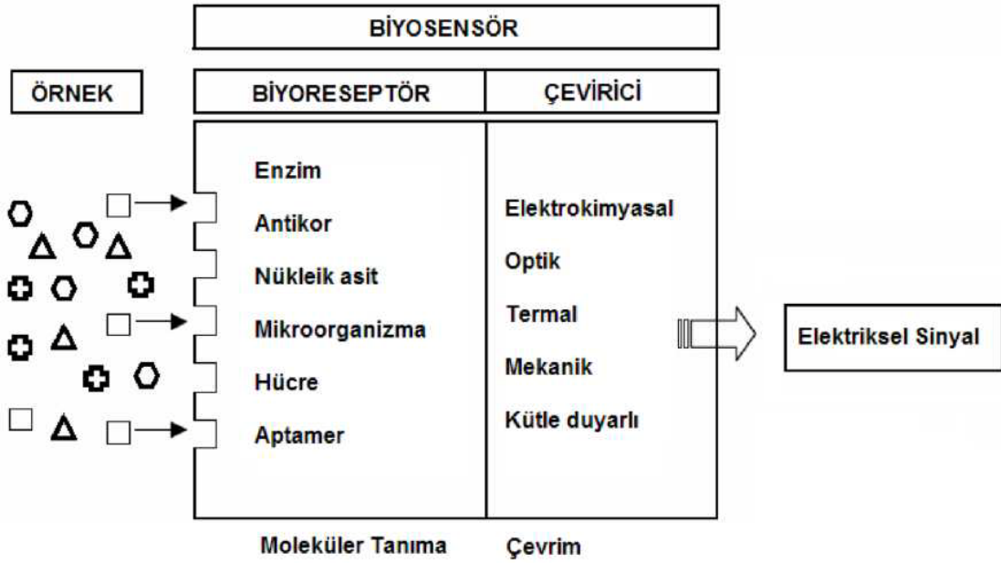
Şekil 2.3. Biyosensörlerin yapısı ve çalışma prensibi (Temiz, 2006)
