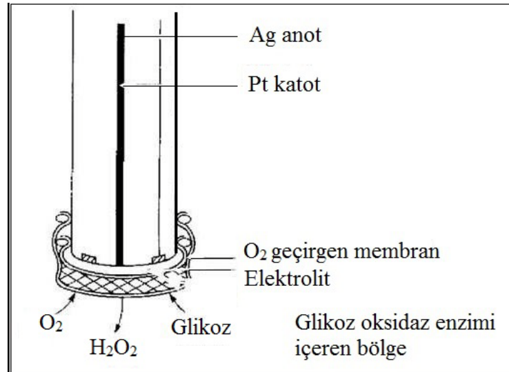
Şekil 2.1. Clark'ın enzim elektrodu
