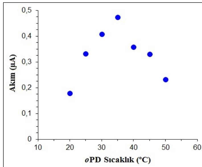
Şekil 8.9. Gox-PoPD/PtNPs/PVF + ClO 4 - /Pt biyosensörü için akım cevabı üzerine sıcaklığın etkisi (2,02×10 -7 mol PVF cm -2 2,0 mM H 2 PtCl 6 2,00×10 -2 C Pt film kalınlığı, 5µM oPD, 1,0 mg Gox mL -1 , 0,10 M pH 7 fosfat tamponu)
