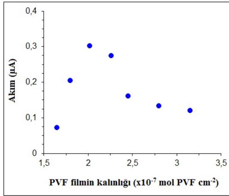
Şekil 8.4. Gox-PoPD/PtNPs/PVF + ClO 4 - /Pt biyosensörü için akım cevabı üzerine PVF + ClO 4 - film kalınlığının etkisi (5 μM oPD, 1,0 mg Gox mL -1 , 0,10 M pH 7,4 fosfat tamponu, 30°C)
