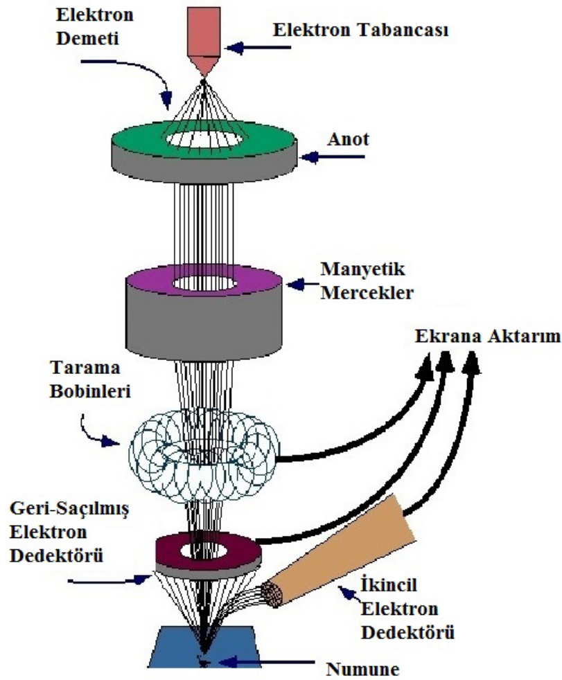
Şekil 7.4. Taramalı elektron mikroskopunun şematik görünüşü
