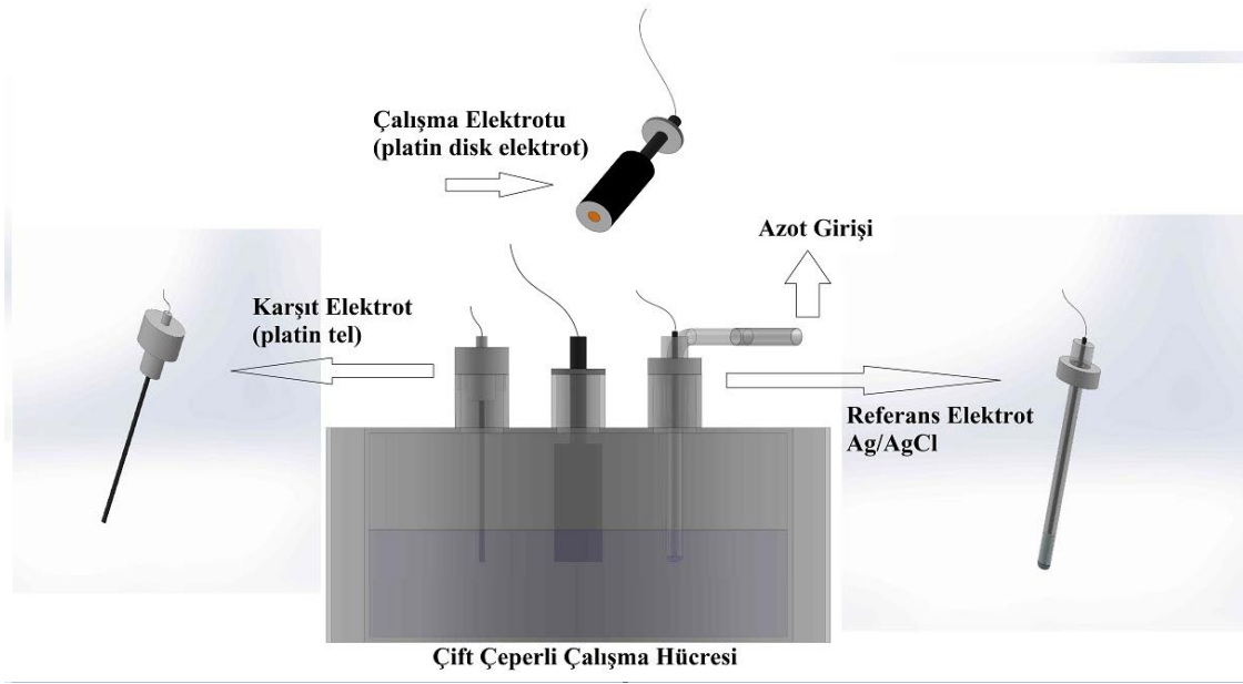
Şekil 7.1. Deneysel çalışmalarda kullanılan hücre ve elektrotlar
