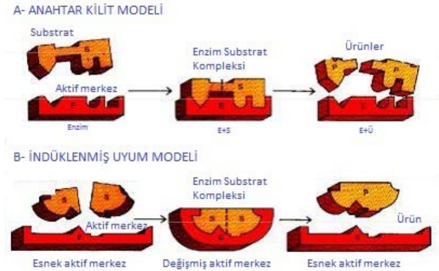
Şekil 3.2. Enzim-Substrat birleşme modelleri
