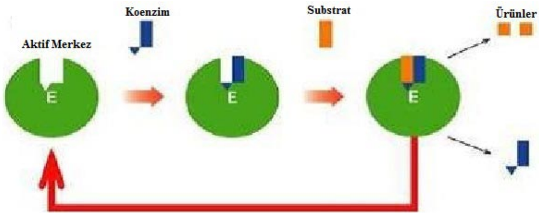
Şekil 3.1. Bir aktif enzimin yapısı
