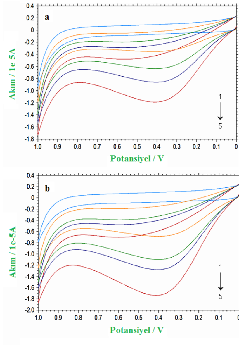
Şekil 8.1. (a) PoPD/PtNPs/PVF + ClO 4 - /Pt elektrodunun 0 mM(1), 0.5 mM(2), 1 mM(3), 1.5 mM(4), 2 mM(5) H 2 O 2 eklenmesiyle elde edilen voltamogramları. (b) Gox-PoPD/PtNPs/PVF + ClO 4 - /Pt elektrodunun 0 mM(1), 1 mM(2), 2 mM(3), 3 mM(4), 4 mM(5) glikoz eklenmesiyle elde edilen voltamogramları. Tarama hızı: 100 mVs -1
