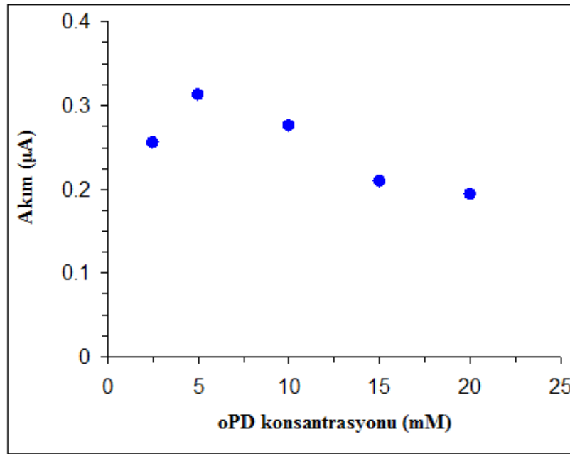
Şekil 8.6. Gox-PoPD/PtNPs/PVF + ClO 4 - /Pt biyosensörüne oPD konsantrasyonunun akım cevabı üzerine etkisi (2,02 \times 10^{-7} mol PVF cm -2 2,0 mM H 2 PtCl 6 2,00 \times 10^{-2} C Pt film kalınlığı, 2,5-20 \mu M oPD, 1,0 mg Gox mL -1 , 0,10 M pH 7,4 fosfat tamponu, 30°C)
