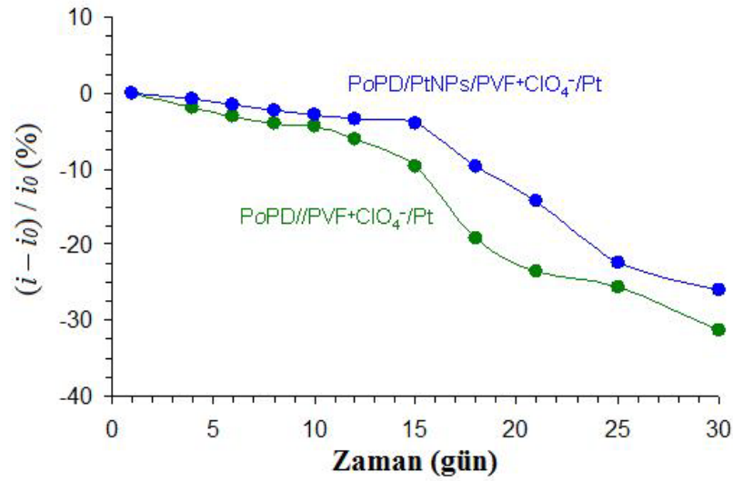
Şekil 8.12. Gox-PoPD/PtNPs/PVF + ClO 4 - /Pt ve Gox-PoPD/PVF + ClO 4 - /Pt biyosensörlerinin akım depolanma kararlılığı (2,02×10 -7 mol PVF cm -2 2,0 mM H 2 PtCl 6 2,00×10 -2 C Pt film kalınlığı, 5µM oPD, 1,0 mg Gox mL -1 , pH'ı 7 olan 0,1 M fosfat tamponu, 30°C)
