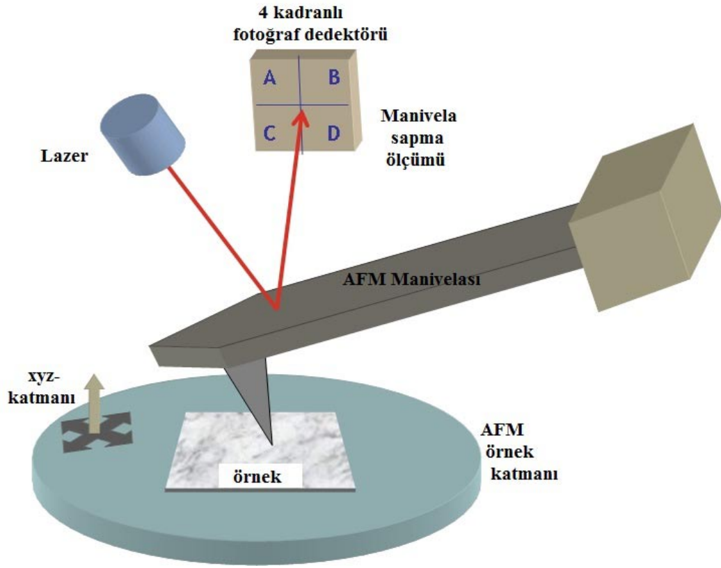
Şekil 7.5. Atomik kuvvet mikroskobu şematik görünüşü
