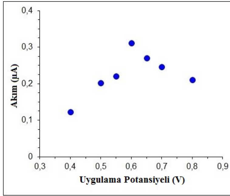
Şekil 8.3. Gox-PoPD/PtNPs/PVF + ClO 4 - /Pt biyosensörüne akım cevabı üzerine uygulama potansiyelinin etkisi (2,02×10 -7 mol PVF cm -2 2,0 mM H 2 PtCl 6 2,00×10 -2 C Pt film kalınlığı, 5μM oPD, 1,0 mg Gox mL -1 , 0,10 M pH 7,4 fosfat tamponu, 30°C)
