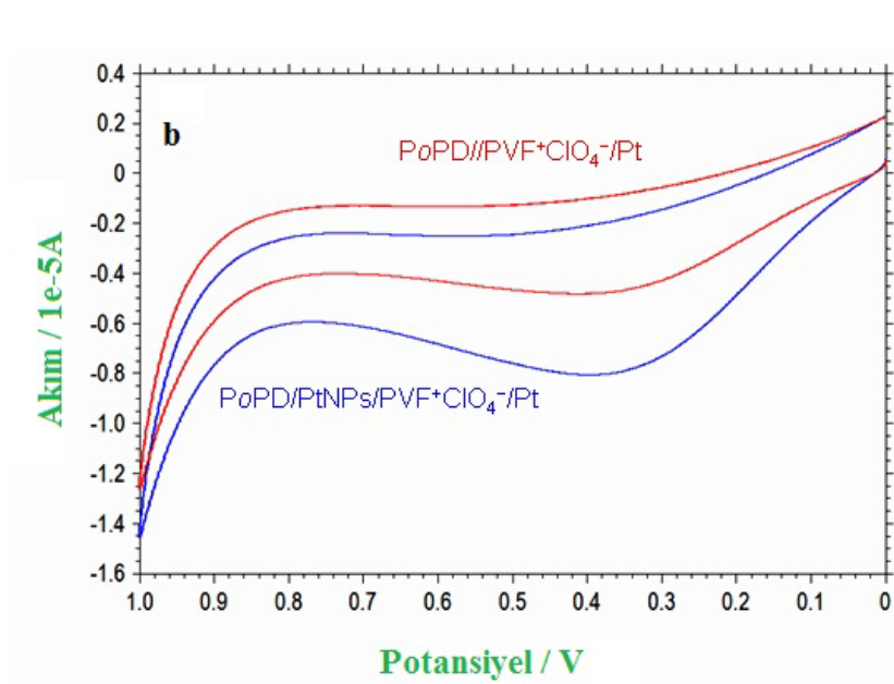
Şekil 8.2. PoPD/PVF + ClO 4 - /Pt ve PoPD/PtNPs/PVF + ClO 4 - /Pt elektrotlarının 1 mM H 2 O 2 eklenmesiyle elde edilen voltamogramları. Tarama hızı: 100 mV s -1
