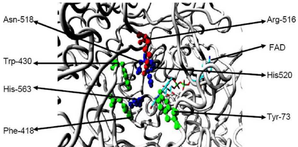
Şekil 4.2. Gox'ın monomerindeki FAD ve aktif bölge artıkları protein yapısı
