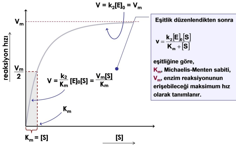
Şekil 3.4. Reaksiyon hızı-substrat konsantrasyonu grafiği
