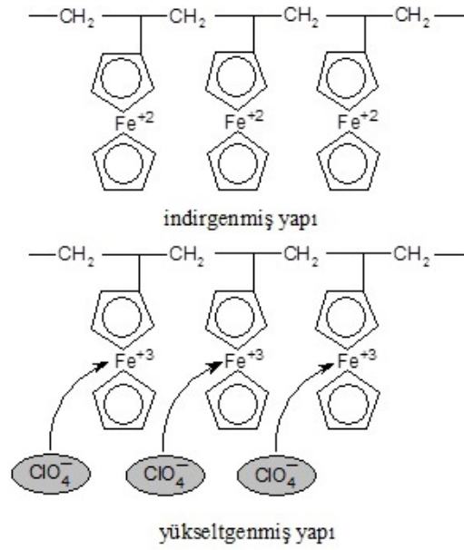
Şekil 5.3. Polivinilferrosenin indirgenmiş ve yükseltgenmiş yapıları
