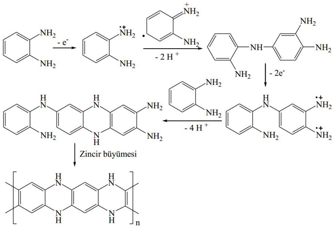
Şekil 7.11. Merdiven yapılı PoPD'nin oluşumu için önerilen mekanizma (Sivakkumar ve Saraswathi, 2004)
