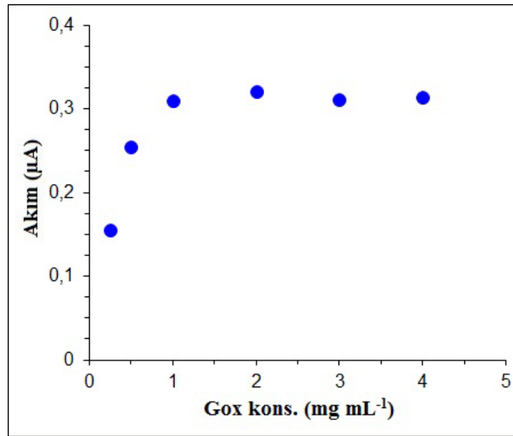
Şekil 8.7. Gox-PoPD/PtNPs/PVF + ClO 4 - /Pt biyosensörü için akım cevabı üzerine Gox enzim konsantrasyonunun etkisi ( 2,02 \times 10^{-7} \text{ mol PVF cm}^{-2} , 2,0 \text{ mM H}_2\text{PtCl}_6 , 2,00 \times 10^{-2} \text{ C Pt} film kalınlığı, 5 \mu\text{M oPD} , 0,10 \text{ M pH } 7,4 fosfat tamponu, 30^\circ\text{C} )
