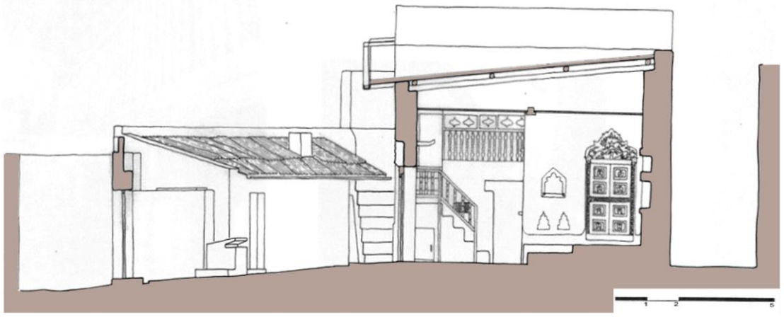
Resim 4.50: Aşa sabit evinin B-B kesiti (HPNRS, 31 Ocak 2004)
