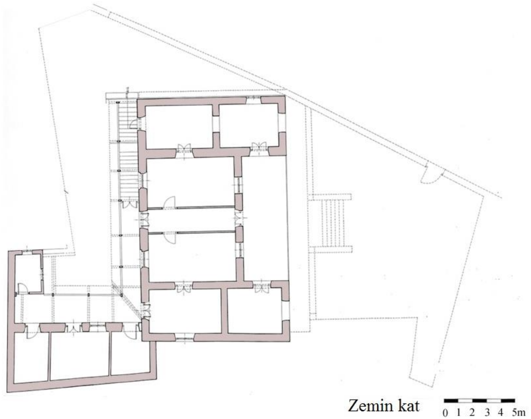
Resim 4.37: Ras teferi evin Zemin kat planı
