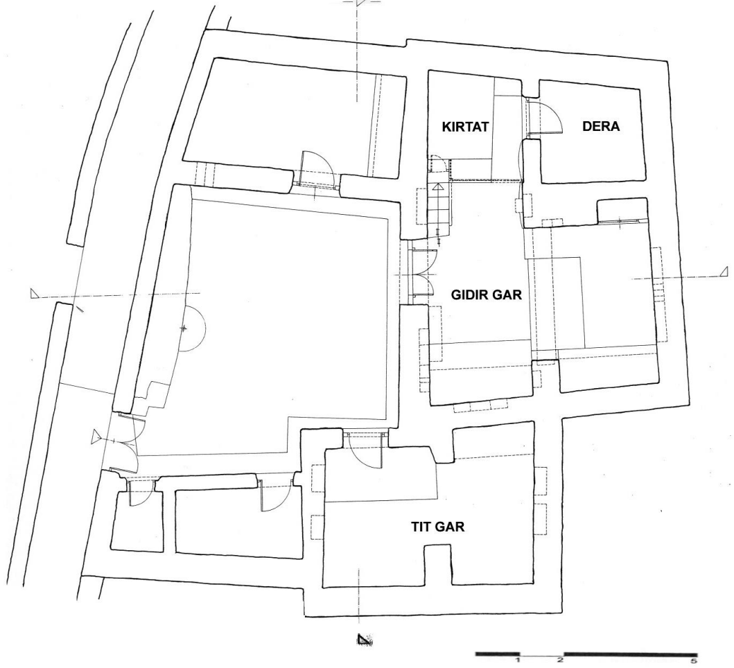
Resim 4.33: Mahdi hados evinin planı, ge gar tipinin örneği (HPNRS, 31 Ocak 2004)
