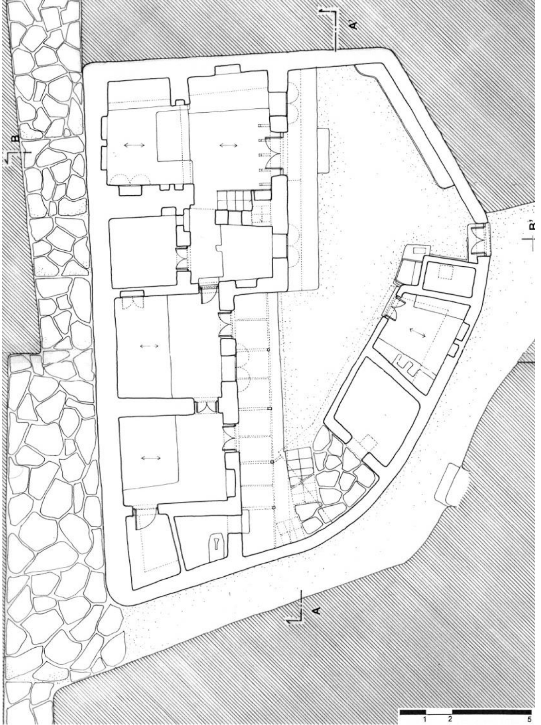
Resim 4.47: Aşa sabit evinin Zemin kat planı (HPNRS, 31 Ocak 2004)
