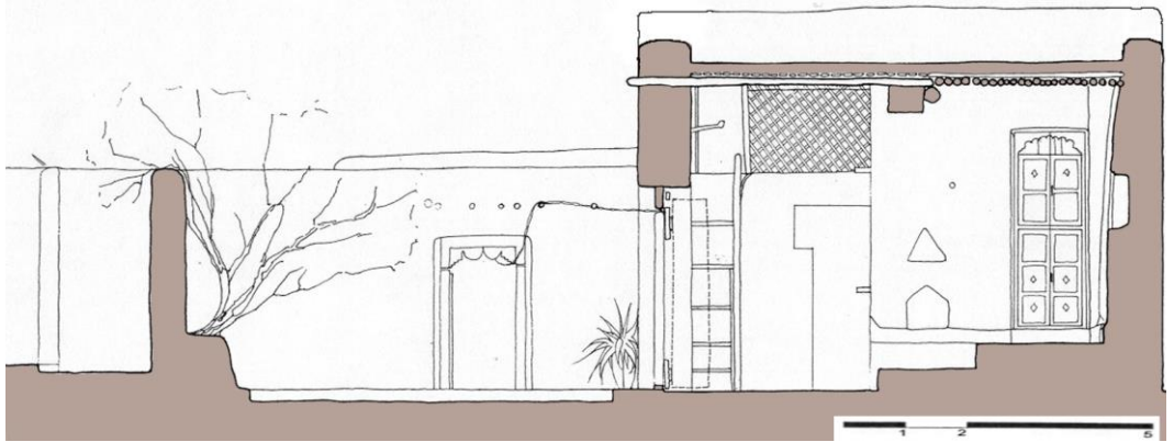
Resim 4.34: Mahdi hados evinin kesiti, ge gar tipinin örneği (HPNRS, 31 Ocak 2004)
