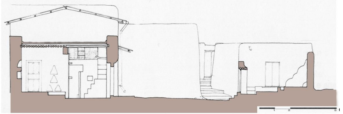
Resim 4.4: Şaş abdolis evi, A-A kesit (HPNRS, 31 Ocak 2004)
