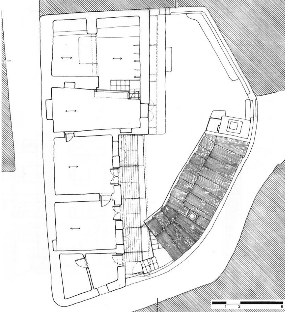
Resim 4.48: Aşa sabit evinin üst kat planı (HPNRS, 31 Ocak 2004)
