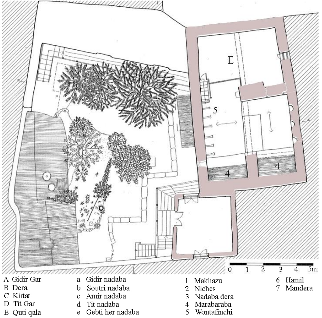
Resim 4.43: Kadija Ahmed evinin üst kat planı (Revault, Santelli, 2004, s:136)
