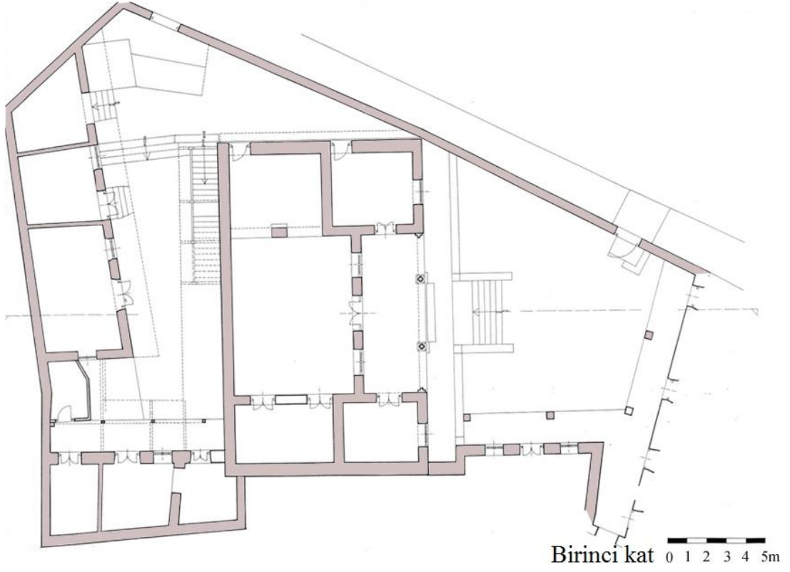
Resim 4.38: Ras teferi evin üst kat planı (Revault, Santelli, 2004, s:139)
