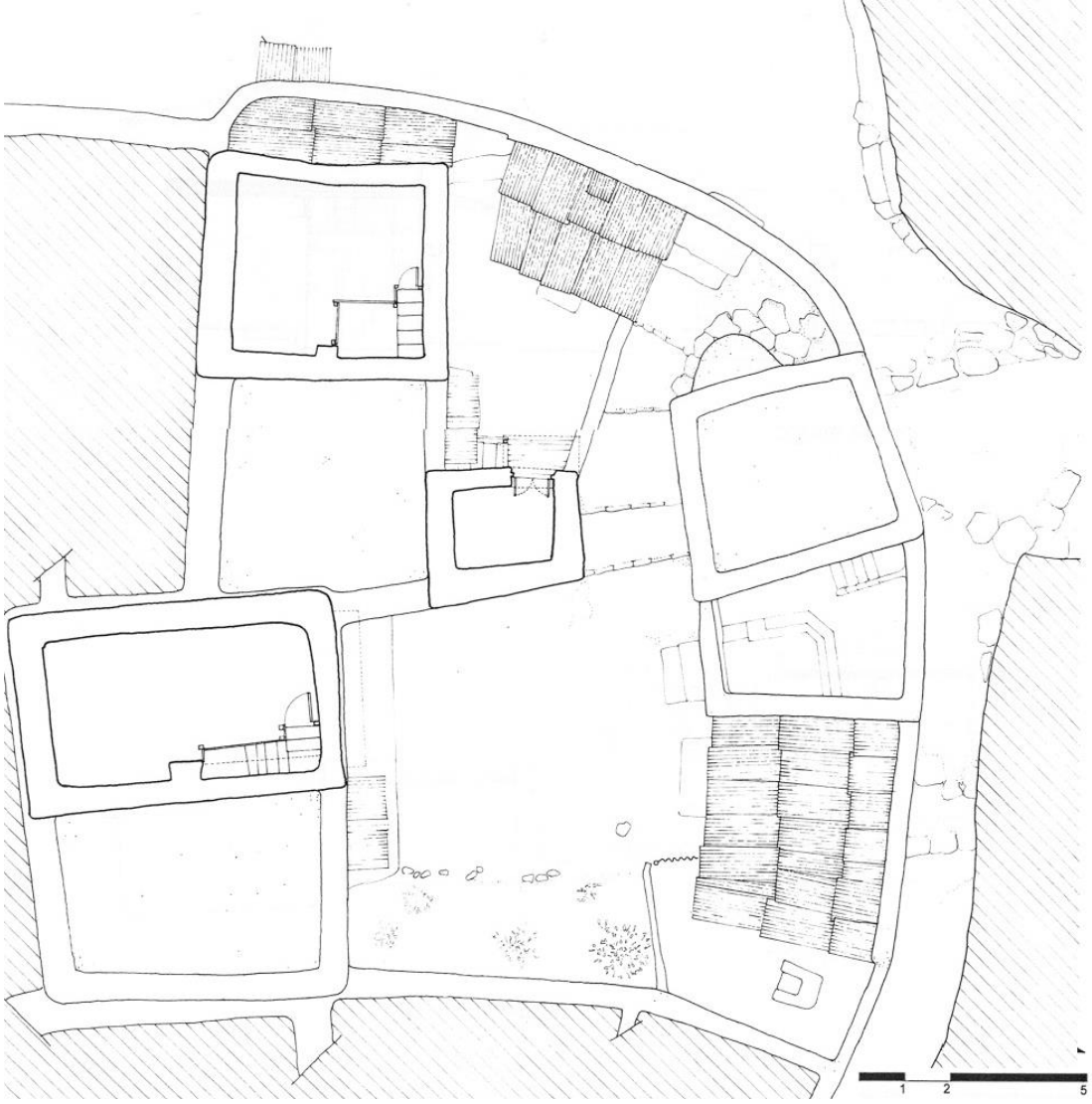
Resim 4.2: Şaş abdolis evinin üst kat planı (HPNRS, 31 Ocak 2004)
