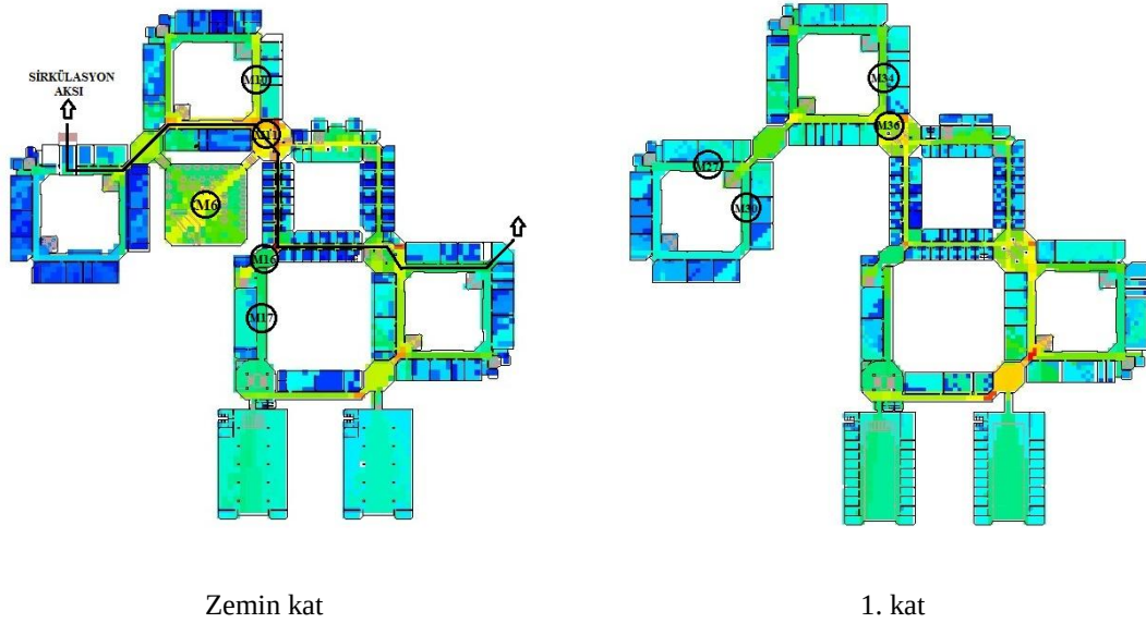
Şekil 5.4. Mühendislik Fakültesi bütünleşme grafiği ile sosyal etkileşim mekanlarının ilişkisi
