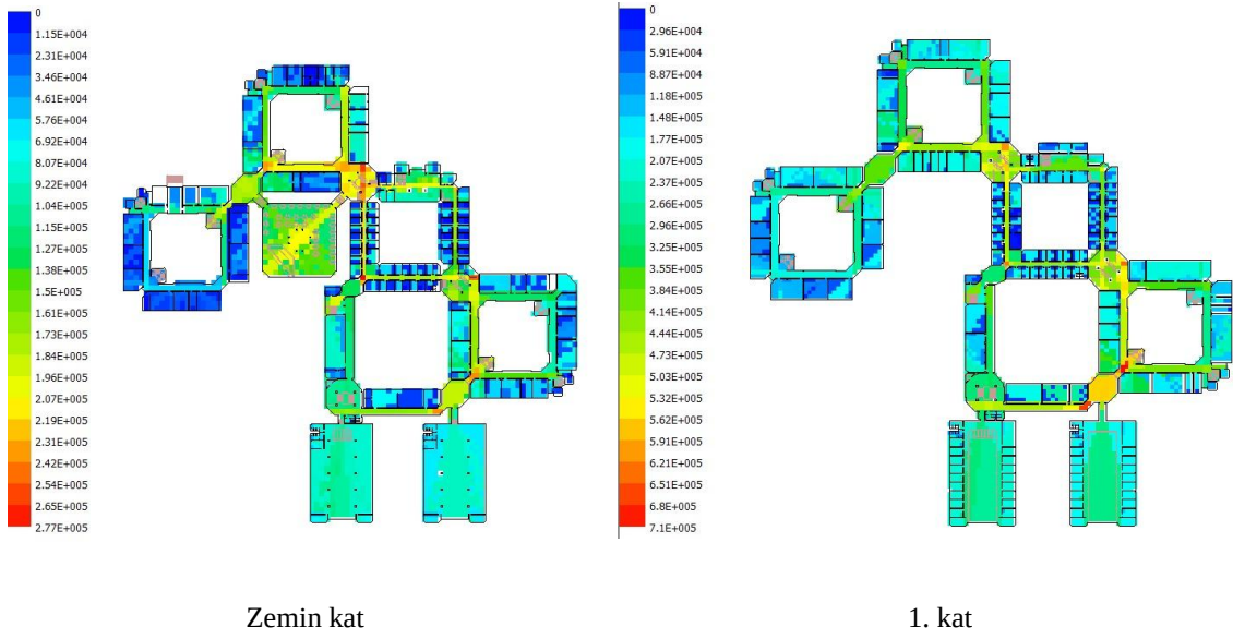
Şekil 5.3. Mühendislik Fakültesi kat planlarının bütünleşme (integration-n) grafiği
