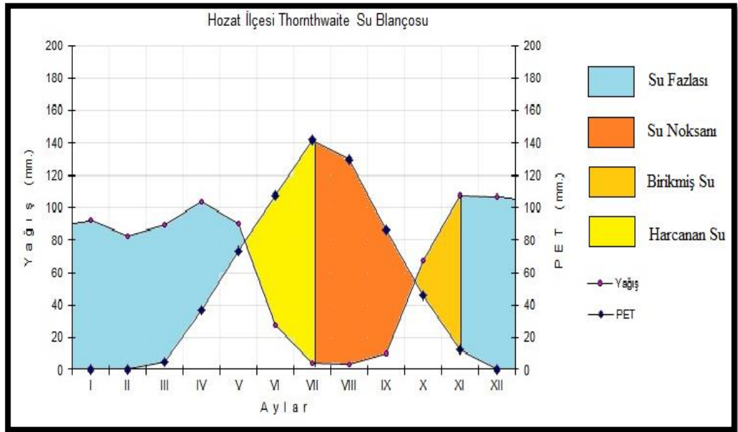
Şekil 14. Hozat İlçesinin 1966-1995 Dönemine Ait Thornthwaite Su Blançosu Diyagramı
