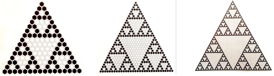
Şekil 4.25: Pascal üçgeninde 2 ile tam bölünebilirlik
