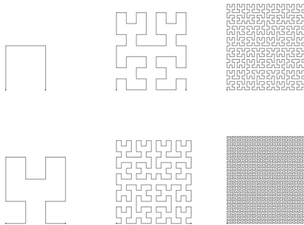
Şekil 4. 32: Hilbert uzayı algoritması
