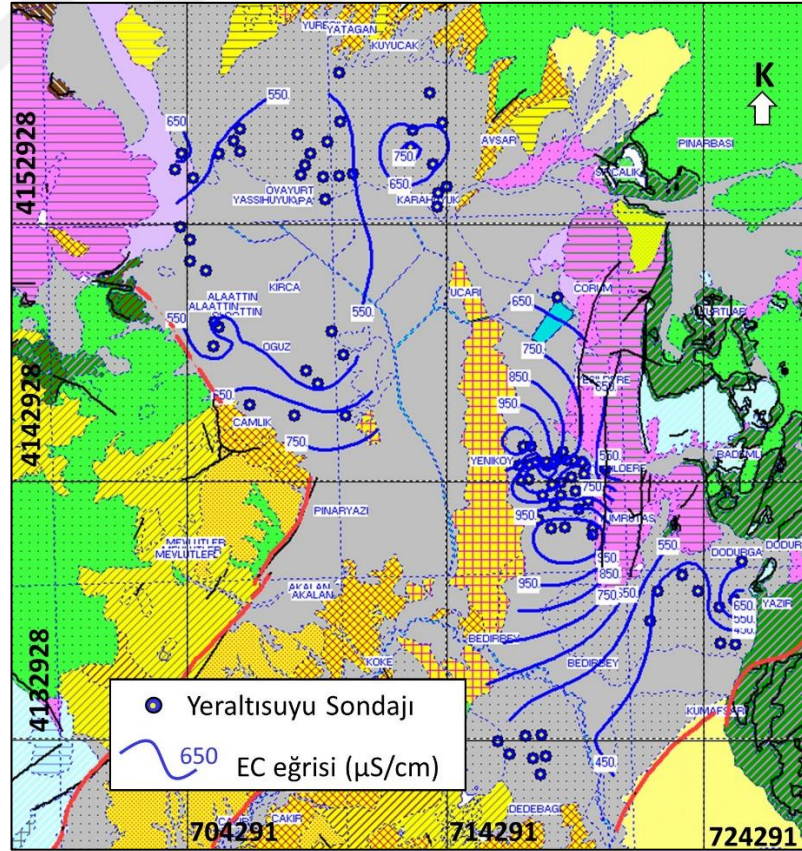
Şekil 5.13: a) YAS-CBS sistemi kullanılarak elde edilen Acıpayam ovası YAS PH haritası, b) YAS elektriksel iletkenlik (EC) haritası (Kumsar ve Sarayköylü 2021).
