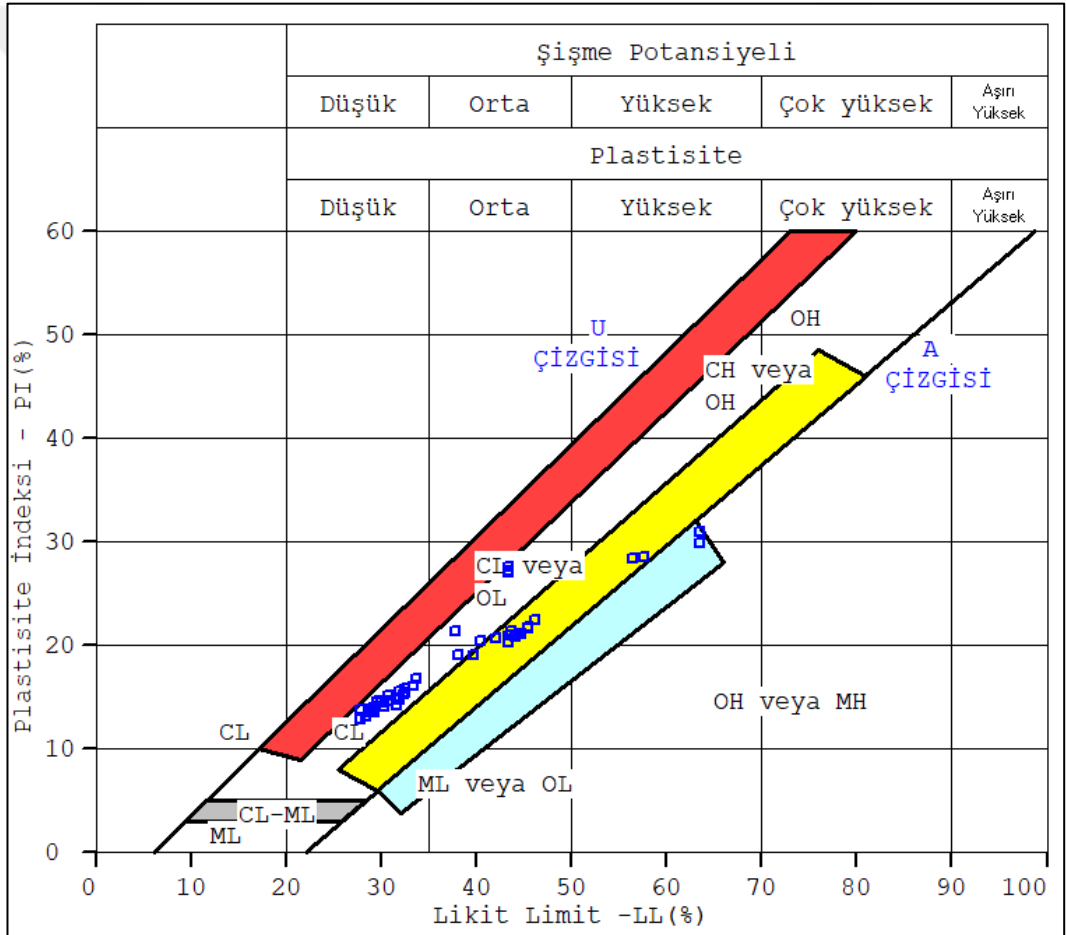
Şekil 6.29: Dakshanamurthy and Raman (1973) tarafından önerilen plastisite kartı üzerinde çalışma alanındaki zeminlerin sınıfları ve şişme potansiyeli ile ilişkisi.
