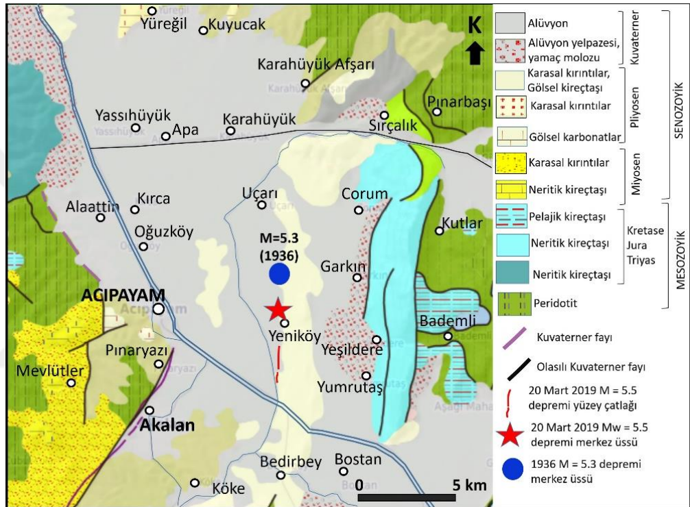
Şekil 4.7: Acıpayam ve civarının jeolojik ve tektonik yapısı, 1900 sonrası meydana gelen M > 5 depremlerin ve jeoteknik sondajların dağılımı (Emre ve diğ. 2013; MTA, 2019; Akbaş ve diğ. 2002; KOERI 2019; DDB 2019; Kondakçı 2017; Hançer ve diğ. 2022).
