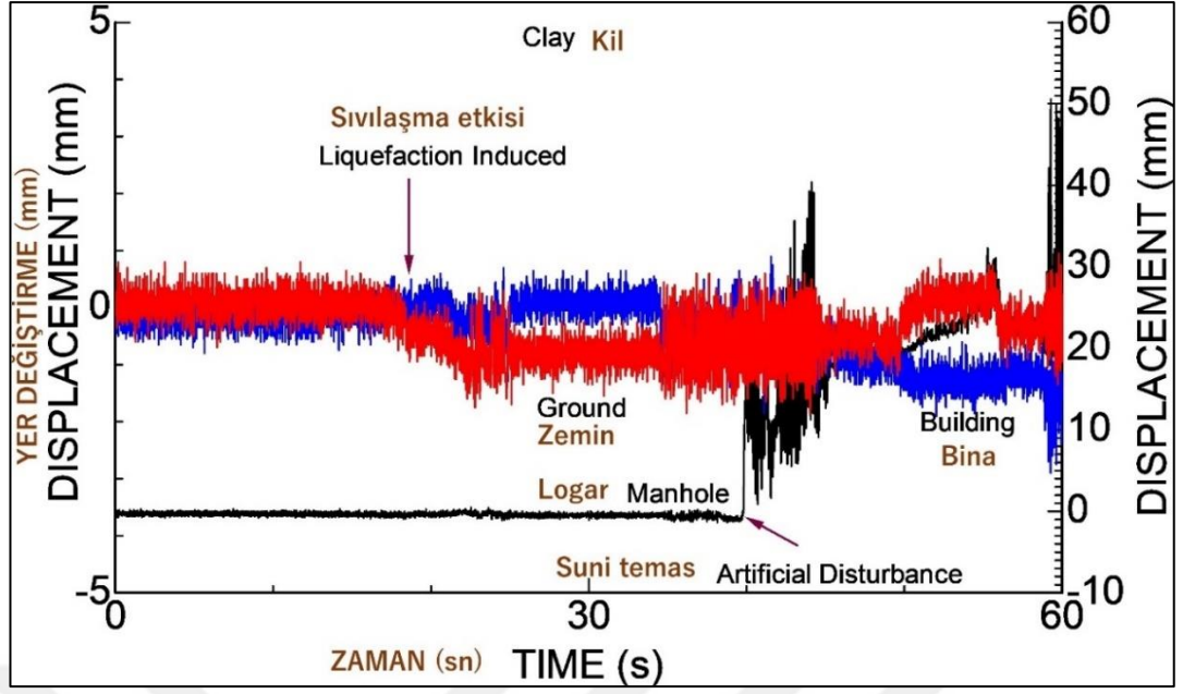
Şekil 7.11: Sıvılaşma model deneyi sırasında zeminde (ground), loggar (manhole) ve bina (building) modellerindeki yer değiştirme ölçümleri ve sıvılaşma (liquefaction) anının belirlenmesi
