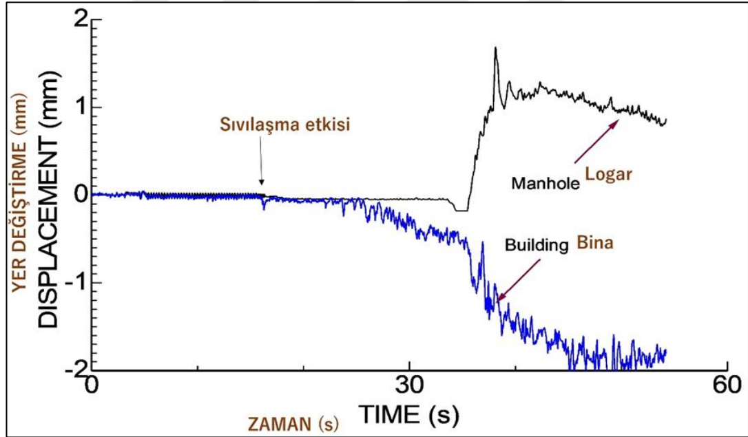
Şekil 7.12: Sıvılaşma modeli sırasında bina ve loggar modellerindeki yer değiştirme
