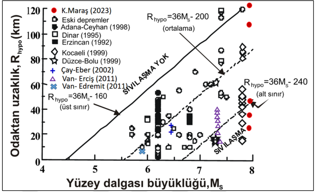
Şekil 7.4: Aydan ve diğ. (2000) tarafından geliştirilen Türkiye'deki depremlerde sıvılaşmanın gözlemlendiği alanların depremin odağına olan uzaklığı ile deprem büyüklüğü ( M_s ) arasındaki ilişki (Ulusay ve diğ. 2023'den alınmıştır).
