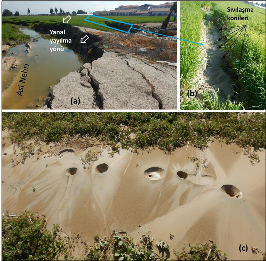
Şekil 7.2: Kahramanmaraş 6 Şubat 2023 depremleri sırasında meydana gelen a) Yanal yayılma, b) Yanal yayılma çatlağı içindeki zemin sıvılaşması, c) Zemin sıvılaşması sonucu oluşan kum kaynama kraterlerinin dizilimi (Resimler Halil KUMSAR’ dan alınmıştır).
