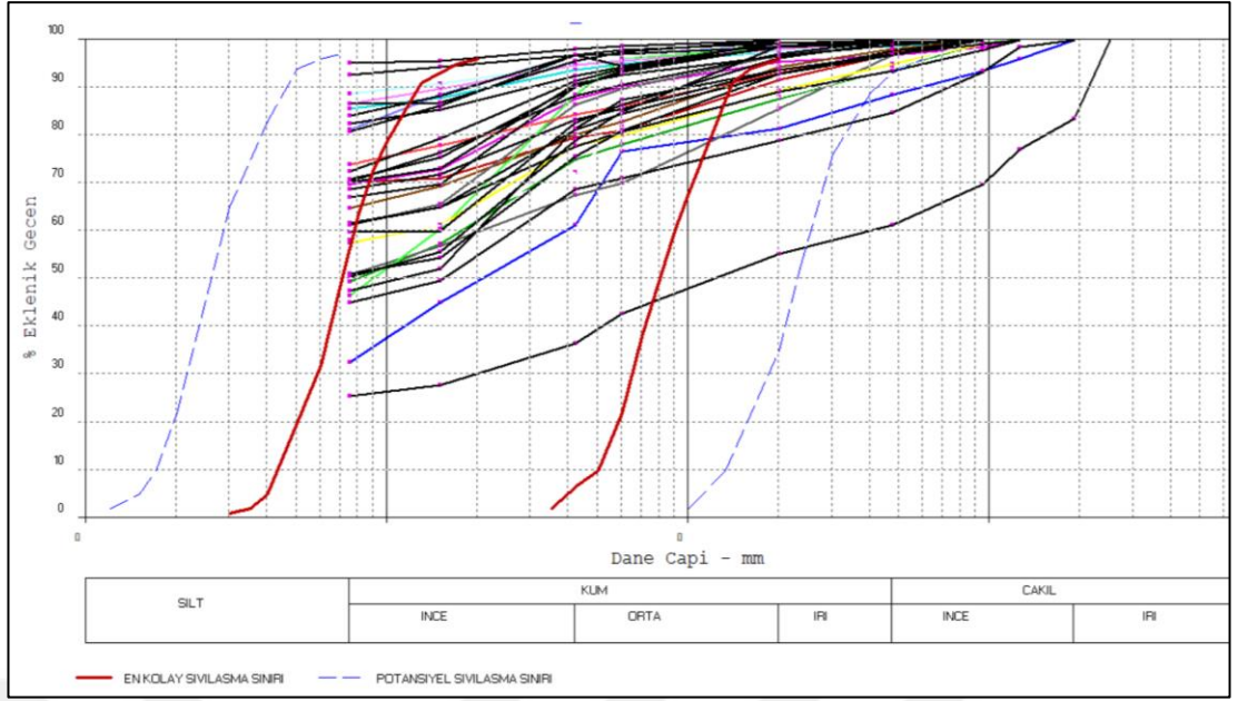
Şekil 7.6: Acıpayam ovası içinde açılan jeoteknik sondajlardan alınan zemin örneklerinin tane boyu dağılımı grafiği ve sınırları (Port and Harbour Research Institute of Japan, 1997) ile ilişkisi.
