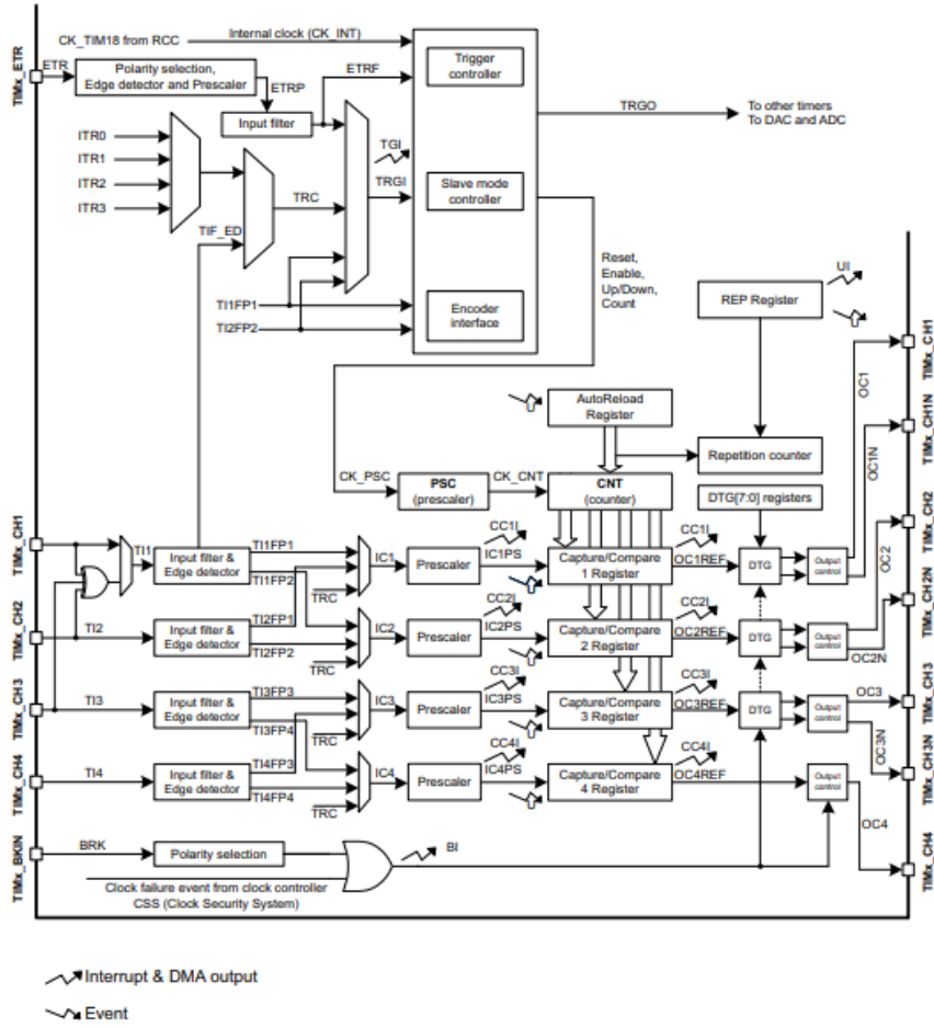
Şekil 2.2. Gelişmiş kontrol zamanlayıcı blok şeması (RM0008, 2021)
