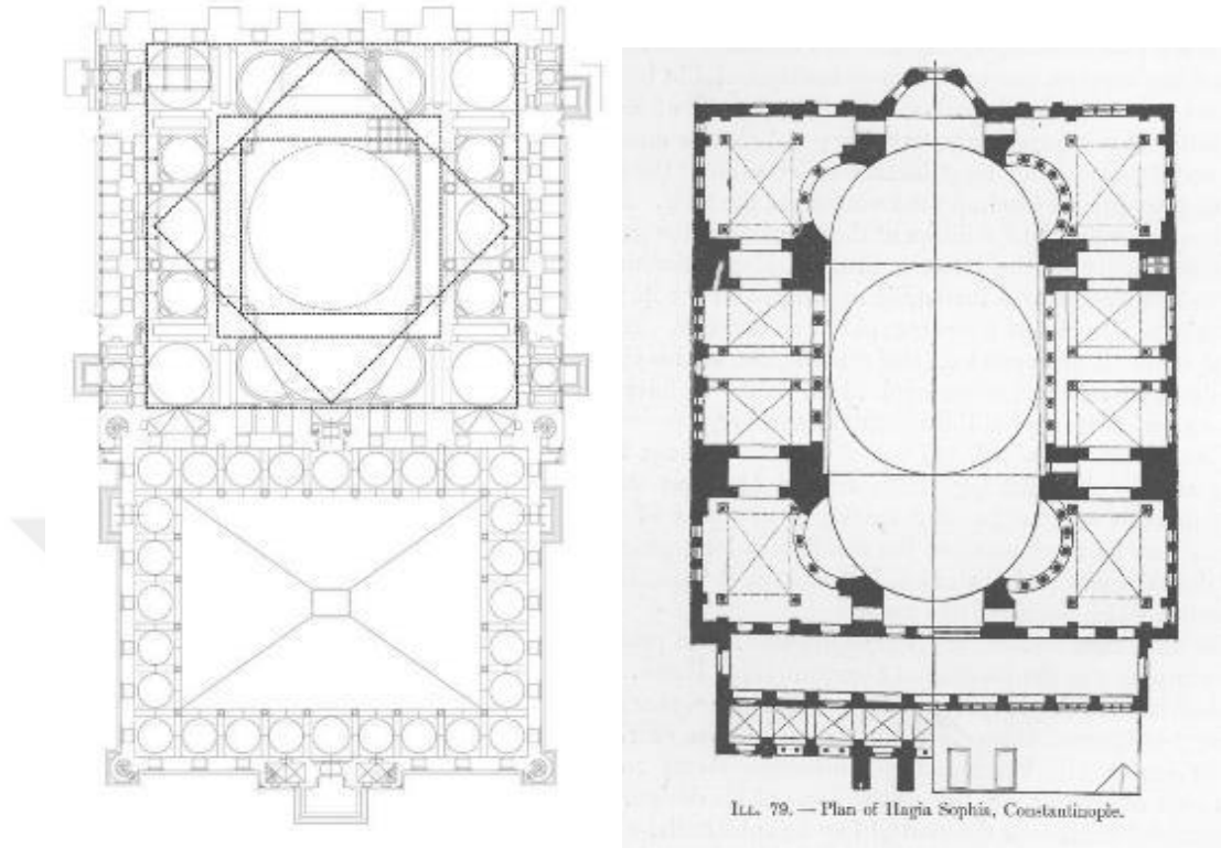
Resim 5. 112. Süleymaniye Camii Planı ve Ayasofya Planı (Sol Süleymaniye, Sağ Ayasofya)
