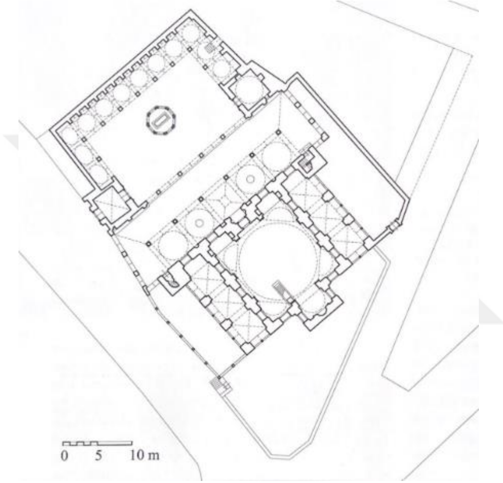
Resim 5. 79. Mesih Ali paşa Camii Vaziyet Planı (Necipoğlu, 2017)
