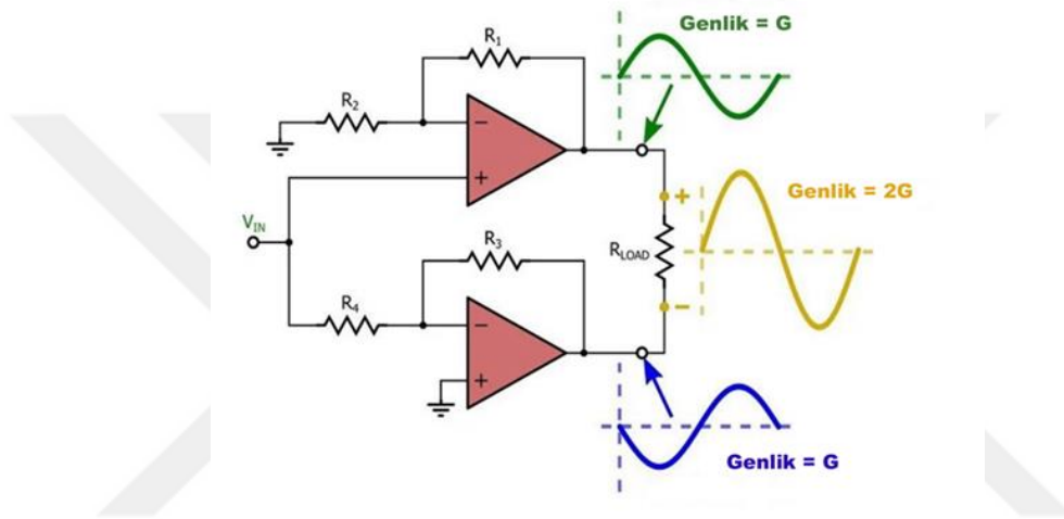
Şekil 3.9. Temel köprü yükselteç devresi ( R_1 , R_2 , R_3 : Farklı direnç değerleri, R_{LOAD} : Yük direnci) [57]
