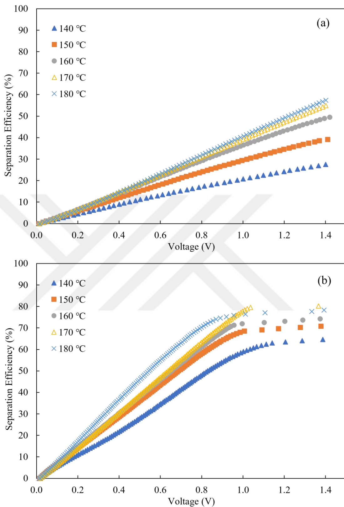
Figure 5.8 The separation efficiency of a) Pt/GNP, and b) PtRu/GNP catalyst
