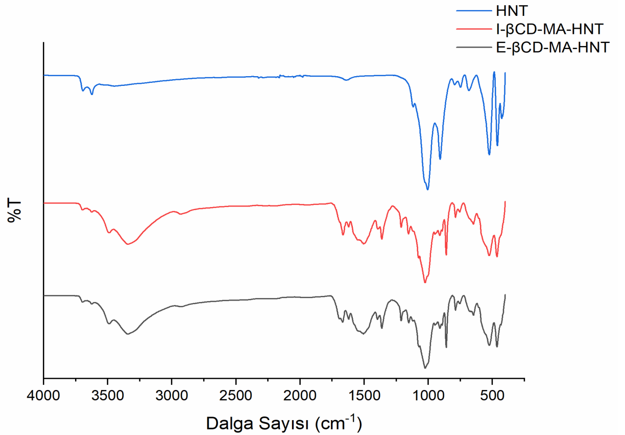
Şekil 4.3. HNT, I- \beta CD-MA-HNT ve E- \beta CD-MA-HNT NS'lere ait FTIR spektrumları
