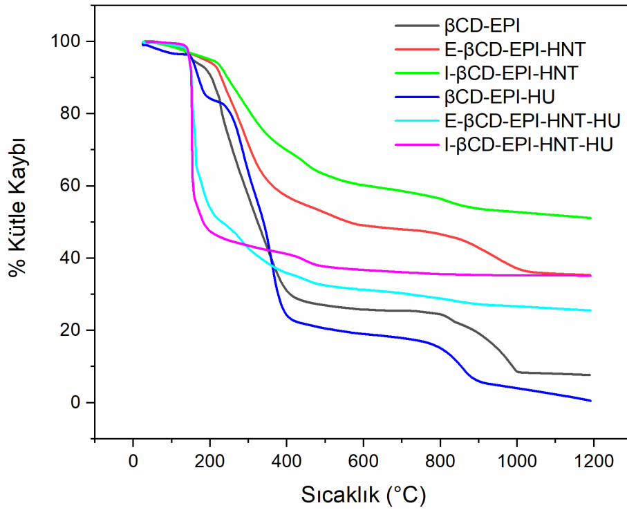
Şekil 4.23. βCD-EPI nanosüngerin, βCD-EPI-HNT nanosünger yapının ve nanosünger-ileç konjüge yapıya ait termogramlar
