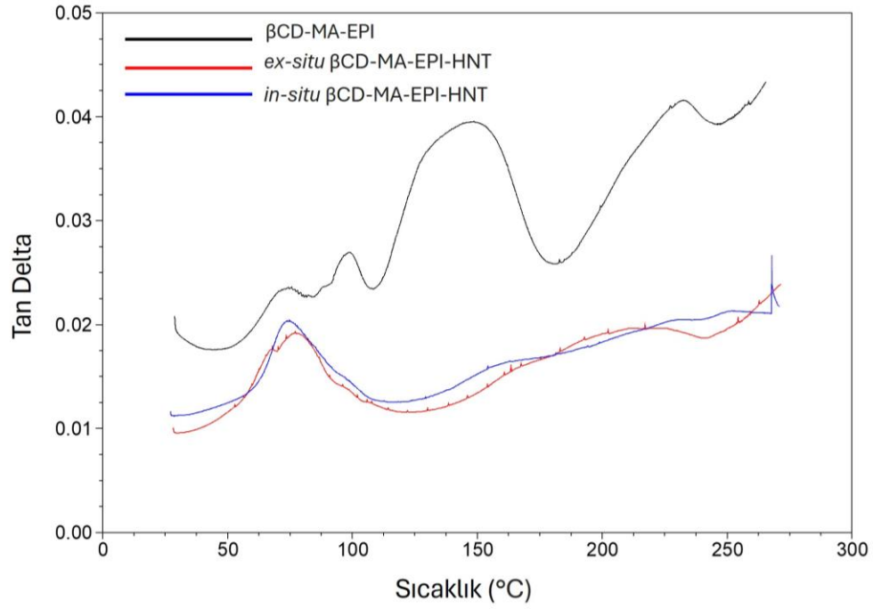
Şekil 4.42. \beta CD-MA-EPI nanosünger yapının ve HNT katkılı nanosünger yapıların Tan \delta -Sıcaklık grafiği.
