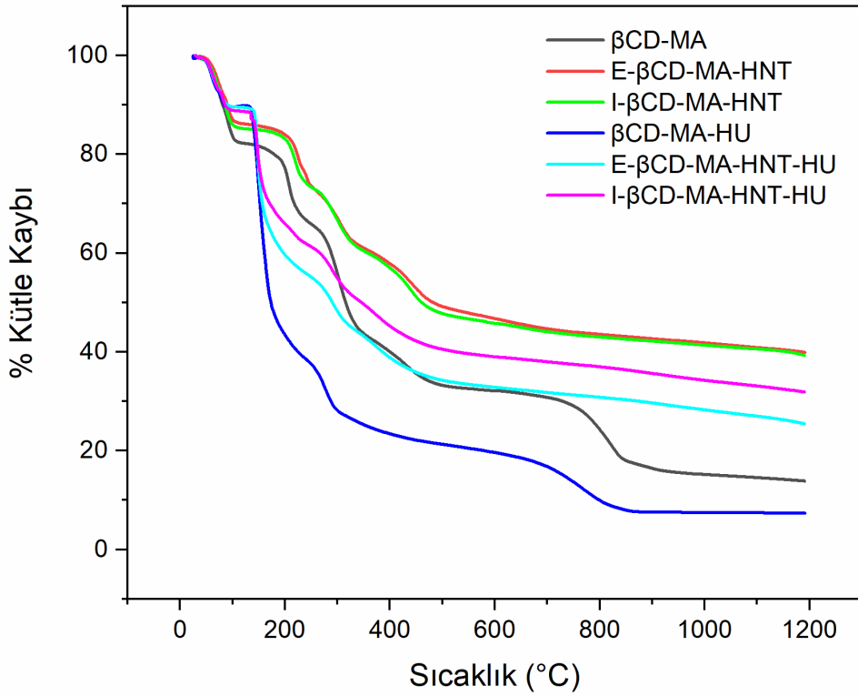
Şekil 4.6. \beta CD-MA NS, HNT katkılı NS ve bu nanosüngerlerin-ilaç konjugatlarının termogramları
