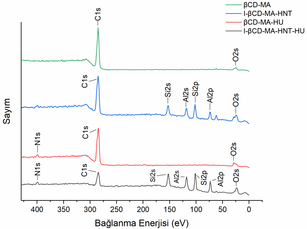
Şekil 4.14. \beta CD-MA nanosünger ve in-situ yöntemle HNT katkılı nanosünger ve nanosünger-ilaç konjugatlarına ait 0-400 eV arası XPS taramasının büyütülmüş hali
