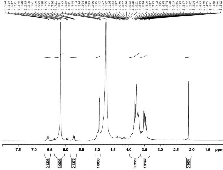
Şekil 4.38. MA-EPI ile sentezlenen \beta CD bazlı nanosüngerlerin ^1\text{H} -NMR spektrumu
