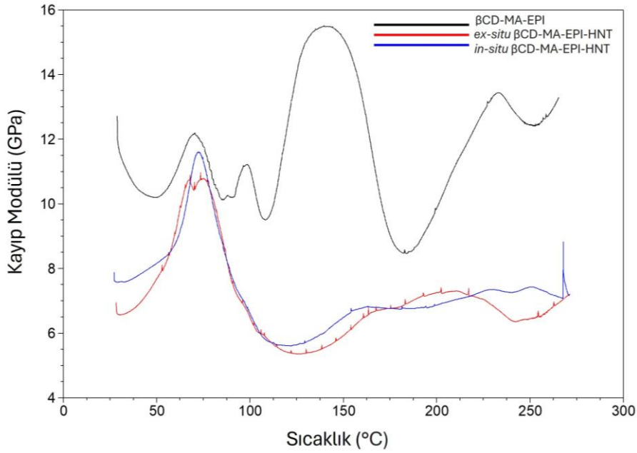
Şekil 4.41. \beta CD-MA-EPI nanosünger yapının ve HNT katkılı nanosünger yapıların Kayıp Modülü (LM) (GPa)-Sıcaklık (°C) grafiği.
