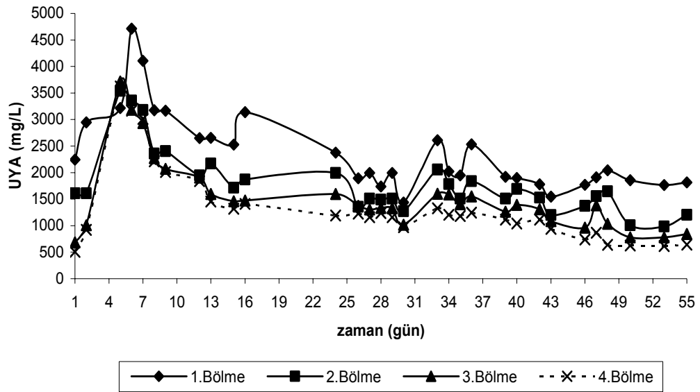
Şekil 4.53. Mezofilik şartlarda 10.2 kg KOİ/m 3 .gün organik yüklemde zamana karşı reaktörün her bir bölmesindeki UYA konsantrasyonları
