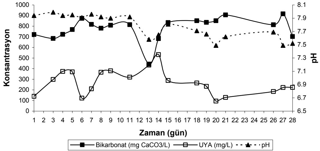
Şekil 4.5. Oda sıcaklığında 0.52 kg KOİ/m 3 .gün organik yükleme hızında zamana karşı çıkış suyu pH değeri, bikarbonat ve UYA konsantrasyonları
