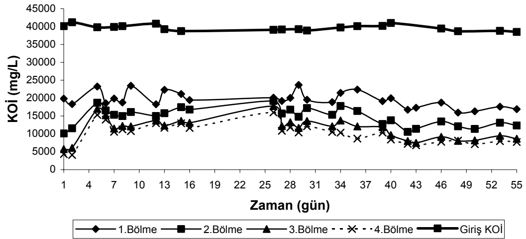
Şekil 4.51. Mezofilik şartlarda 10.2 kg KOİ/m 3 .gün organik yüklemde zamana karşı her bir bölmede KOİ konsantrasyonları
