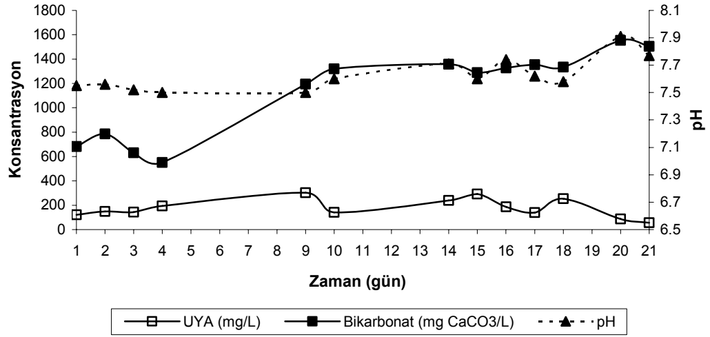
Şekil 4.9. Oda sıcaklığında 0.76 kg KOİ/m 3 .gün organik yüklemeye hızında zamana karşı çıkış suyu pH değeri, bikarbonat ve UYA konsantrasyonları
