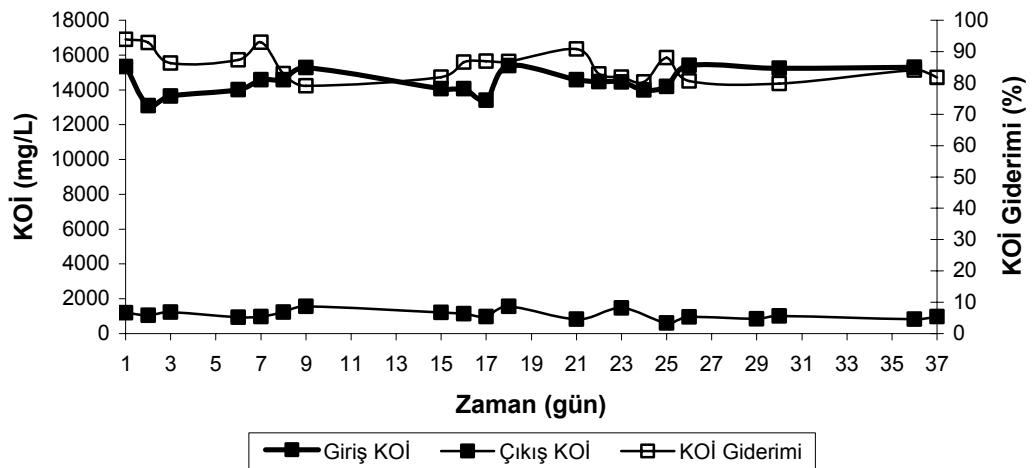
Şekil 4.37. Mezofilik şartlarda 3.8 kg KOİ/m 3 .gün organik yüklemde giriş KOİ, çıkış KOİ ve KOİ giderimi
