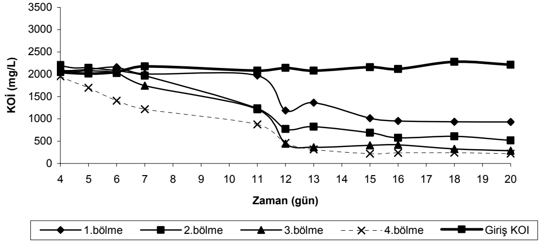
Şekil 4.15. Mezofilik şartlarda 0.52 kg KOİ/m³.gün organik yüklemde zamana karşı her bir bölmede KOİ konsantrasyonları
