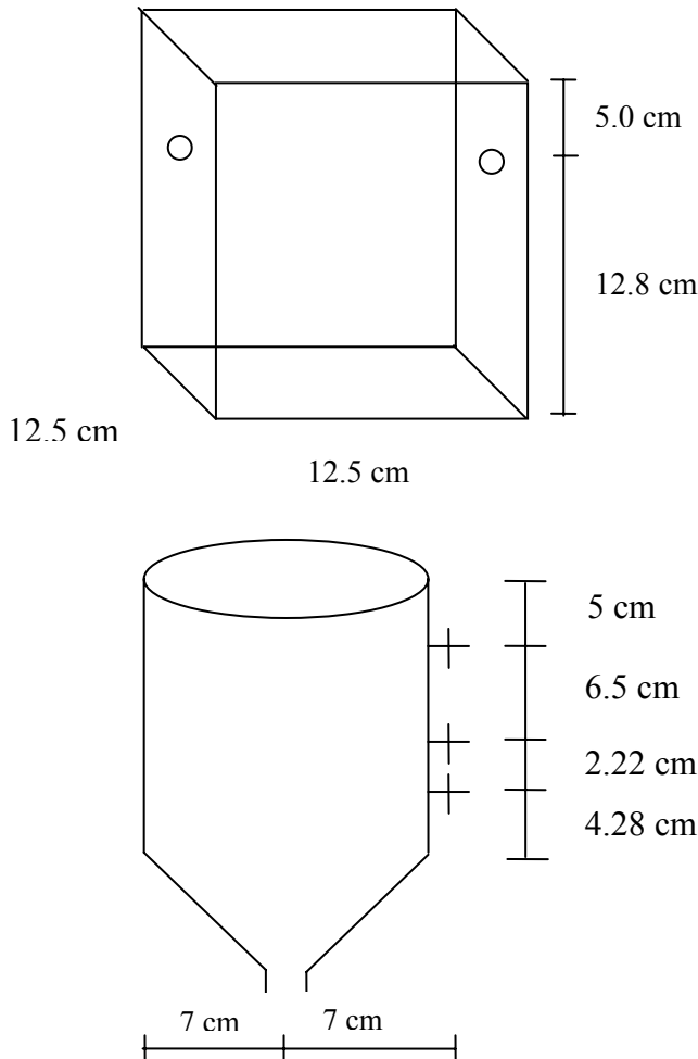
Şekil 3.9. Çalışmada kullanılan Hareketli Yatak Biofilm Reaktör, çökeltme tankı ve boyutları
