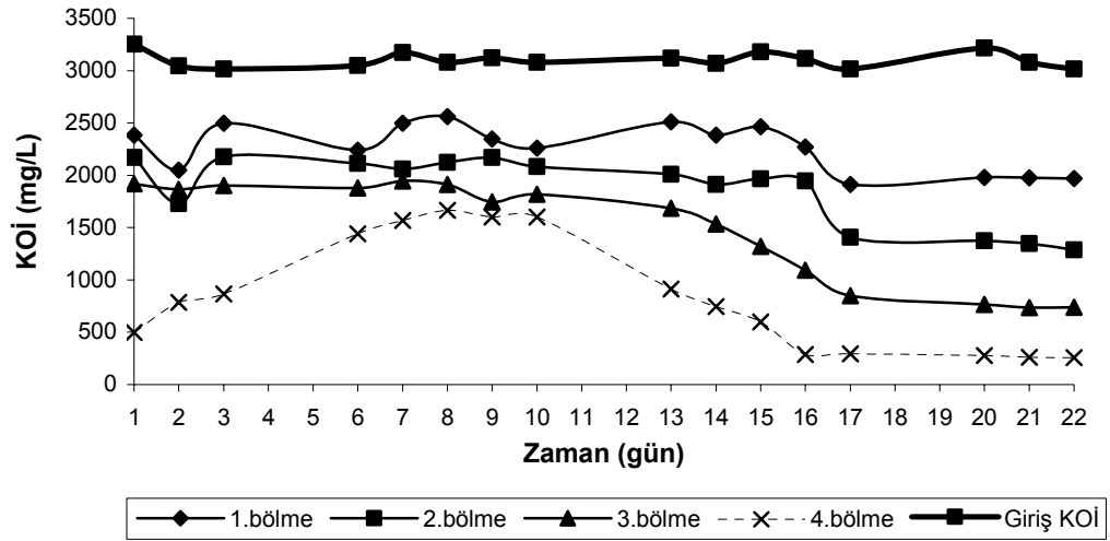
Şekil 4.19. Mezofilik şartlarda 0.76 \text{ kg KOİ/m}^3 .gün organik yüklemde zamana karşı her bir bölmede KOİ konsantrasyonları
