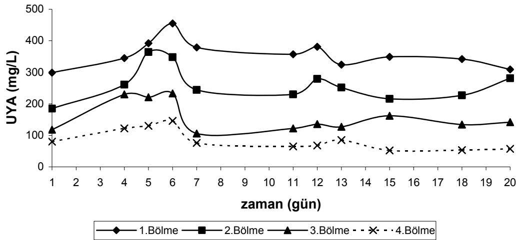
Şekil 4.17. Mezofilik şartlarda 0.52 \text{ kg KOI/m}^3\text{.gün} organik yüklemde zamana karşı reaktörün her bir bölmesindeki UYA konsantrasyonları
