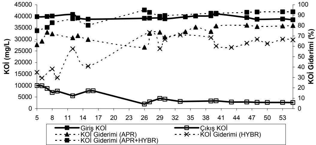
Şekil 4.55. Mezofilik şartlarda 10.2 kg KOİ/m 3 .gün organik yüklemde giriş, çıkış suyu KOİ konsantrasyonları ile APR ve HYBR’de KOİ giderimi (%)
