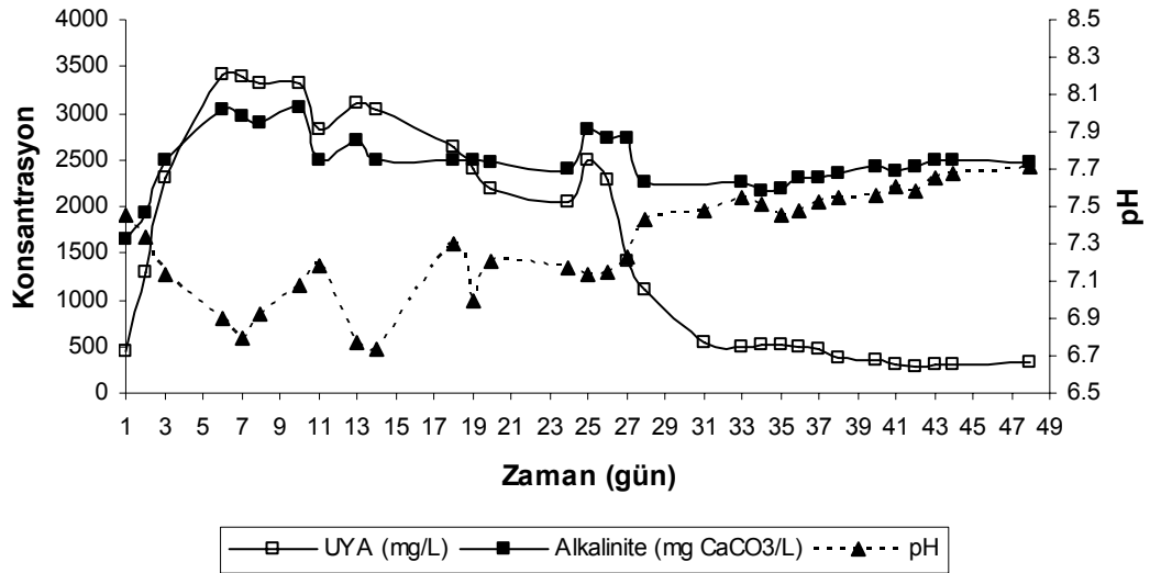
Şekil 4.49. Mezofilik şartlarda 8.32 \text{ kg KOİ/m}^3\text{.gün} organik yüklemde zamana karşı çıkış suyu pH değeri, alkalinite ve UYA konsantrasyonları
