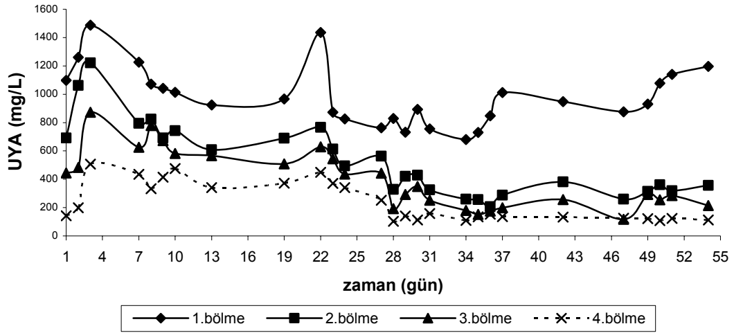
Şekil 4.25. Mezofilik şartlarda 1.05 \text{ kg KOİ/m}^3 .gün organik yüklemde zamana karşı reaktörün her bir bölmesindeki UYA konsantrasyonları
