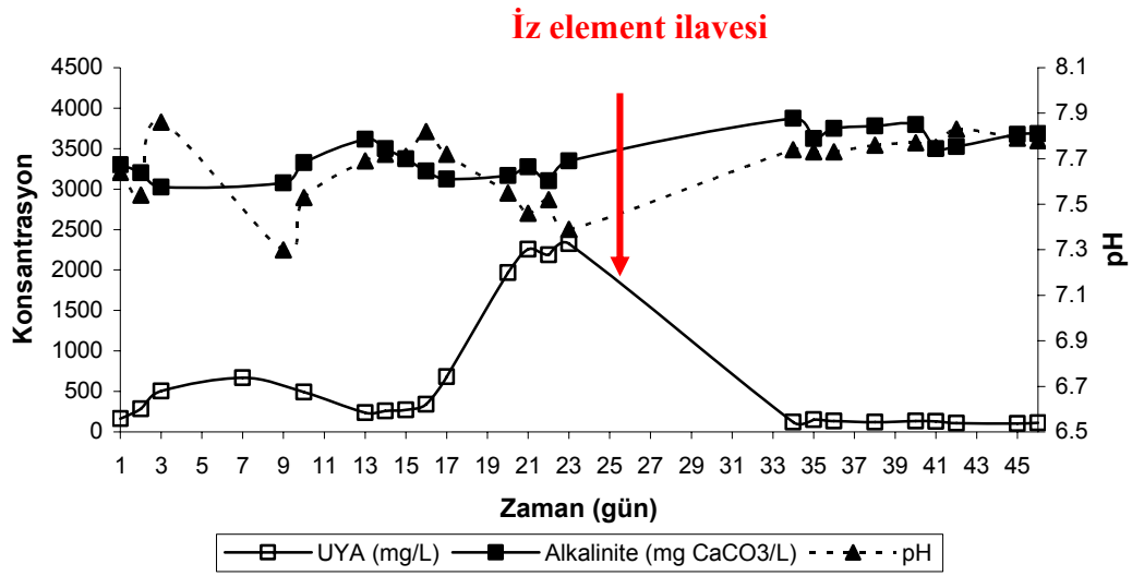
Şekil 4.34. Mezofilik şartlarda 3.12 kg KOİ/m³.gün organik yüklemde zamana karşı çıkış suyu pH değeri, alkalinite ve UYA konsantrasyonları
