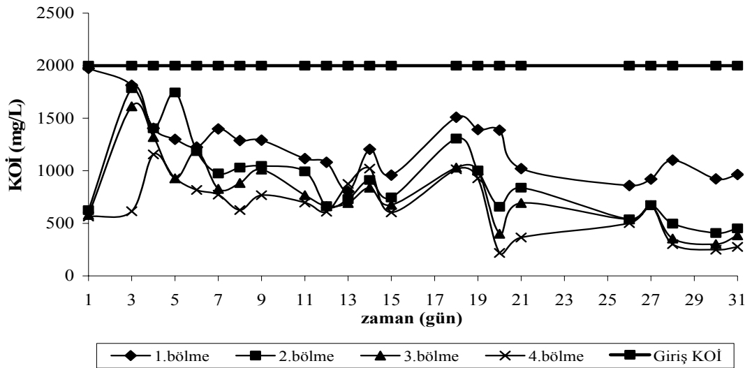
Şekil 4.2. Oda sıcaklığında 0.52 kg KOİ/m 3 .gün organik yüklemeye zamana karşı her bir bölmede KOİ konsantrasyonları
