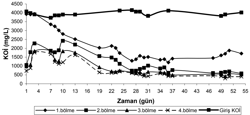
Şekil 4.23. Mezofilik şartlarda 1.05 kg KOİ/m 3 .gün organik yüklemde zamana karşı her bir bölmede KOİ konsantrasyonları
