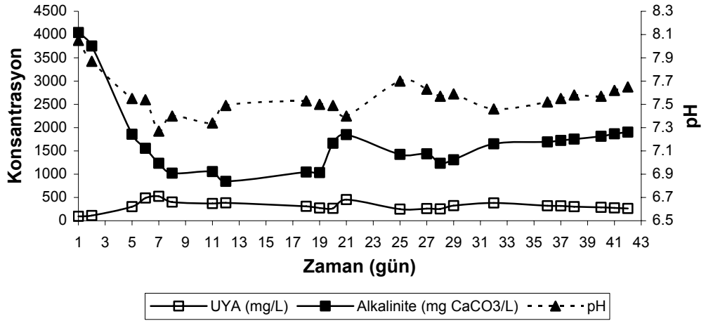
Şekil 4.44. Mezofilik şartlarda 6.5 kg KOİ/m 3 .gün organik yüklemeye zamana karşı çıkış suyu pH değeri, alkalinite ve UYA konsantrasyonları
