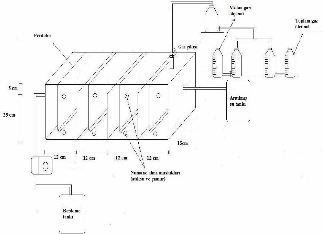
Şekil 3.7. Anaerobik Perdeli Reaktörün şematik olarak işletimi
