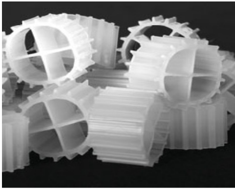
Şekil 3.10. HYBR’de kullanılan taşıyıcı malzeme (biyokütle oluşumu öncesi ve sonrası)
