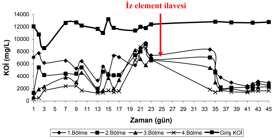
Şekil 4.31. Mezofilik şartlarda 3.12 kg KOİ/m 3 .gün organik yüklemde zamana karşı her bir bölmede KOİ konsantrasyonları
