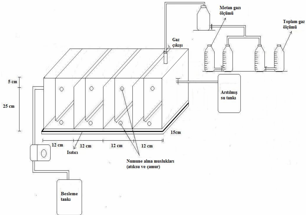
Şekil 3.8. Mezofilik şartlarda işletilen Anaerobik Perdeli Reaktör
