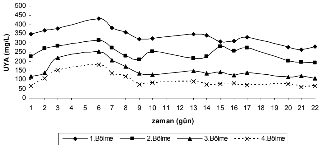
Şekil 4.21. Mezofilik şartlarda 0.76 \text{ kg KOI/m}^3\text{.gün} organik yüklemde zamana karşı reaktörün her bir bölmesindeki UYA konsantrasyonları
