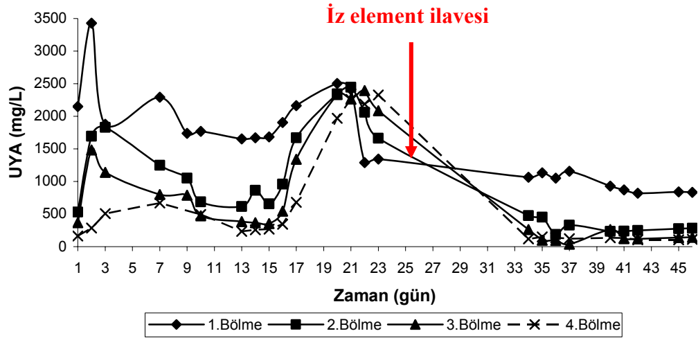
Şekil 4.33. Mezofilik şartlarda 3.12 \text{ kg KOI/m}^3\text{.gün} organik yüklemde zamana karşı reaktörün her bir bölmesindeki UYA konsantrasyonları
