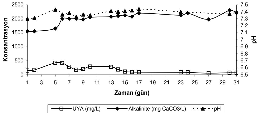
Şekil 4.30. Mezofilik şartlarda 1.62 kg KOİ/m 3 .gün organik yüklemeye zamana karşı çıkış suyu pH değeri, alkalinite ve UYA konsantrasyonları
