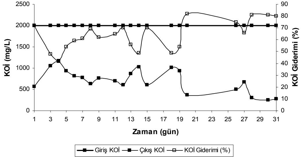
Şekil 4.3. Oda sıcaklığında 0.52 kg KOİ/m 3 .gün organik yüklemde giriş KOİ, çıkış KOİ ve KOİ giderimi (%)
