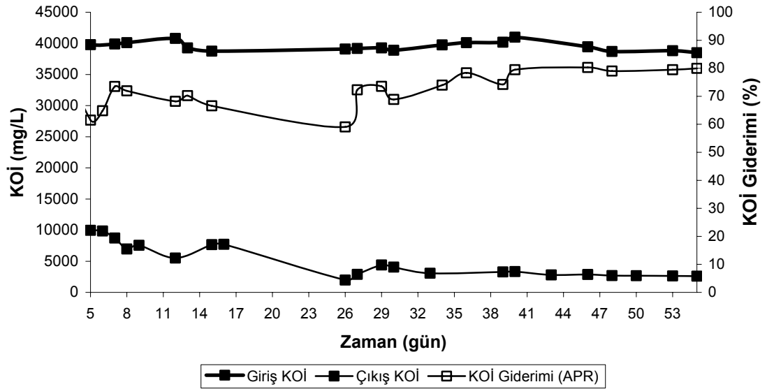
Şekil 4.52. Mezofilik şartlarda 10.2 kg KOİ/m 3 .gün organik yüklemde giriş KOİ, çıkış KOİ ve KOİ giderimi (%)
