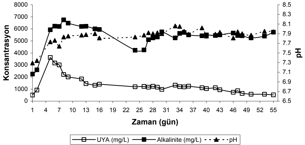
Şekil 4.54. Mezofilik şartlarda 10.2 kg KOİ/m 3 .gün organik yüklemde zamana karşı çıkış suyu pH değeri, alkalinite ve UYA konsantrasyonları
