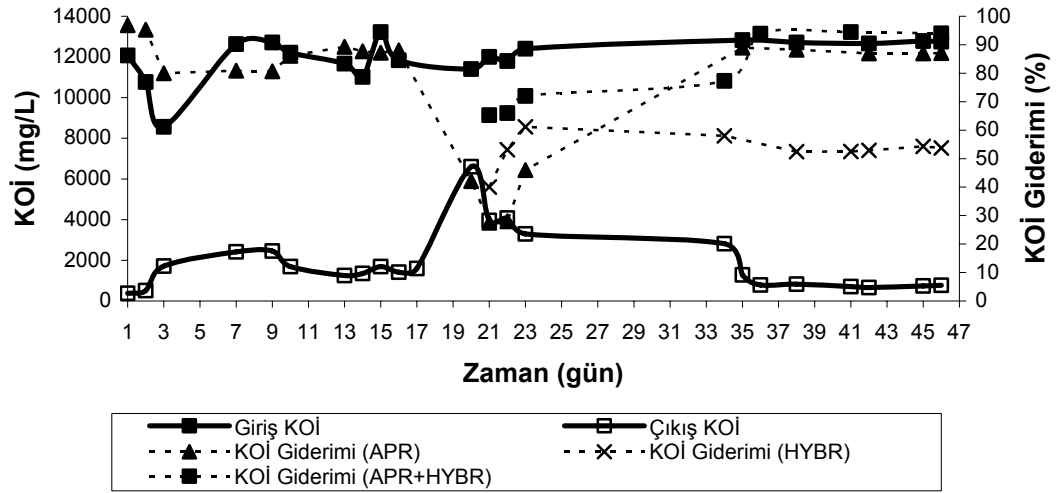
Şekil 4.35. Mezofilik şartlarda 3.12 kg KOİ/m 3 .gün organik yüklemeye giriş, çıkış suyu KOİ konsantrasyonları ile APR ve HYBR'de KOİ giderimi (%)
