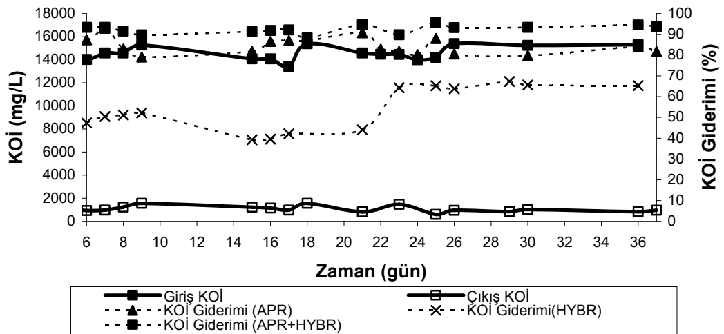
Şekil 4.40. Mezofilik şartlarda 3.8 kg KOİ/m 3 .gün organik yüklemde giriş, çıkış suyu KOİ konsantrasyonları ile APR ve HYBR'de KOİ giderimi (%)
