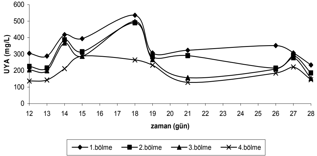
Şekil 4.4. Oda sıcaklığında 0.52 \text{ kg KOİ/m}^3 \cdot \text{gün} organik yükleme hızında zamana karşı reaktörün her bir bölümündeki UYA konsantrasyonları
