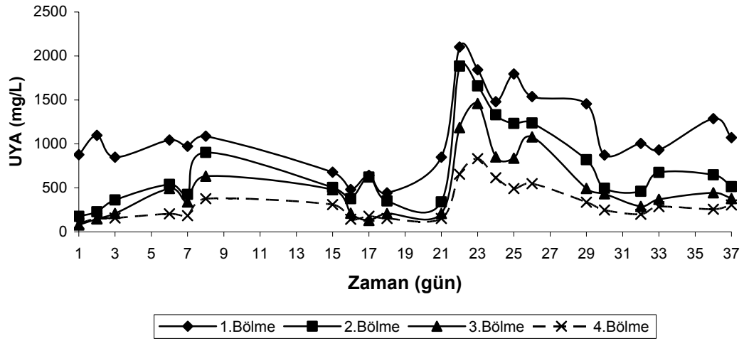
Şekil 4.38. Mezofilik şartlarda 3.8 kg KOİ/m 3 .gün organik yüklemde zamana karşı reaktörün her bir bölmesindeki UYA konsantrasyonları
