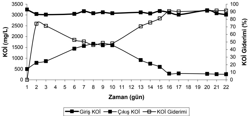
Şekil 4.20. Mezofilik şartlarda 0.76 \text{ kg KOİ/m}^3 .gün organik yüklemde giriş KOİ, çıkış KOİ ve KOİ giderimi (%)
