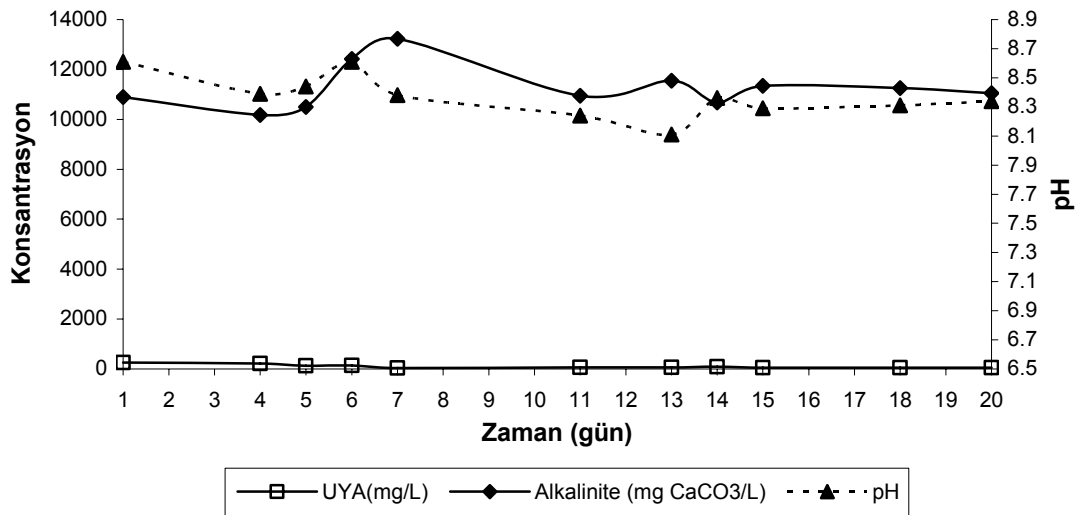
Şekil 4.18. Mezofilik şartlarda 0.52 \text{ kg KOİ/m}^3\text{.gün} organik yüklemde zamana karşı çıkış suyu pH değeri, alkalinite ve UYA konsantrasyonları
