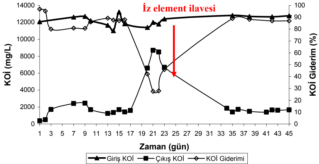
Şekil 4.32. Mezofilik şartlarda 3.12 kg KOİ/m 3 .gün organik yüklemde giriş KOİ, çıkış KOİ ve KOİ giderimi (%)
