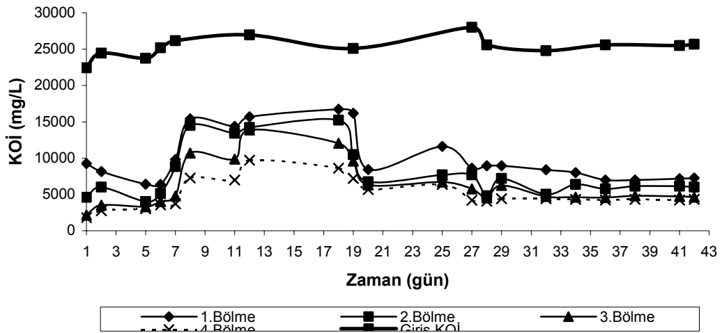
Şekil 4.41. Mezofilik şartlarda 6.5 kg KOİ/m 3 .gün organik yüklemede zamana karşı her bir bölmede KOİ konsantrasyonları
