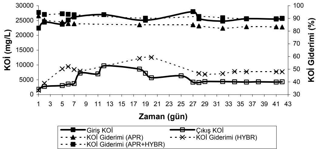
Şekil 4.45. Mezofilik şartlarda 6.5 kg KOİ/m 3 .gün organik yüklemde giriş, çıkış suyu KOİ konsantrasyonları ile APR ve HYBR'de KOİ giderimi (%)
