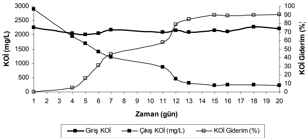
Şekil 4.16. Mezofilik şartlarda 0.52 kg KOİ/m³.gün organik yüklemde giriş KOİ, çıkış KOİ ve KOİ giderimi (%)
