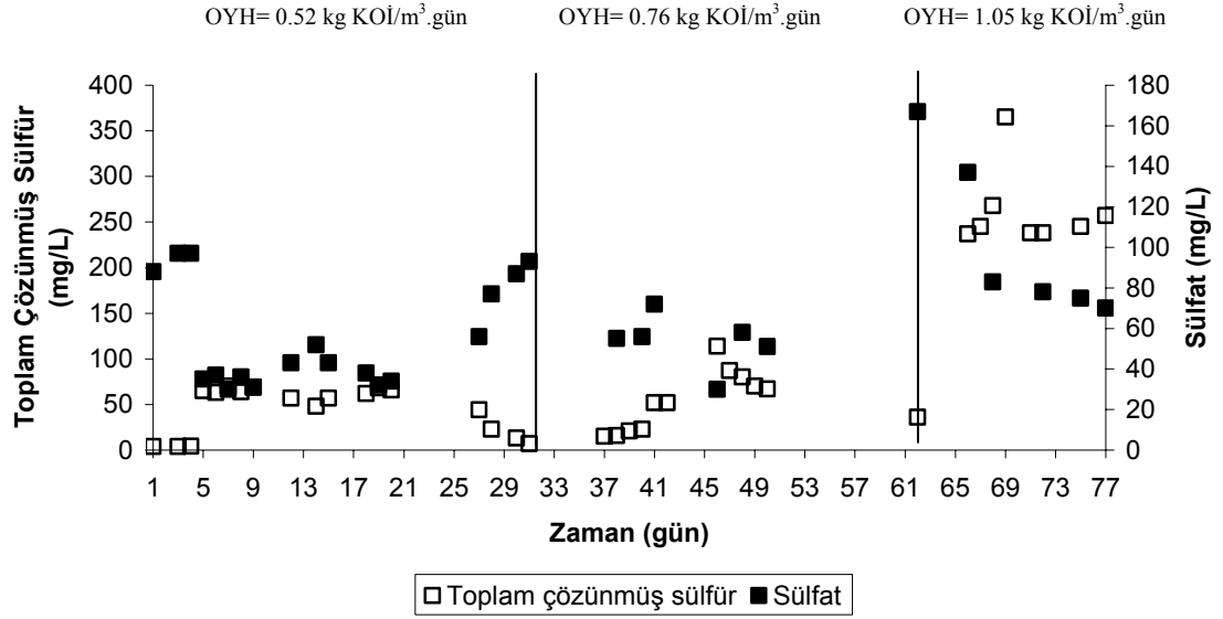
Şekil 4.14. Oda sıcaklığında, artan organik yüklemelerde zamana karşı çıkış suyundaki toplam çözünmüş sülfür ve sülfat konsantrasyonlarının değişimi
