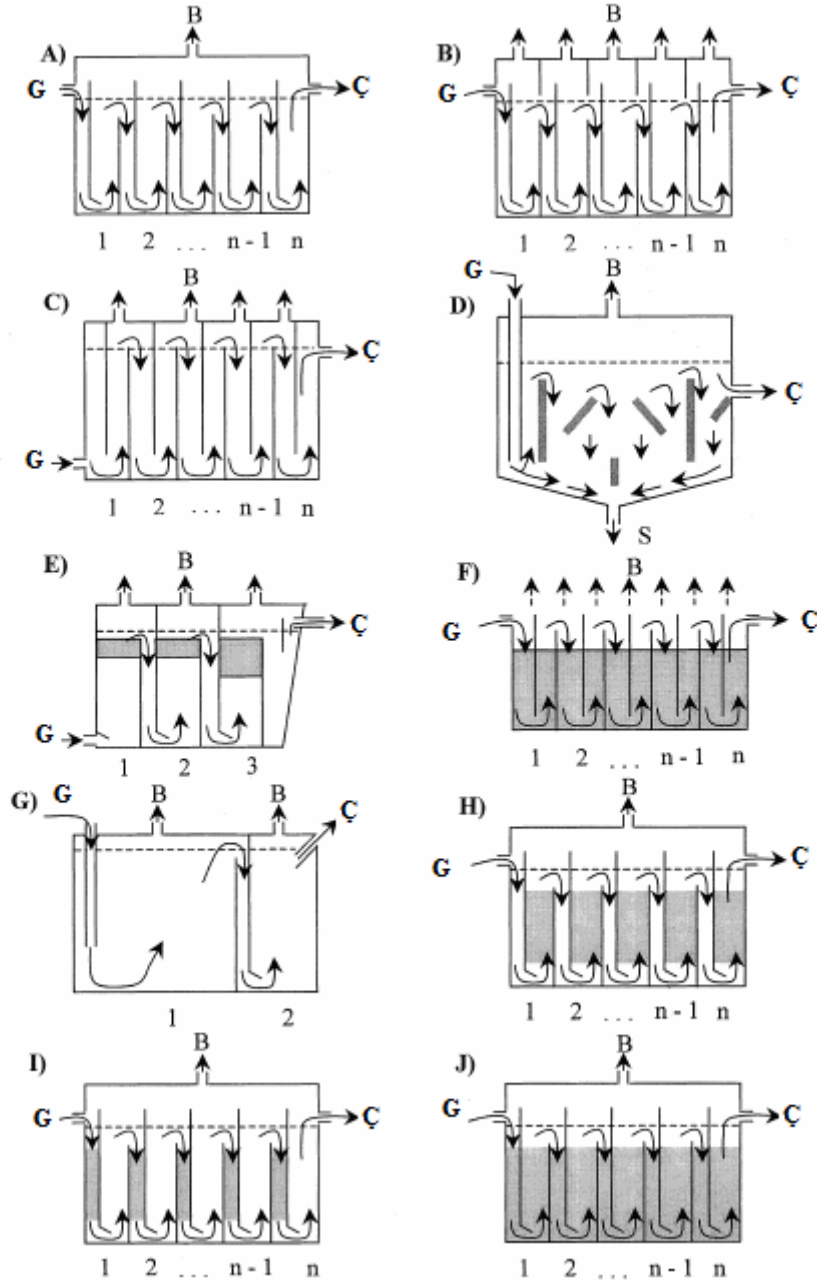
Şekil 2.7. Anaerobik Perdeli Reaktör çeşitleri A) Tek gaz toplama hazneli B) Bölmeli gaz toplama hazneli C) Dikey D) Yatay E) Çökeltme zonlu hibrit reaktör F) Üstü açık G) Genişletilmiş ilk bölmesi H-J arası çeşitli uygulamaları H)yukarı köşeli I) aşağı köşeli J) Bütün reaktör ( G: Atıksu girişi, Ç: Atıksu çıkışı, B: biyogaz, S: Katılar)
