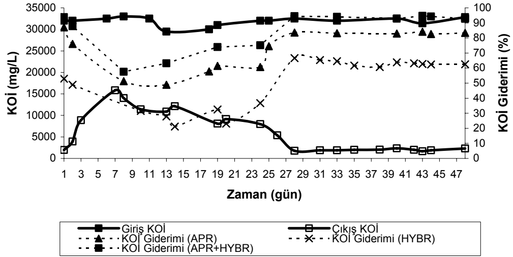
Şekil 4.50. Mezofilik şartlarda 8.32 kg KOİ/m 3 .gün organik yüklemde giriş, çıkış suyu KOİ konsantrasyonları ile APR ve HYBR’de KOİ giderimi (%)
