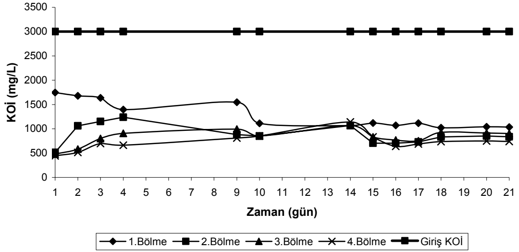
Şekil 4.6. Oda sıcaklığında 0.76 \text{ kg KOİ/m}^3 .gün organik yüklemde zamana karşı her bir bölmede KOİ konsantrasyonları
