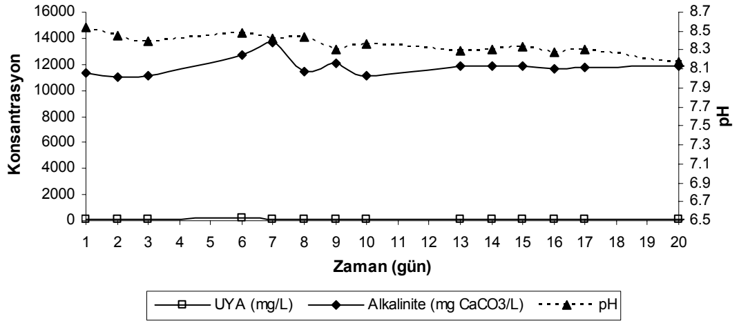
Şekil 4.22. Mezofilik şartlarda 0.76 kg KOİ/m 3 .gün organik yüklemde zamana karşı çıkış suyu pH değeri, alkalinite ve UYA konsantrasyonları
