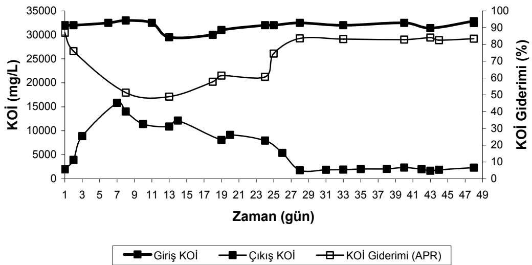
Şekil 4.47. Mezofilik şartlarda 8.32 \text{ kg KOİ/m}^3 \cdot \text{gün} organik yüklemde giriş KOİ, çıkış KOİ ve KOİ giderimi (%)
