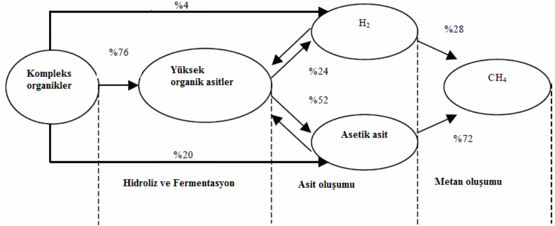
Şekil 2.5. Anaerobik proseslerde enerji akımı
