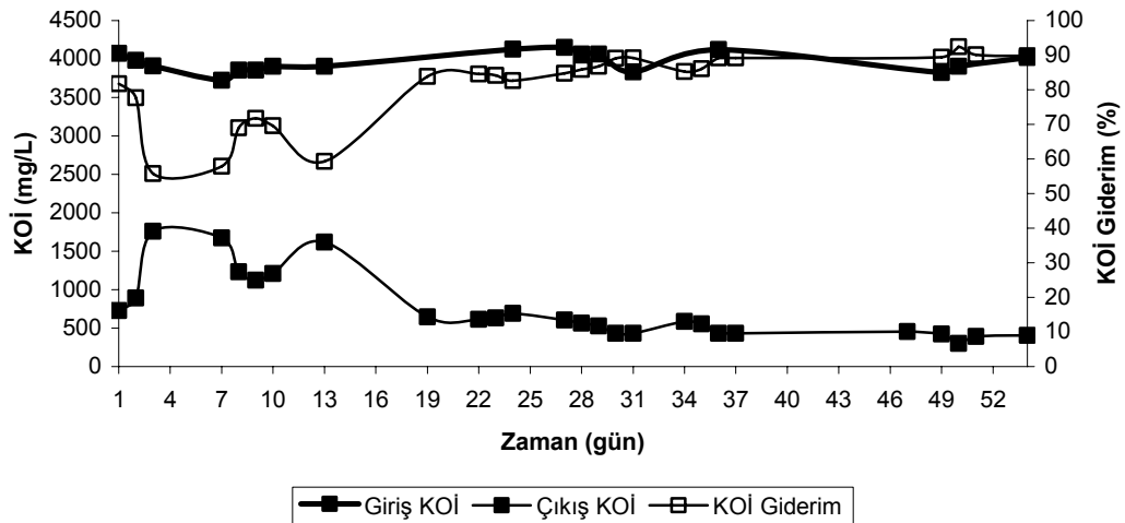
Şekil 4.24. Mezofilik şartlarda 1.05 kg KOİ/m 3 .gün organik yüklemde giriş KOİ, çıkış KOİ ve KOİ giderimi (%)
