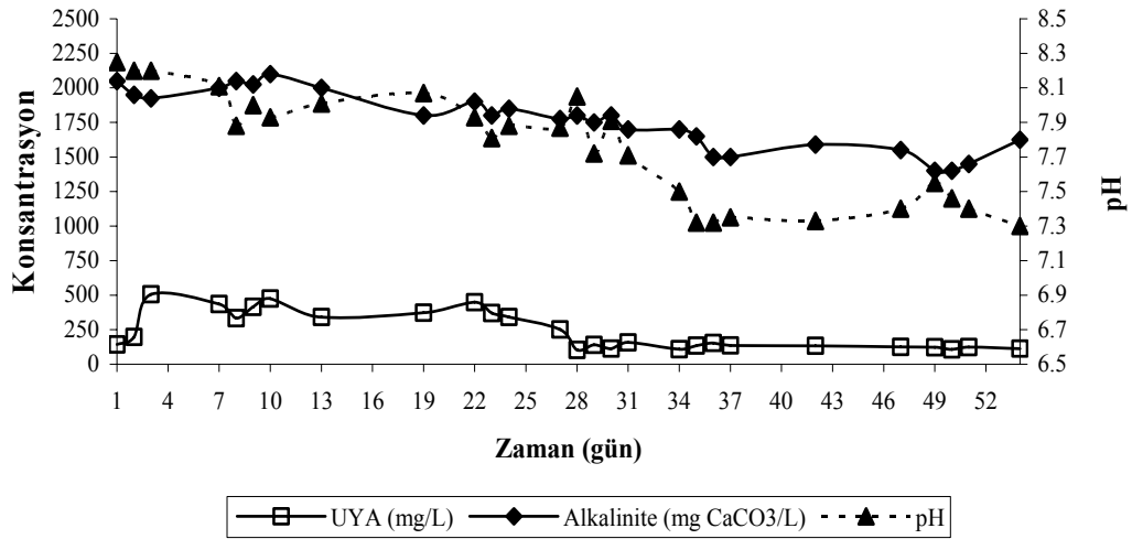
Şekil 4.26. Mezofilik şartlarda 1.05 kg KOİ/m 3 .gün organik yüklemede zamana karşı çıkış suyu pH değeri, alkalinite ve UYA konsantrasyonları
