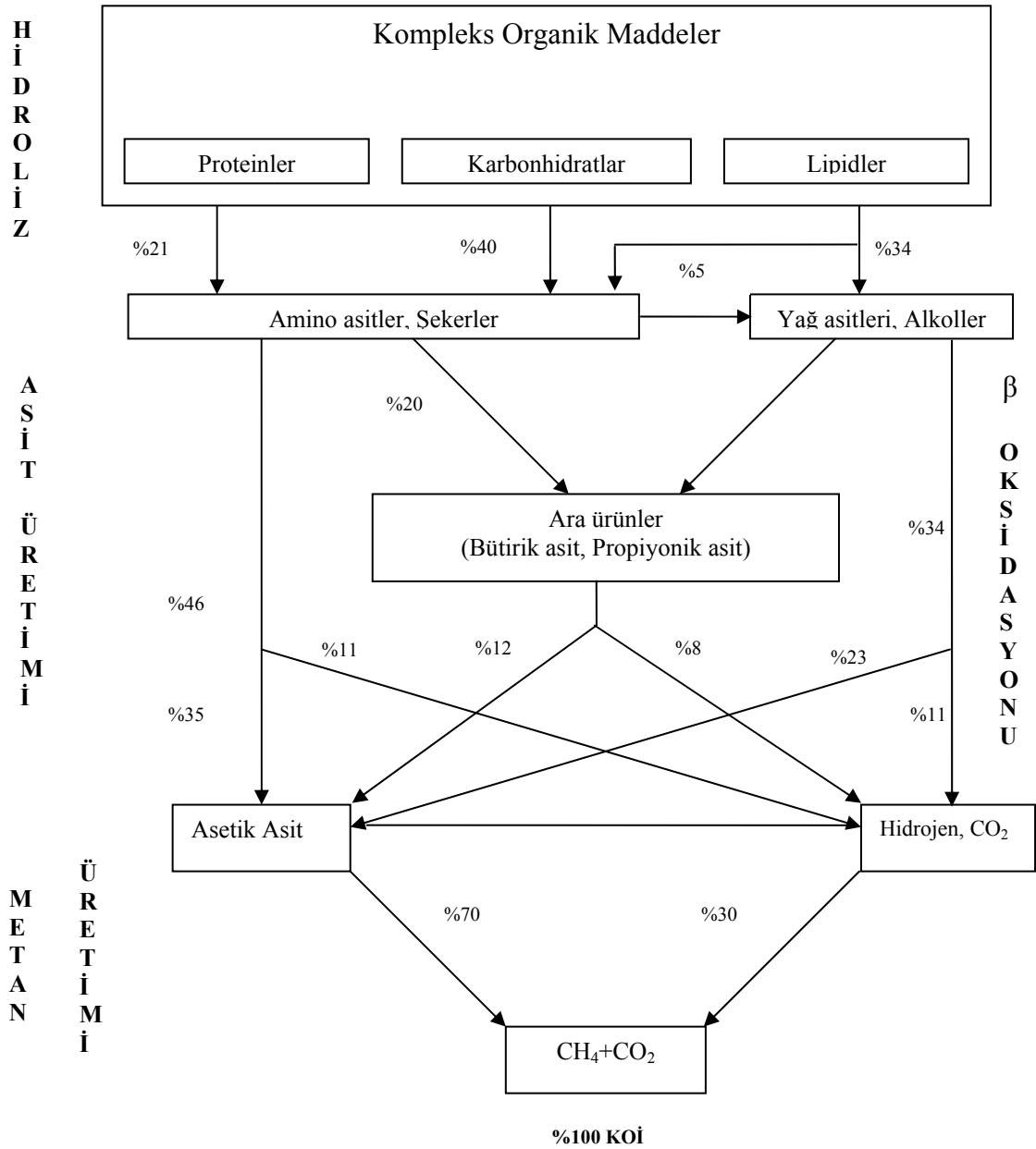
Şekil 2.1. Anaerobik parçalanma prosesi ve metan oluşumu (Anderson ve diğ., 2003)
