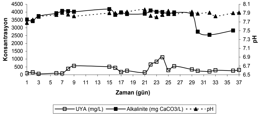
Şekil 4.39. Mezofilik şartlarda 3.8 kg KOİ/m 3 .gün organik yüklemde zamana karşı çıkış suyu pH değeri, alkalinite ve UYA konsantrasyonları
