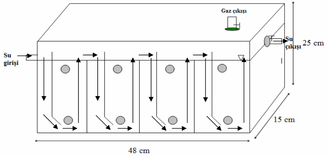
Şekil 3.6. Çalışmada kullanılan Anaerobik Perdeli Reaktör ve boyutları
