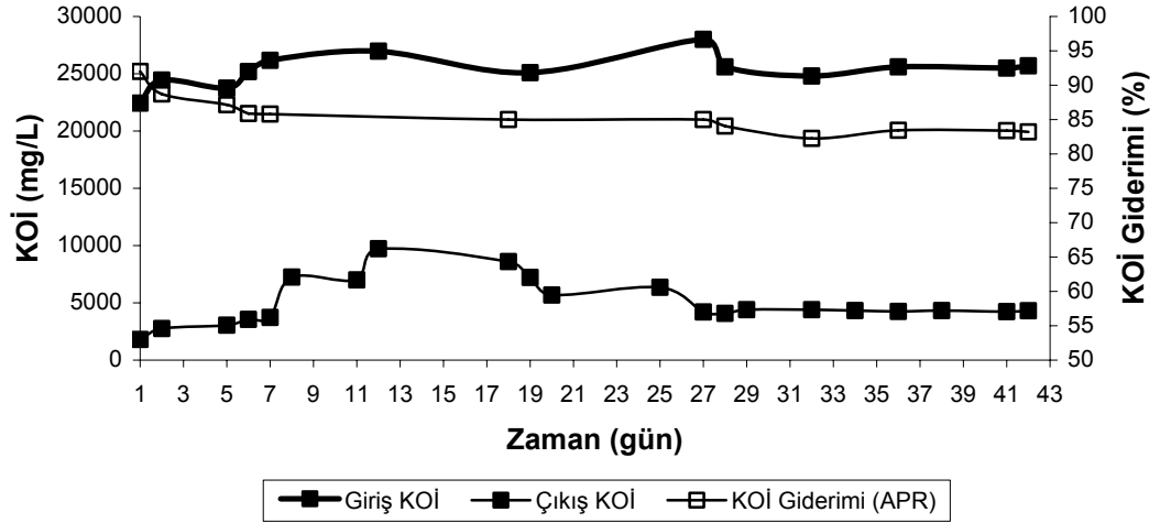
Şekil 4.42. Mezofilik şartlarda 6.5 kg KOİ/m 3 .gün organik yüklemede giriş KOİ, çıkış KOİ ve KOİ giderimi (%)
