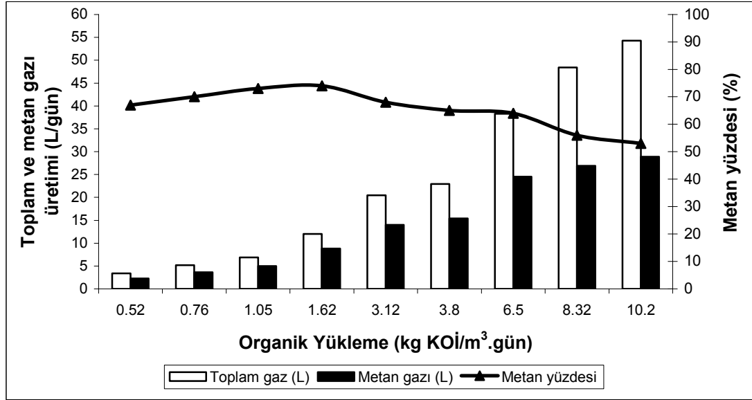
Şekil 4.56. Değişen organik yüklemelerde elde edilen toplam gaz, metan gazı üretim hızları ve metan gazı yüzdesi
