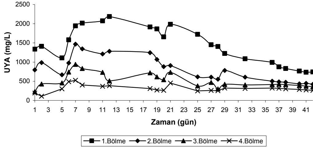
Şekil 4.43. Mezofilik şartlarda 6.5 \text{ kg KOI/m}^3 \cdot \text{gün} organik yüklemde zamana karşı reaktörün her bir bölümündeki UYA konsantrasyonları
