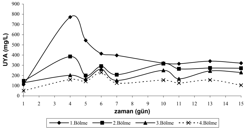
Şekil 4.12. Oda sıcaklığında 1.05 kg KOİ/m 3 .gün organik yüklemde zamana karşı reaktörün her bir bölmesindeki UYA konsantrasyonları
