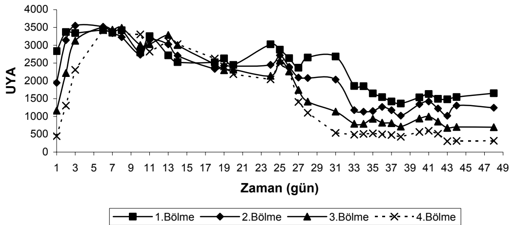
Şekil 4.48. Mezofilik şartlarda 8.32 \text{ kg KOİ/m}^3 \cdot \text{gün} organik yüklemde zamana karşı reaktörün her bir bölmesindeki UYA konsantrasyonları
