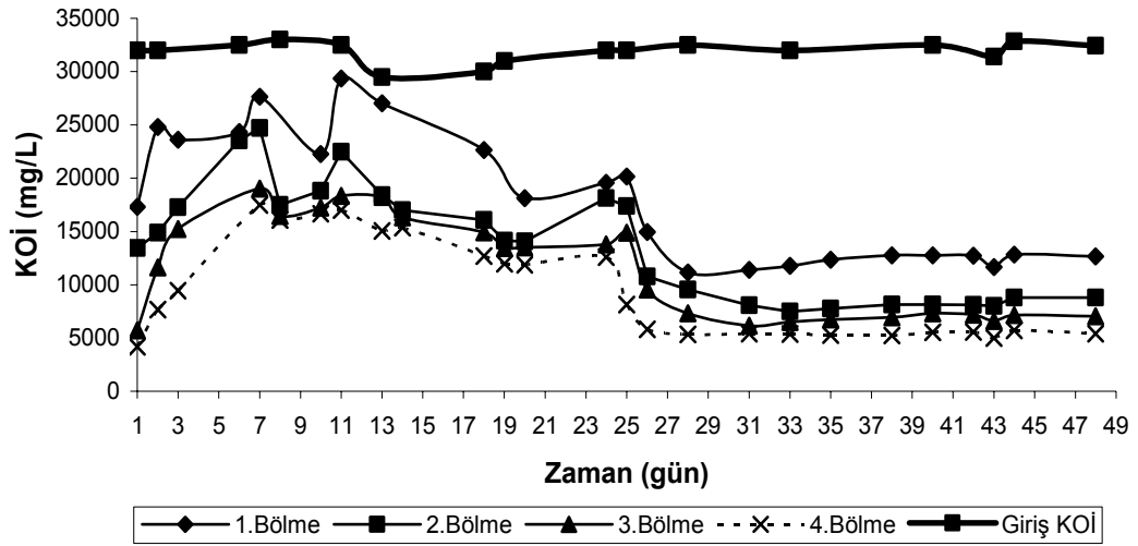
Şekil 4.46. Mezofilik şartlarda 8.32 \text{ kg KOİ/m}^3 \cdot \text{gün} organik yüklemde zamana karşı her bir bölme KOİ konsantrasyonları
