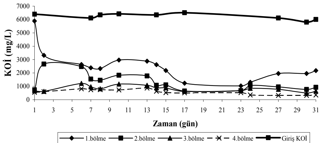
Şekil 4.27. Mezofilik şartlarda 1.62 \text{ kg KOİ/m}^3.\text{gün} organik yüklemede zamana karşı her bir bölmede KOİ konsantrasyonları
