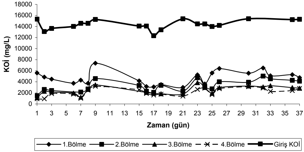
Şekil 4.36. Mezofilik şartlarda 3.8 kg KOİ/m 3 .gün organik yüklemde zamana karşı her bir bölmede KOİ konsantrasyonları
