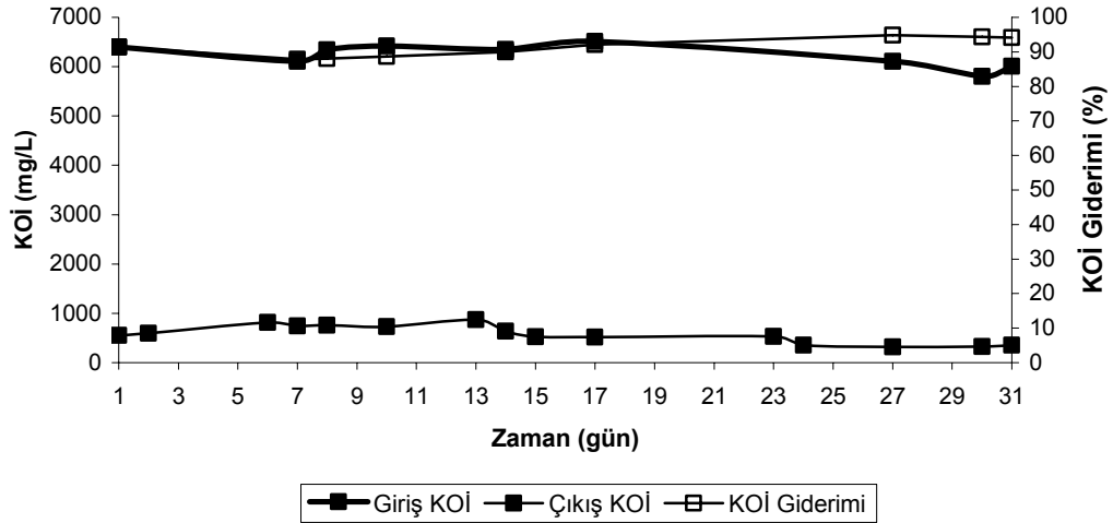
Şekil 4.28. Mezofilik şartlarda 1.62 kg KOİ/m 3 .gün organik yüklemde giriş KOİ, çıkış KOİ ve KOİ giderimi (%)
