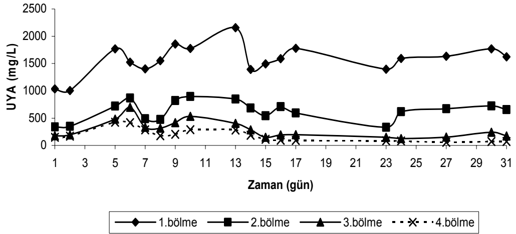
Şekil 4.29. Mezofilik şartlarda 1.62 kg KOİ/m 3 .gün organik yüklemeye zamana karşı reaktörün her bir bölümündeki UYA konsantrasyonları
