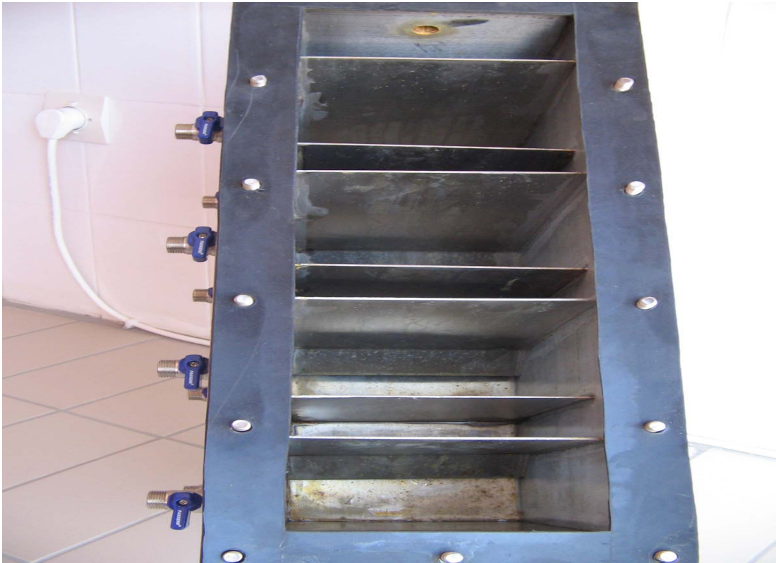
Şekil 3.5. Anaerobik Perdeli Reaktörün üstten görünüşü ve reaktördeki bölmeler
