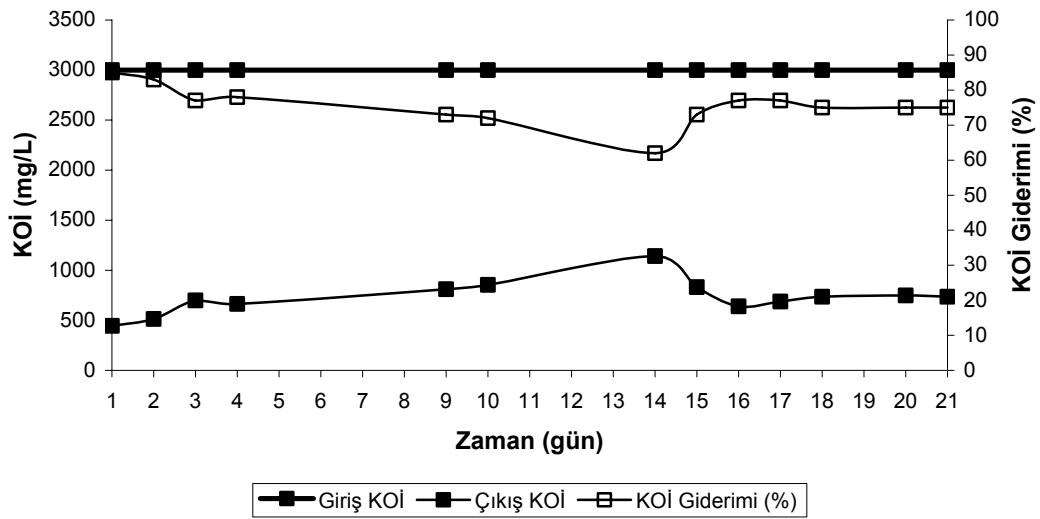
Şekil 4.7. Oda sıcaklığında 0.76 \text{ kg KOİ/m}^3 .gün organik yüklemde giriş KOİ, çıkış KOİ ve KOİ giderimi (%)
